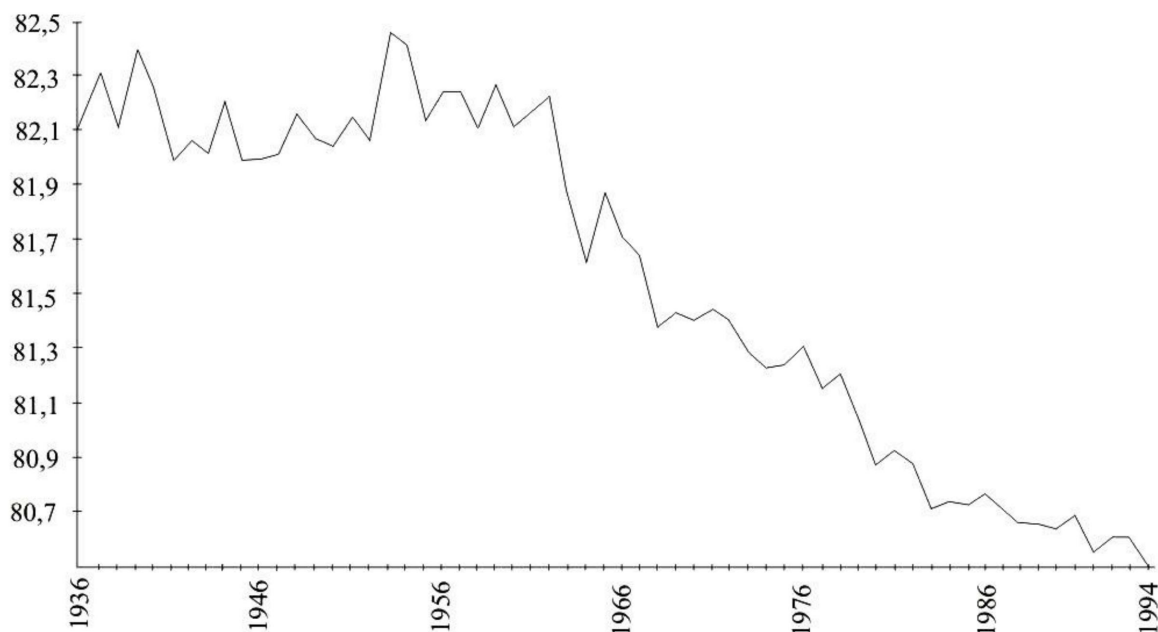
Рисунок 1 – Хронологический график хода уровней, приведенных к условному расходу 360 \text{ м}^3/\text{с} , по р. Белой у г. Уфы
