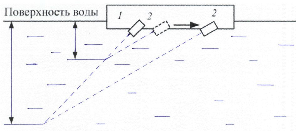
Рис. 2. Изменение положения датчиков для измерений на различной глубине: 1 – передвижная площадка; 2 – ультразвуковые датчики
