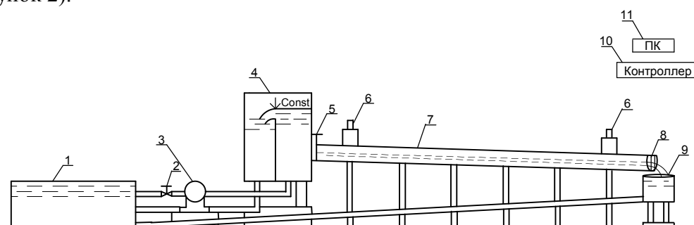
1 – емкость для используемой воды; 2 – задвижка; 3 – насос; 4 – емкость для подачи воды; 5 – затвор; 6 – датчики уровня воды для определения h_1 и h_2 в верхнем и нижнем створах; 7 – труба; 8 – жалюзи; 9 – емкость для сбросной воды; 10 – контроллер для приема и обработки дистанционного сигнала с датчиков уровня воды; 11 – компьютер с программой вычисления расхода воды
