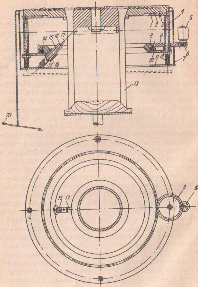
Рис. I. Оборудование для резки гончарных труб с фасками.
