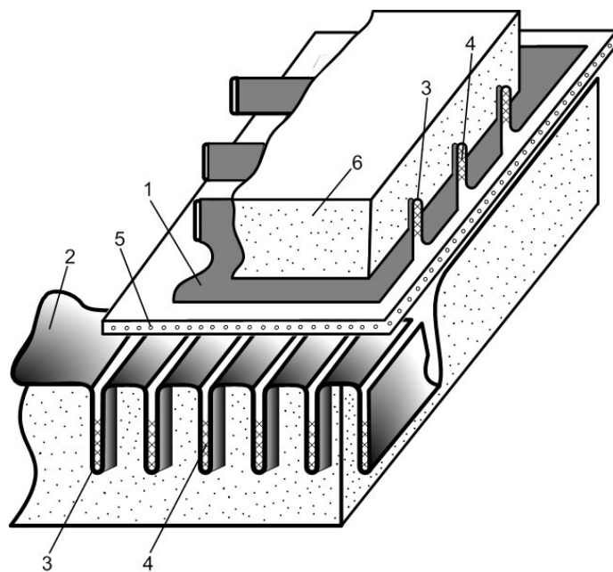
1, 2 – полимерные полотна; 3 – компенсатор деформаций; 4 – антифирикционный состав; 5 – бентонитовые маты; 6 – защитный слой грунта
