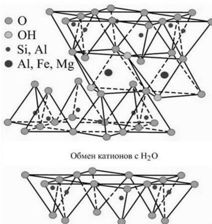
Рисунок 2 – Структура монтмориллонита
