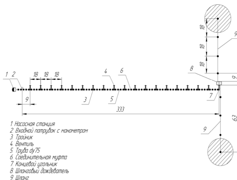
Рисунок 2 - Технологическая схема полива полосовым шланговым дождевателем
