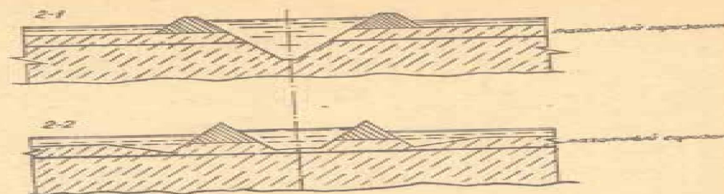
Рис.2. Стыки нарезки продольного оросителя: 1 - катковидным; 2 - валковидным.
