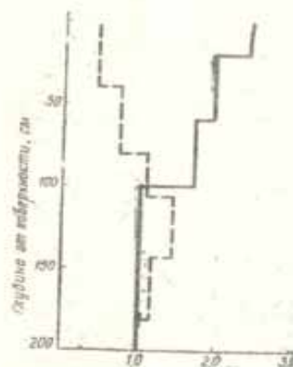
Засоление, плотный остаток (%) — до промывки --- после промывки
