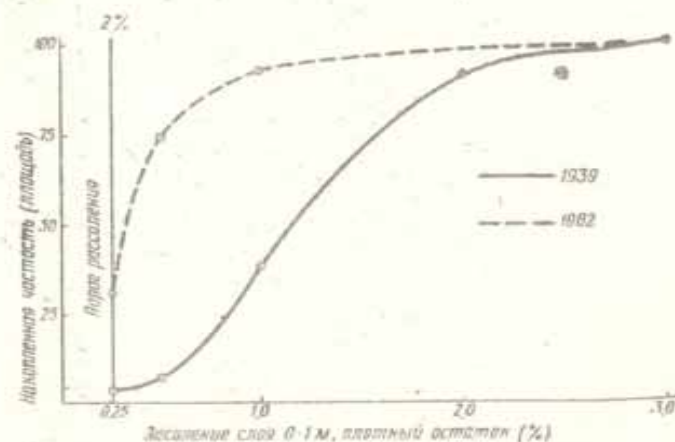
Рис. 2. Кумуляты засоления Покровского участка Северной Мугани Азербайджанской ССР.
