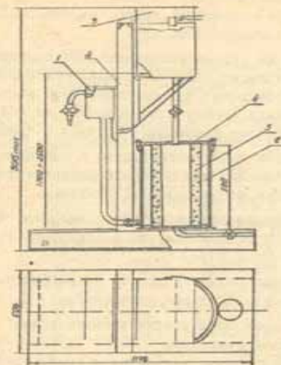
Рис. II, 2. Установка для определения фильтрационных характеристик пористых труб:
