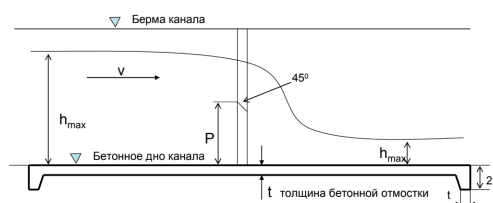
Рис. 3. Гидропост с водосливом Чиполетти.
