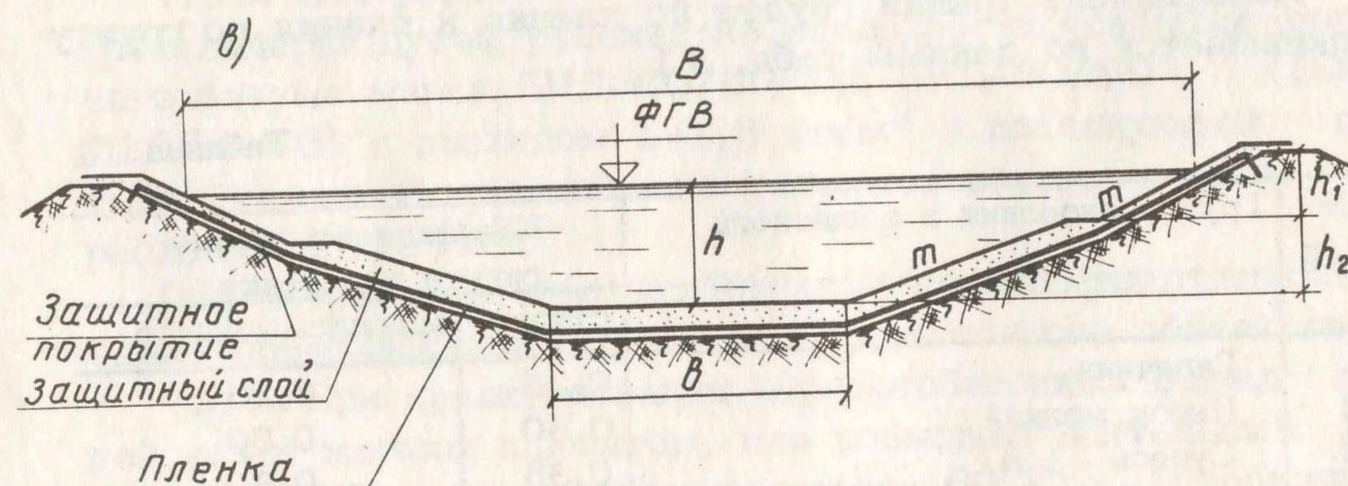
Схемы устройства экранов из пленки: а — траншейная; б — периметрическая; в — комбинированная
