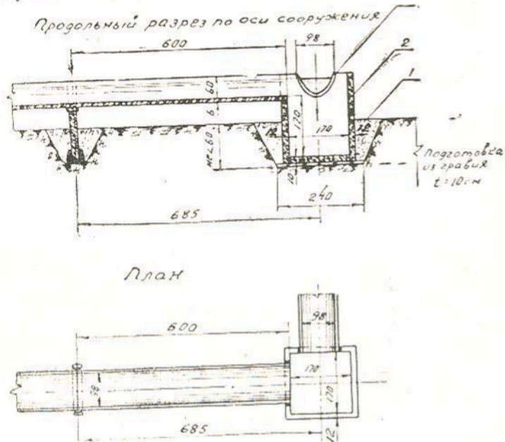
Рис. 13. Поворотное сооружение (на 90°) 1— нижний блок; 2— верхний блок; 3— лоток
