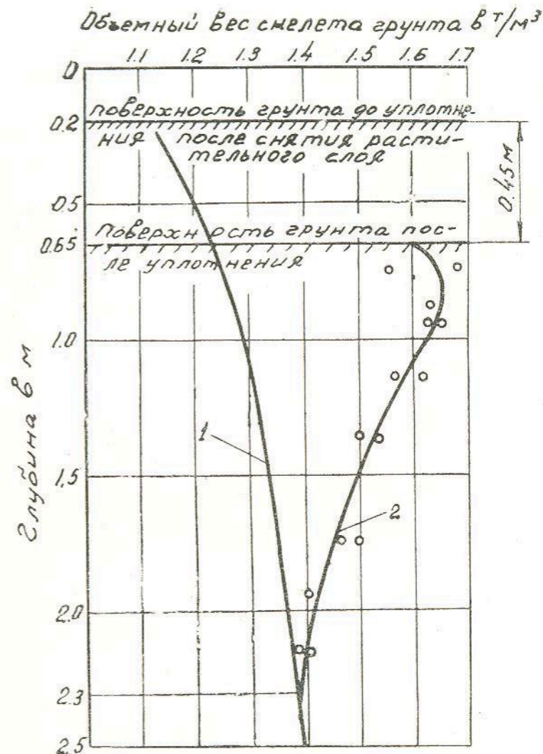
Рис. 5. Распространение уплотнения грунта по глубине в результате трамбования (высота падения трамбовки — 4 м; удельное статическое давление -0,45 \text{ кг/см}^2 ) 1 — объемный вес скелета грунта в естественном залегании 2 — объемный вес скелета грунта после уплотнения 4-мя ударами.
