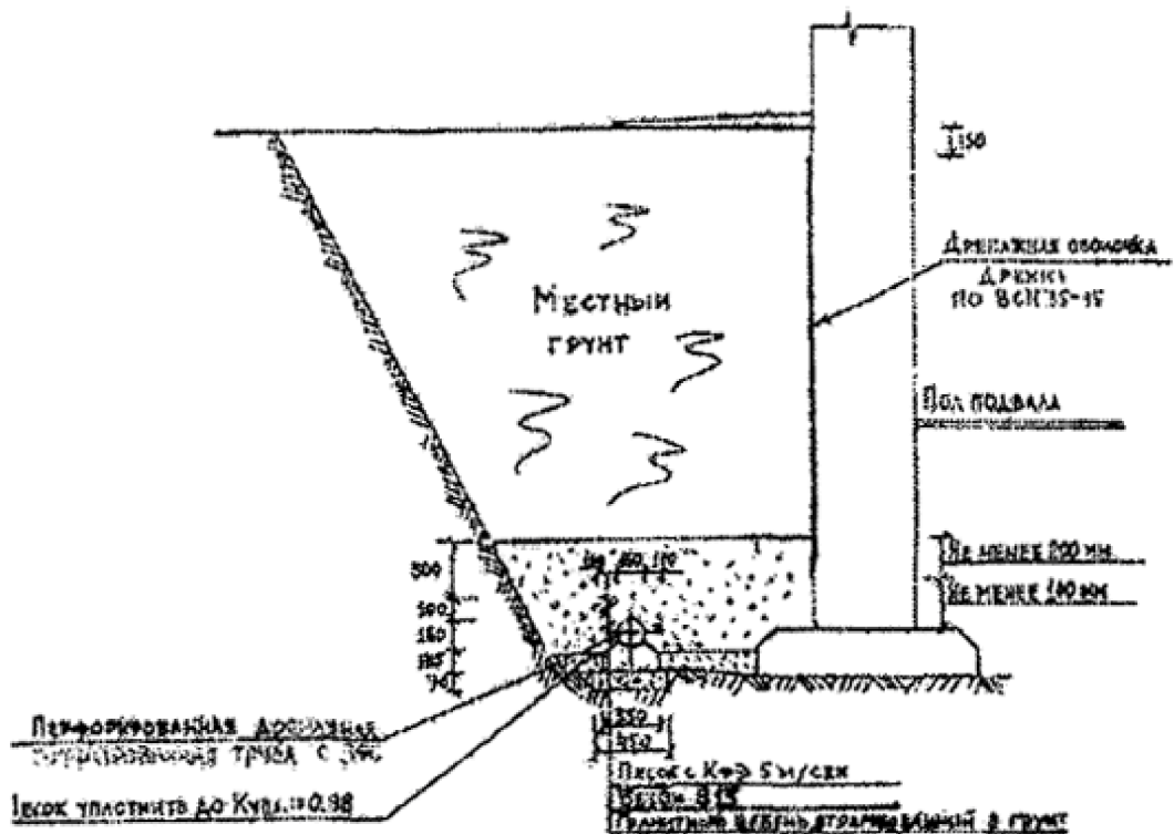
Рис. 8. Принципиальная конструктивная схема пристенного дренажа
