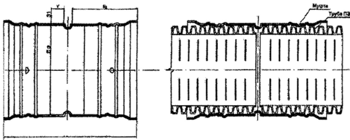
Рис. 4. Муфтовое соединение дренажных труб
