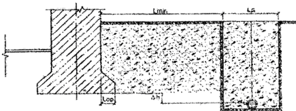
Рис. 6. К определению безопасного расстояния дренажной траншеи от контура заглубленной части (фундамента) сооружения
