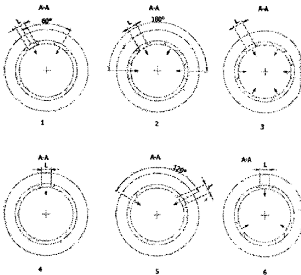
Рис. 3. Схема расположения пропилов в дренажных трубах
