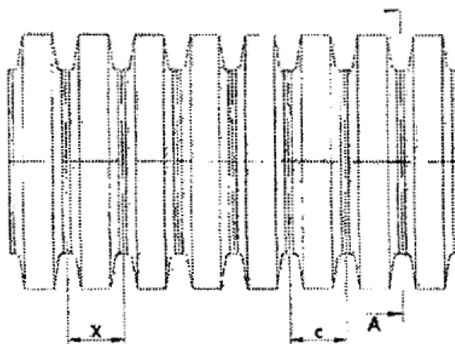
Рис. 1. Двухслойная полиэтиленовая гофрированная труба
