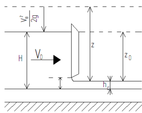
Рис. 4. Расчетная схема истечения из-под затвора “под уровень”
