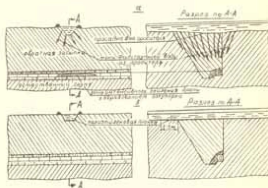
Схема прохождения оросителя через дренаж: а - неправильно; б - правильно.
