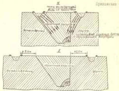
Схема прохождения оросителя параллельно дренам: а - неправильно; б - правильно.
