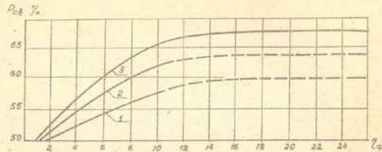
Рис. 2. График зависимости процентного содержания оводобру- зующих частиц от коэффициента неоднородности грунта.
