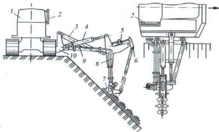
Рис. 1.20. Схема косилки PP-41: 1 – базовый трактор; 2 – защитный экран; 3, 4, 5 – гидроцилиндры стрелы, рукояти, подъема рабочего органа; 6 – механизм подвески; 7 – рабочий орган с приводом; 8 – рукоять; 9 – стрела; 10 – охватывающая рама каналаочистителя
