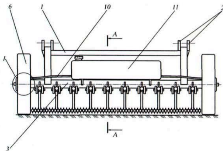
Рис. 3.87. Орудие для нанесения арборицидной смеси на пни:
