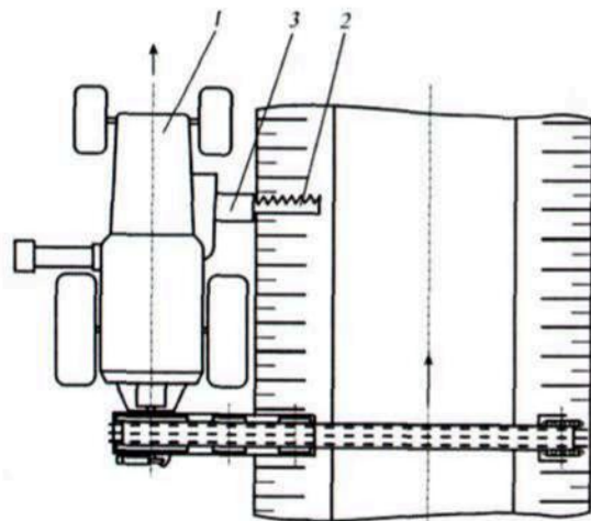
Рис. 3.97. Машина для очистки каналов от растительности:
