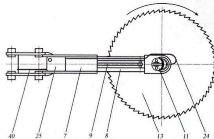
Рис. 3.16. Рабочее оборудование кустореза на базе одноковшового экскаватора, вид сверху: 7 – телескопическая стрела; 8 – телескоп; 9 – гидроцилиндр; 11 – гидромотор; 13 – дисковая пила; 24 – трубопровод; 25 – емкость для арборицидной смеси; 40 – гибкий трубопровод
