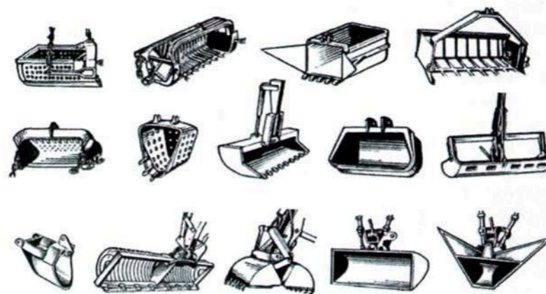
Рис. 1.72. Ковшовые рабочие органы одноковшовых экскаваторов
