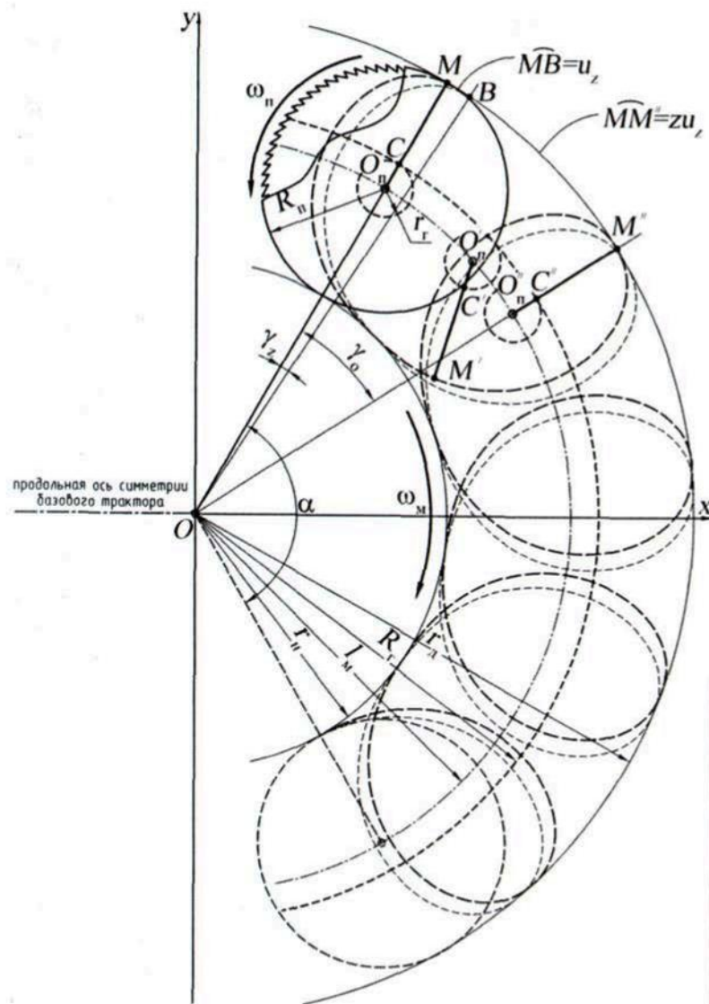
Рис. 3.30. Схема для определения траектории движения зуба пилы маятниковго кустореза
