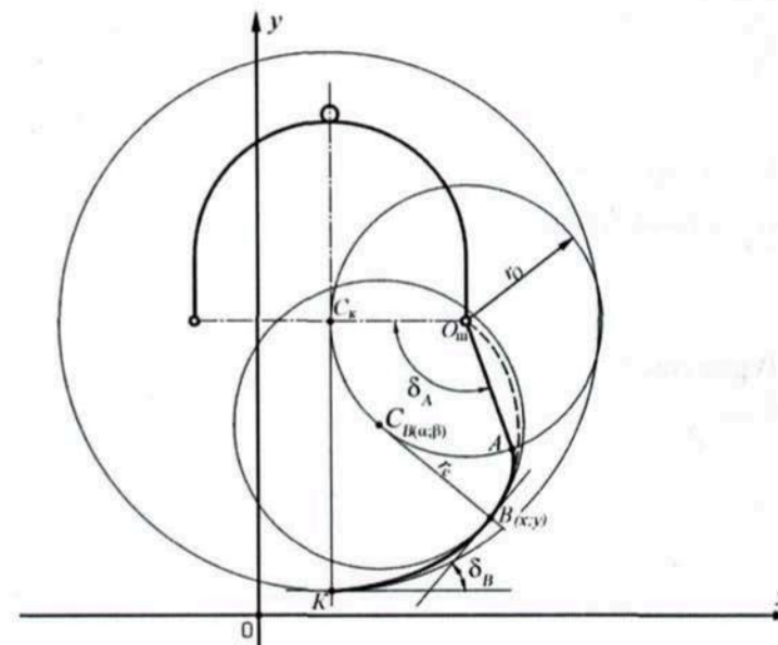
Рис. 3.77. Положение зубьев на начальном этапе подъема ствола
