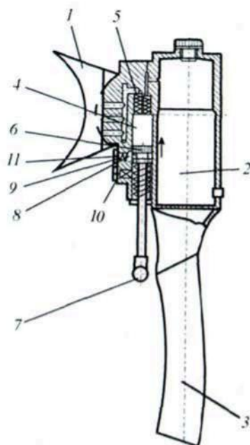
Рис. 1.70. Топор-инъектор: 1 – лезвие; 2 – обух-резервуар; 3 – рукоять; 4 – дозировочная емкость; 5 – блок клапанов; 6 – подпружиненный поршень; 7 – рукоять взвода; 8 – стопор; 9 – пружина; 10 – прорези; 11 – гнездо
