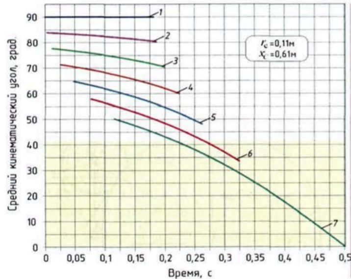
Рис. 3.39. Изменение среднего кинематического угла встречи во времени в зависимости от смещения центра ствола по оси y :
