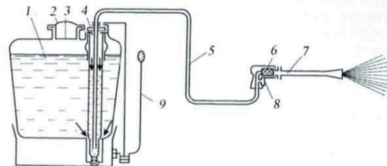
Рис. 1.66. Опрыскиватель ручной ранцевый ОРР-1 «Эра-1»: 1 – резервуар для рабочей жидкости; 2 – заливная горловина; 3 – фильтр; 4 – крышка; 5 – шланг; 6 – брандспойт; 7 – распылитель; 8 – запорное устройство; 9 – ручной насос
