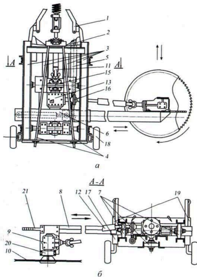
Рис. 3.10. Кусторез КН-1(СГАУ) с механическим приводом: а – вид сверху; б – сечение А-А: 1 – система навески трактора; 2 – рама навески; 3 – направляющие бруссы; 4 – тяги; 5 – гидроцилиндр; 6 – тележка; 7 – катки; 8 – стрела; 9 – редуктор; 10 – дисковый пильный рабочий орган; 11, 12 – телескопические карданные передачи; 13 – промежуточный редуктор; 15 – упругая муфта; 16 – предохранительная муфта; 17 – направляющие втулки; 18 – опорные колеса; 19 – гидроцилиндры; 20 – кожух; 21 – пружинная лапка
