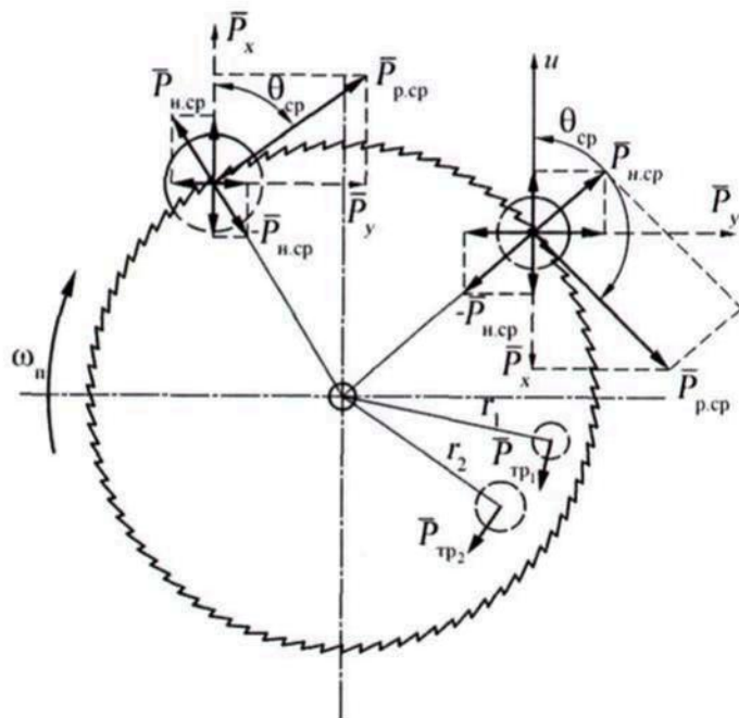
Рис. 3.48. Силы, действующие на рабочий орган кустореза
