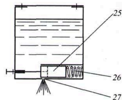
Рис. 3.5. Схема работы клапанов для подачи арборицидной смеси, смонтированных в толкающем брус: 25 – пластина; 26 – возвратная пружина; 27 – сопло
