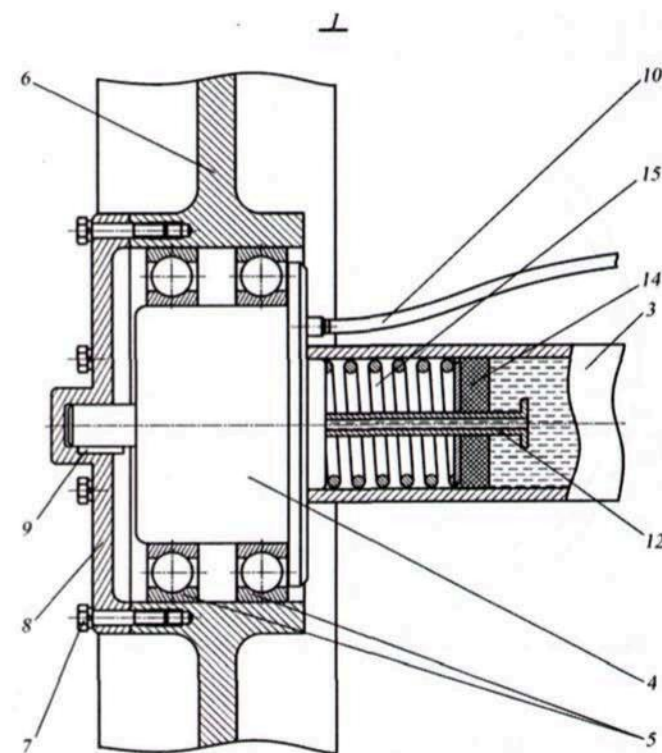
Рис. 3.88. Узел орудия для нанесения арборицидной смеси на пни (узел 1 на рис. 3.87): 3 – полая ось; 4 – гидронасос; 5 – подшипники; 6 – опорное колесо; 7 – болтовое соединение; 8 – крышка; 9 – шпонка; 10 – магистраль; 12 – перепускная трубка; 14 – поршень; 15 – пружина
