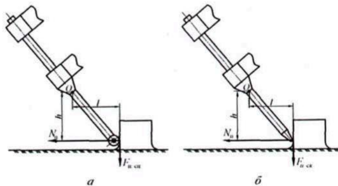
Рис. 3.68. Схемы для определения изгибающего момента, возникающего при взаимодействии зубьев с пнем: a — для зуба, оснащенного контактным роликом; b — для зуба без ролика
