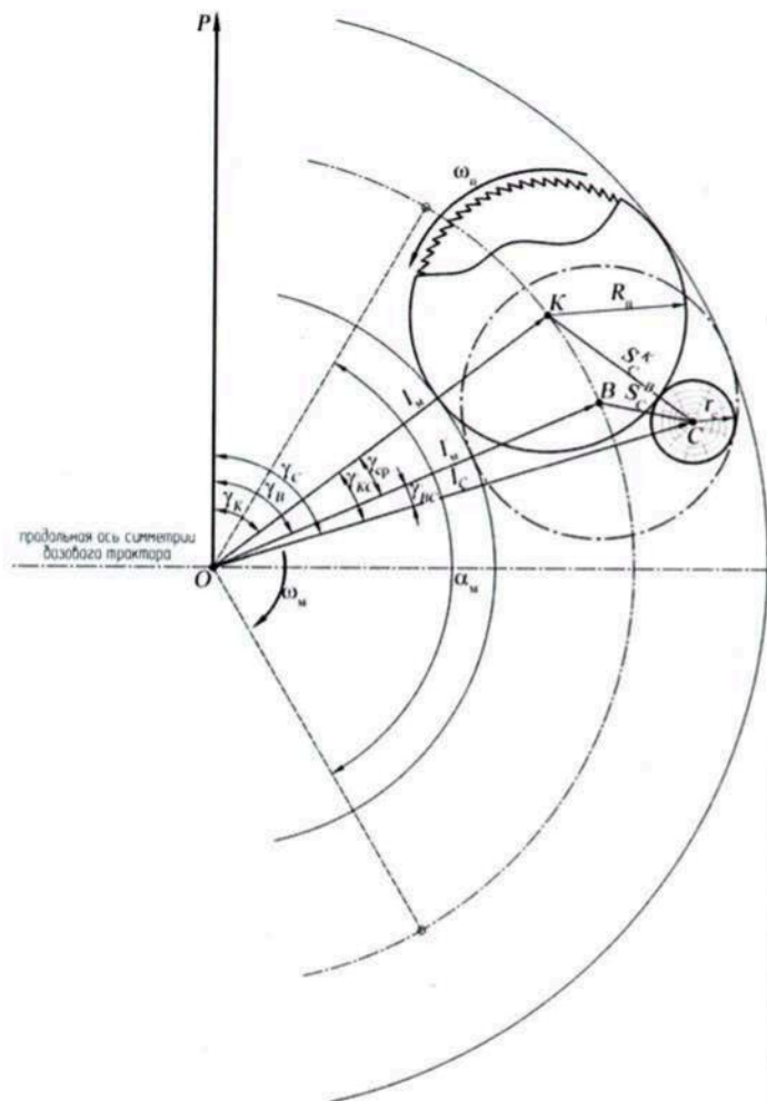
Рис. 3.44. Схема для определения необходимого угла поворота маятниковой стрелы при срезке единичного ствола
