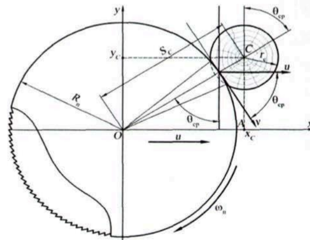
Рис. 3.38. Схема к определению среднего кинематического угла встречи
