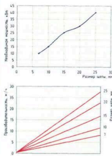
Рис. 1.61. Характеристики рубильной машины CH260 HF-2EL при частоте вращения рабочего органа 540 об./мин
