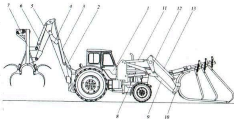
Рис. 3.53. Принципиальная схема подборщика – собирателя срезанной древесно-кустарниковой растительности: 1 – базовый трактор МТЗ-82; 2 – гидроцилиндр экскаваторной стрелы; 3 – гидроцилиндр управления рукоятью; 4 – стрела экскаватора; 5 – рукоять; 6 – напорный гидроцилиндр; 7 – грейфер; 8 – гидроцилиндр стрелы погрузчика; 9 – стрела погрузчика; 10 – подборщик срезанной древесно-кустарниковой растительности; 11 – гидроцилиндр; 12 – поворотный рычаг; 13 – тяга
