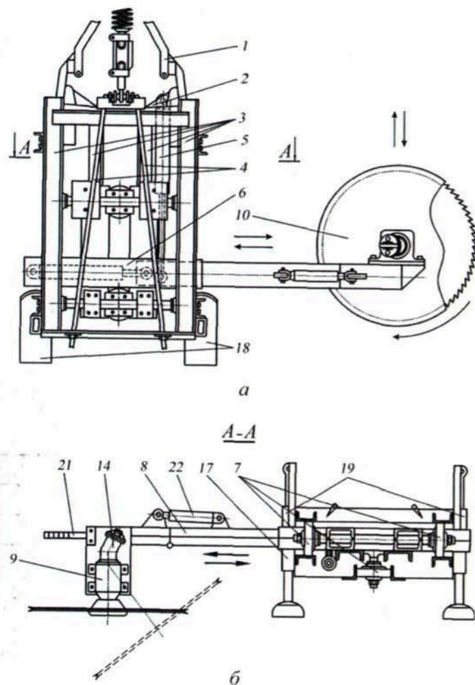
Рис. 3.11. Кусторез КН-1(СГАУ) с гидравлическим приводом: а – вид сверху; б – сечение А-А: 1 – система навески трактора; 2 – рама навески; 3 – направляющие бруссы; 4 – тяги; 5 – гидроцилиндр; 6 – тележка; 7 – катки; 8 – стрела; 9 – редуктор; 10 – дисковый пильный рабочий орган; 14 – гидромотор; 17 – направляющие втулки; 18 – опорные лыжи; 19, 22 – гидроцилиндры; 21 – пружинная лапка
