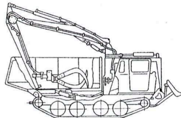
Рис. 1.51. Подборочно-транспортная машина ЛП-23
