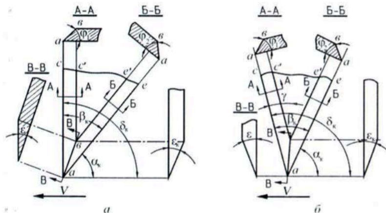
Рис. 1.34. Угловые характеристики зубьев пил для поперечной распиловки древесины: а – исполнение 1; б – исполнение 2; \alpha_k, \beta_k, \gamma_k, \delta_k – соответственно контурные углы: задний, заострения, передний и резания; \phi_1, \phi_2 – линейные углы боковой заточки по передней и задней граням зуба, град; \epsilon – угол наклона главной кромки от боковой стенки пропила
