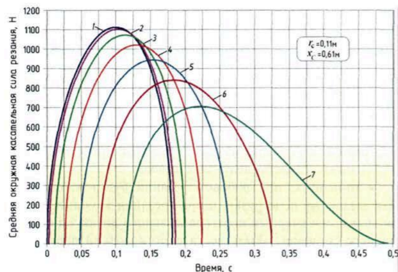
Рис. 3.40. Изменение средней окружной касательной силы резания во времени в зависимости от смещения центра ствола по оси y : 1 — при y_C = 0 ; 2 — при y_C = 0,065 м; 3 — при y_C = 0,13 м; 4 — при y_C = 0,195 м; 5 — при y_C = 0,26 м; 6 — при y_C = 0,325 м; 7 — при y_C = 0,39 м
