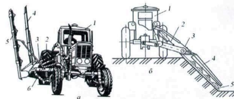
Рис. 1.21. Ротационная косилка PP-26: а и б – в транспортном и рабочем положении; 1 – трактор; 2 – гидроцилиндр; 3 – пружинный механизм подвески; 4 – защитный козырек; 5 – режущий аппарат; 6 – рама для навески режущего аппарата
