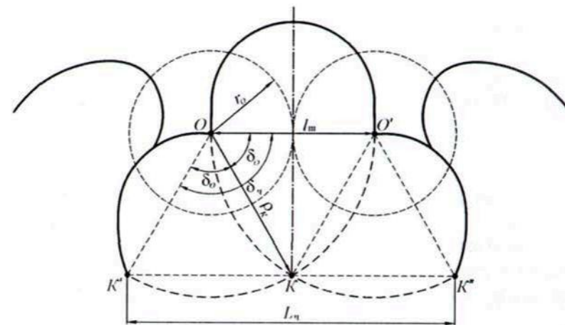
Рис. 3.81. Положение зубьев грейфера при полностью раскрытых челюстях
