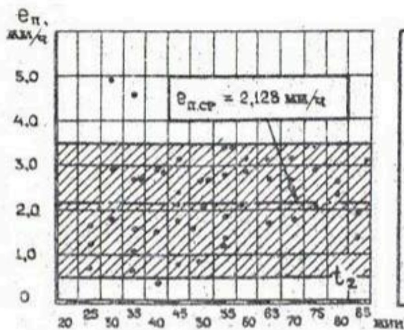
Рис. 3,4 Изменение скорости испарения во времени.
