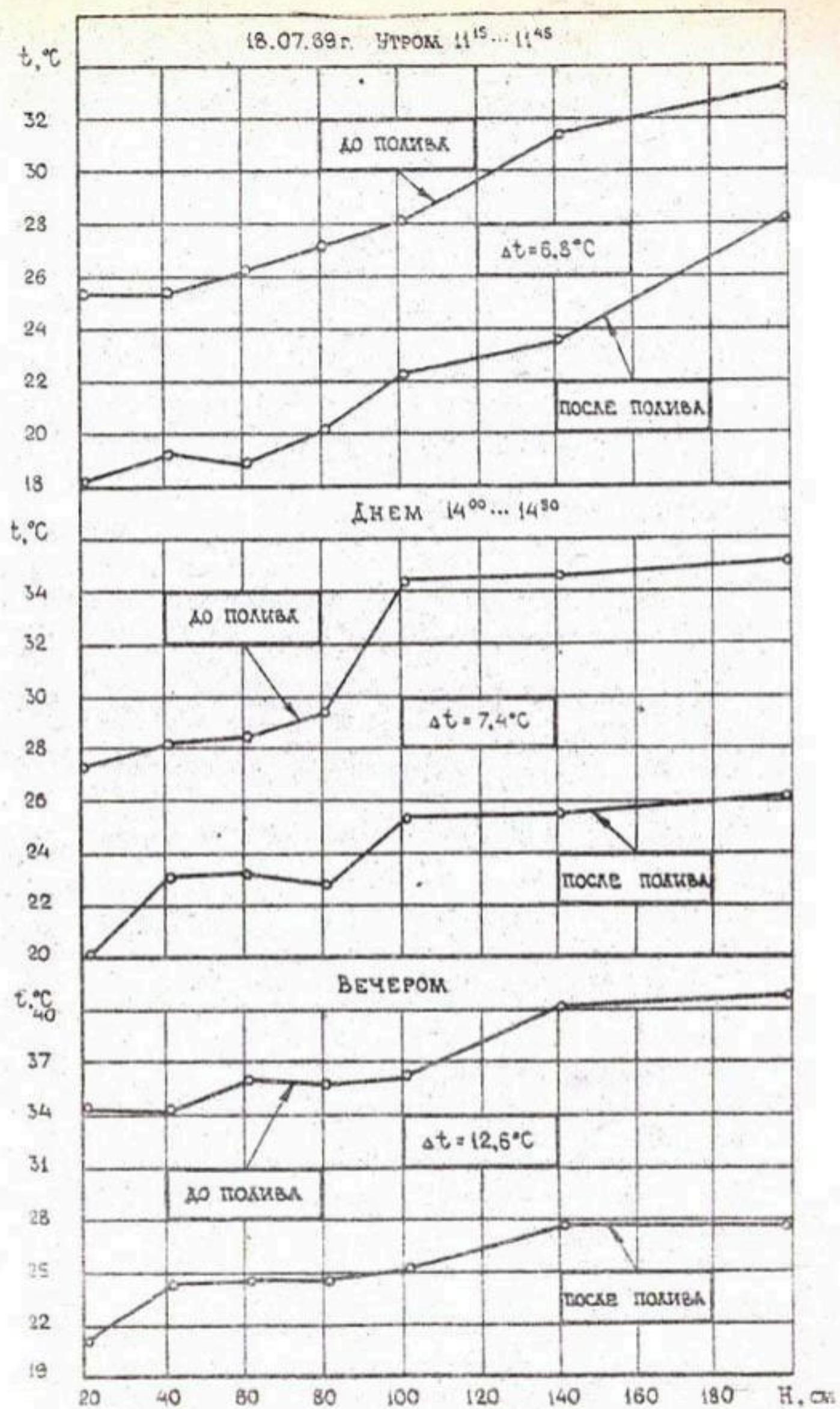
Рис. 416 Влияние полива на температуру воздуха
