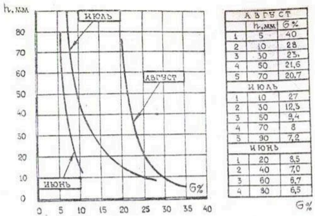
Рис. 3.10 Влияние поливной нормы и фазы развития хлопчатника на величины задержания воды листьями
