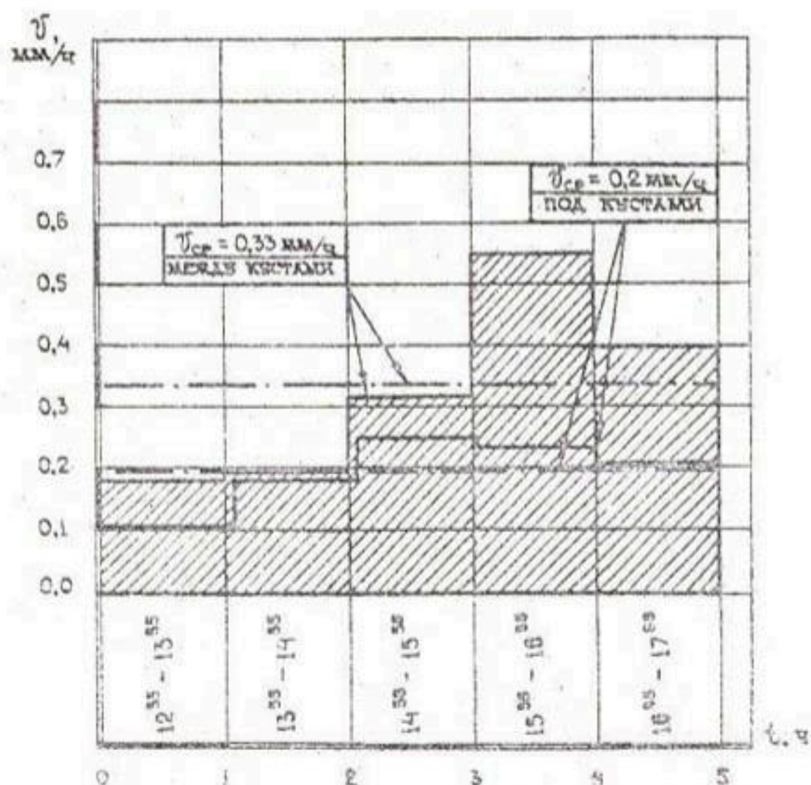
Рис. 3.11. Влияние моста установки дождемеров и времени суток на скорость испарения.
