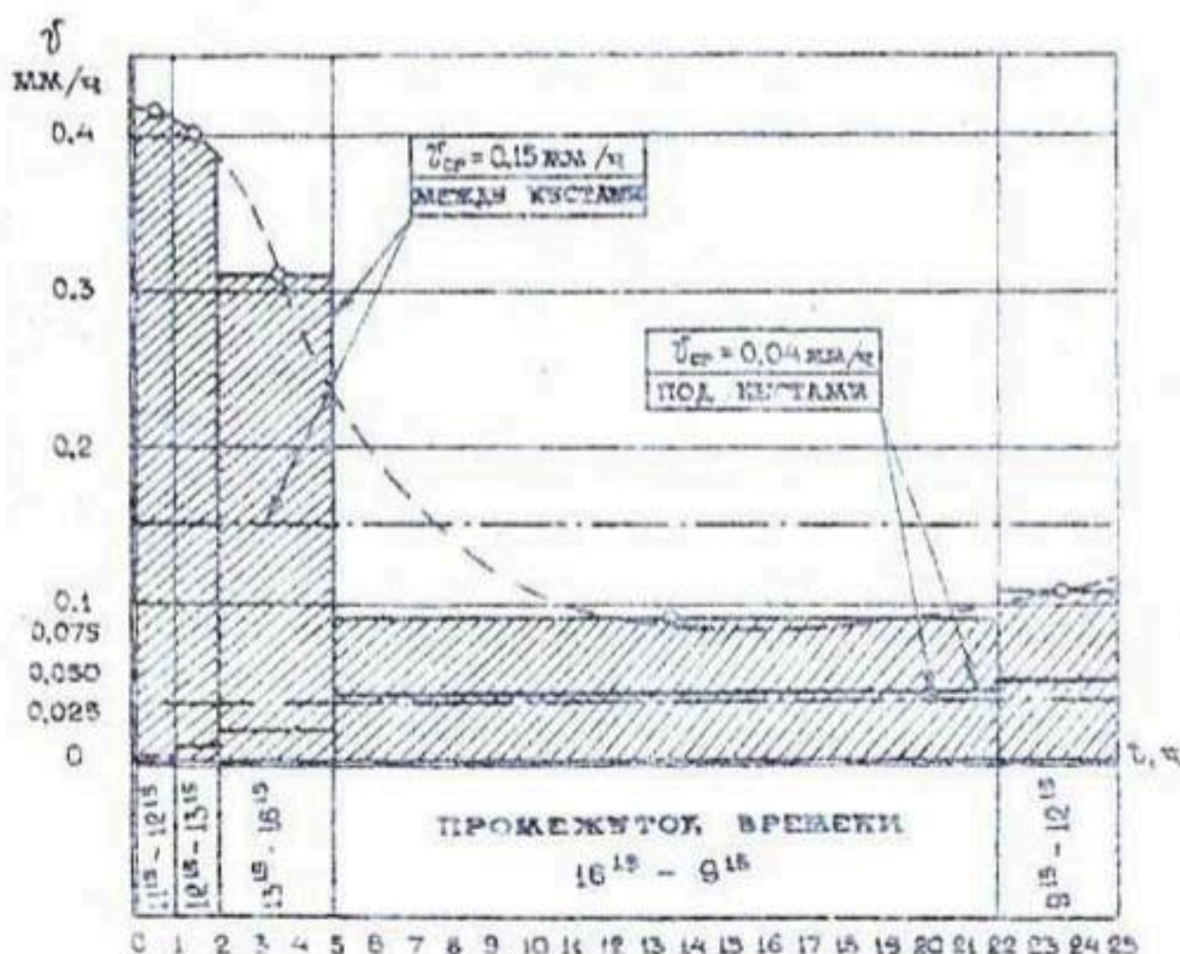
Рис. 5.10 Средние значения скорости испарения в дождемерах в интервалах времени.
