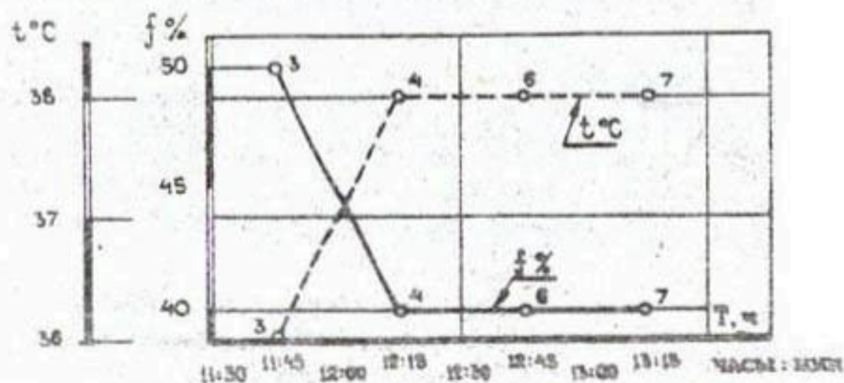
Рис. 4.8 ИЗМЕНЕНИЕ ПАРАМЕТРОВ МИКРОКЛИМАТА ПЕРЕД МАШИНОЙ "КУБАНЬ"
