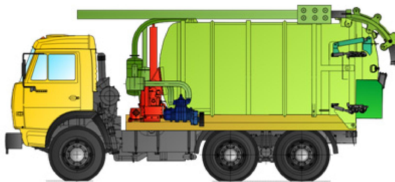
Рис. 1. Машина ДКТ-305 для эксплуатации до -10°C с самосвальным механизмом разгрузки и кассетой всасывающего рукава
