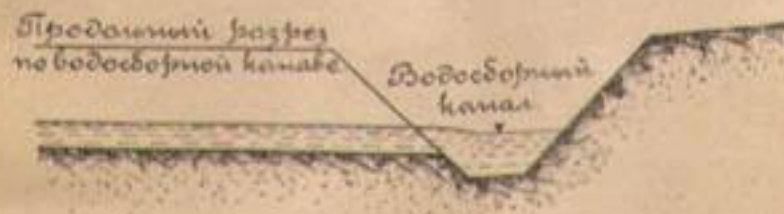
Черт. 40. Поперечное сечение по водосборному каналу и продольное по водосборной канаве.
