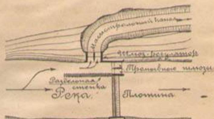
Черт. 24. Водоподъемная плотина со шлюзом-регулятором.
