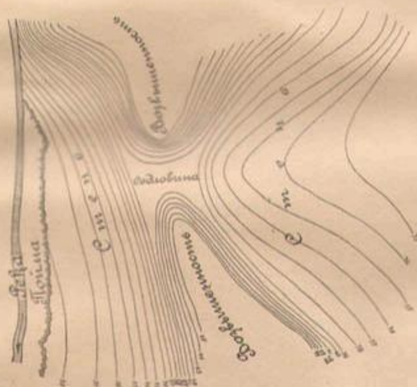
Черт. 68. „Долинный“ тип рельефа. Местность замкнута с верховой стороны и соединена через „седловину“ окаймляющей возвышенности с соседней степью, расположенной по другой стороне.
