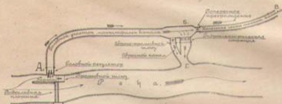
Черт. 138. Схема головных сооружений в случае устройства плотины и очень засоренного песчаными наносами потока.
