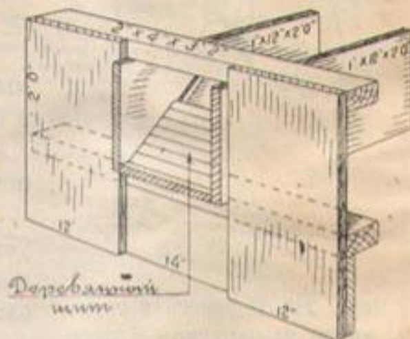
Черт. 224. Деревянный хозяйственный шлюзик со щитом.
