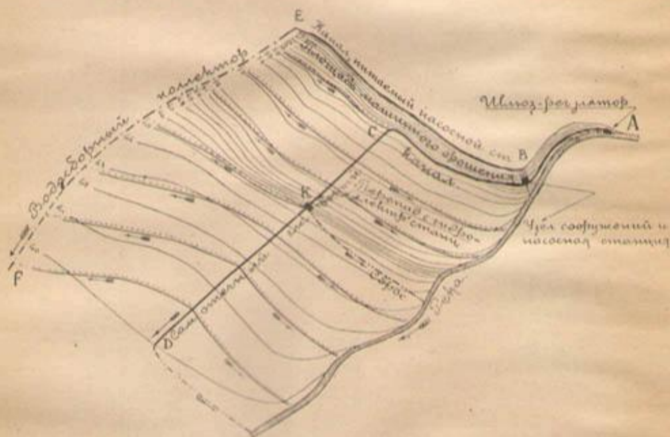
Черт. 48. Схема оросительной сети для предгорного района.
