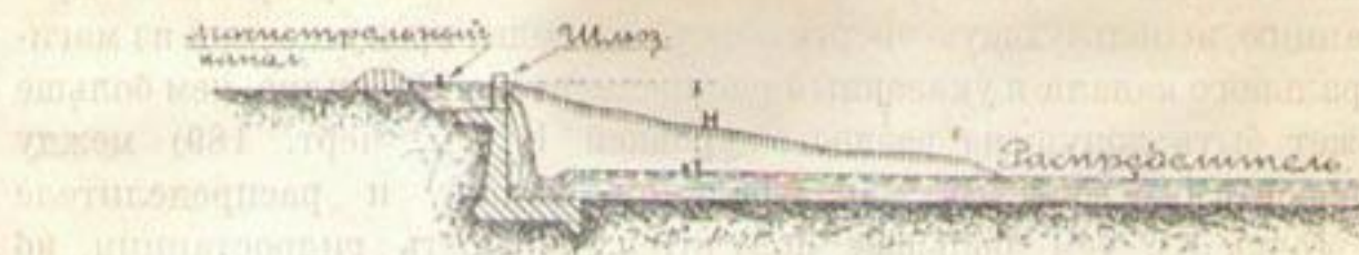
Черт. 189. Продольный разрез по оси распределителя на участке АБ (см. черт. 188).
