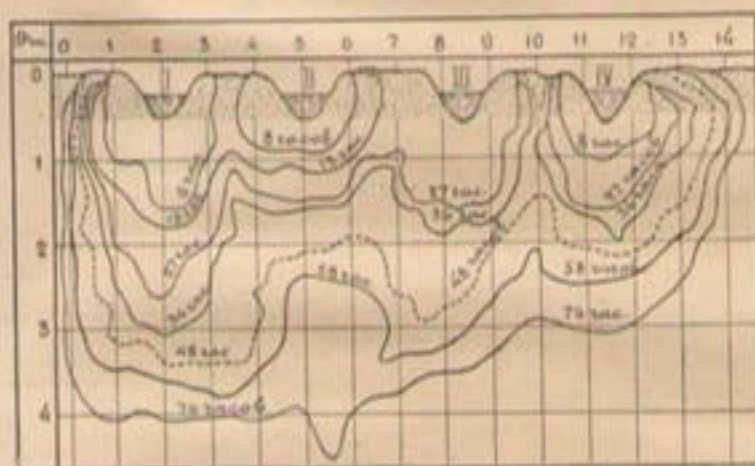
Черт. 16. Изолинии быстроты просачивания под глубокими поливными бороздами в тяжелом суглинке.
