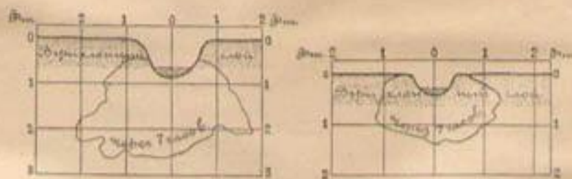
Черт. 14 и 15. Изолинии быстроты просачивания воды из борозд, глубиною в 10" и 5" за период времени в 7 часов.
