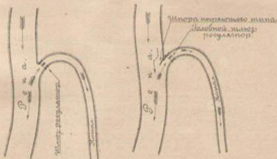
Черт. 134 и 135. Схемы устройства головной части канала петель (без шпору и со шпору ныряющего типа).
