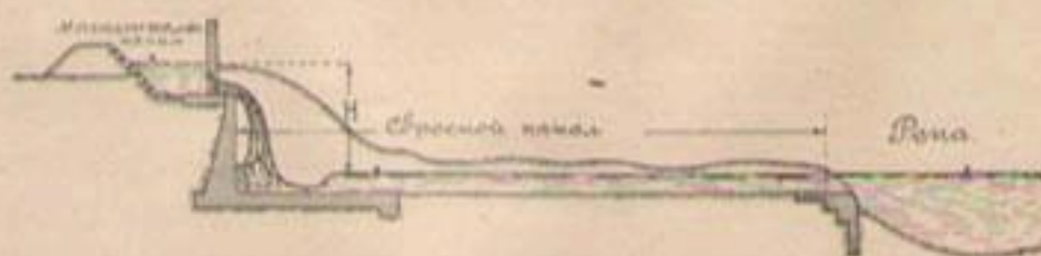
Черт. 156. Разрез по оси сбросного канала.
