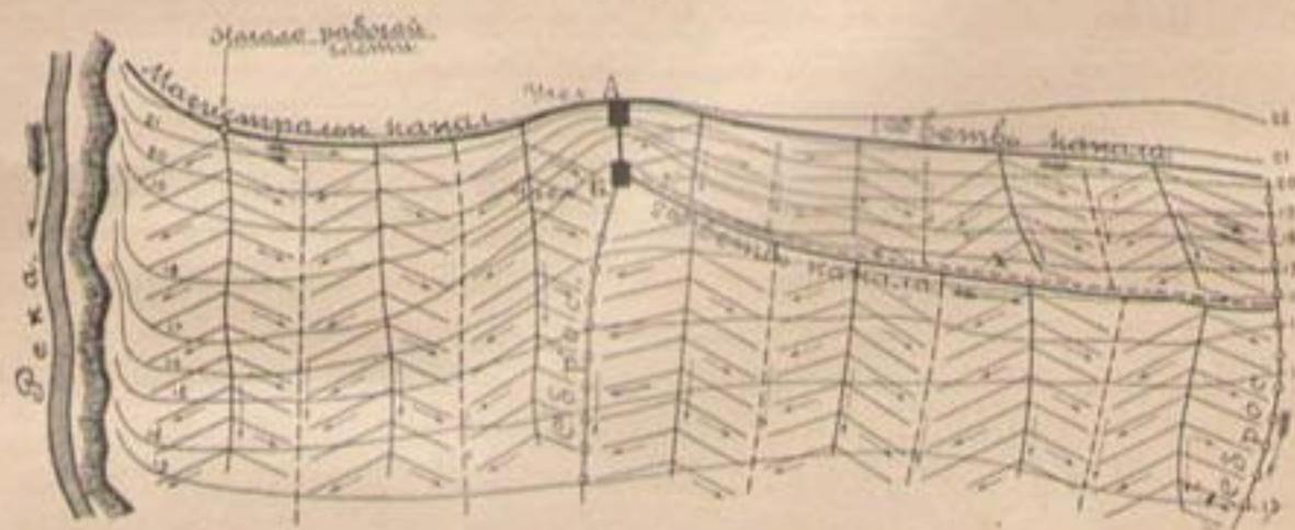
Черт. 163. Третий тип трассы магистрального канала.
