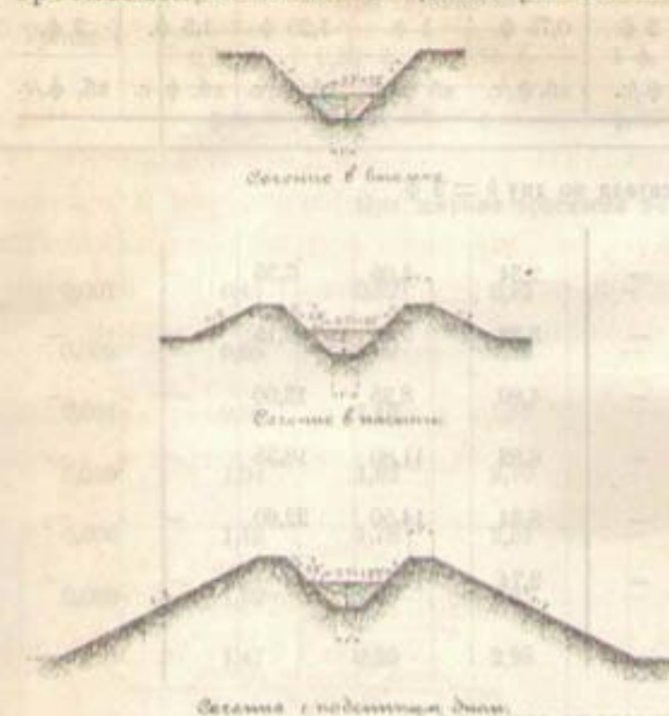
Черт. 200. Типы сечения оросителей (размеры в футах).
