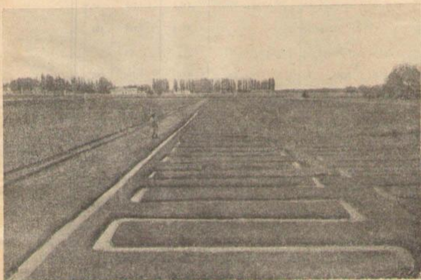
Фот. XVII. Зигзагообразные джояки. А. И. Шах-Назирев.
