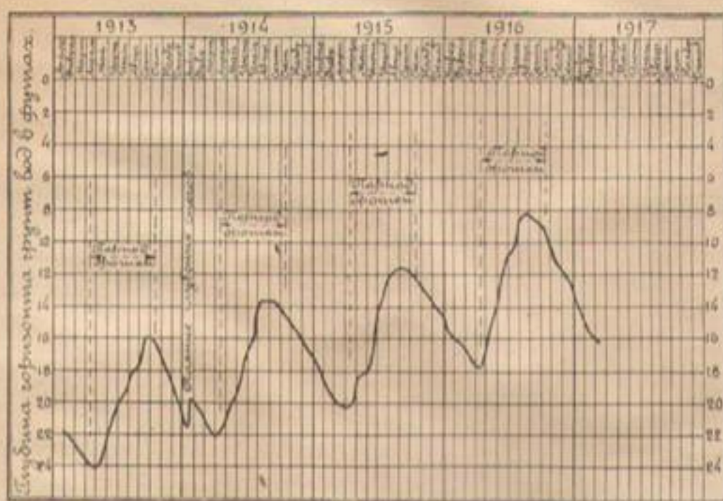
Черт. 74.—Кривая периодического колебания и поднятия грунтовых вод в Boise Valley, по Бёркхолдеру (Barkholder, J. L.—Reclamation Record, Dec. 1917 г.).
