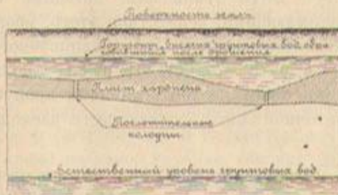
Черт. 289. Горизонт „висячих“ грунтовых вод, образовавшийся после орошения вследствие наличия слоя хардпена.
