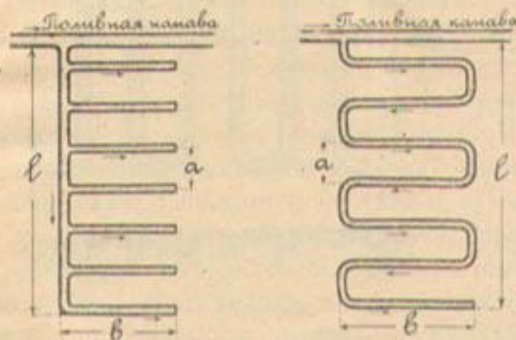
Черт. 271. Гребенчатое и зигзагообразное расположение джояков.
