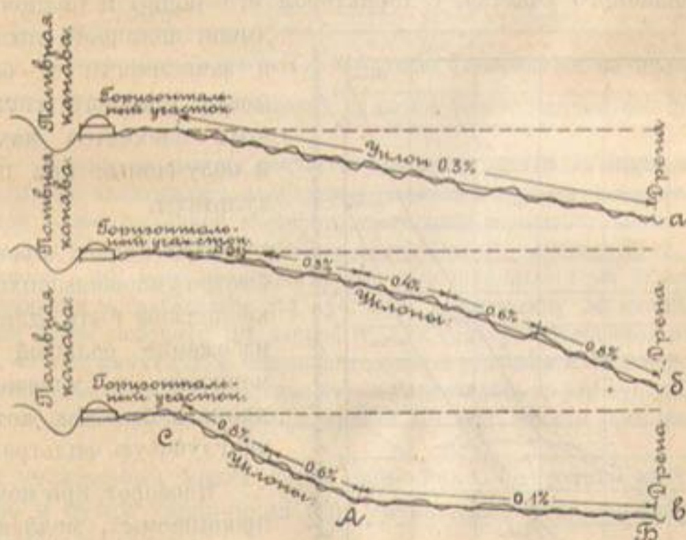
Черт. 240. Продольные профили типовых полос с показанием поверхности земли до и после планировки.
