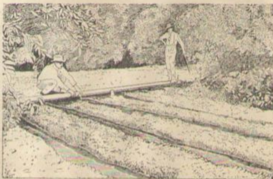
Фот. XVI. Орошение трубами. Питание борозд производится из трубопровода, расположенного между гидрантами.
