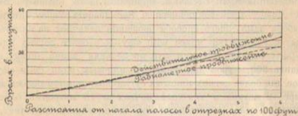
Черт. 242. Скорость продвижения воды на полосе длиной 600 футов.
