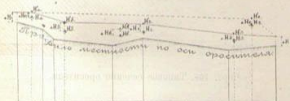
Черт. 197. К построению продольного профиля оросителя.
