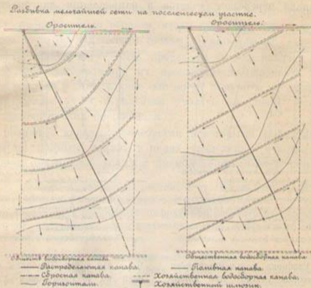
Черт. 220 а и б. Разбивка мельчайшей сети на поселепческом участке при наличии водораздела.
