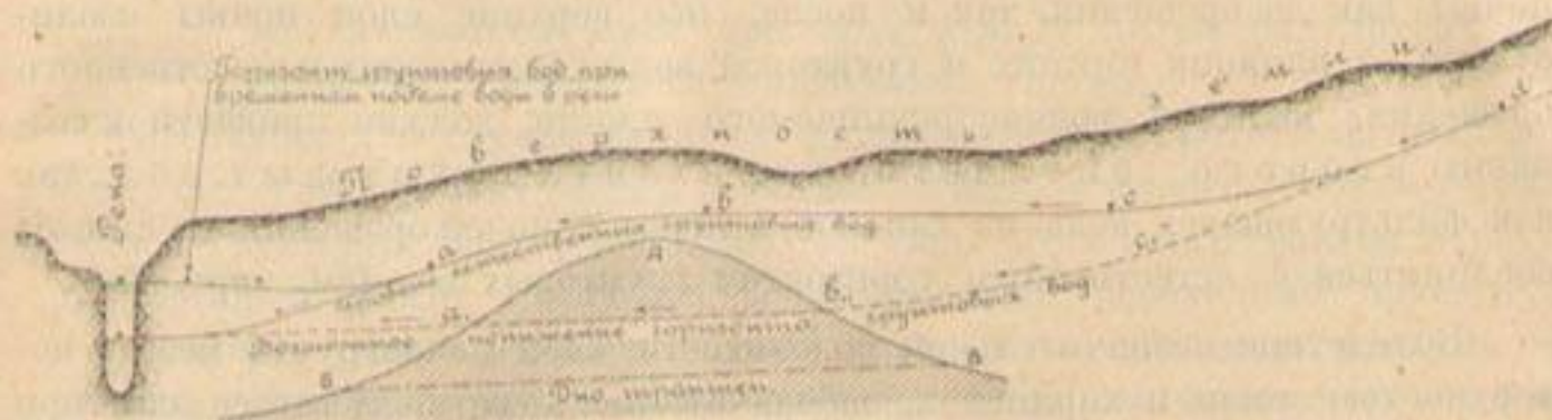
Черт. 290. Подземный водонепроницаемый холм, подпирющий уровень грунтовых вод.
