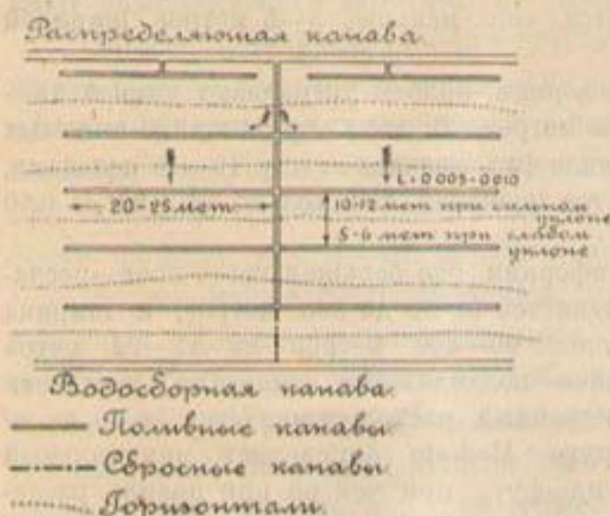
Черт. 244. Односкатная естественная система в ровной местности без водосборных канав на каждой делянке.
