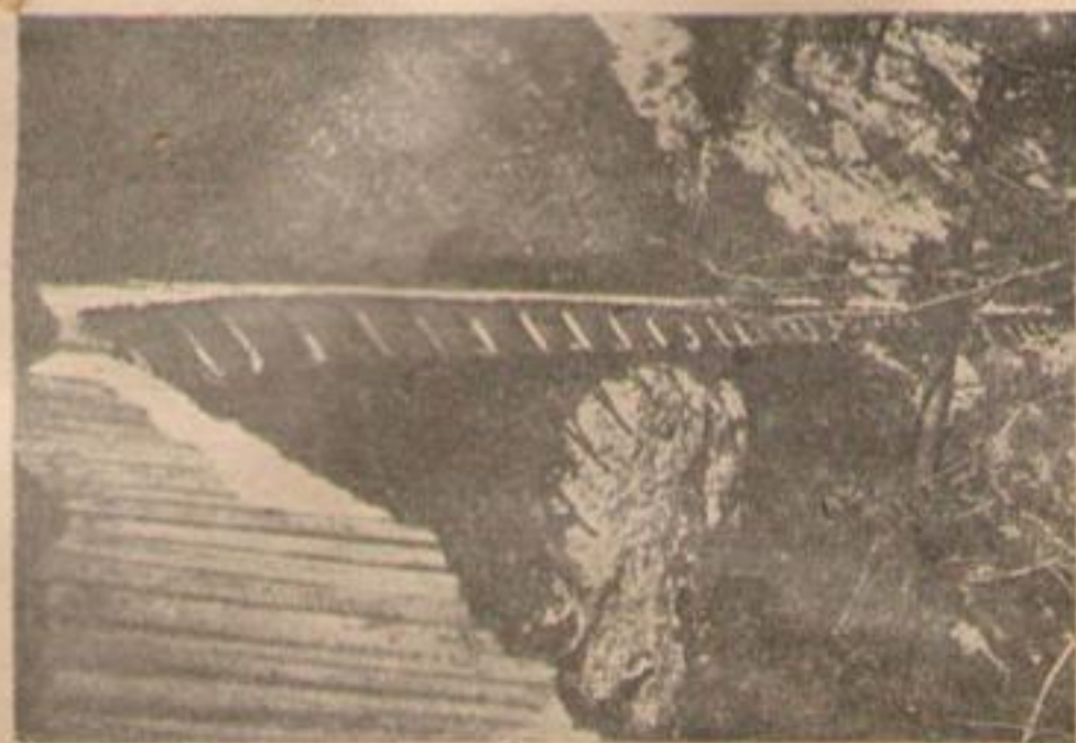
Фотогр. III. Маленький деревянный лоток на консолях. (С. III. С. Америки. Система Пенниктон).
