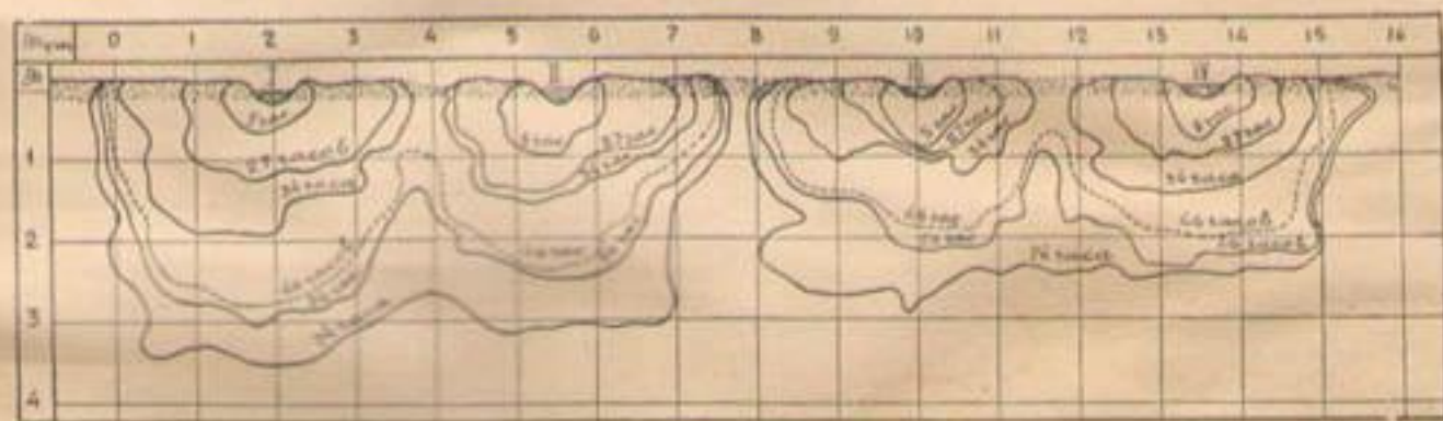
Черт. 17. Изолинии быстроты просачивания под мелкими поливными бороздами в тяжелом суглинке.
