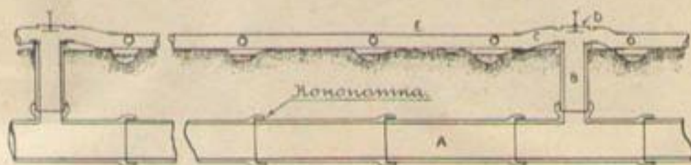
Черт. 270. Орошение трубами. Питание борозд производится из трубопровода, расположенного между гидрантами.
