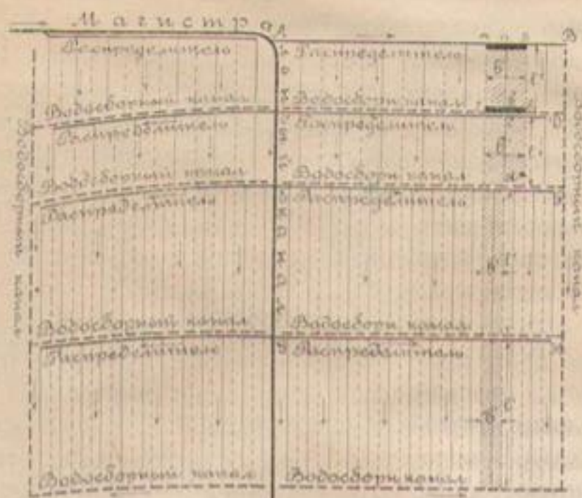
Черт. 185. Схема разбивки сети по второму типу.
