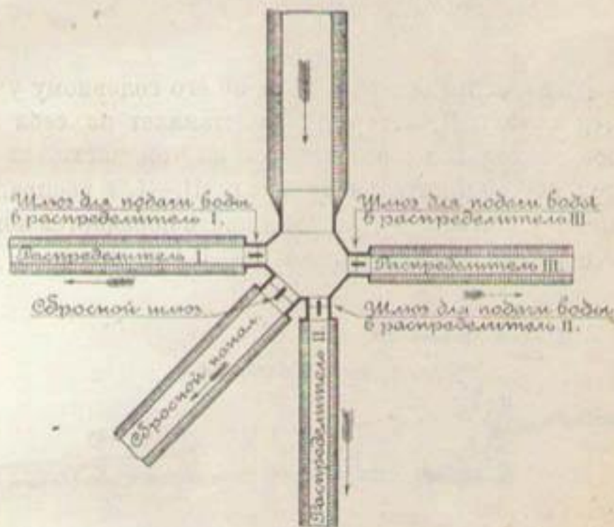
Черт. 195. Схема узла Д (см. черт. 192 и 193).
