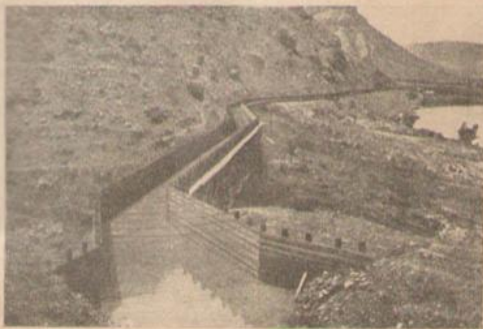
Фотогр. VIII. Переход канала в лоток (деревянный) С. И. С. Америки, шт. Колорадо, канал Меса).
