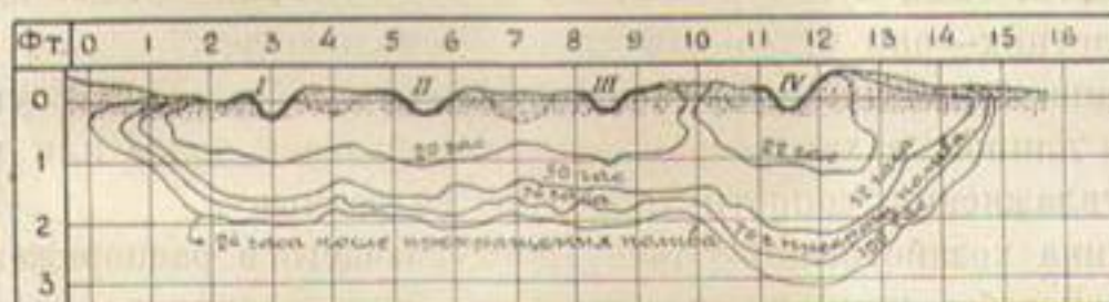
Черт. 268. Изолинии просачивания под мелкими поливными бороздами в тяжелом глинистом грунте.
