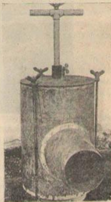
Фот. X. Переносный распределительный гидрант.
