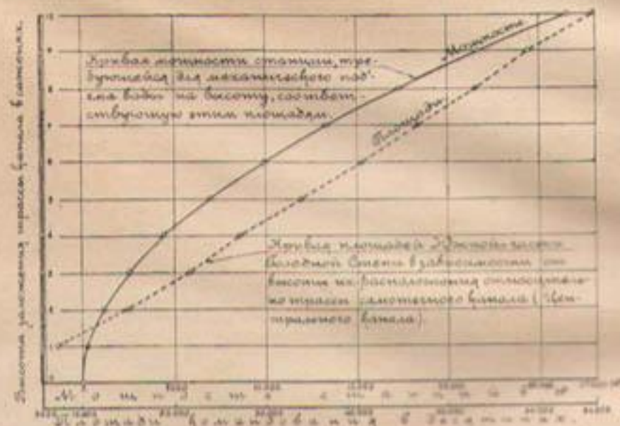
Черт. 109. Сопоставление кривой характеристики рельефа с кривой зависимости мощности станций от площади орошения.
