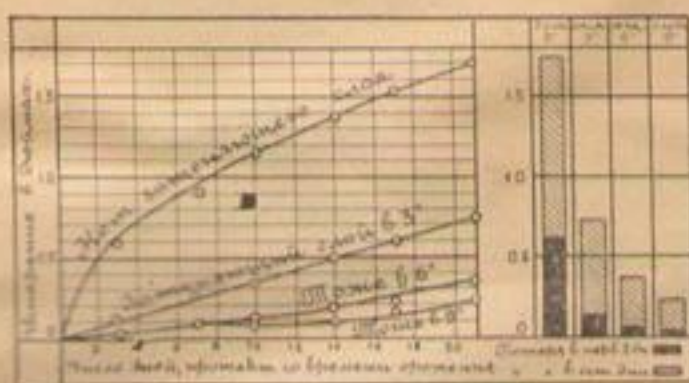
Черт. 10. Потери через испарение с поверхности почвы, защищенной затеяющим слоем 1) .
