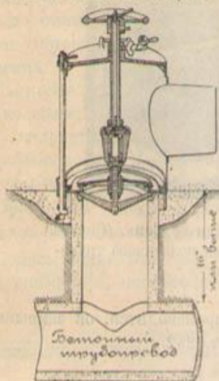
Переносный гидрант
