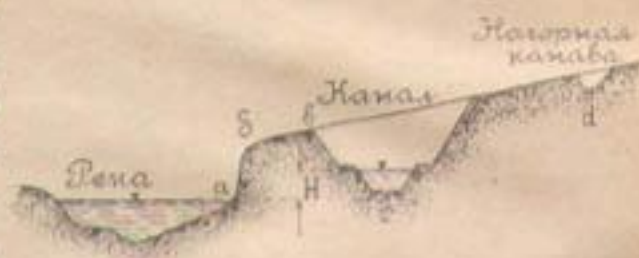
Черт. 146. Проложение холостой части канала в высоком берегу.
