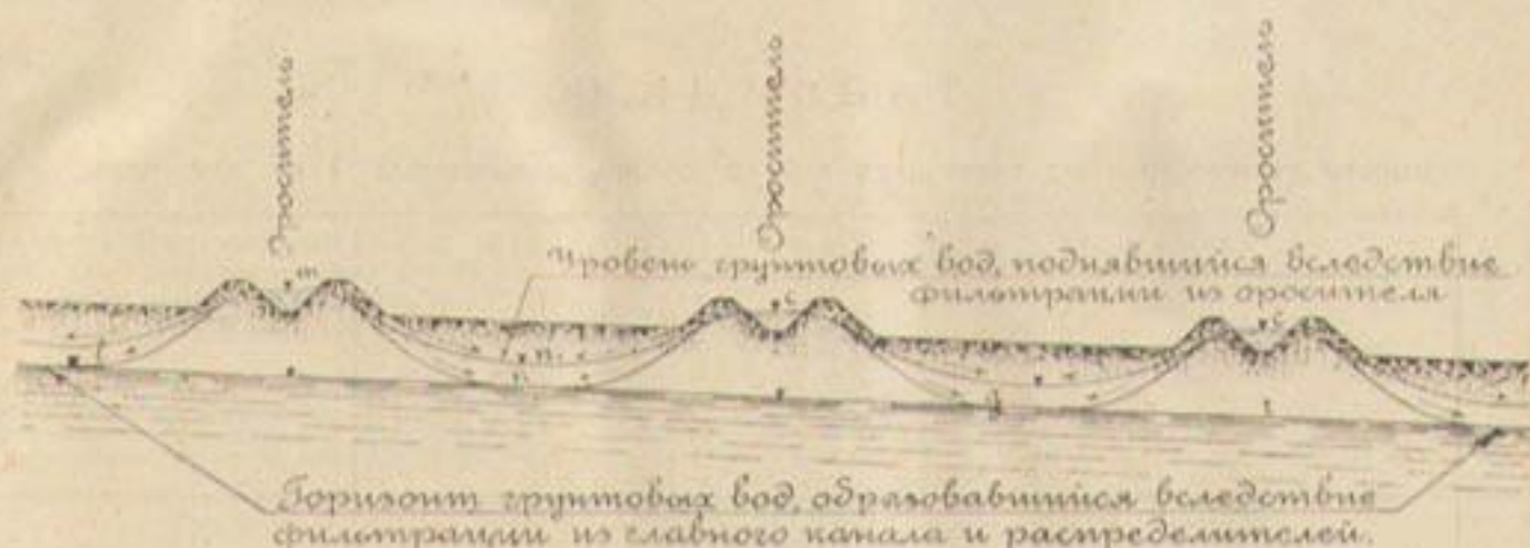
Черт. 281. Разрез по ab (см. черт. 279).
