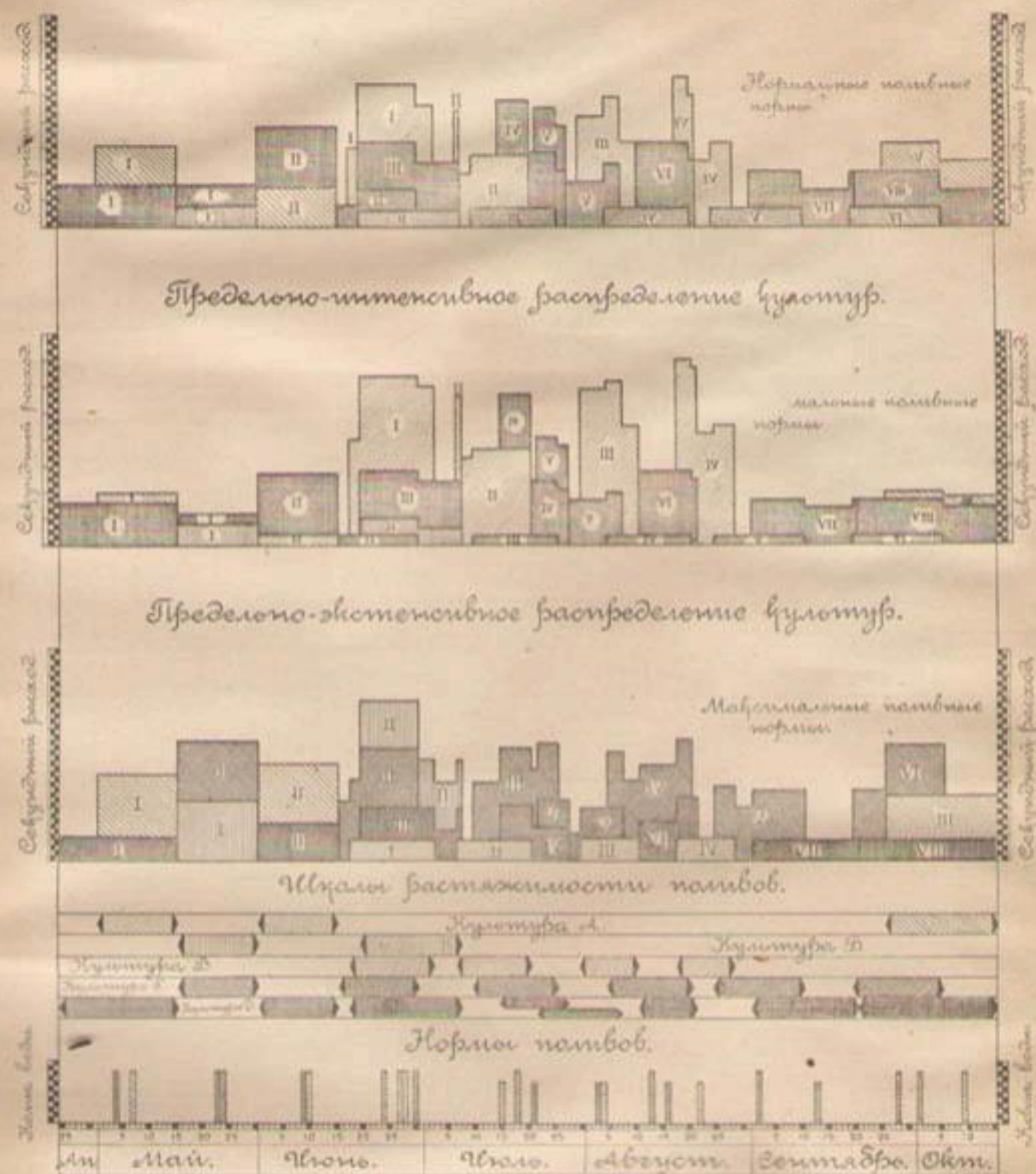
Черт. 78. Графики отдачи воды на поля орошения при нормальном, предельно-интенсивном и предельно-экстенсивном распределении культур.
