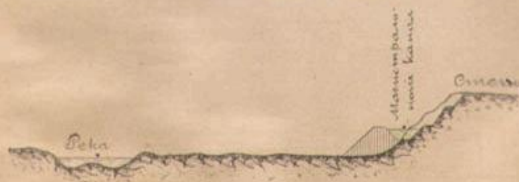
Черт. 34. Типовое поперечное сечение магистрального канала при прохождении им косогора.
