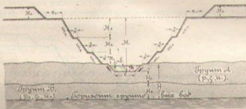
Черт. 169. Сечение канала в глубокой выемке.
