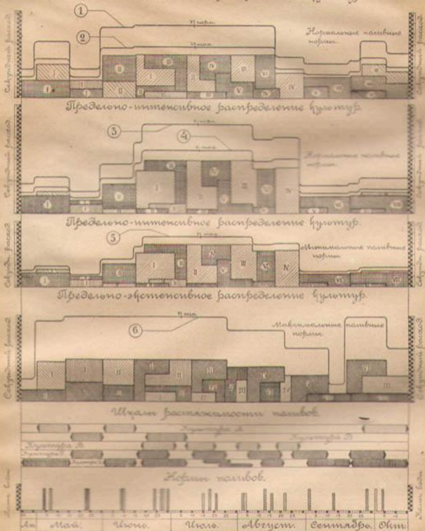
Черт. 81. Графики отдачи воды на поля и графики потребления воды из источника орошения при различном распределении культур и разных коэффициентах полезного действия.
