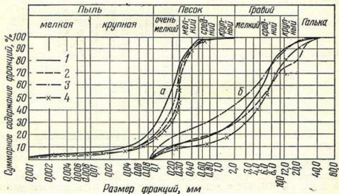
Рис. 48. Гранулометрический состав водовмещающих пород (а) и гравийной обсыпки (б) (Волгоградское Заволжье, Кисловская сросительная система), 1977 г.:
