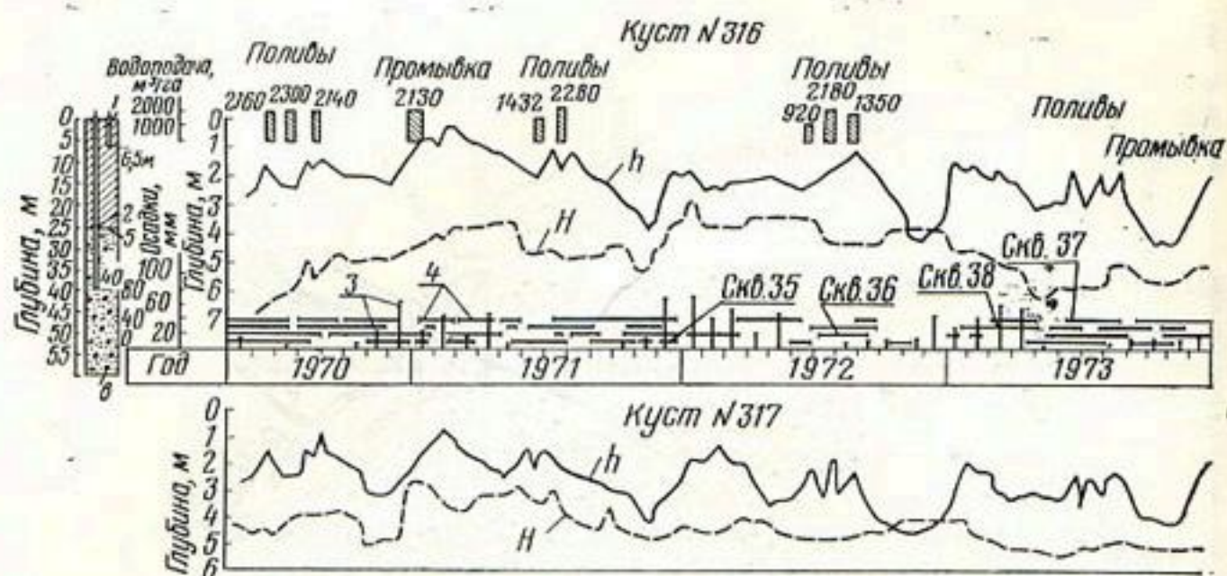
Рис. 26. Режим грунтовых и напорных вод орошаемого поля на фоне вертикального дренажа (Шурузьякский массив):
