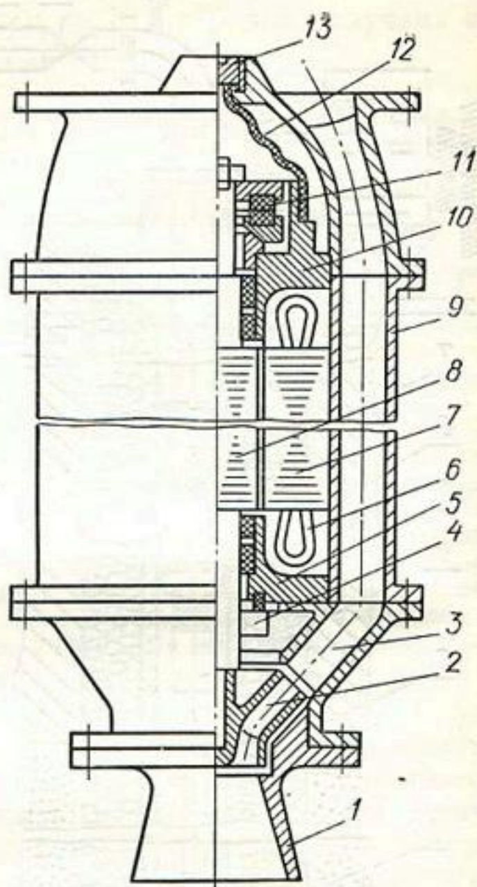
Рис. 56. Схема скважинного капсульного электронасоса СКЭН16-315-30:
