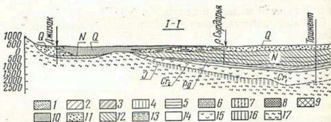
Рис. 16. Схема Голодностепеского гидрогеологического бассейна:
