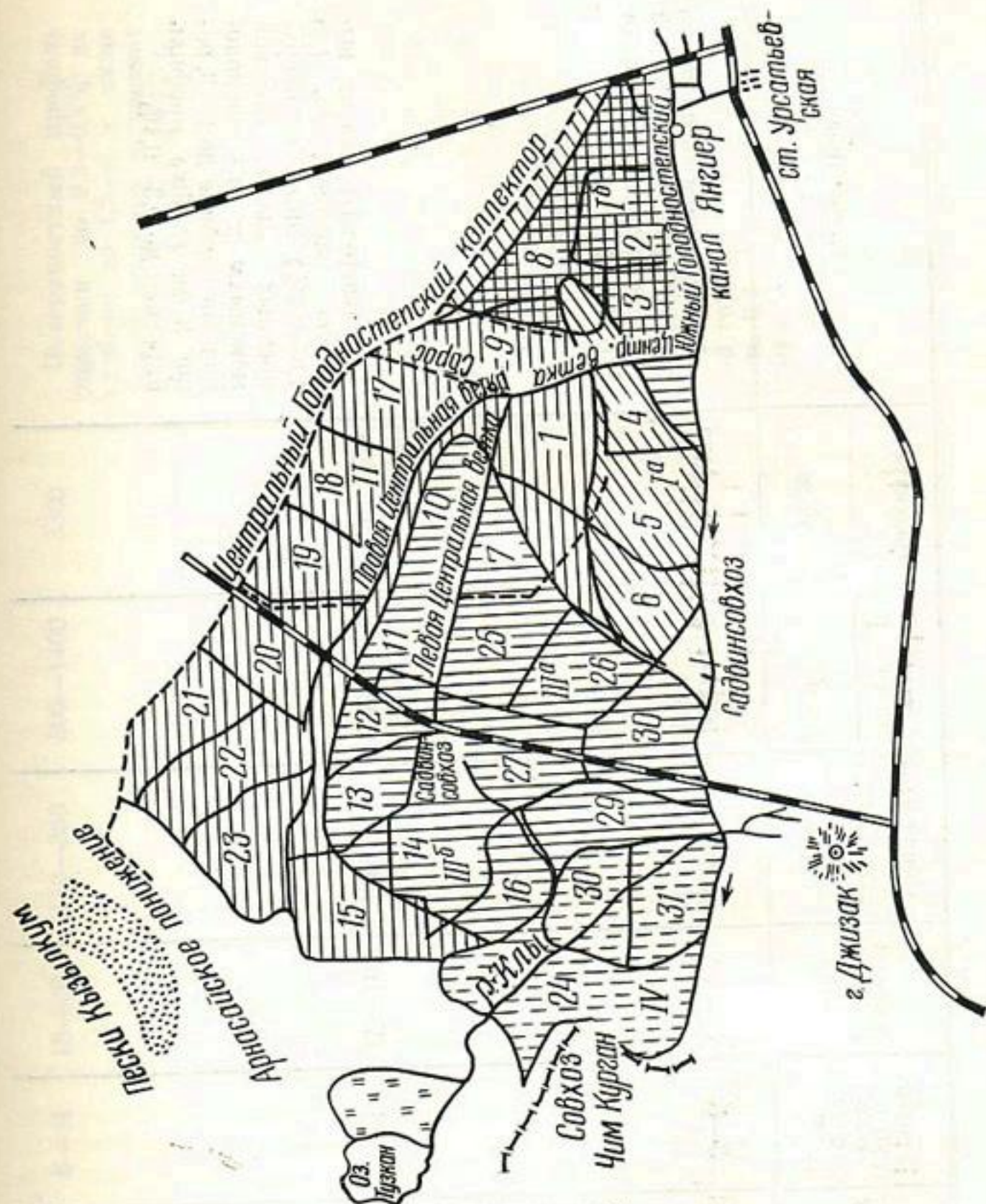
Рис. 19. Схема распределения первичных засоленных легкорастворимых солей в 20-метровой толще почвогрунтов. Зона нового орошения Голодной степи (по данным З. П. Пушкаревой и Н. М. Решеткиной); 1, 2, 3, ..., 31 — номера хлопководческих совхозов (см. на обороте).
