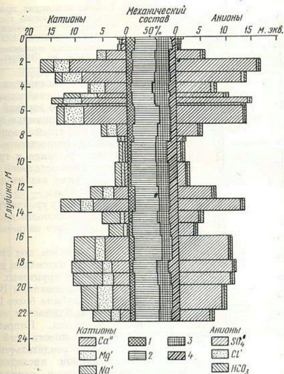
Рис. 8. Солевой профиль типичного серозема на лессе Ташкентского цикла:
