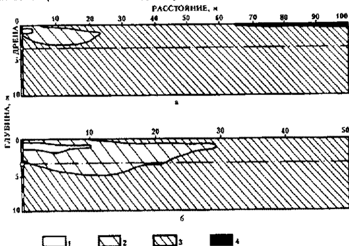
Рис. 7.7. Расслоение почвогрунта (конец вегетации — 10-й год), %: а — на фоне разрезженного дренажа; б — на фоне расчетного дренажа; 1 — 0,5; 2 — 0,5...1,0; 3 — 1,0...8,0; 4 — 8,0
