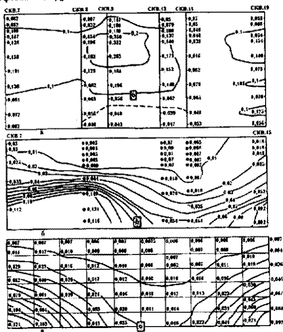
Рис. 7.6. Засоление почвогрунтов на междренье (по иону хлора, %). Совхоз Узакова, 1973 (по В.С.Борисову, Л.М.Рексу, Л.В.Киричевой): а — исходное; б — конечное; в — теоретическое распределение солей по профилю междренья и окончании промывки; 0,1; 0,2 — изолинии концентрации иона Cl, % в водной вытяжке; дрена: 0,180 — содержание иона Cl в водной вытяжке, %.
