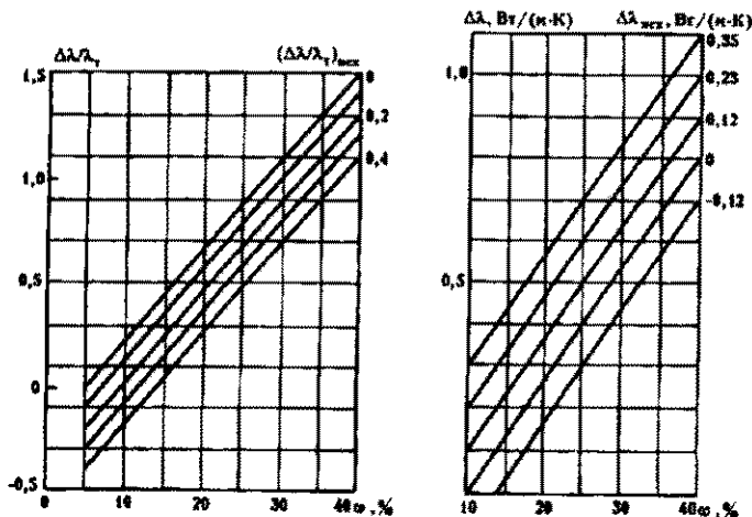
Рис. 7.2. Зависимость критерия \Delta\lambda/\lambda_T для промерзших песчаных горных пород от влажности при различных значениях (\Delta\lambda/\lambda_T)_{исх} . Зависимость \Delta\lambda для промерзших глинистых горных пород от влажности при различных значениях \Delta\lambda_{исх} .
