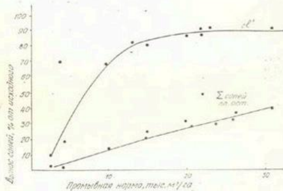
Рис. 10. Вынос водорастворимых солей в зависимости от нормы промывки.
