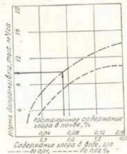
Рис. 18 Номограмма для расчета норм доpromывки суглинистых и супесчаных почв по хлор-иону.
