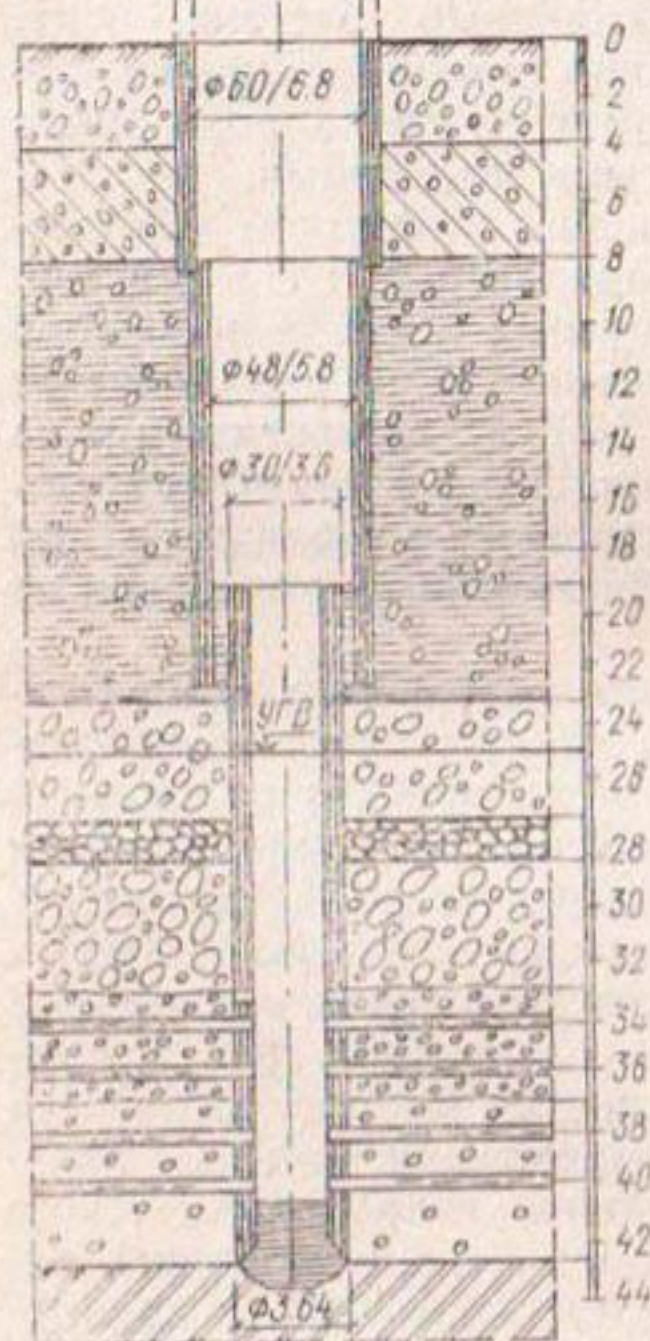
Рис. 1.18. Четырехъярусный лучевой водозабор с телескопической водосборной камерой в г. Турине (Италия)
