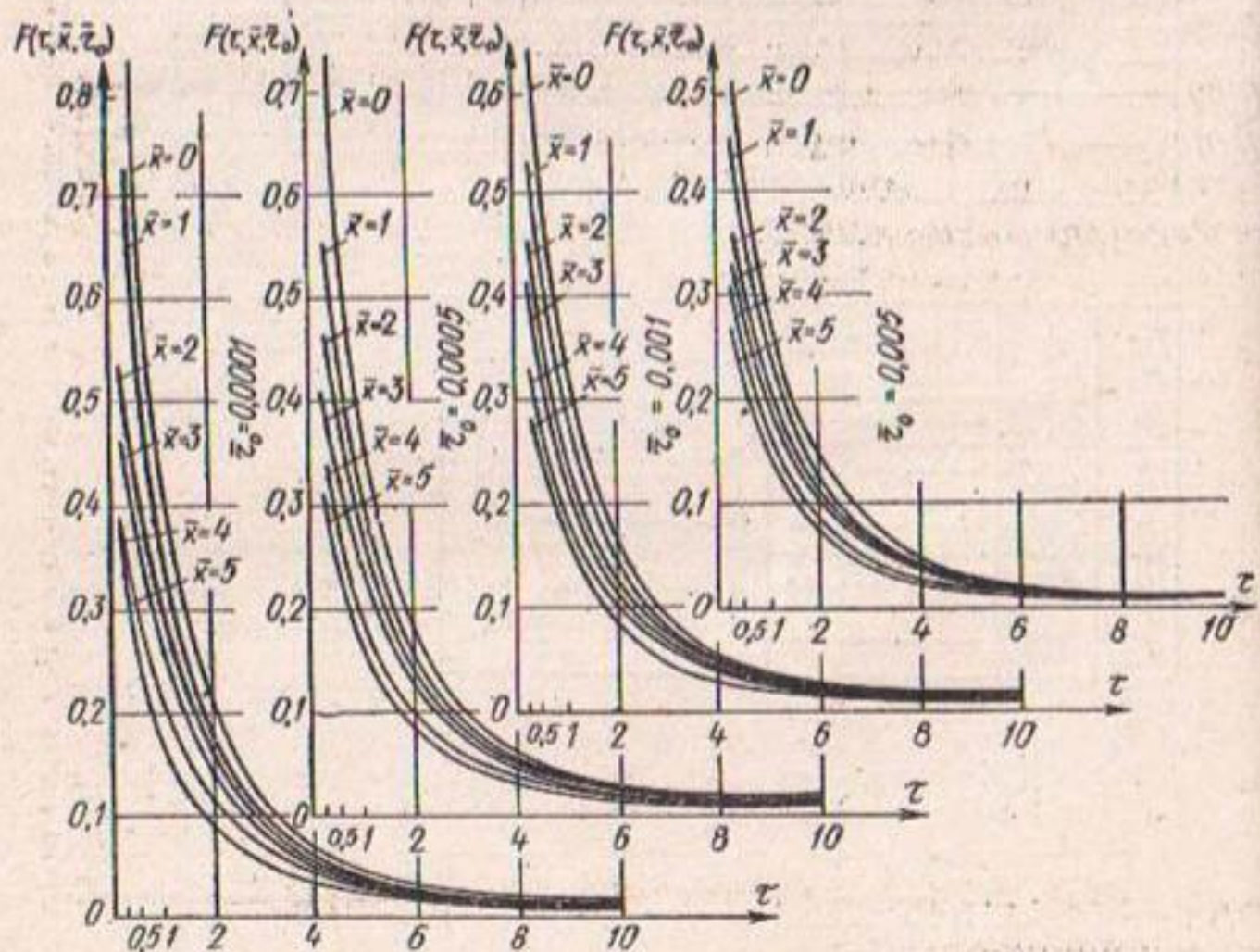
Рис. 2.5. Кривые F(\tau, \bar{x}, \bar{r}_0) для расчета комбинированного дренажа
