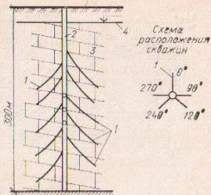
Рис. 1.13. Многозабойные пуче- вые криволинейные буровые скважины (Урал)
