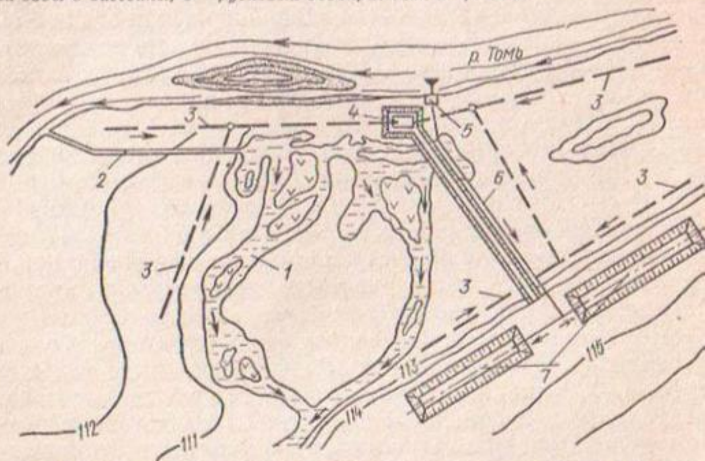
Рис. 1.3. Горизонтальный водозабор на р. Томь с подпиткой из затопляемых в межень естественных речных проток и стариц [Новокузнецк]
