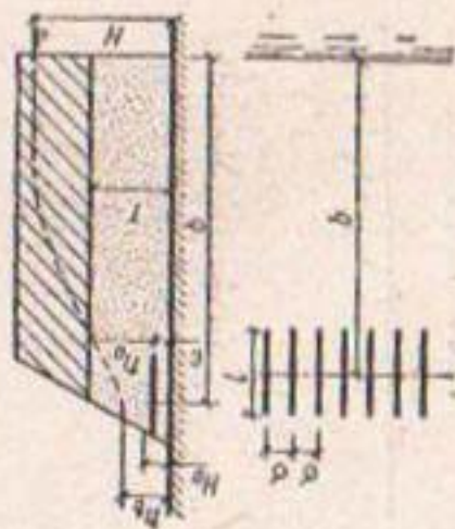
12. Ряд параллельных скважин в пологоранченном пласте с боковым прямолинейным контуром питания
