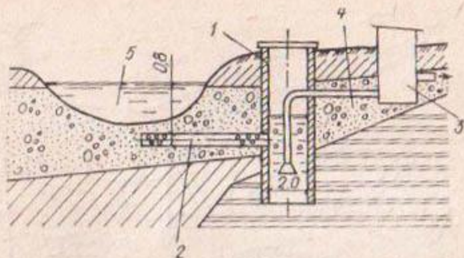
Рис. 4.5. Двухлучевой трубчатый водозабор Абанского зерносовхоза
