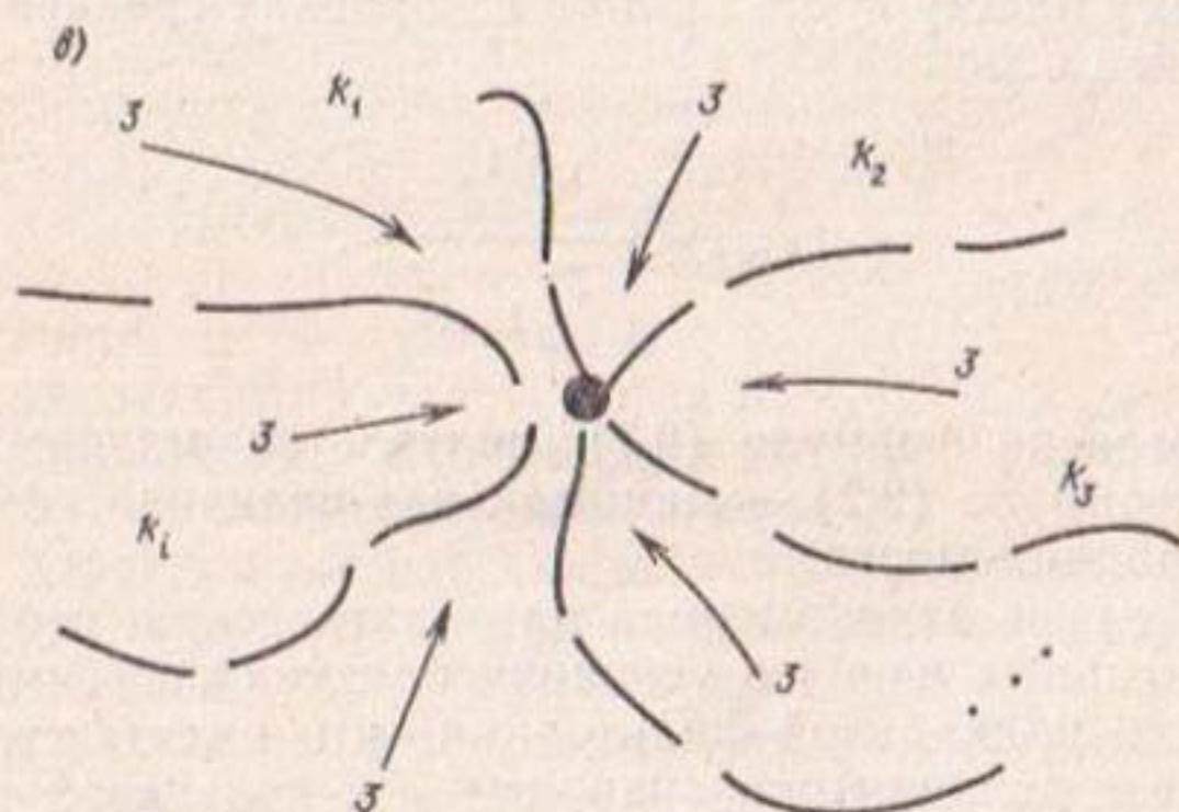
Рис. 2.1. Виды [а, б, в] плановой фильтрационной неоднородности 1 — граница питания пласта; 2 — непроницаемая граница пласта; 3 — линия тока
