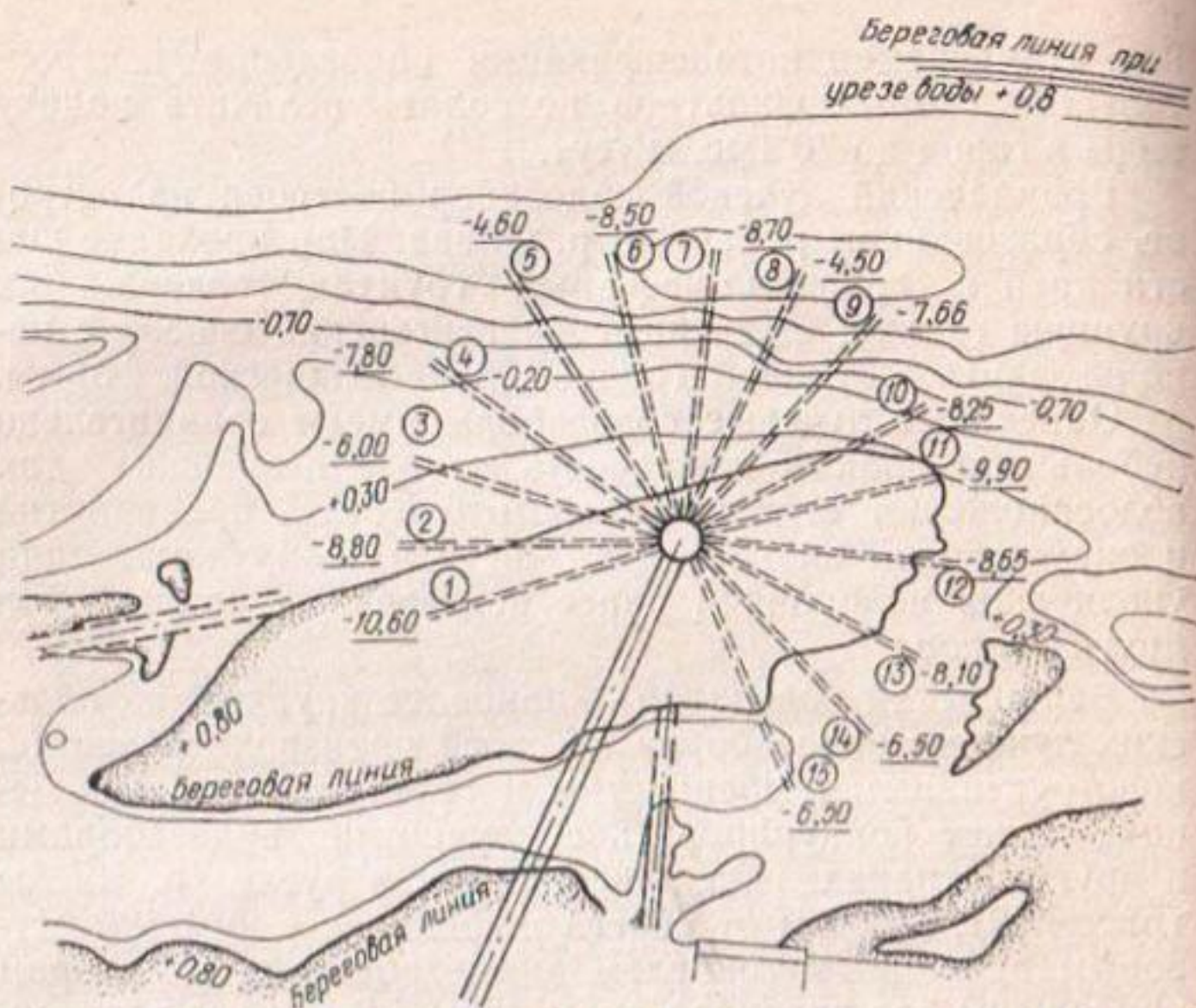
Рис. 4.13. Схема подруслового лучевого водозабора варшавского городского водопровода
