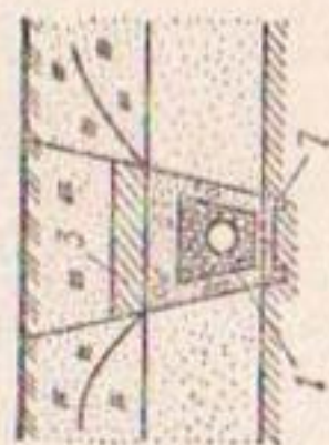
3. Трубчатый водозабор
