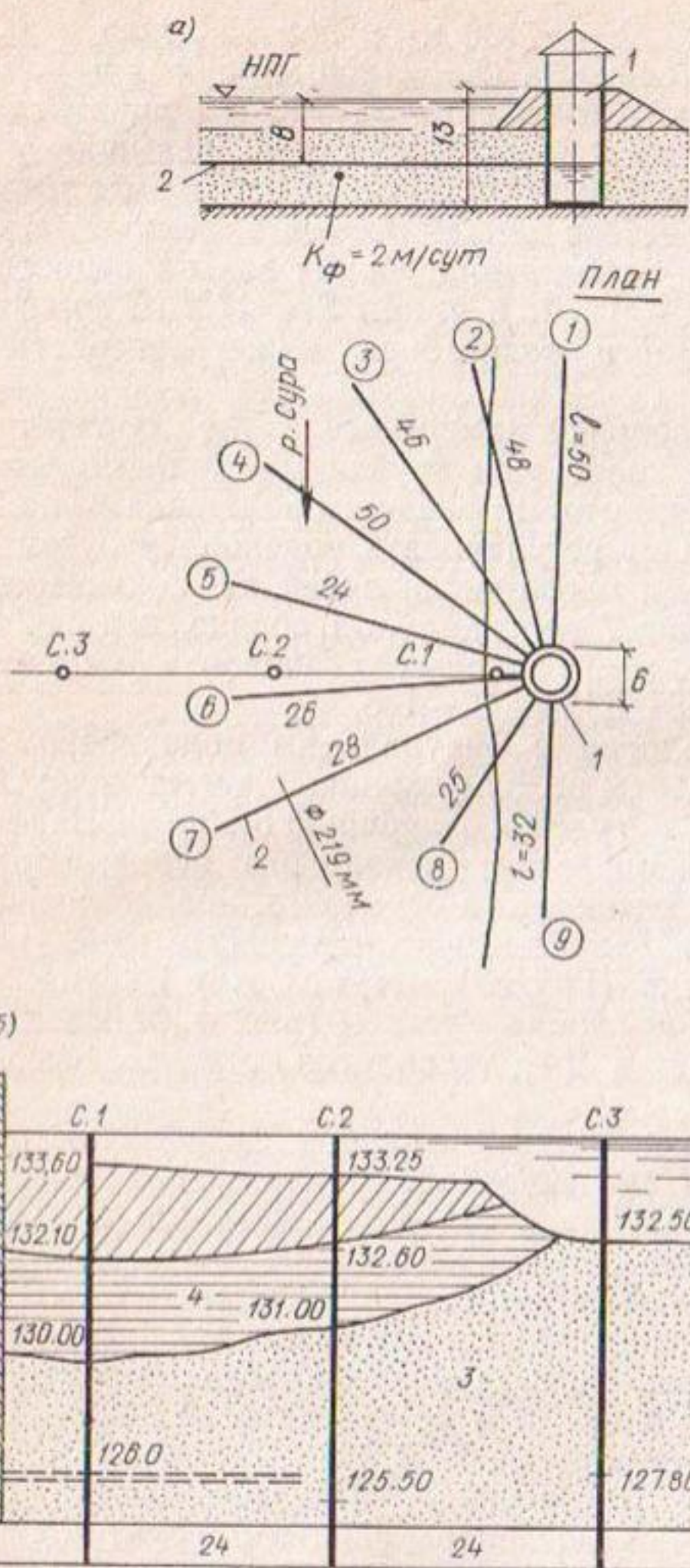
Рис. 4.3. Лучевой водозабор на р. Сура в Пензе
