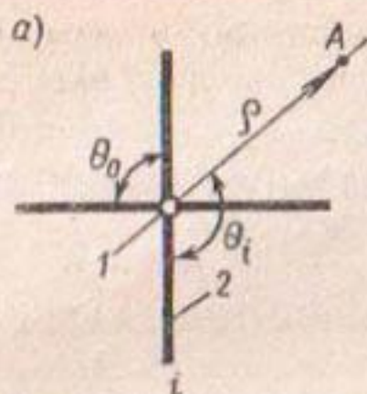
Рис. 2.7. Одиночный лучевой дренаж с равномерно расположенными по кругу лучами
