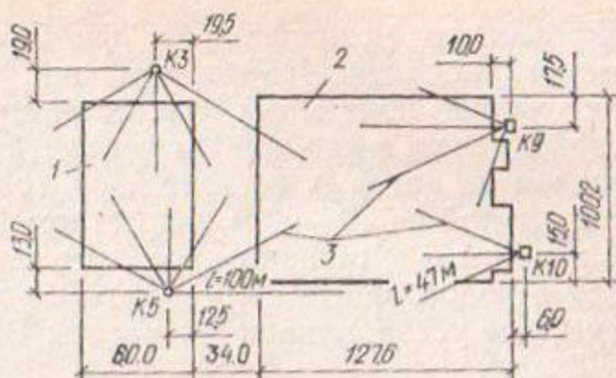
1 — обрубной корпус; 2 — сталеалитовый корпус; 3 — лучи-дрены (КЗ, К5, К9, К10 — колодцы ли- чевых дренажей)
