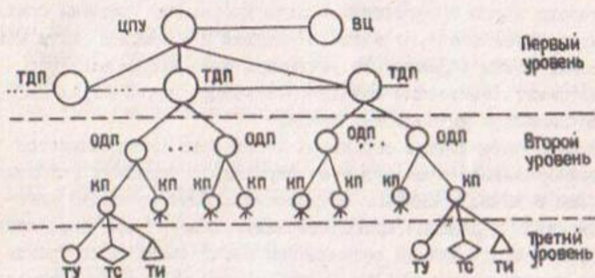
Структура сети связи и ТМ
