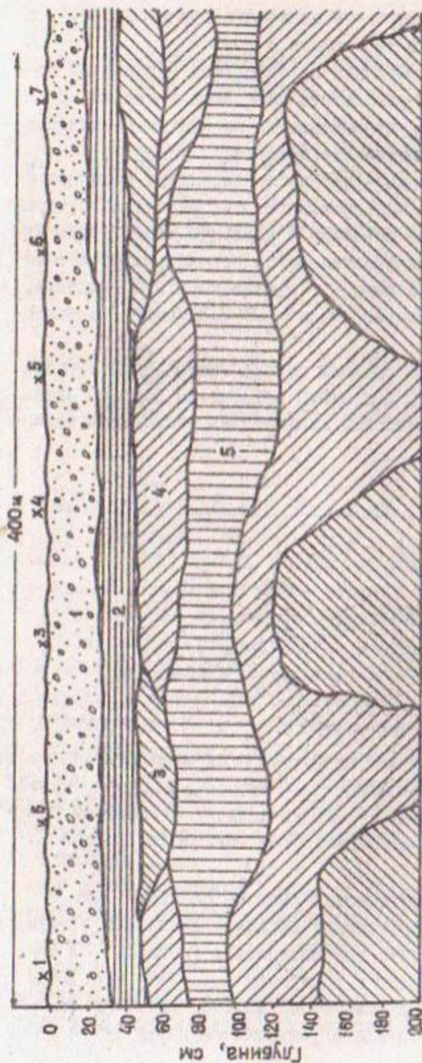
Рис. I. Литологический профиль опытно-производственного участка: I - пахотный легкосуглинистый горизонт с содержанием гипса до 5%; 2 - подпахотный легкосуглинистый плотный слой с содержанием гипса до 5%; 3 - супесчаный горизонт с содержанием гипса 10...25%; 4 - то же, с содержанием гипса 25...50%; 5 - супесчано-песчаный слой с содержанием гипса 50...70%; xI - номер бурфа
