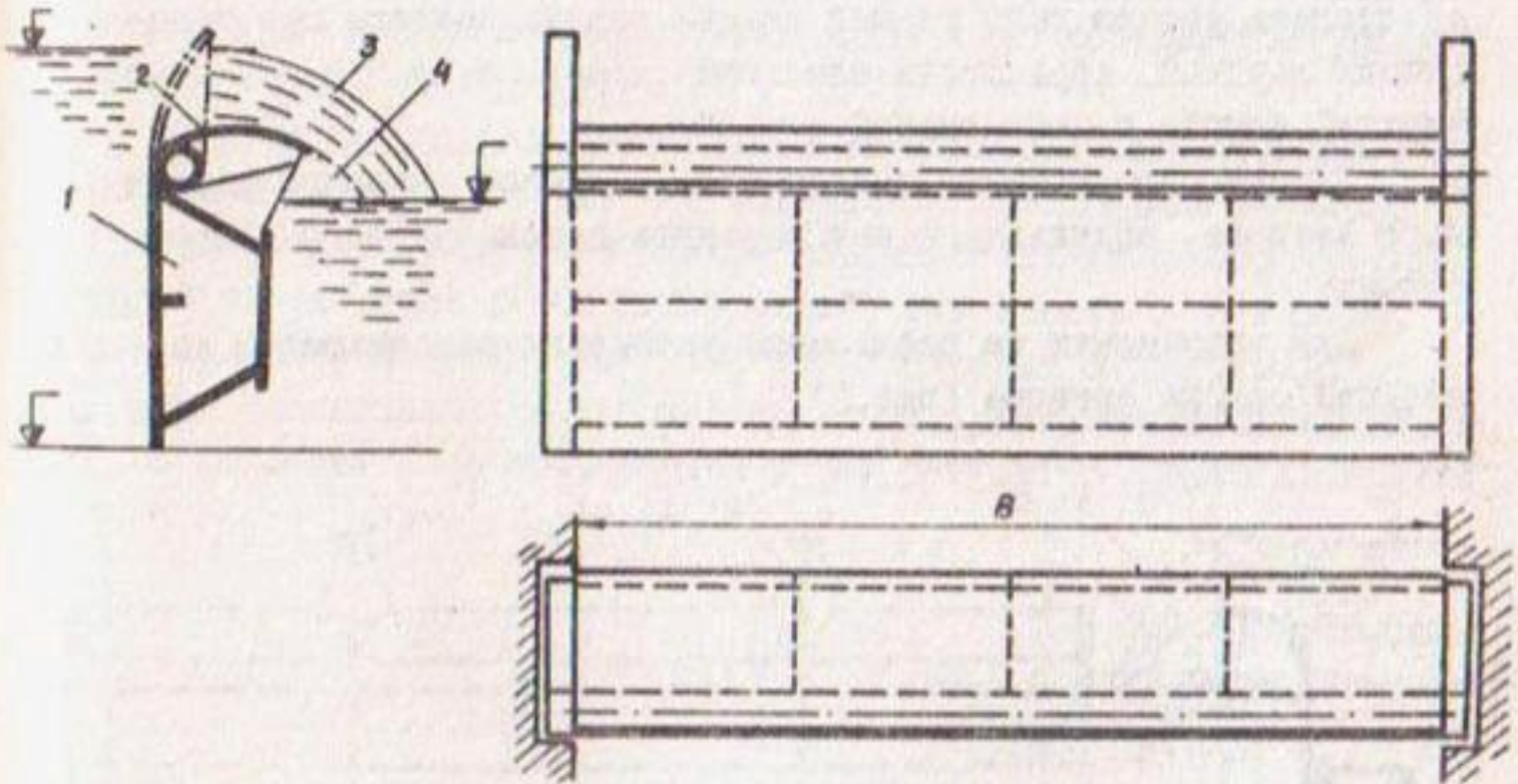
Рис. I. Затвор с клапаном: I - основание затвора; 2 - клапан; 3 - переливаемая струя; 4 - вакуумная полость; В - пролет
