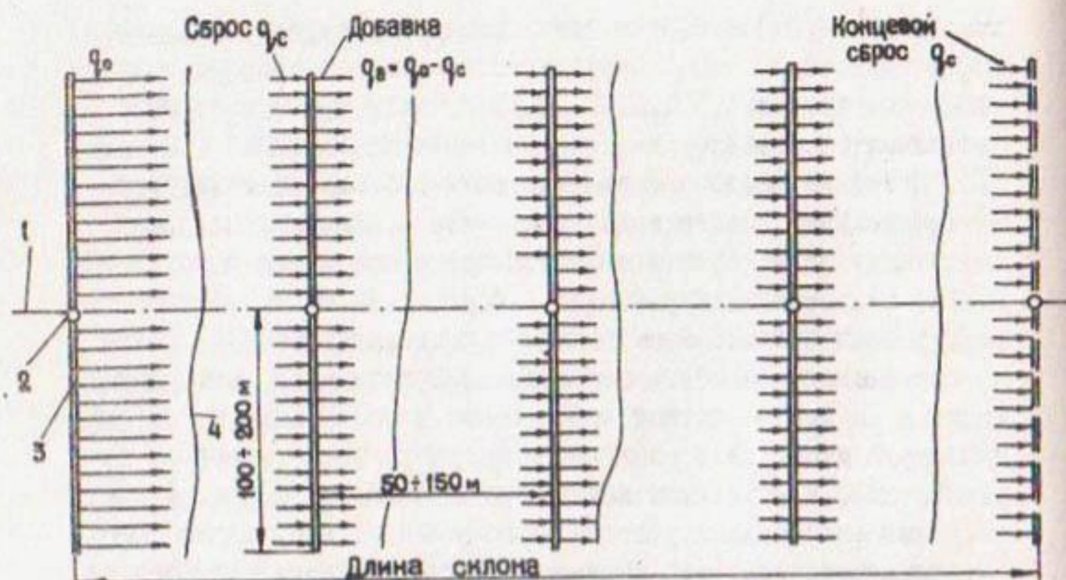
Рис. I. Продольная технологическая схема полива из закрытых оросителей при уклонах 0,005 \dots 0,15 и однообразном рельефе: 1 - закрытый ороситель; 2 - гидрант; 3 - поливной трубопровод; 4 - горизонталь
