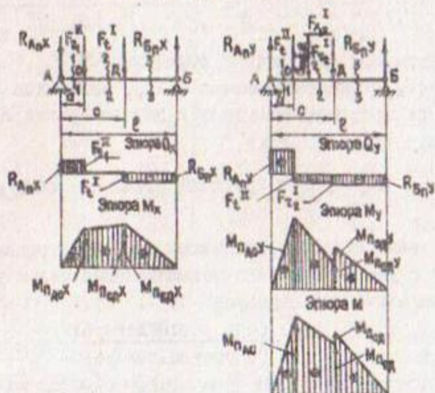
Рис.8. Схемы загрузки промежуточного вала
