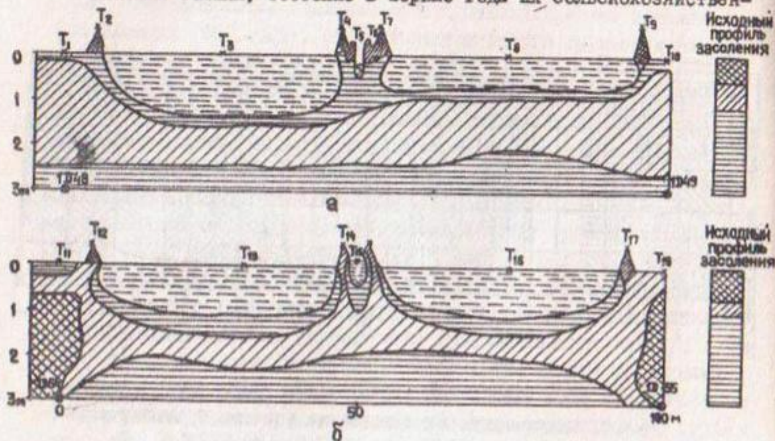
Рис.4. Засоленность почв после промывок: а - междуренье с временной дрена; б - междуренье с временным оросителем: \otimes постоянная дрена; \times скважина солевой съемки. Засоление по Na (мг.экв на 100 г почвы): \square <2; \square 2...6; \square 6...12; \square >12
