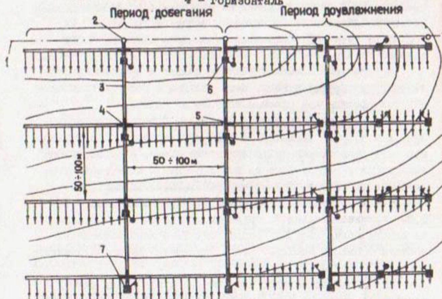
Рис.2. Поперечная технологическая схема полива из закрытых оросителей при уклонах 0,05...0,2 и пересеченном рельефе: 1 - закрытый ороситель; 2 - гидрант; 3 - поливной трубопровод; 4 - крестовина; 5 - тройник; 6 - стабилизатор напора; 7 - ограничитель напора
