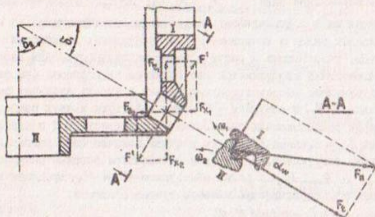
Рис.5. Схема для определения усилий в коническом зубчатом зацеплении
