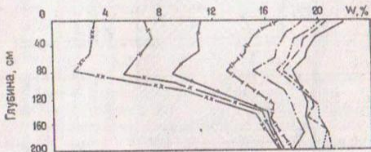
Рис.2. Динамика влажности почвы ( W ) в межполивной период хлопчатника: — первый день; --- второй день; - - - третий день; - . - пятый день; - + - седьмой день; —>— десятый день; —х— пятнадцатый день; —хх— двадцатый день после полива
