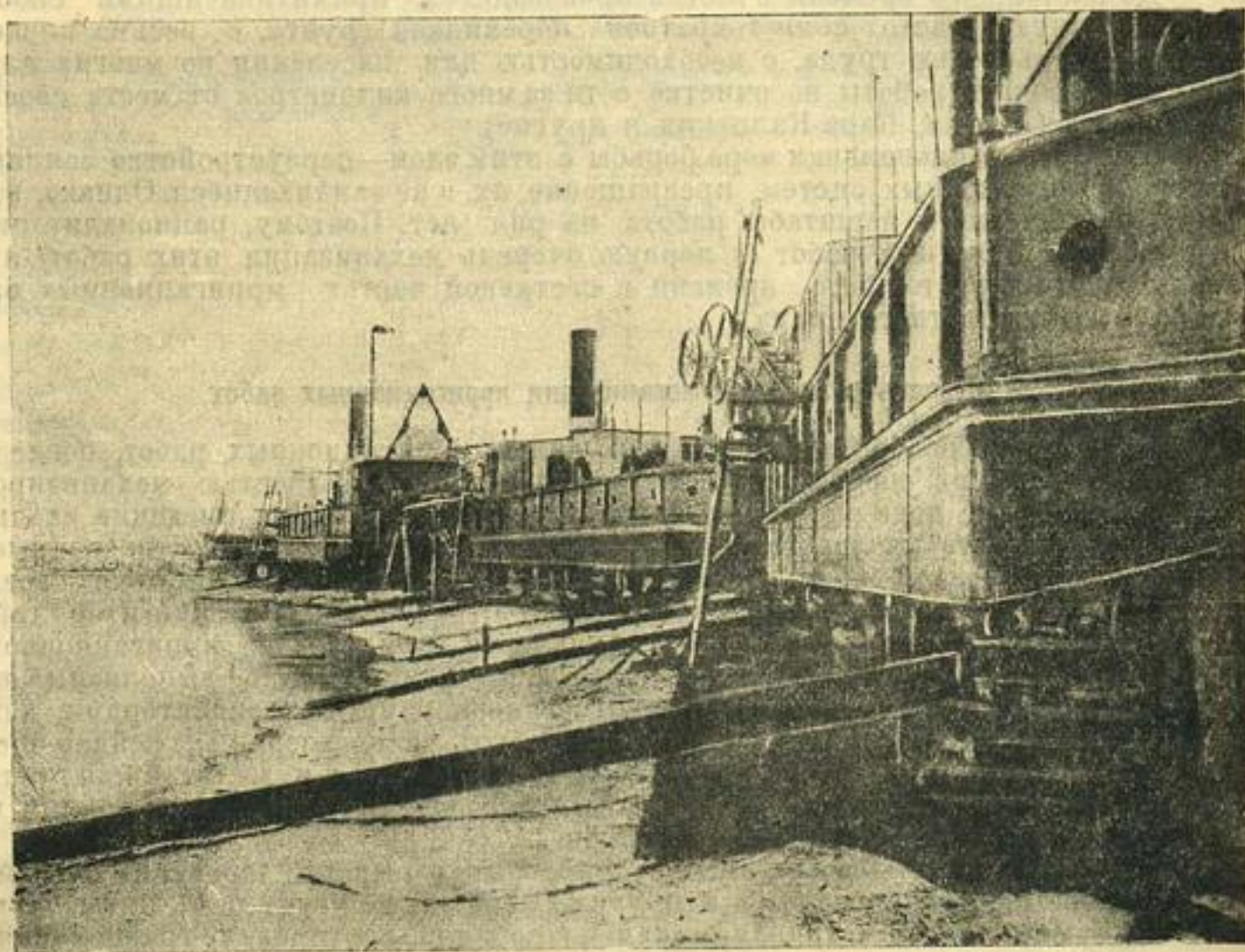
Рис. 11. Землечерпательный караван в Южном Хорезме на Аму-Дарье.
