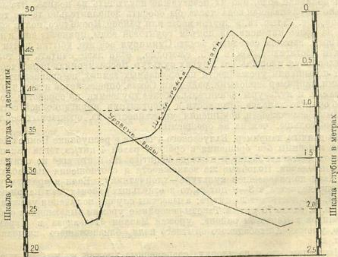
Рис. 10. Шкала урожая хлопка в Египте в зависимости от уровня подпочвенных вод (по Феррару)
