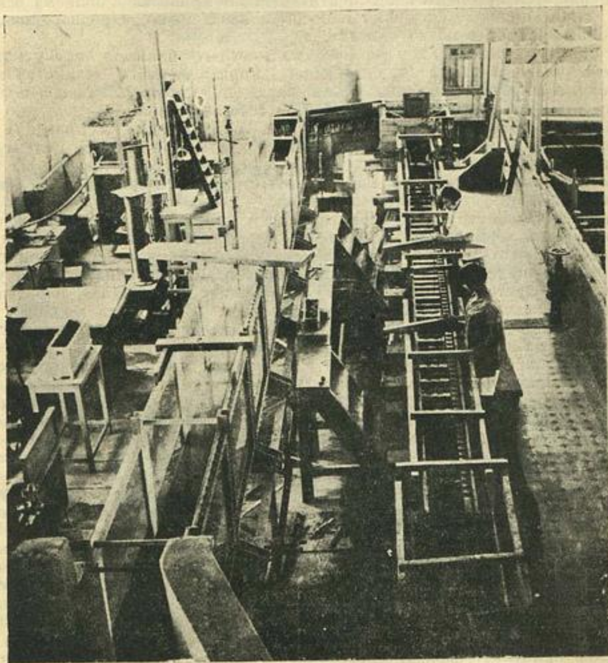
Рис. 16. Гидротехническая лаборатория. Производство замеров при испытании Вахшского быстротока
