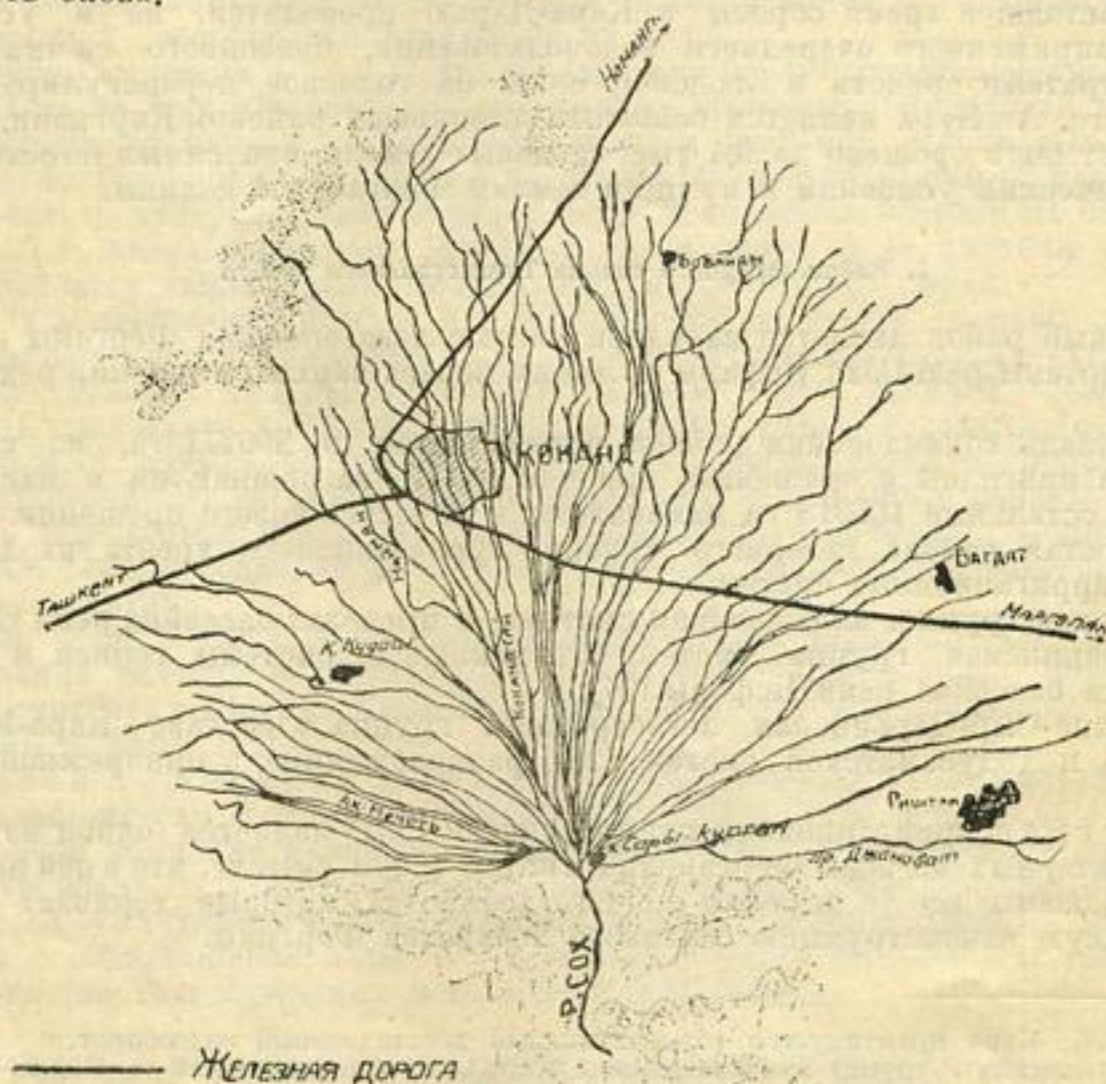
Рис. 3. Схема ирригационной сети Сохского веера
