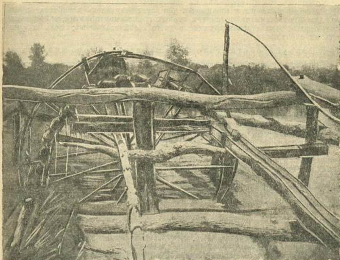
Рис. 6. Местная самодействующая водоподъемная установка—«чигир».
