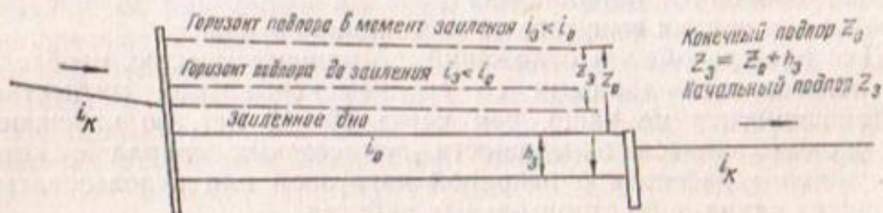
Рис. 4. Схема отстойника третьего типа.
