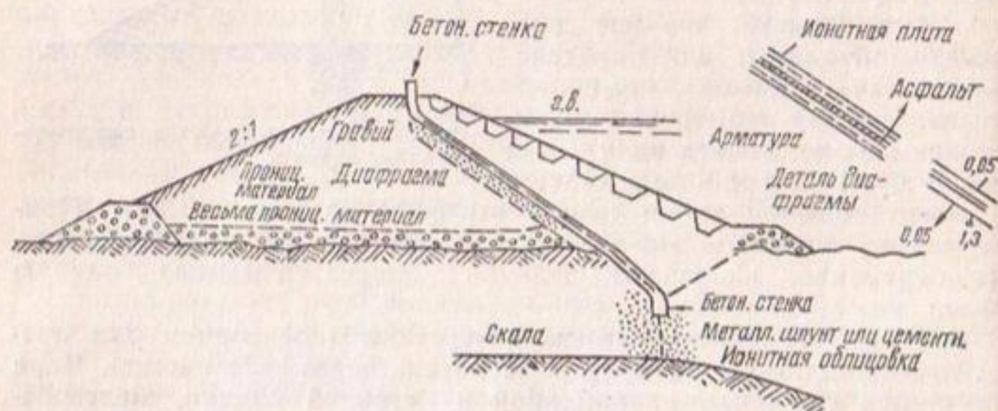
Рис. 8. Поперечное сечение плотины и диафрагмы.
