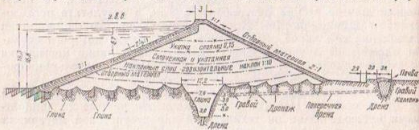
Рис. 5. Дренаж плотины.
