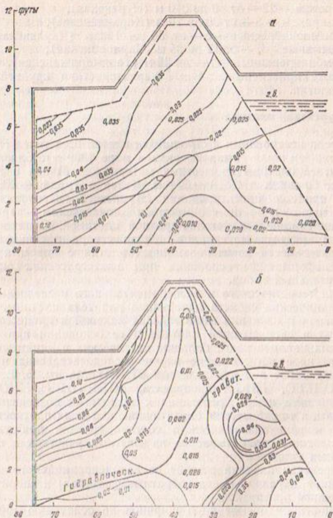
Рис. 10. Распределение материала намыва по эффективному размеру зерен при подаче с низовой стороны (а) и с обеих откосов (б).
