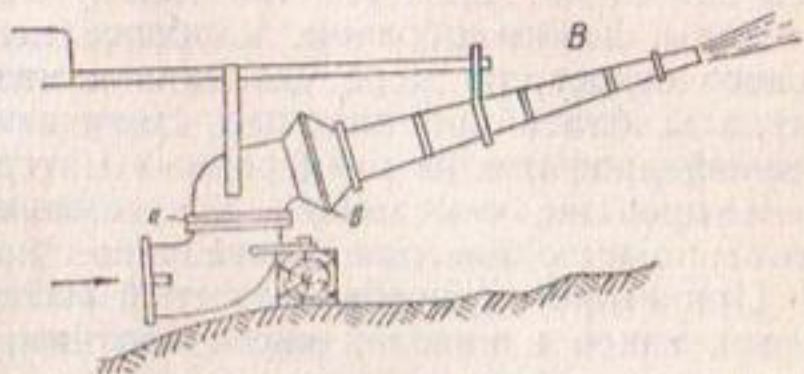
Рис. 9. Двухшарнирный монитор.
