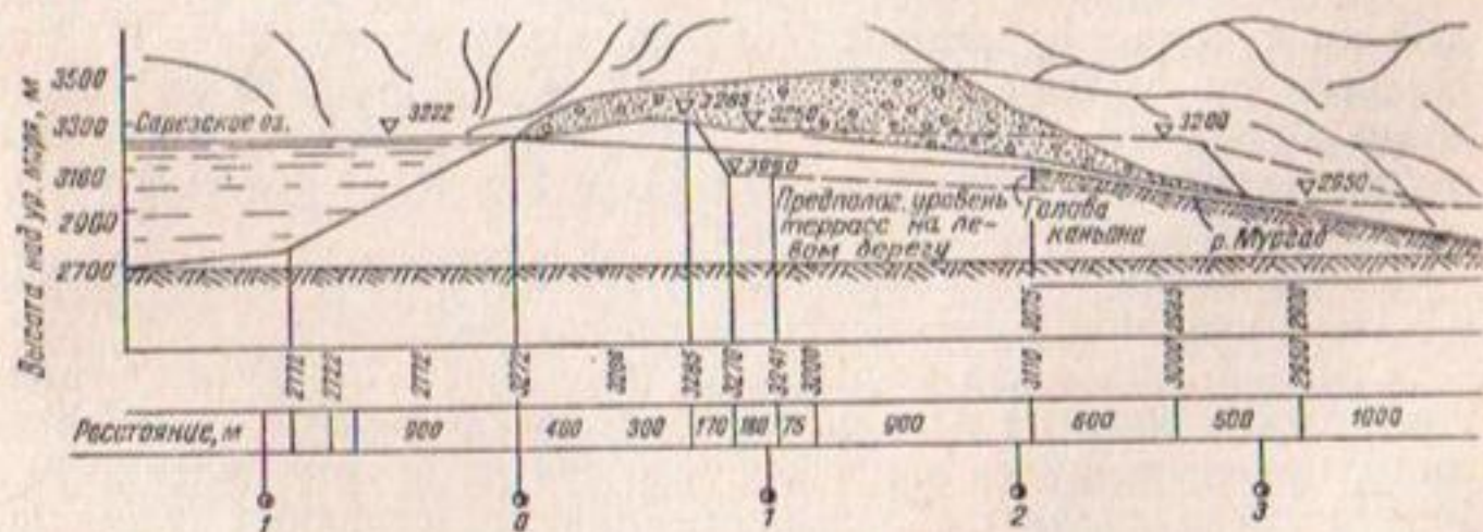
Рис. 4. Поперечный профиль через пониженную часть завала, далее вдоль подошвы главного хребта завала и по руслу р. Мургаба (Бартанг).
