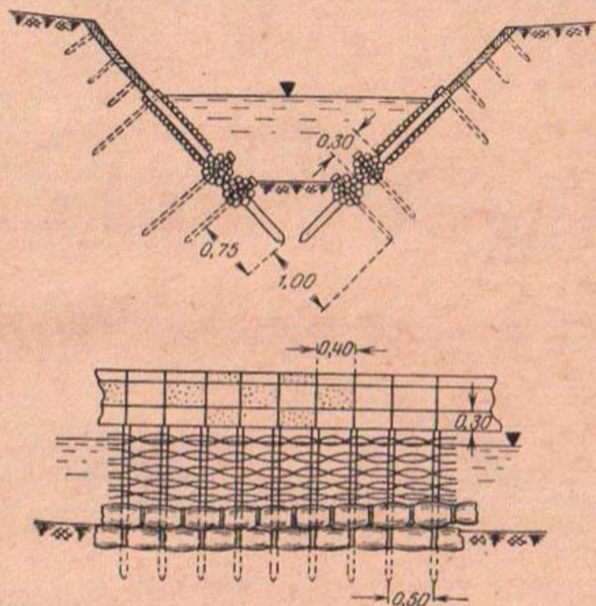
Рис. 53. Крепление откосов осушительного канала с применением fascии, плетня и дерна.
