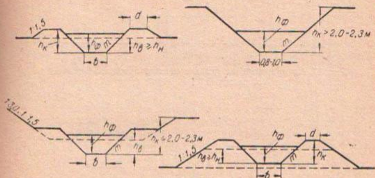
Рис. 16. Стандартные сечения каналов оросительной сети на расходы до 1,0 м 3 /сек.
