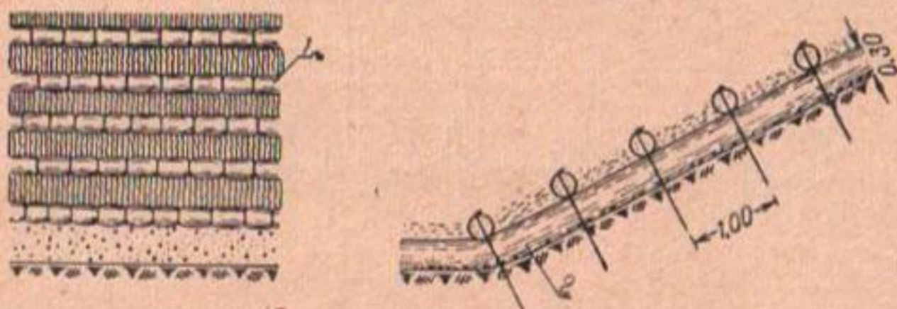
Рис. 50. Применение хворостяной выстилки и фашинных канатов для крепления откосов:
