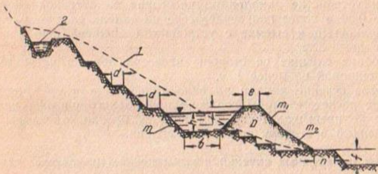
Рис. 10. Типовое поперечное сечение канала на косогорном участке:
