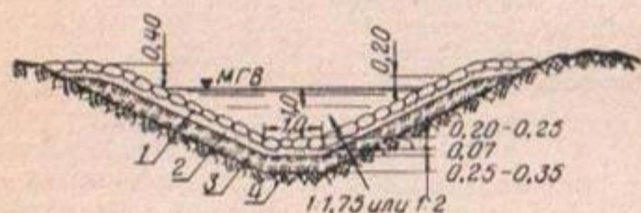
Рис. 37. Глиняная облицовка с защитным слоем из одиночной мостовой:
