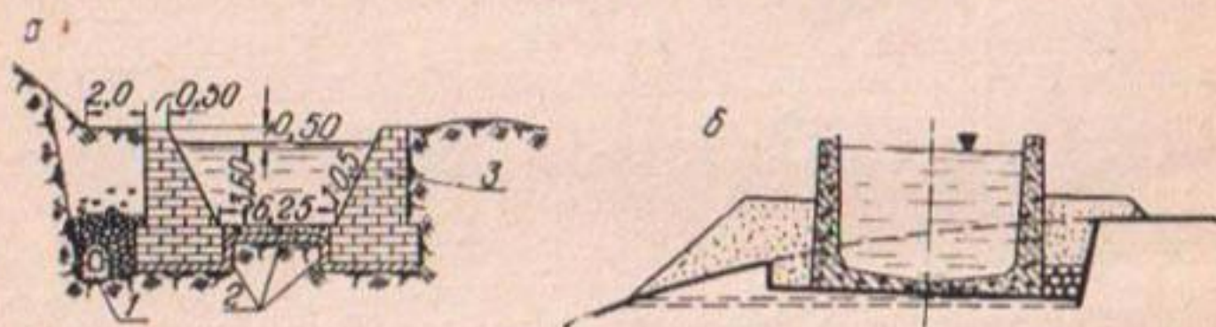
Рис. 44. Лотки на сплошных основаниях:
