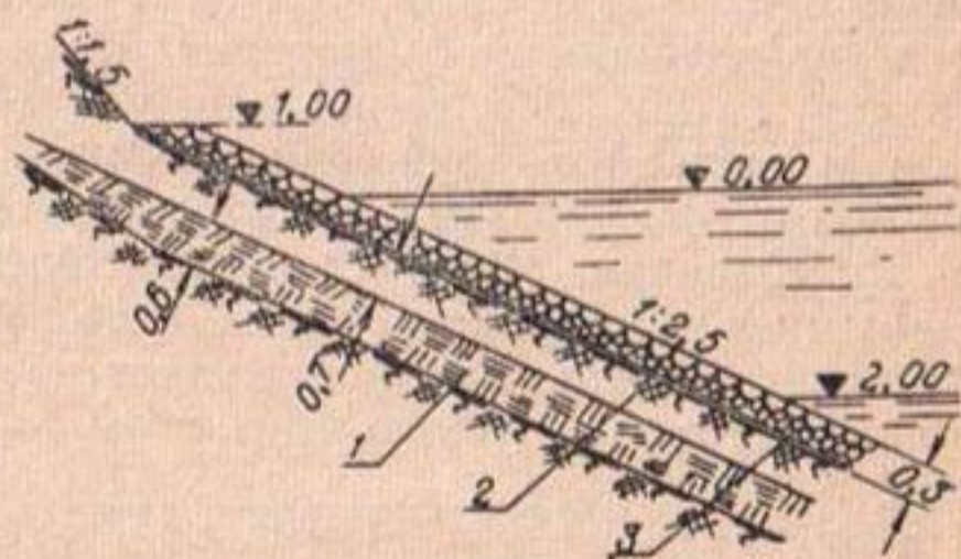
Рис. 36. Тип крепления из каменной наброски:
