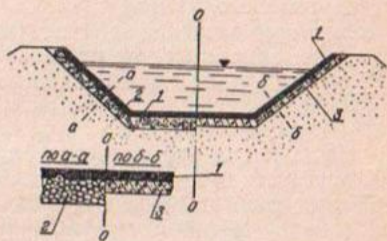
Рис. 34. Асфальтированная облицовка: 1 — облицовка; 2 — подготовка; 3 — жесткое основание из бетона или грунтоцемента.
