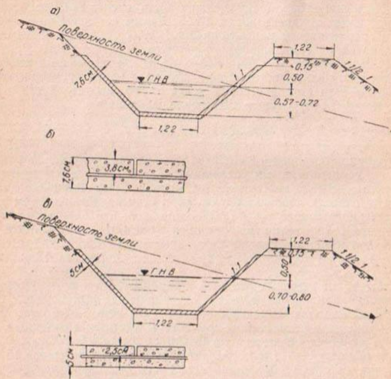
Рис. 25. Типовая конструкция бетонной (а) и торкретной (б) облицовок канала с деталями поперечных температурных швов (б и г).
