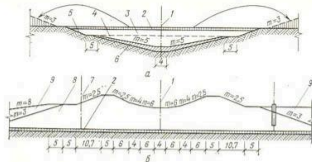
Рис. 32. Технологии строительства II очереди Большого Ставропольского канала: а, б — канал в выемке и в насыпи; 1 — ось канала; 2 — срезка растительного слоя; 3, 4 — грунт, разработанный соответственно скреперами и экскаваторами; 5 — покрытие откосов растительным слоем; 6 — грунт, разработанный бульдозерами при срезке защитного слоя под экран; 7 — ось дренажа; 8, 9 — уплотненная и неуплотненная насыпи. (Размеры в м.)
