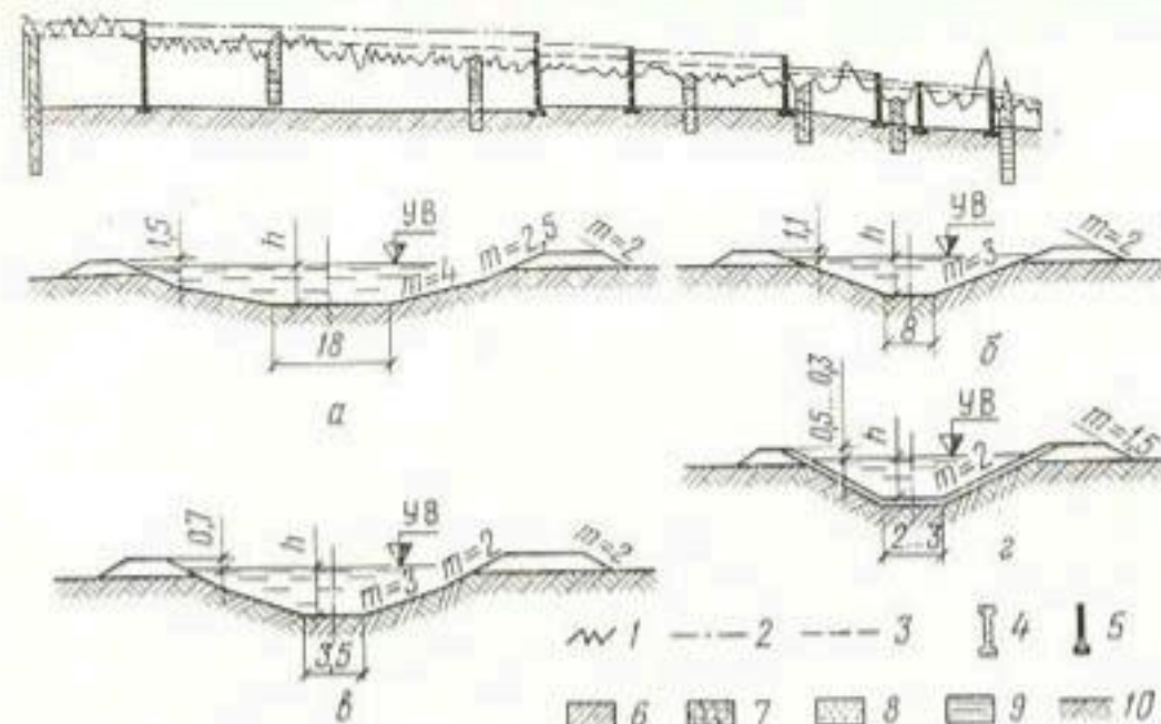
Рис. 20. Продольный и поперечный профили Южно-Голодноостепского канала им. А. А. Саркисова:
