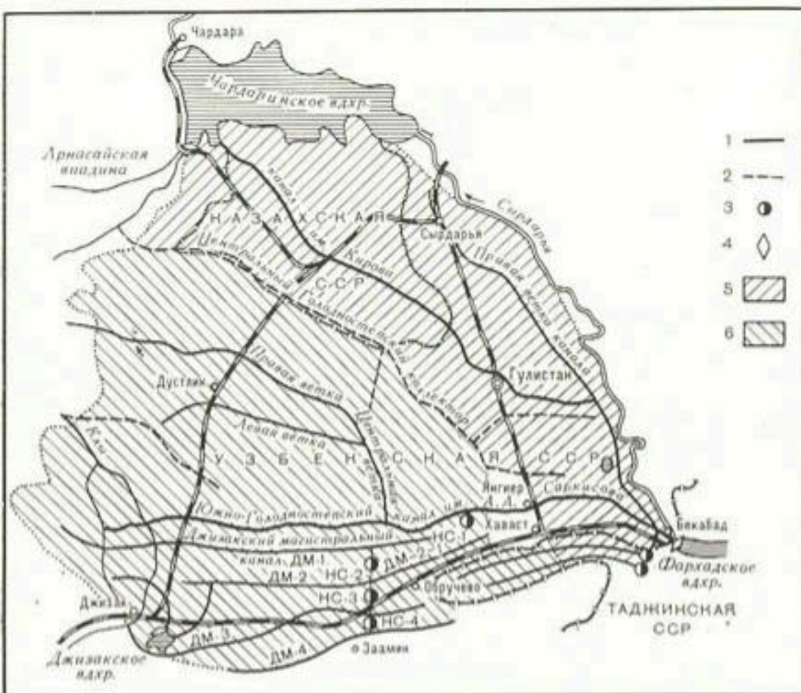
Рис. 19. Схемы Южно-Голодноостепского канала им. А. А. Саркисова и Джизакского магистрального канала ДМ-1:
