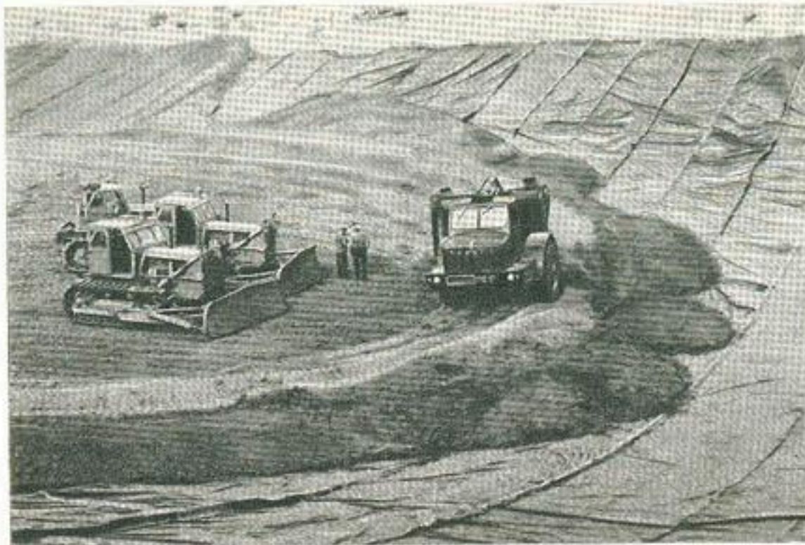
Рис. 26. Покрывание пленочного противодиффузионного экрана Главного Каховского магистрального канала защитным слоем суглинистого грунта.
