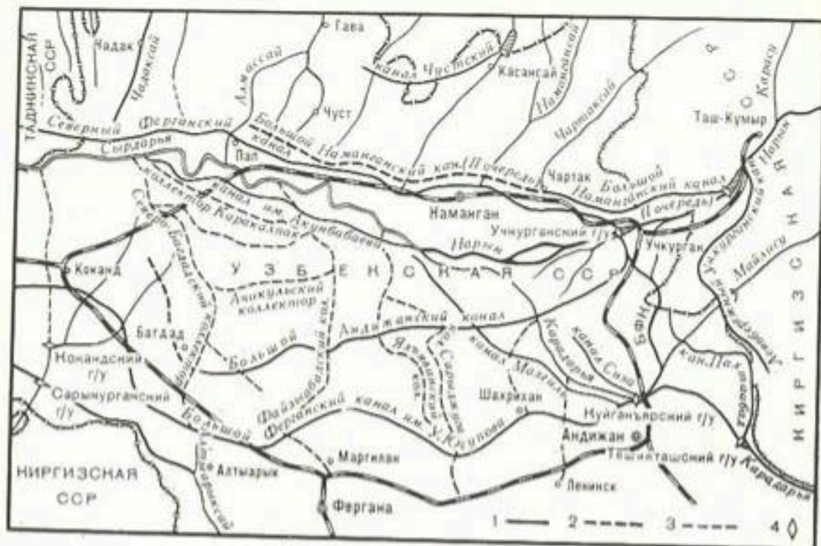
Рис. 8. Схемы Большого Андижанского и Большого Наманганского каналов: 1 — каналы; 2 — II очередь строительства каналов; 3 — коллекторы; 4 — гидроузлы.
