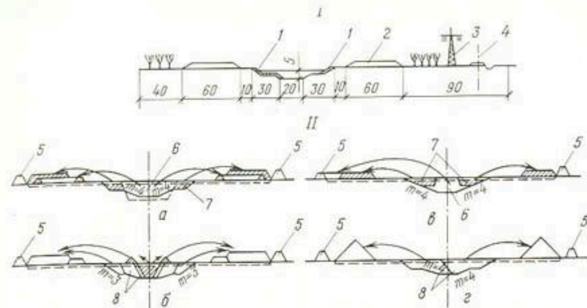
Рис. 28. Поперечное сечение канала Днепр — Донбасс и схемы механизации: I — типовое поперечное сечение канала; II — технологические схемы разработки выемки канала: а — схемы разработки участка от 0 до 166-го километра; б — то же, от 166 до 198-го километра; в — то же, от 198 до 208-го километра; 2 — участок канала, разработанный экскаваторами ЭИИ-5/45; 1 — крепление щебнем; 2 — кавальер; 3 — линия электропередачи 35 кВ; 4 — автомобильная дорога; 5 — кавальер срезки растительного слоя; 6 — грунт, разработанный земснарядами; 7 — береговые траншеи (разработаны экскаваторами драглайн); 8 — забой экскаваторов. (Размеры в м.)
