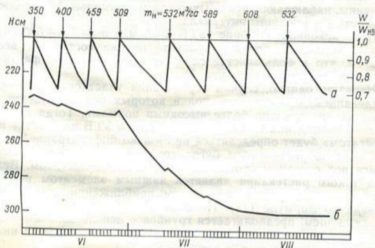
Рис. 34. Вариант режима орошения хлопчатника дождевальной машиной «Фрегат» при глубине УГВ 2—3 м. Штриховкой отмечен период работы машины. Остальные обозначения см. рис. 32.
