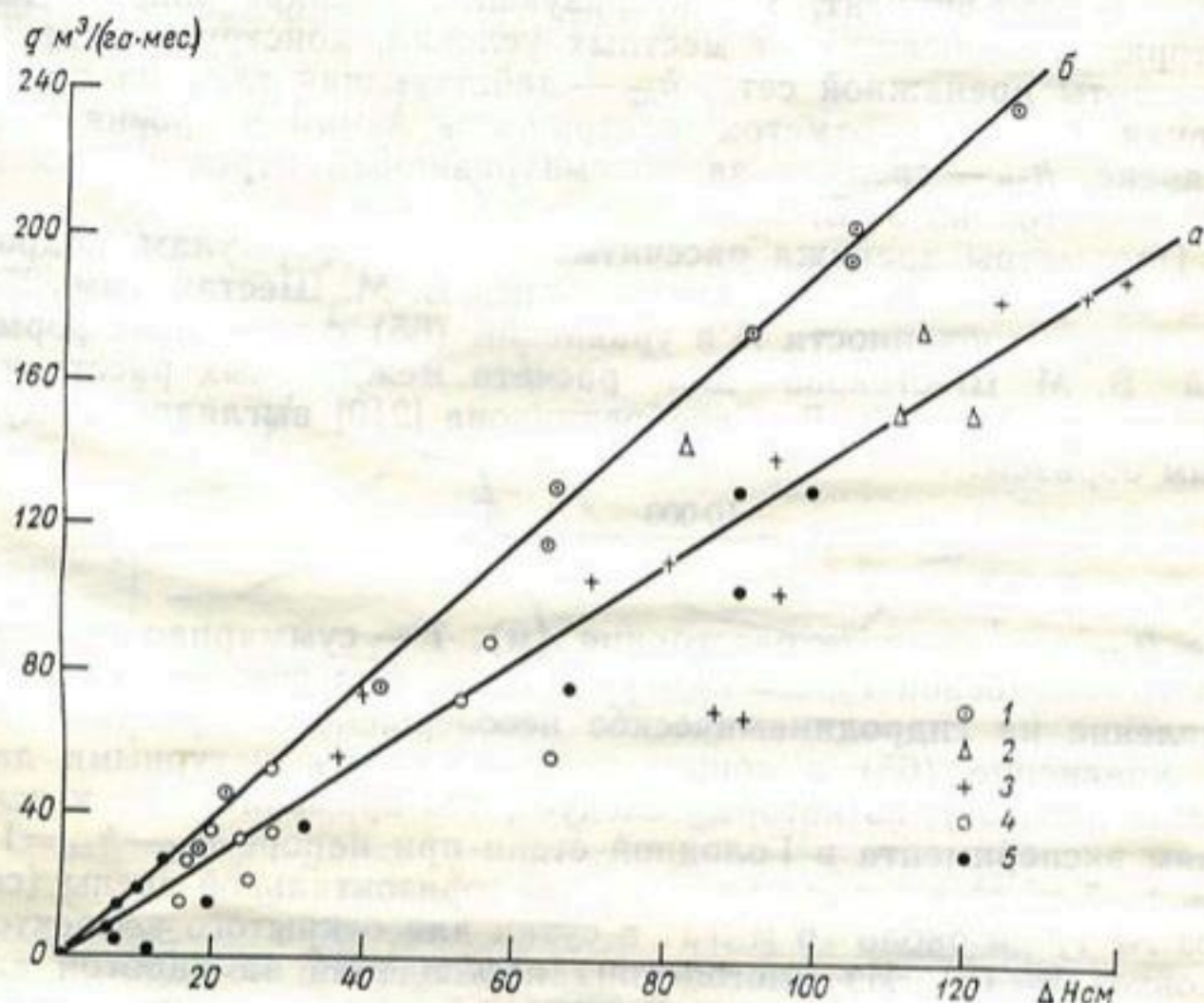
Рис. 37. Зависимость дренажного стока от напора в середине междуренья \Delta H .
