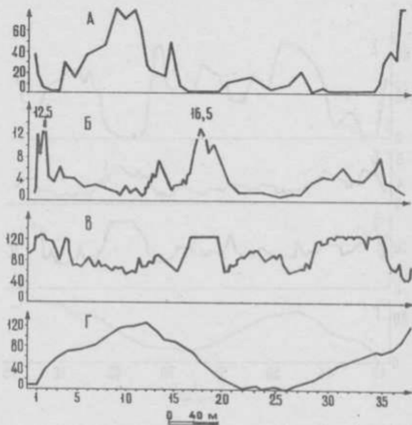
Рис. 30. Характеристика клеевого участка, полученная по профилю 1:
