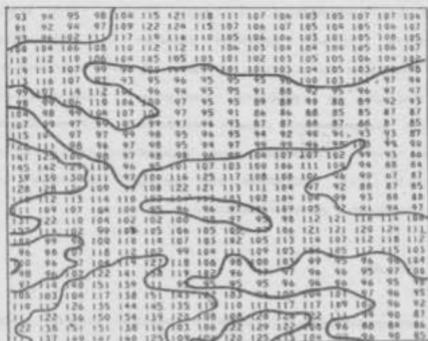
Рис. 5. Результат обработки сканерной информации. Фрагмент оцифрованного сканерного изображения поля хлопчатника свидетельствует о неоднородности поля
