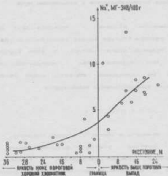
Рис. 29. Зависимость среднеевменного засоления почвы в слое 0-100 см от расстояния до границы ближайшего выпад (после корректировки фотонизображения и включения скважин, заложённых в контурах выпадов)
