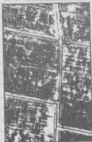
Рис. 18. Динамика засоления почв, установленная при сопоставлении фотонизображения полей хлопчатника по осенним аэрофотоснимкам
