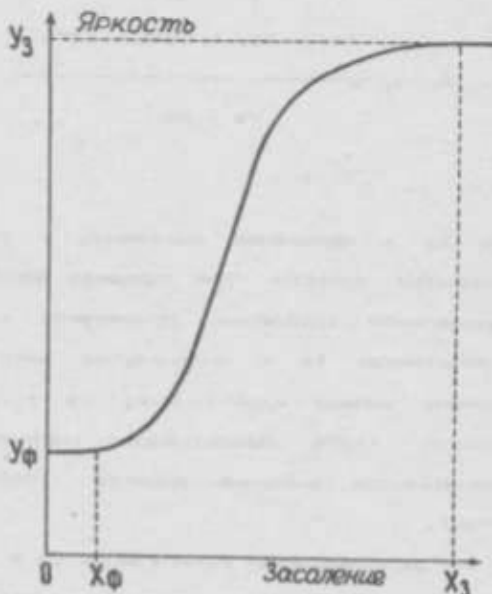
Рис. 28. Принципиальный вид зависимости яркости фотонизображения от засоления почвы: X_\Phi - минимальное засоление, приводящее к угнетению хлопчатника; X_3 - максимальное засоление, при котором происходит полный выпад растений; Y_\Phi - яркость при 100%-ном проективном покрытии хлопчатника; Y_3 - яркость при полном отсутствии растений (100% открытой поверхности почвы)
