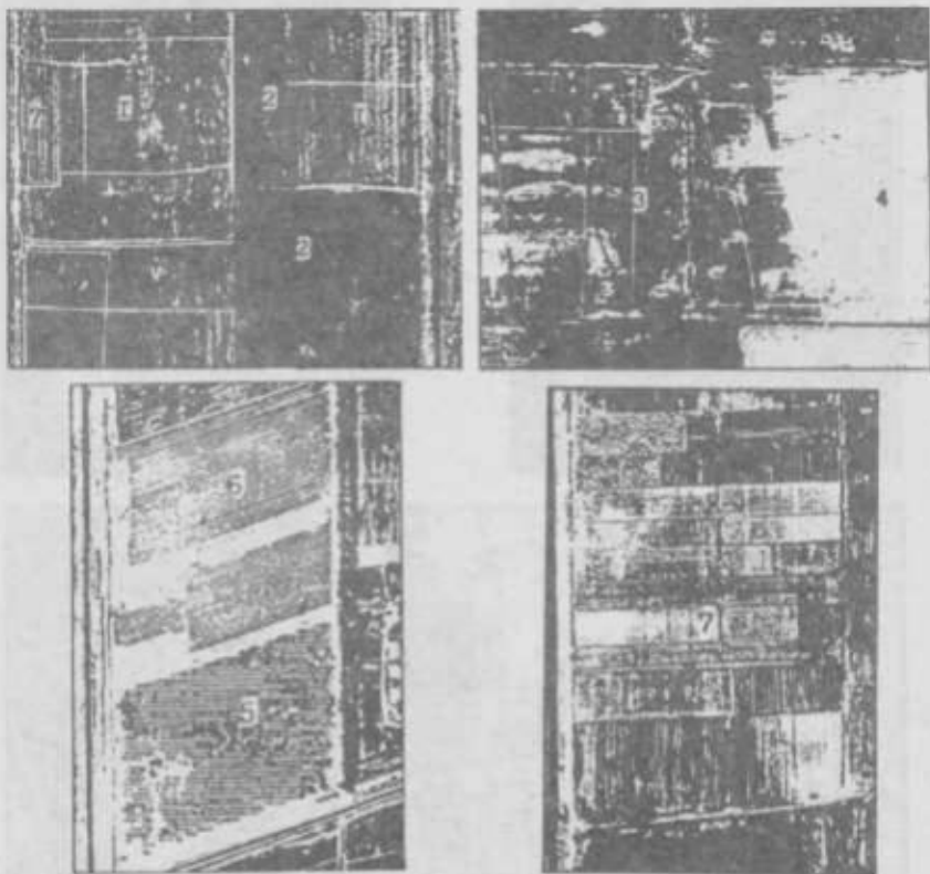
Рис. 12. Фотоизображение различных сельскохозяйственных культур на раннеосенних аэрофотоснимках масштаба 1:100000: 1 — хлопчатник; 2 — кукуруза; 3 — люцерна; 4 — люцерна скошенная; 5 — сады; 6 — виноградники; 7 — бабки, огороды
