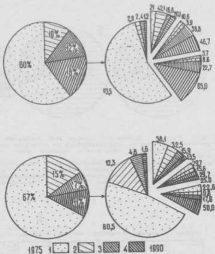
Рис. 24. Направление солевого процесса в землях НЗО Голодной (А) и Дзизакской (Б) степей при различном исходном засолении почвы.
