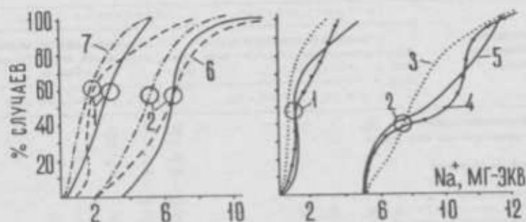
Рис. 10. Характеристика засоления почв неоднородных по фото-изображению контуров: 1 - темные компоненты контуров; 2 - светлые.
