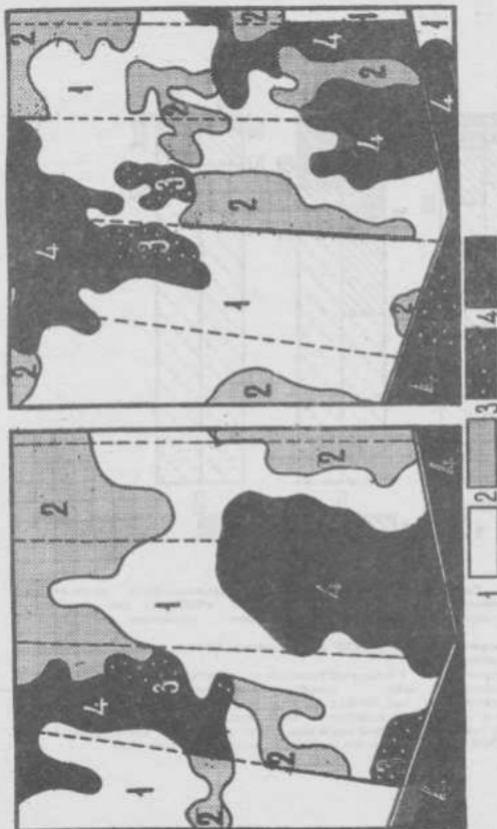
Рис. 19. Фрагменты карт засоления почвы на одну и ту же территории: А - 1975г., Б - 1989г. Показ: 1 - преимущественно незасоленные и слабозасоленные; 2 - преимущественно средnezасоленные с участком слабозасоленными; 3 - преимущественно средnezасоленные с участком сильнозасоленными; 4 - преимущественно сильнозасоленные.
