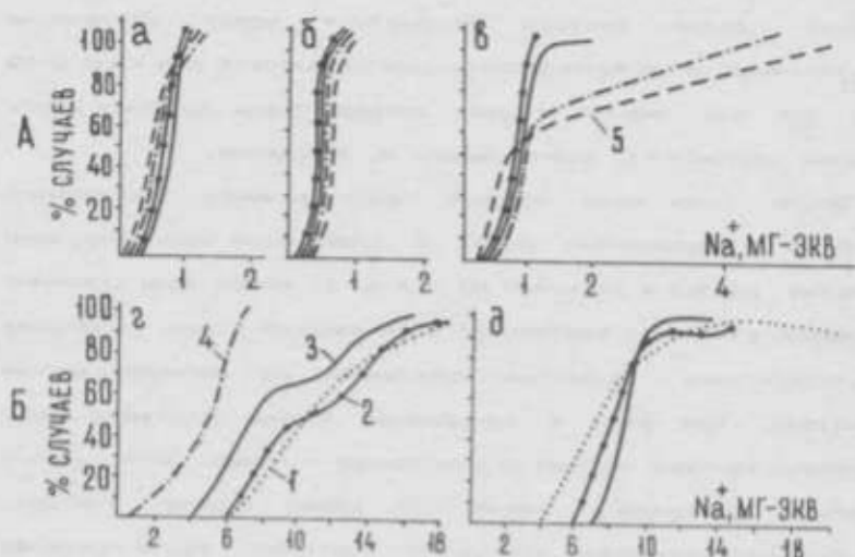
Рис. 9. Характеристика засоления почв однородных (однотонных) по фотонзображению тенных (А) и светлых (Б) контуров по слоям: 1 - 0-25 см; 2 - 0-50 см; 3 - 0-100 см; 4 - 100-200 см; 5 - 200-300 см. Участки: а - 5 н; б - 6 н; в - 8 н; г - 29 н; д - 30 н
