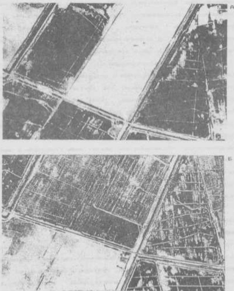
Рис. 3. Дешифрирование по аэрофотоснимкам состояния кормовых культур.
