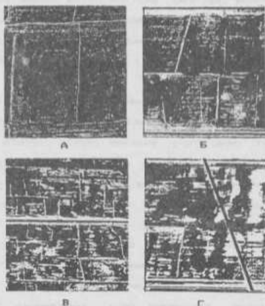
Рис.8. Фотоизображение полей клеверника на черно-белых панхроматических крупномасштабных аэрофотоснимках осеннего срока залета:
