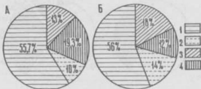
Рис. 22. Баланс орошаемых земель НЗО Голодной (А) и Джизакской (Б) степей, различавшихся по динамике засоления почв, полученный в результате анализа карт динамики засоления почв.
