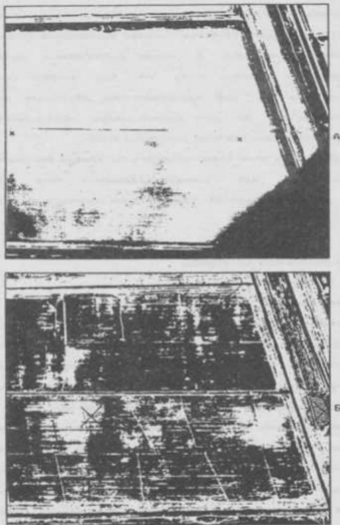
Рис. 2. Аэрофотосъемки весенних (А) и позднелетних (Б) сроков съемки:
