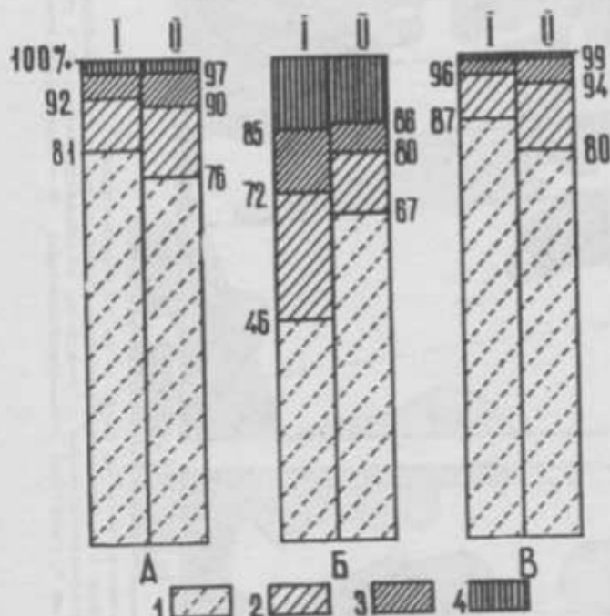
Рис. 20. Сравнение площадей почв различного засоления, подсчитанных по картам 1975 и 1986 гг. по основным почвенно-агролого-геоморфологическим районам Голодной степи.
