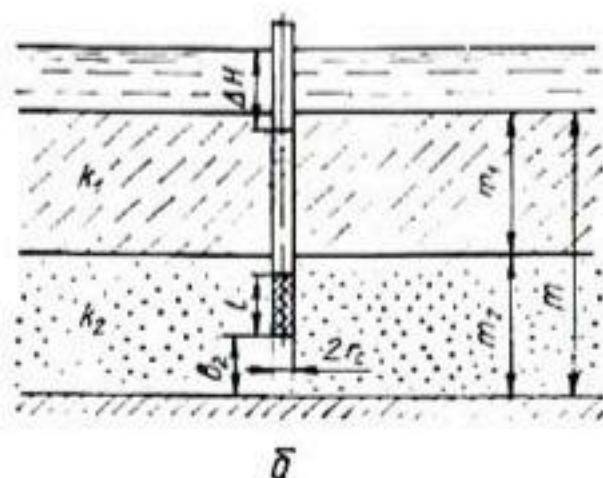
Рис. 11. Схемы фильтрации к несовершенным скважинам в двухслойном грунте: а — при инфильтрационном и напорном питании; б — при питании из водоема.
