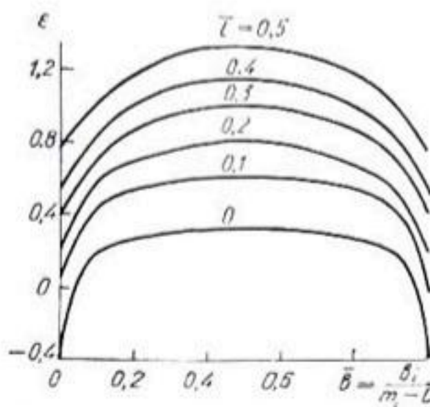
Рис. 5. График для определения параметра \epsilon .
