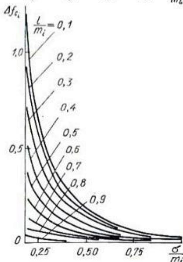
Рис. 6. График для определения добавочного сопротивления \Delta f_{c_i} .
