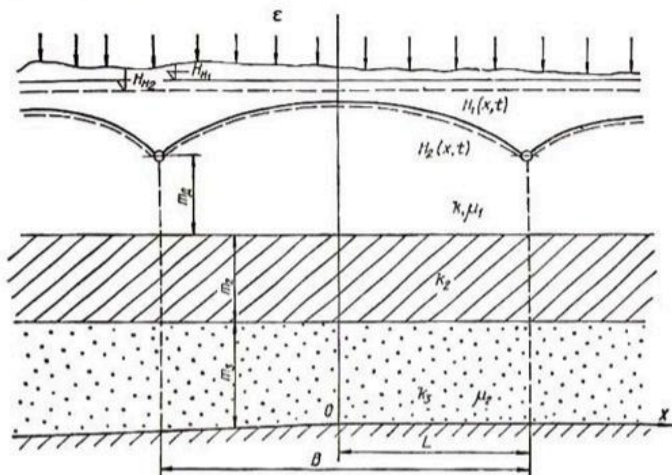
Рис. 37. Схема неустановившейся фильтрации к систематическому дренажу в трехслойном грунте.
