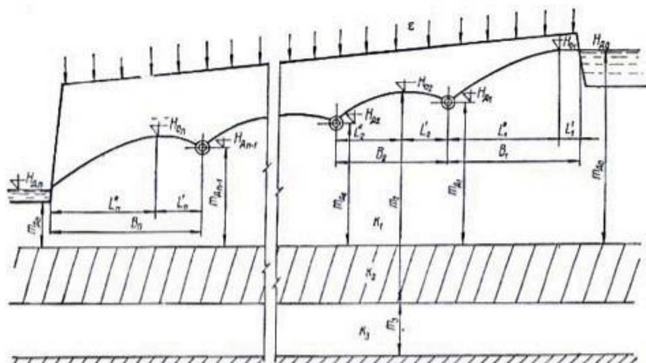
Рис. 28. Расчетная схема дренажа с различным расположением дрен на массиве.
