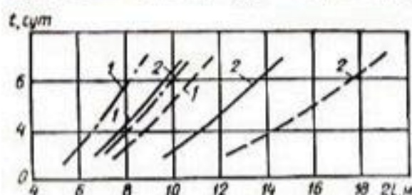
Рис. 58. Зависимость расстояний L от времени в случаях неплотного рыхления (сплошная линия), сплошного рыхления (пунктирная линия), без рыхления (штрихпунктирная линия) при \bar{h} = 0,6 м (1) и \bar{h} = 0,5 м (2).
