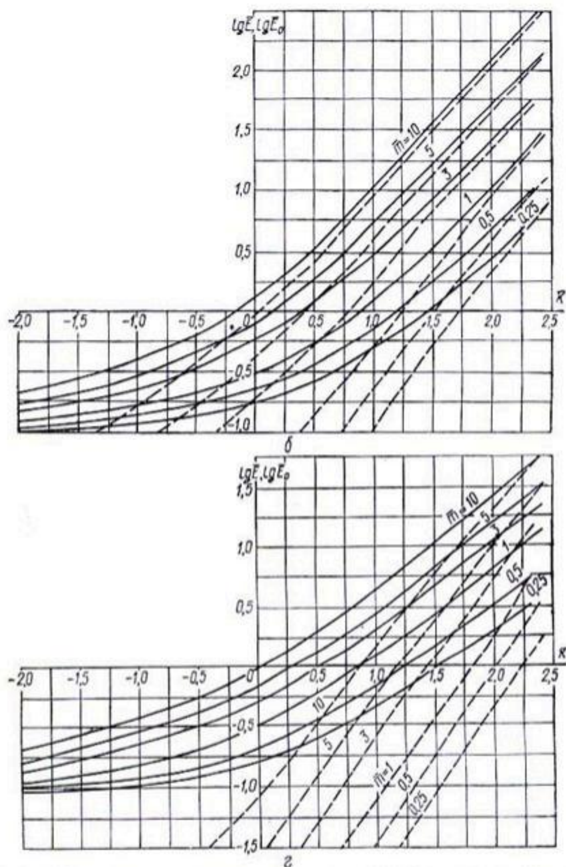
Рис. 13. Графики для определения параметров \bar{E} (сплошная линия) и \bar{E}_0 (штриховая линия) при значениях B/m_1 = 5 (а), 10 (б), 20 (в) и более 40 (г).
