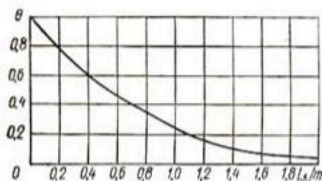
Рис. 26. График для определения параметра \theta .
