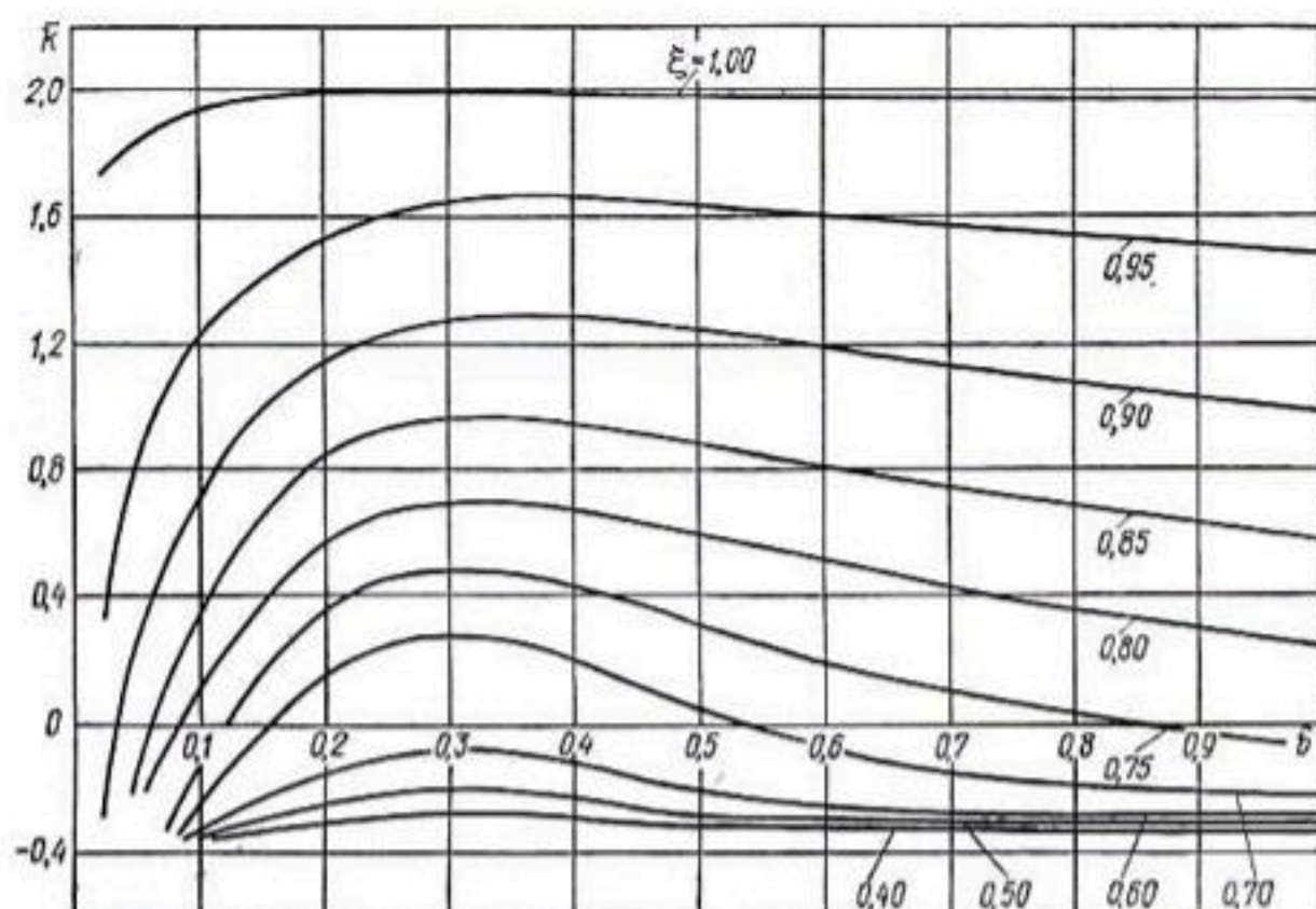
Рис. 14. График для определения поправочного коэффициента \bar{\epsilon} .
