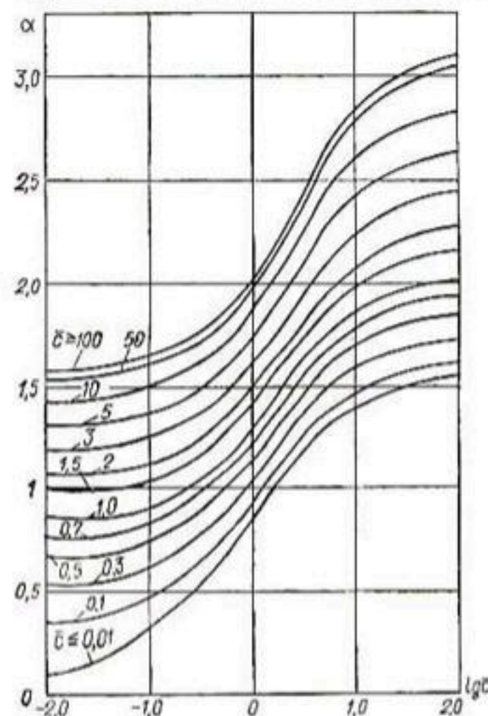
Рис. 39. Графики для определения коэффициента \alpha .
