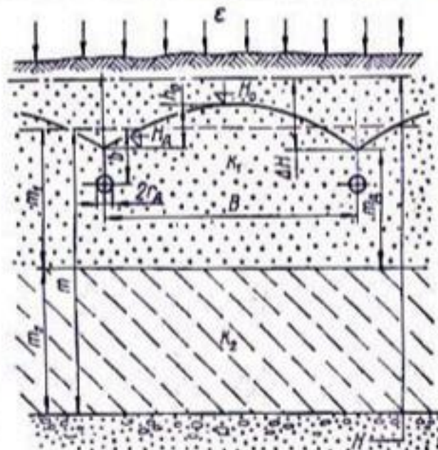
Рис. 12. Расчетная схема систематического дренажа в двухслойном грунте с инфильтрационным и напорным питаниями.
