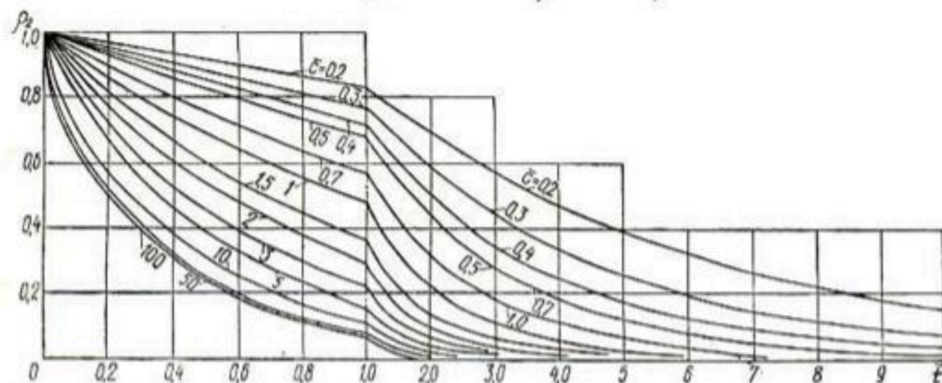
Рис. 43. Графики для определения коэффициента \beta_2 .
