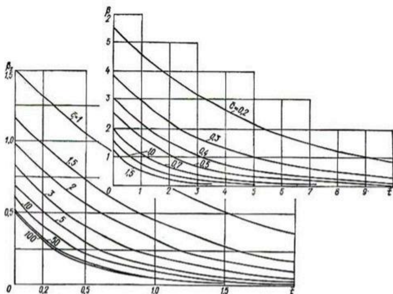
Рис. 41. Графики для определения коэффициента \beta_2 .
