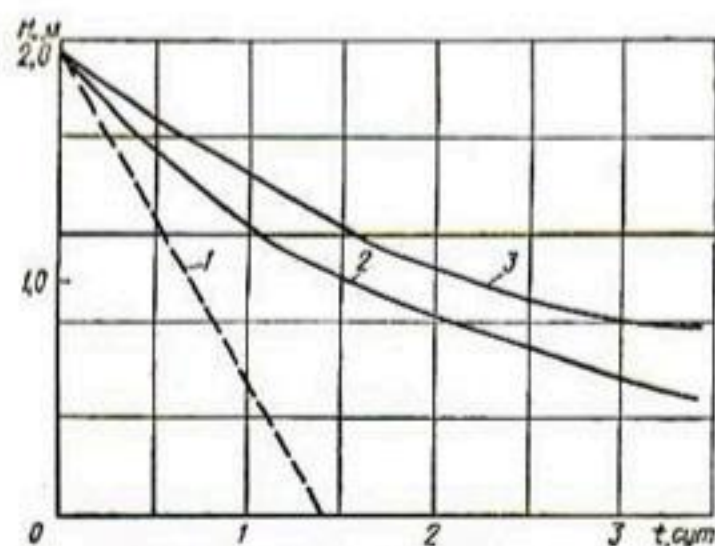
Рис. 52. Уровни H_*(t) в засыпке, вычисленные по формулам (9.49) (1), (9.45) и (9.47) (2) и рассчитанные на ЭВМ (3).
