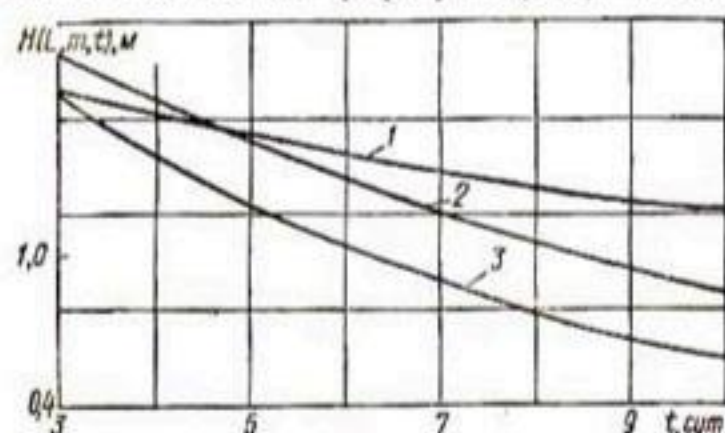
Рис. 49. Уровни H(L, m, t) посередине между дренами, вычисленные по формулам (9.67) (1), (9.8) (2) и (9.20) (3).
