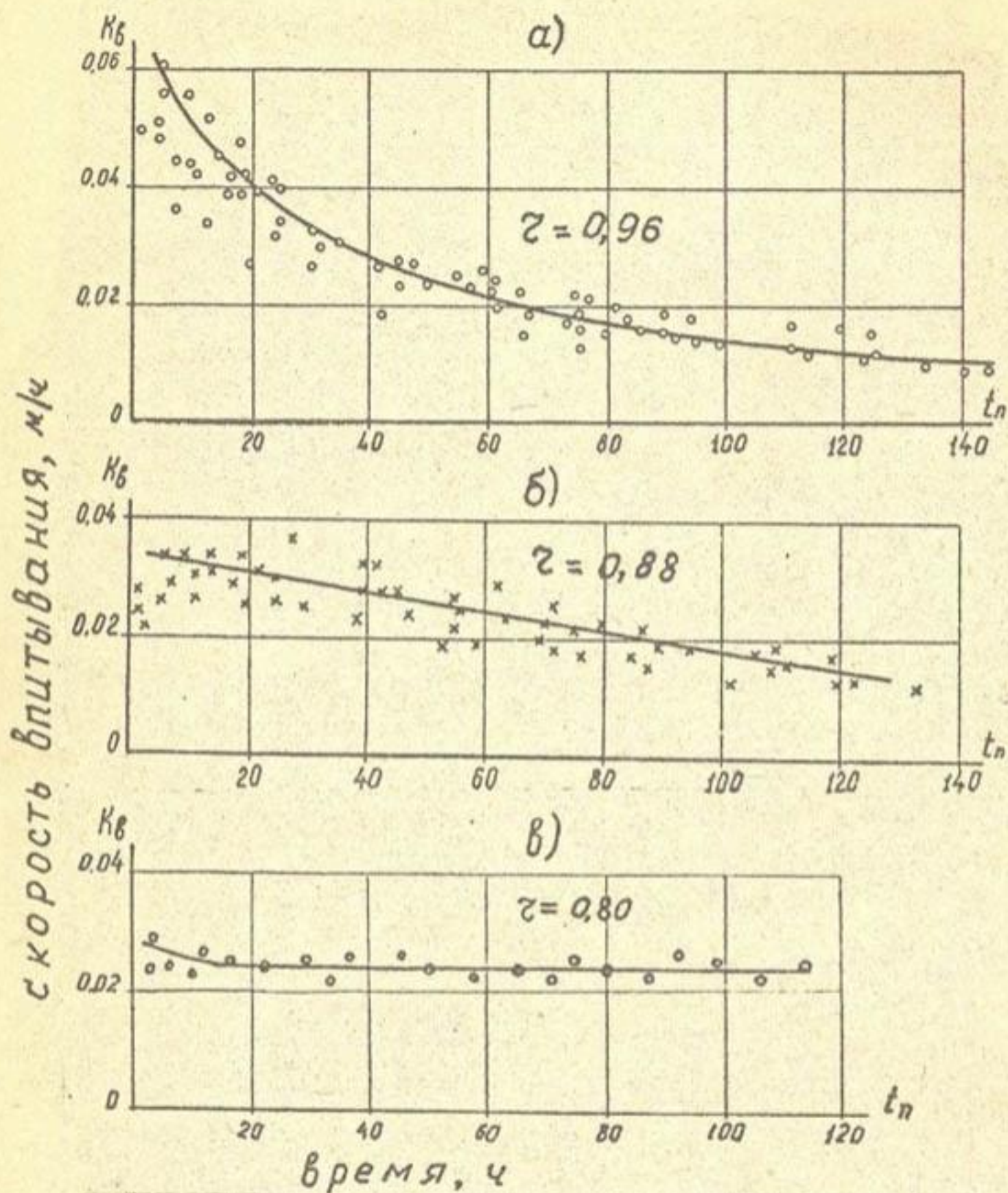
Рис. 2.12. Характер изменения скорости впитывания воды во времени на различных участках зигзагообразной микророзды (а - в начале K_{изв} = 1,0 ; б - середине, K_{изв} = 1,5 ; в - в конце K_{изв} = 2,5 , r - коэффициент корреляции).
