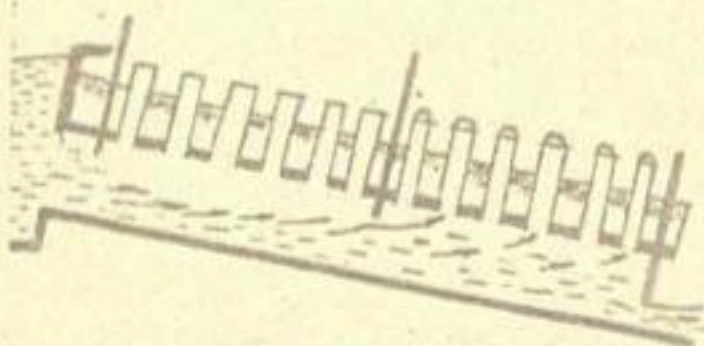
Рис. 3.8. Существующие типы водовыпусков из трубчатой сети в поливные борозды.
