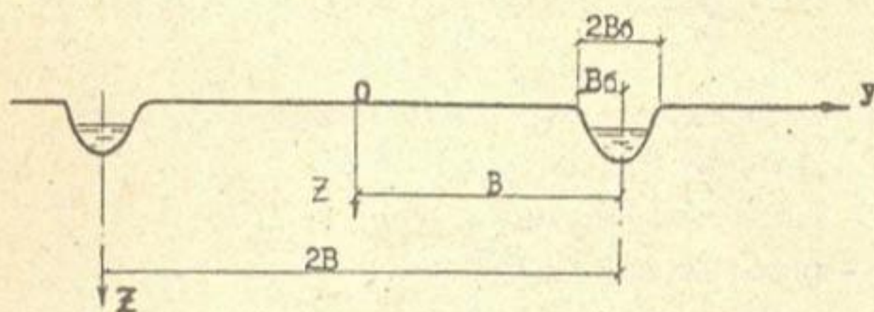
Рис. I.8. Расчетная схема
