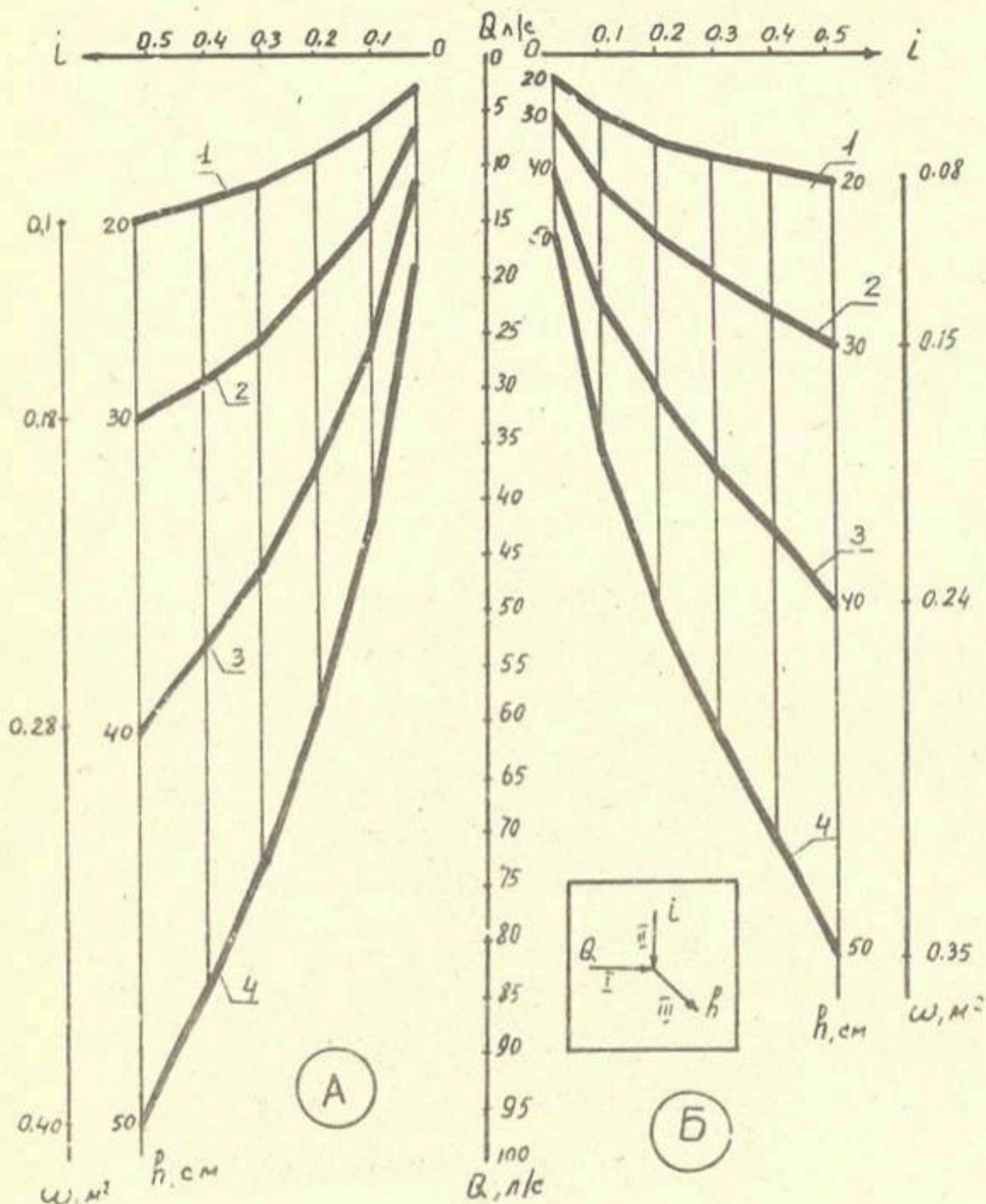
Рис. 3.15. Номограмма для гидравлического расчета водосборной канавки с гравийной засыпкой: А - при b = 20 \text{ см} ; Б - b = 0,30 \text{ м} ; 1 - при H_g = 20 \text{ см} ; 2 - H_g = 0,30 \text{ м} ; 4 - H_g = 50 \text{ см} .
