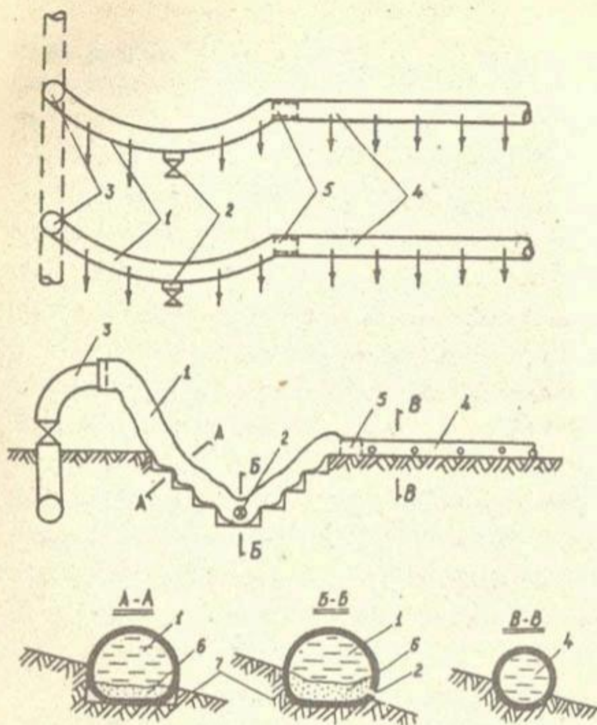
Рис. 3.4. Поливной шланг с осаждающей камерой: 1 — камера отстойника; 2 — промывник; 3 — гидрант; 4 — поливной шланг; 5 — соединительный патрубок; 6 — наносы; 7 — поверхность земли.
