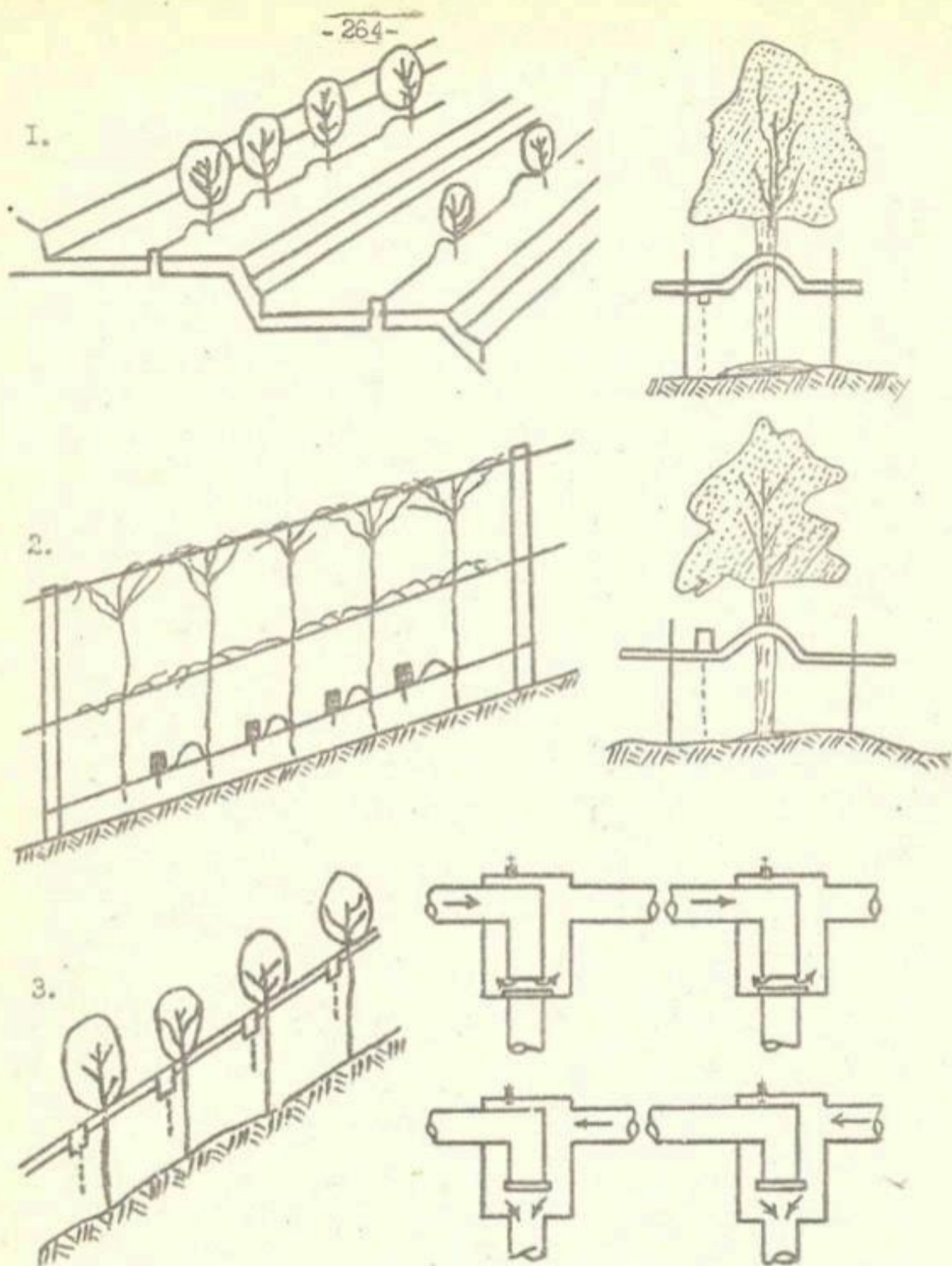
Рис. 4.2 Низконапорные капельные системы: 1 - Таджикистан-1 (непрерывная); 2 - Таджикистан-1м (импульсная); 3 - Таджикистан-2 (импульсная).
