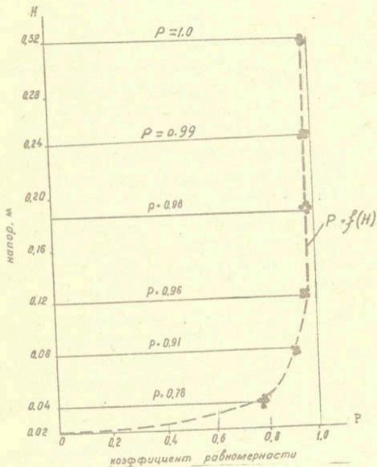
Рис. 4.13. Зависимость равномерности расхода капельницы с фиксированным отверстием от напора.
