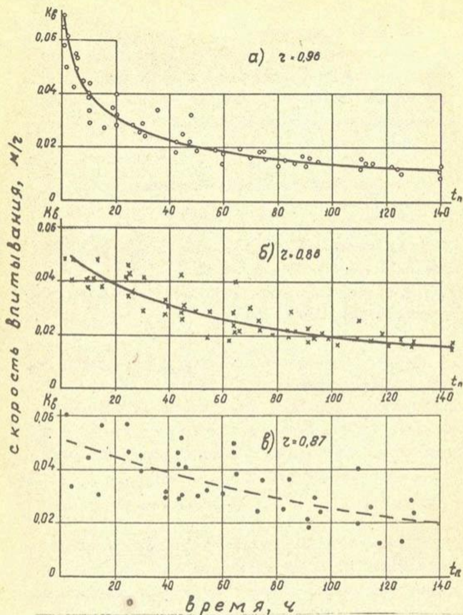
Рис. 2.10. Характер изменения скорости впитывания воды во времени на различных участках обычных борозд: а - начало; б - середина; в - конец, z - коэффициент корреляции.
