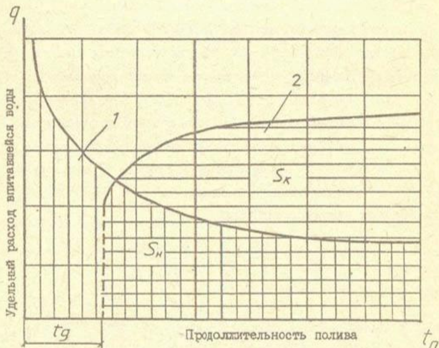
Рис. 2. Изменение удельного расхода впитавшейся воды по зигзагообразной микробороде с монотонно увеличивающимся коэффициентом извилистости: 1 - в начале поливной площадки; 2 - в конце поливной площадки; S_n и S_k - соответственно объем впитавшейся воды, в начале и конце склона.
