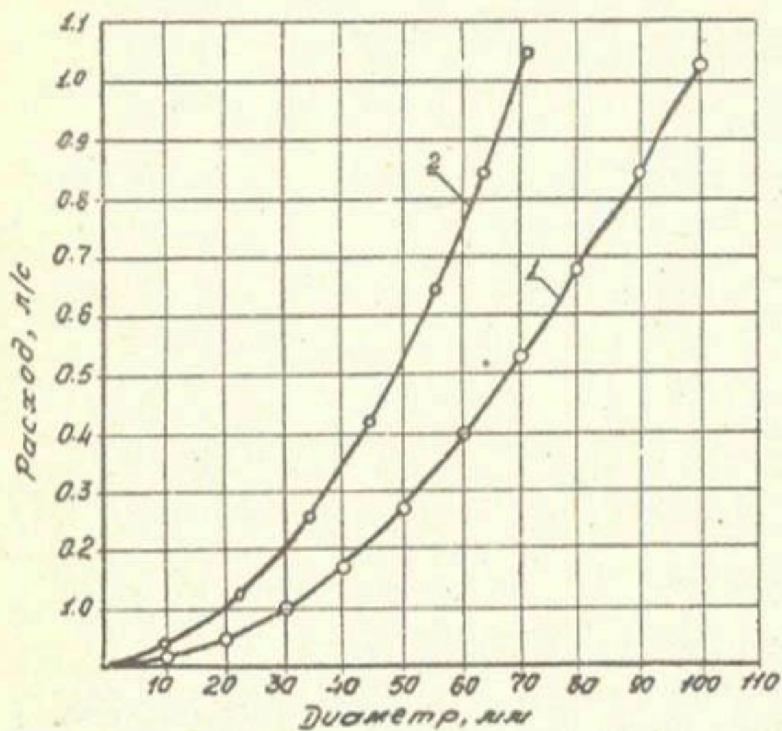
Рис. 4.9. Зависимость заправочных расходов воды от диаметра труб, при 1 \angle = 60^\circ ; 2 - \angle = 120^\circ .
