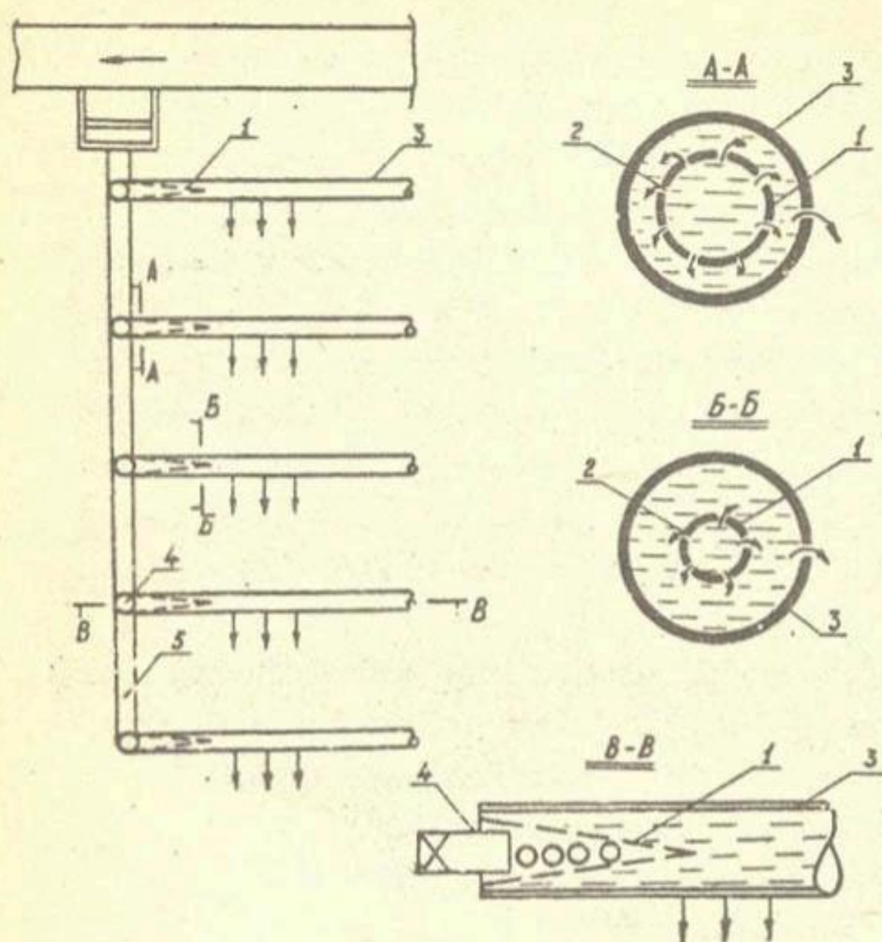
Рис. 3.3. Поливной шланг с сорособирающей сеткой: 1 - с"емная сорособирающая сетка; 2 - ячейка сетки; 3 - поливной шланг; 4 - гидрант; 5 - распределительный трубопровод.
