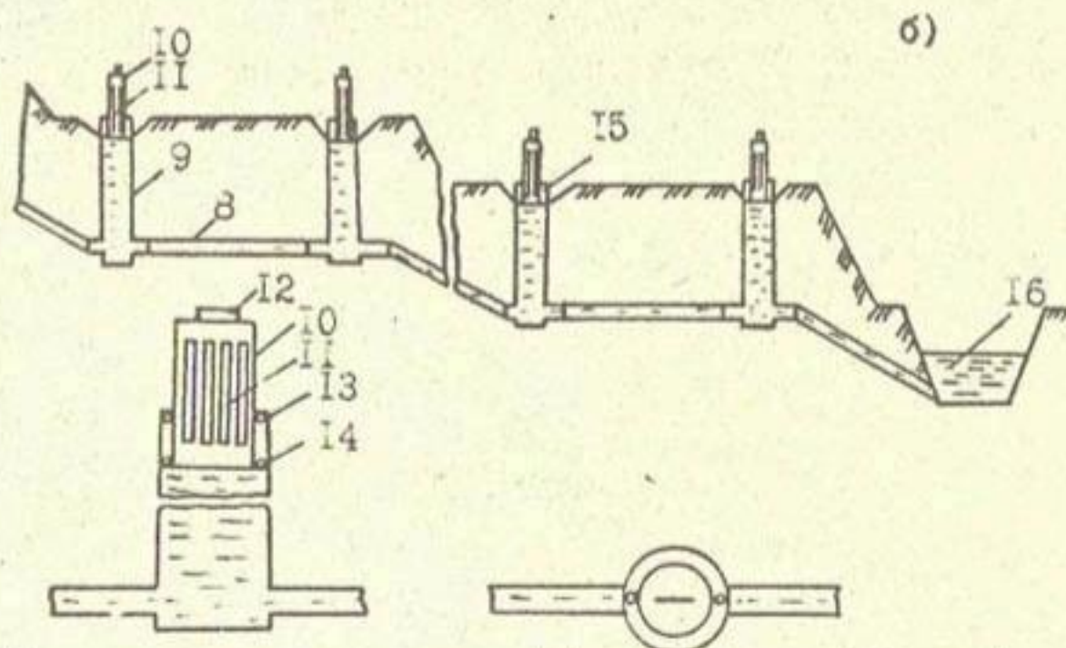
Рис. 3.27 Распределительно-поливная (а) и сбросная (б) трубчатая сеть для орошения садов и виноградников на террасированных склонах: 1 - основной трубопровод; 2 - водовыпускная трубка; 3 - регулятор; 4 - расширенная часть регулятора с упругим кольцом; 5 - отводной пат- рубок; 6 - поливная борозда; 7 - П-образный участок; 8 - сбросной тру- бопровод; 9 - стояк; 10 - водоприемный оголовок; 11 - щели; 12 - руч- ка; 13 - фиксатор; 14 - резиновое кольцо; 15 - полиэтиленовый экран; 16 - главный сбросной канал.
