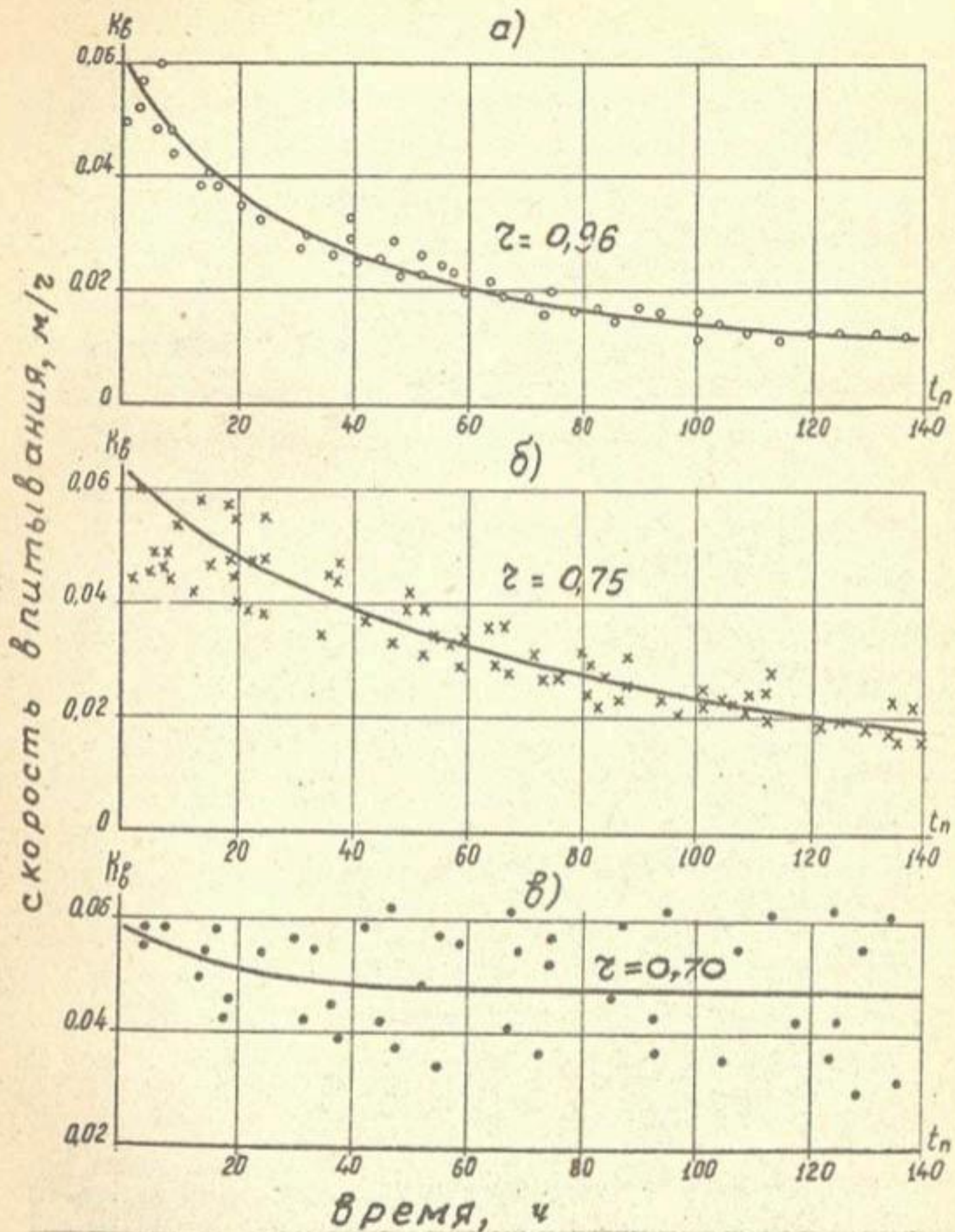
Рис. 2.II. Характер изменения скорости впитывания воды во времени на различных участках прямолинейной микророзды : а - начало; б - середина , в - конец, z - коэффициент корреляции.
