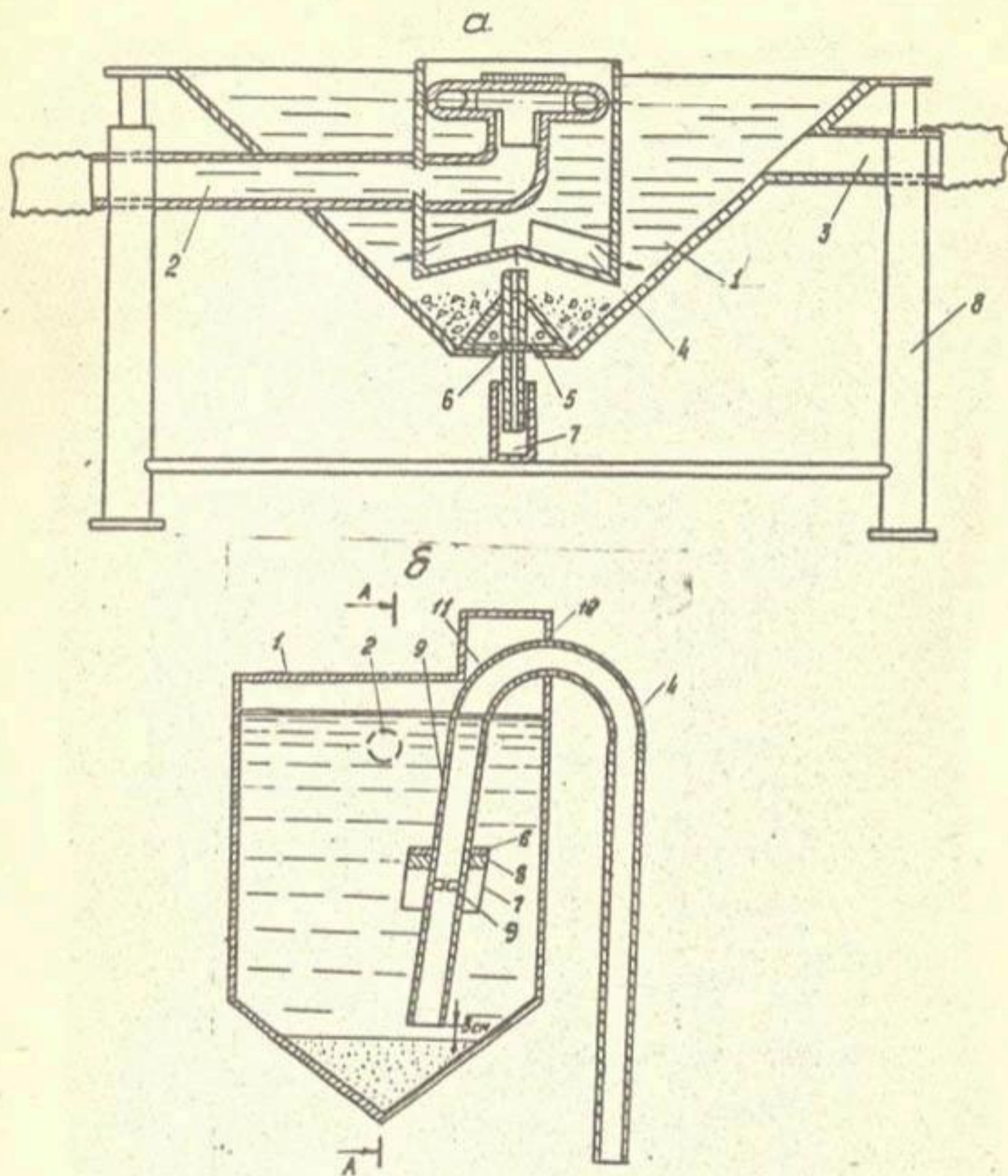
Рис. 4.4. Отстойники-автоматы:
