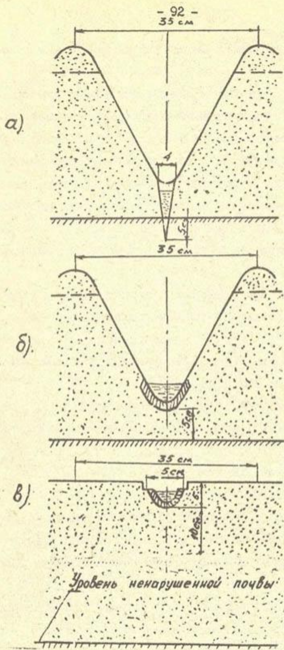
Рис. 2.3. Поперечное сечение поливных борозд: а - обычная, нарезанная окучником НКУ-27А; б - обычная с прикатанным дном; в - микроборозда, вдавленная катками.
