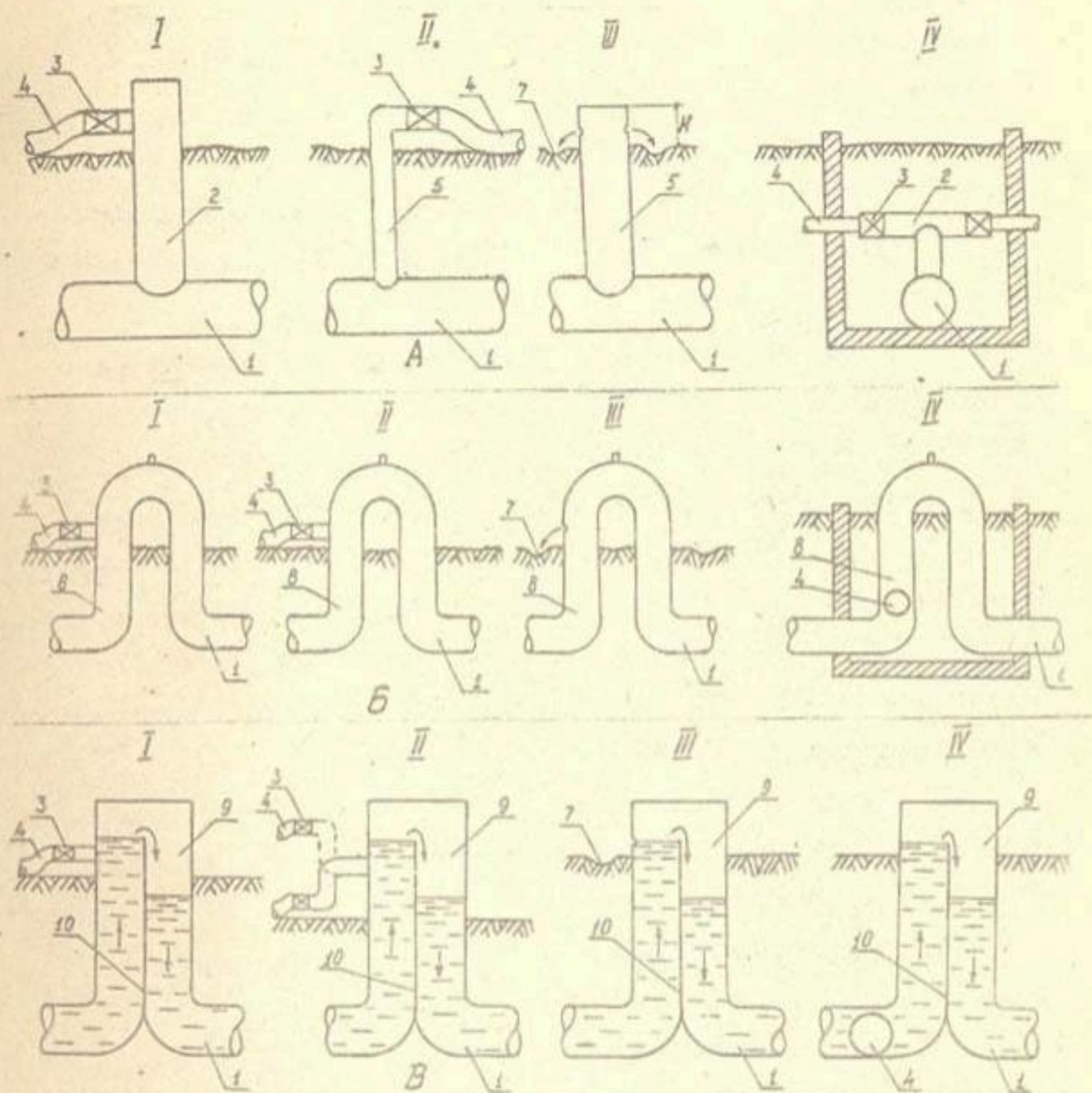
Рис. 3.18. Схема раздачи воды из трубчатой сети на различные элементы поливной сети: А - существующие; Б - предлагаемые с использованием П-образных участков; В - то же, с применением двухкамерных водовыпусков;
