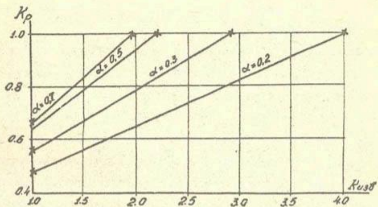
Рис. 2.15. Зависимость K_p = f(\alpha, K_{uzb}^F)
