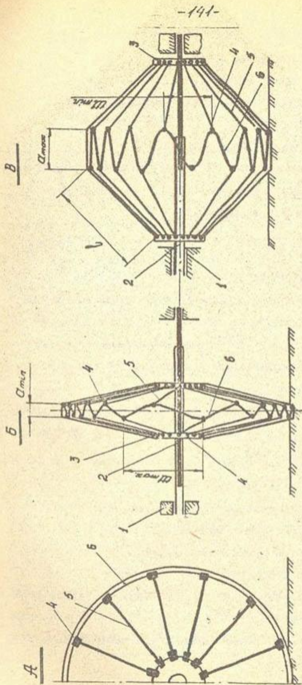
Рис. 2.20. Орудие для формирования микророзд: А - профиль; Б - рабочий орган растянут; В - рабочий орган сжат; 1 - рама; 2 - ось; 3 - ступицы; 4 - шарниры; 5 - рычаги; 6 - рабочий орган; А_{min} - минимальная ширина полосы нарезки; А_{max} - максимальная ширина полосы нарезки; Ш_{min} и Ш_{max} - соответственно минимальные и максимальные амплитуды.
