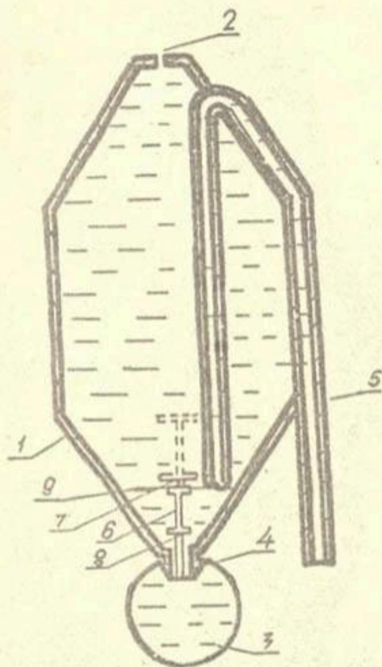
Рис. 4.II. Импульсная капельница "Таджикистан-Im":
