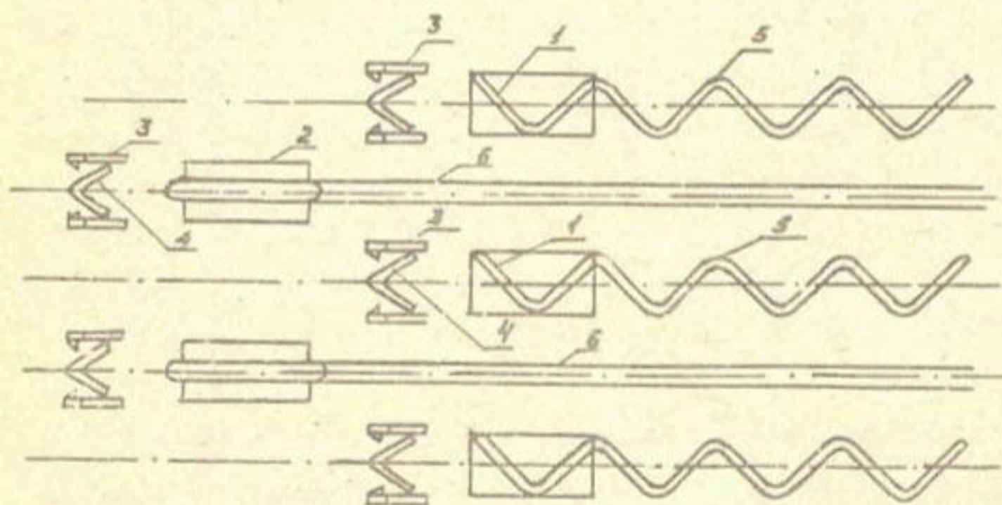
Рис. 2.19. Схема установки катков-бороздоделов КБ-1 на культиваторе Крх-4. 1 - катки с извилистыми выступами; 2 - то же с прямолинейными выступами; 3 - комплект культивирующих органов; 4 - стрелчатые лапки; 5 - извилистые микроборозды на междурядьях, где проходят колеса трактора; 6 - прямолинейные микроборозды, где не проходят колеса трактора.
