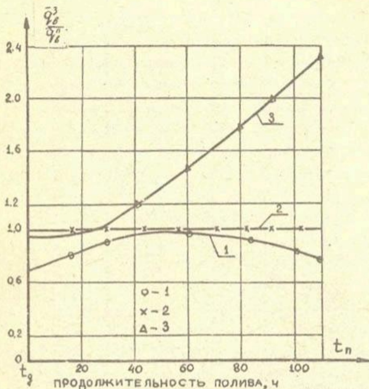
Рис. 2.24. Изменение соотношения расхода воды, впитавшейся на конечном участке склона при различной технологии нарезки: 1 - обычной борозды к прямолинейной микроборозде; 2 - прямолинейная микроборозда; 3 - зигзагообразной микроборозды с K_{\text{изв}} = 2.25 к прямолинейной.
