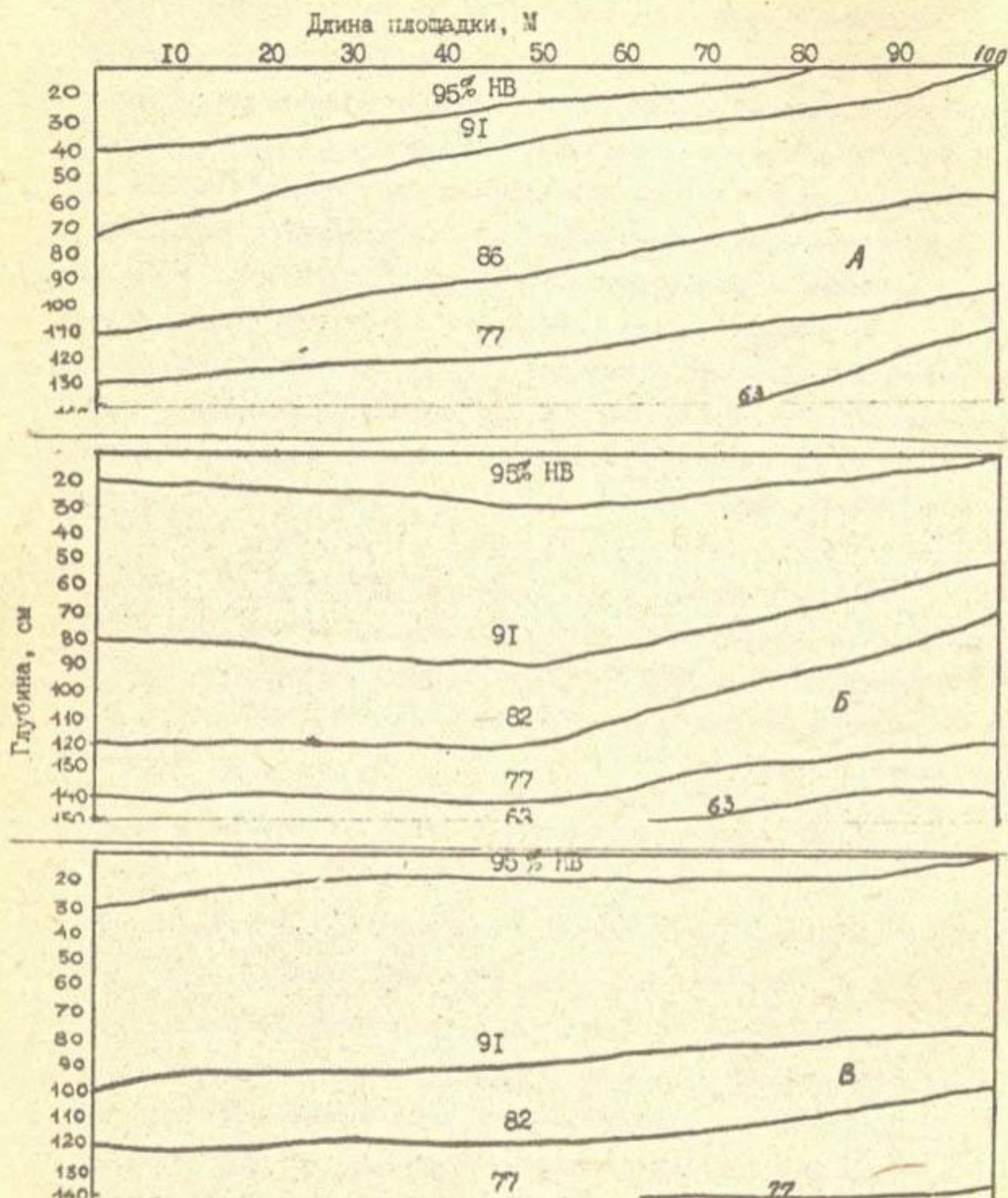
Рис. 2.13. Контуры увлажнения по длине 100-метрового склона при разной технологии полива (А - по обычным бороздам; Б- по прямолинейным микробороздам; В - по зигзагообразным микробороздам).
