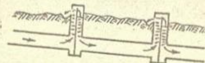
Рис.3.9. Рекомендуемые типы водовыпусков из трубчатой сети
