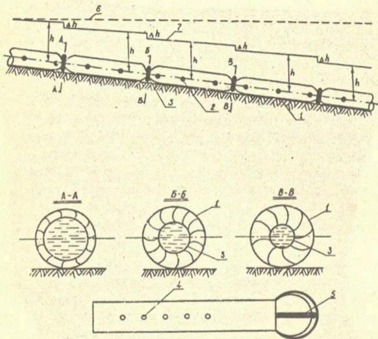
Рис. 3.6. Поливной шланг с напорорегулирующими кольцами: 1 - поливной шланг, 2 - поливные отверстия; 3 - напорорегулирующие кольца; 4 - отверстия; 5 - выступ для регулировки размера кольца; 6 - статический горизонт; 7 - пьезометрическая линия напора; h - напор; \Delta h - потери напора.
