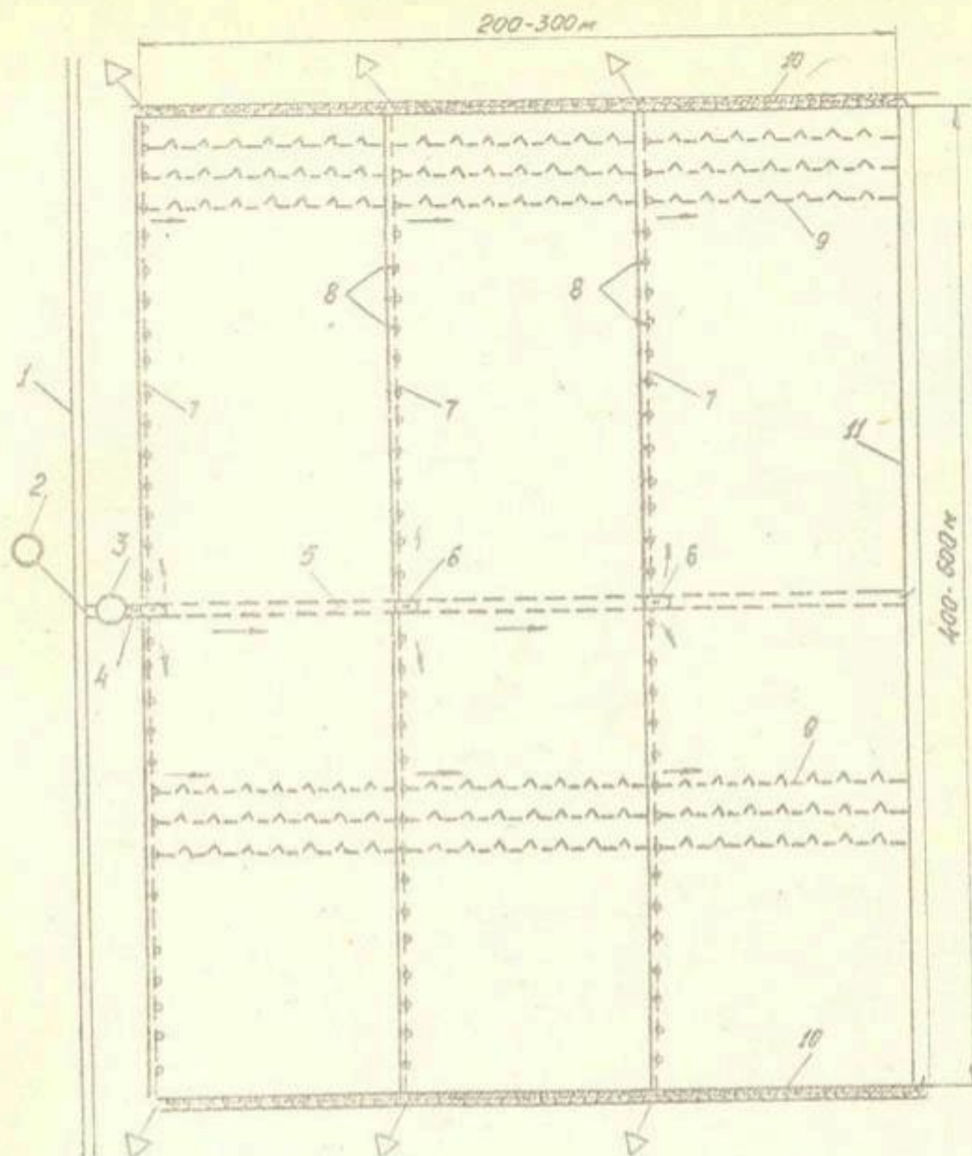
Рис. 4.2. Схема низконапорной капельной системы Таджикистан - I:
