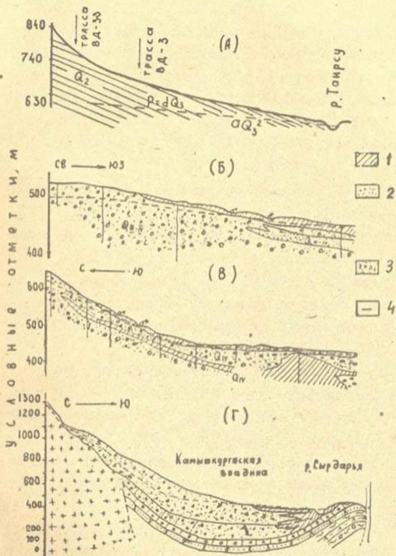
Рис. I.4. Схематические гидрогеологические разрезы: А - Данга-ринский массив; Б - Пянджский конус выноса; В - долина р. Яхсу; Г - Большой Алтский массив: 1 - суглинок; 2 - песок; 3 - мелкий галечник; 4 - уровень грунтовых вод.
