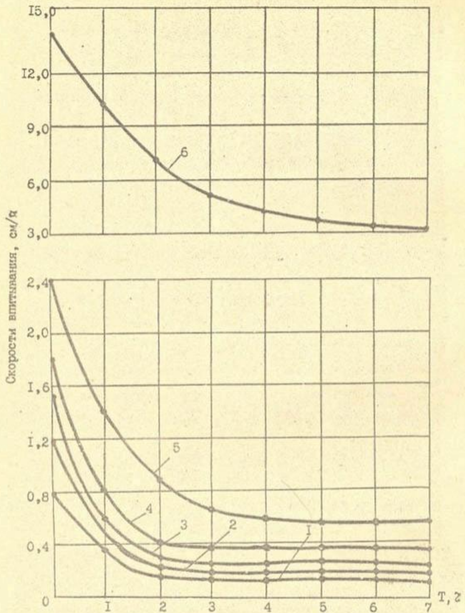
Рис. 1.3 Скорости впитывания воды на различных типах почв Таджикской ССР. 1 - коричневые карбонатные; 2 - обыкновенные сероземы; 3 - светлые сероземы; 4 - темные сероземы; 5 - типичные сероземы; 6 - серобурные каменистые.
