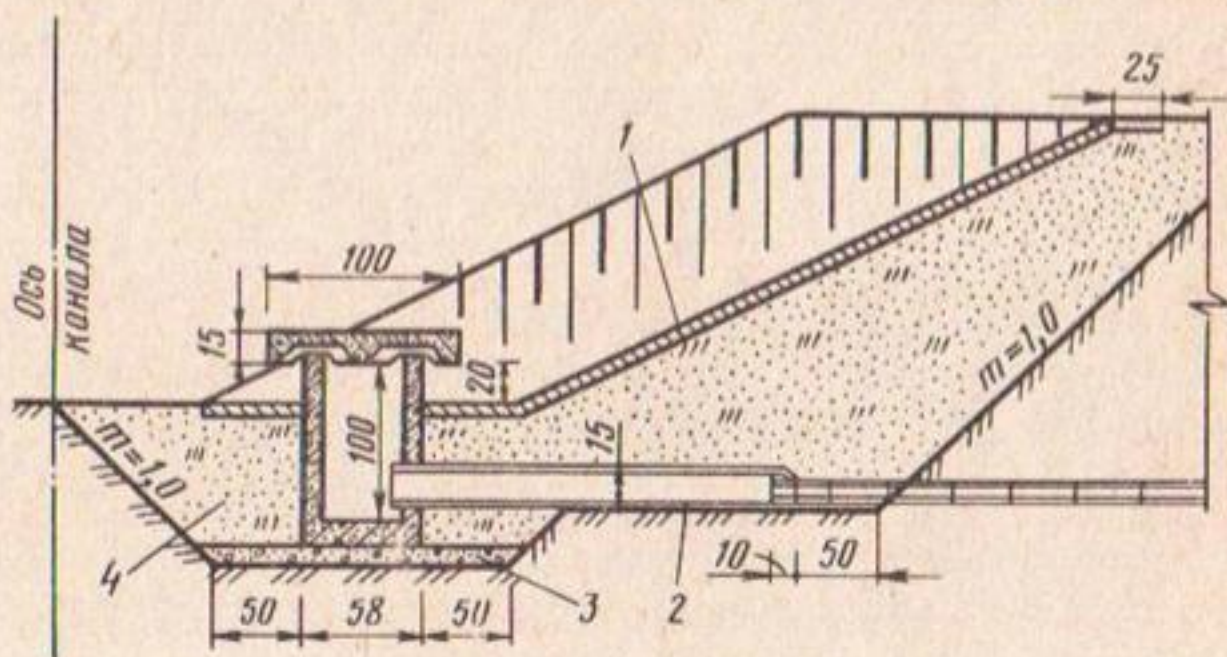
Рис. 14. Дренажный фильтр типа КППК-50-100 для отвода воды из открытого собирателя в закрытый:
