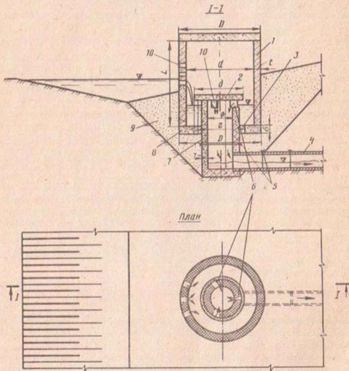
Рис. 8. Дренажный фильтр конструкции VIII:
