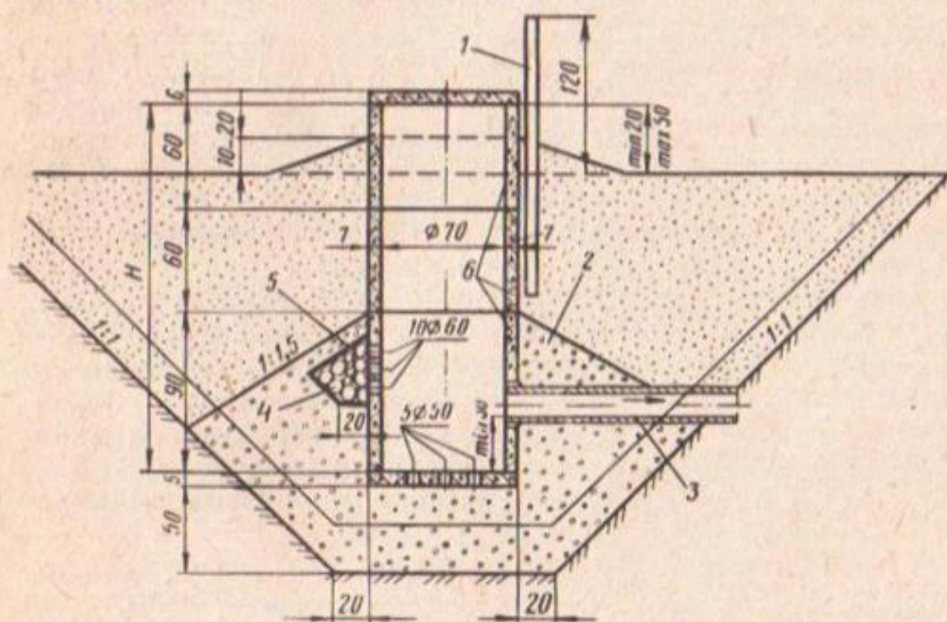
Рис. 19. Дренажный фильтр типа КОФ-III:
