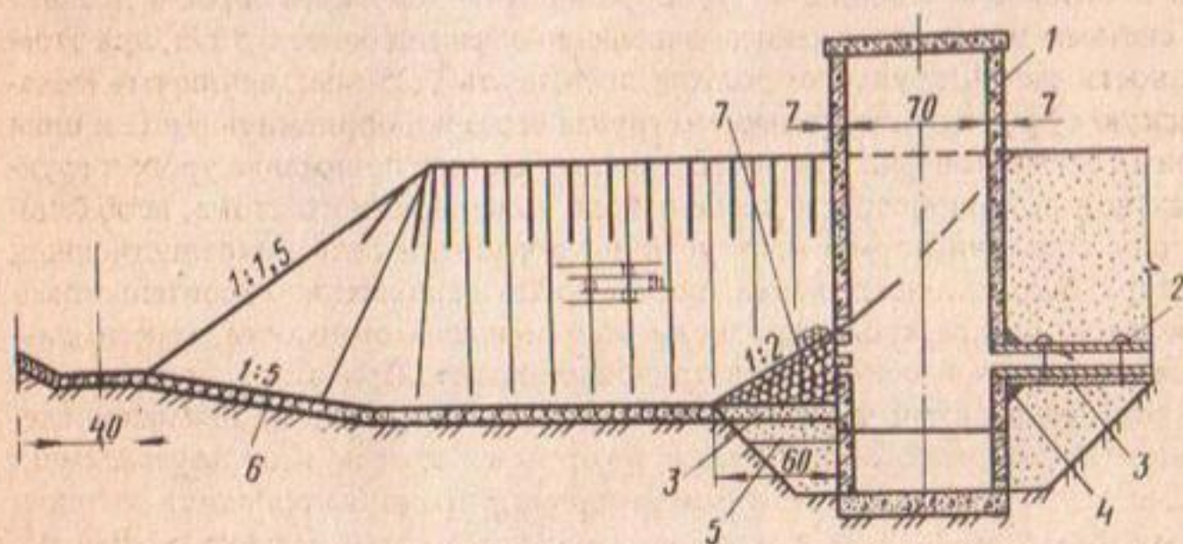
Рис. 1. Дренажный фильтр конструкции 1:
