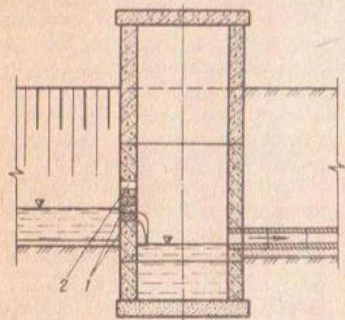
Рис. 4. Дренажный фильтр конструкции IV:
