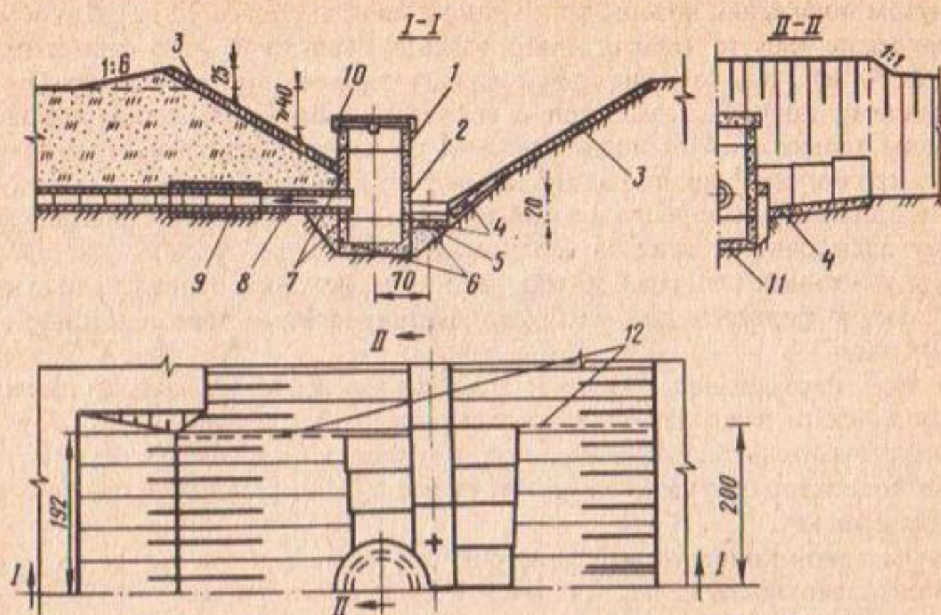
Рис. 11. Фильтр типа КК-1 для ввода воды из открытого собирателя в дренажный коллектор:
