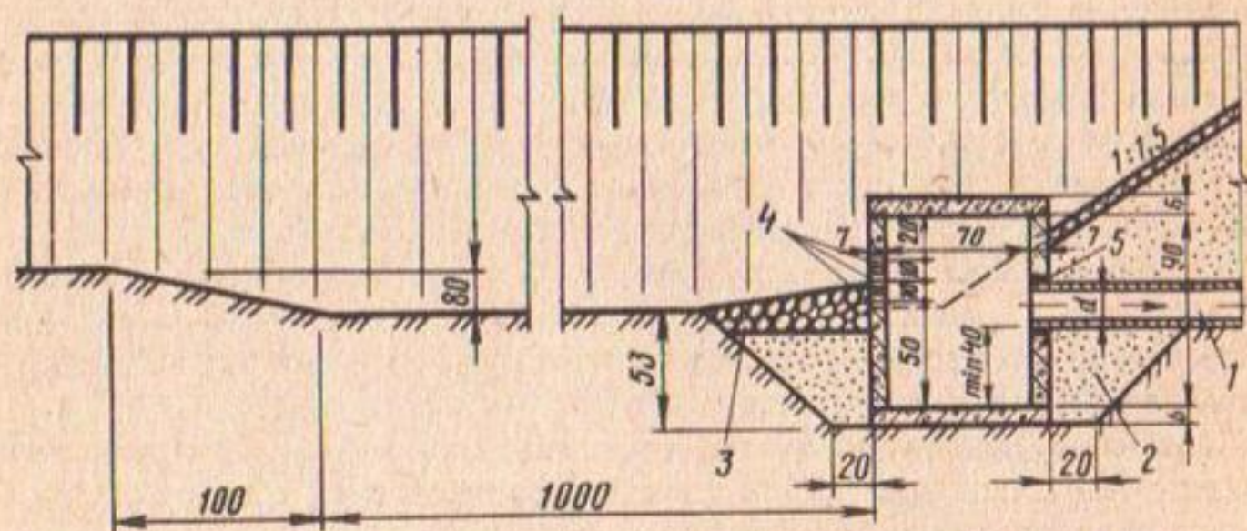
Рис. 12. Дренажный фильтр КОФ-1:
