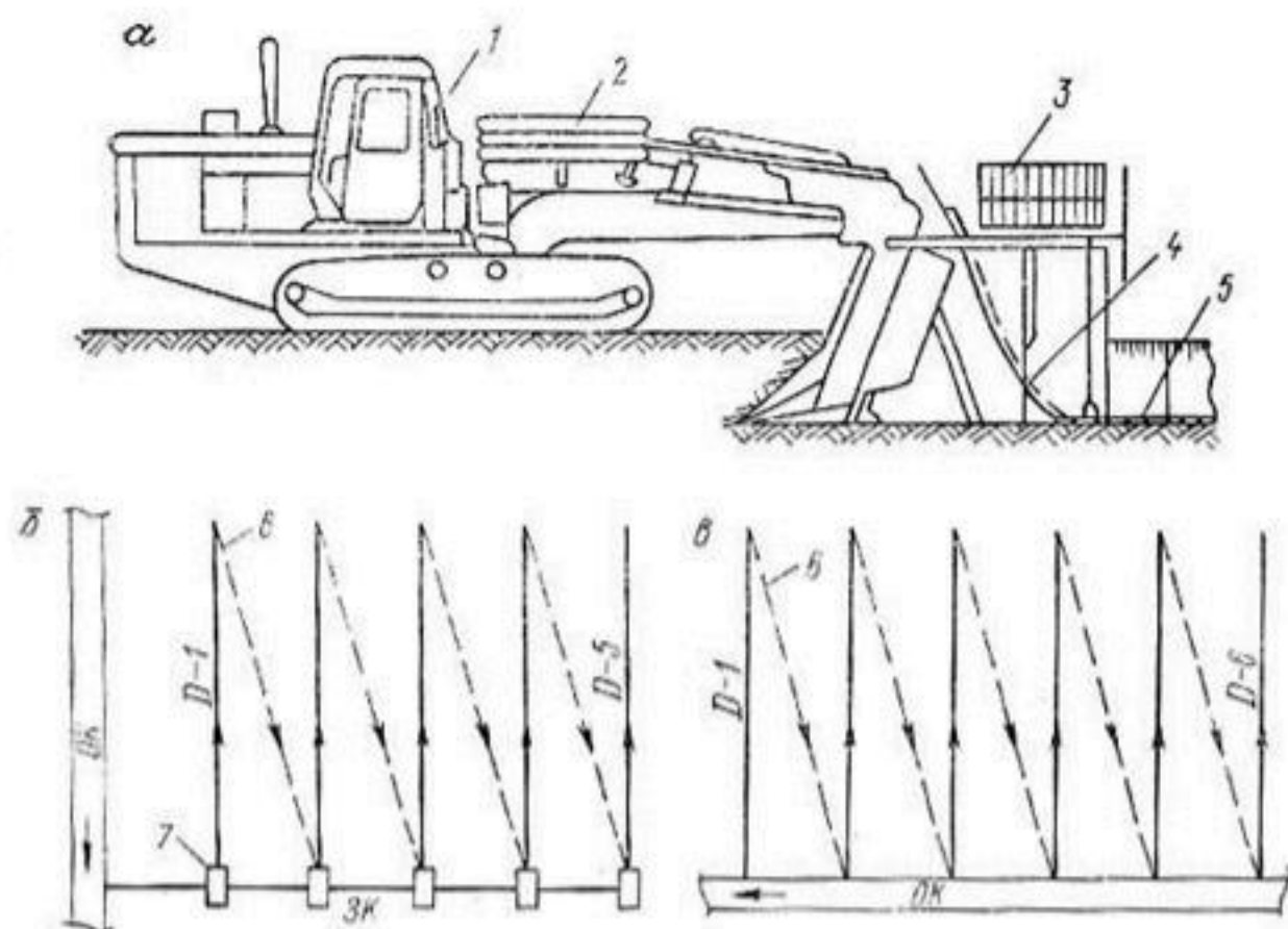
Рис. 26. Общий вид бестраншейного дрепоукладчика МД-4 (а) и технологические схемы прокладки дренажных трубопроводов при впадении дрен в закрытый коллектор (б) и при впадении дрен в открытый осушительный канал (а):
