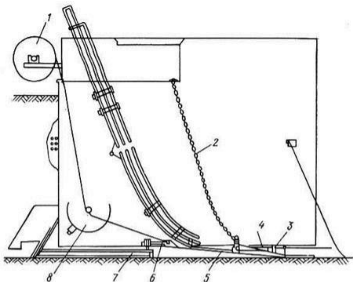
Рис. 18. Устройство к трубоукладчику ЭТЦ-202А для обертывания дренажных труб рулонным ЗФМ (ВНИИводполимер):
