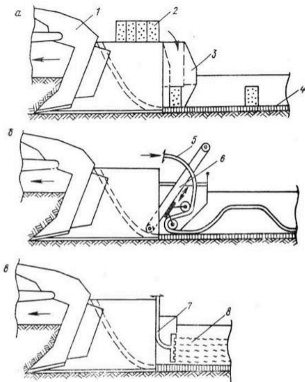
Рис. 29. Схема навесного технологического оборудования для укладки фильтрующих элементов:
