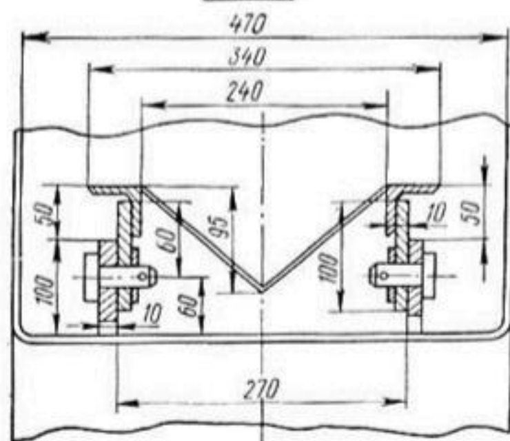
Вид А-А
