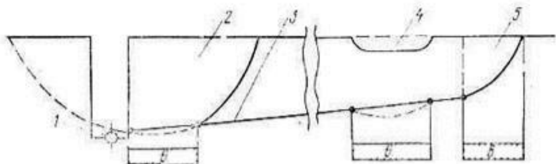
Рис. 27. Местонахождение зон наиболее вероятных отклонений продольных уклонов бестраншейных дренажей:
