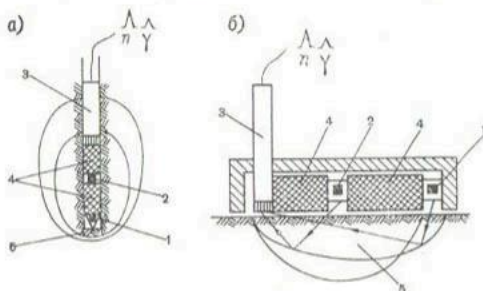
Рис. 40. Совмещенные зонды гамма-нейтронного влагомера-плотнмера.
