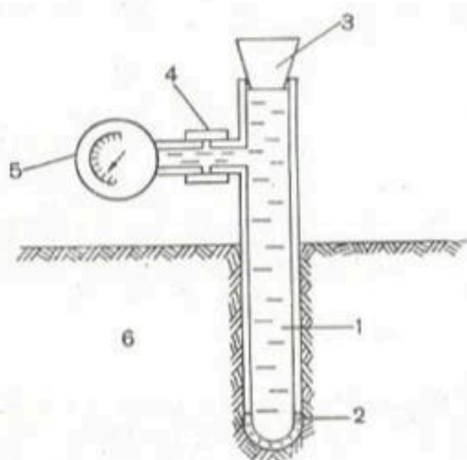
Рис. 17. Схема устройства тензиометра.
