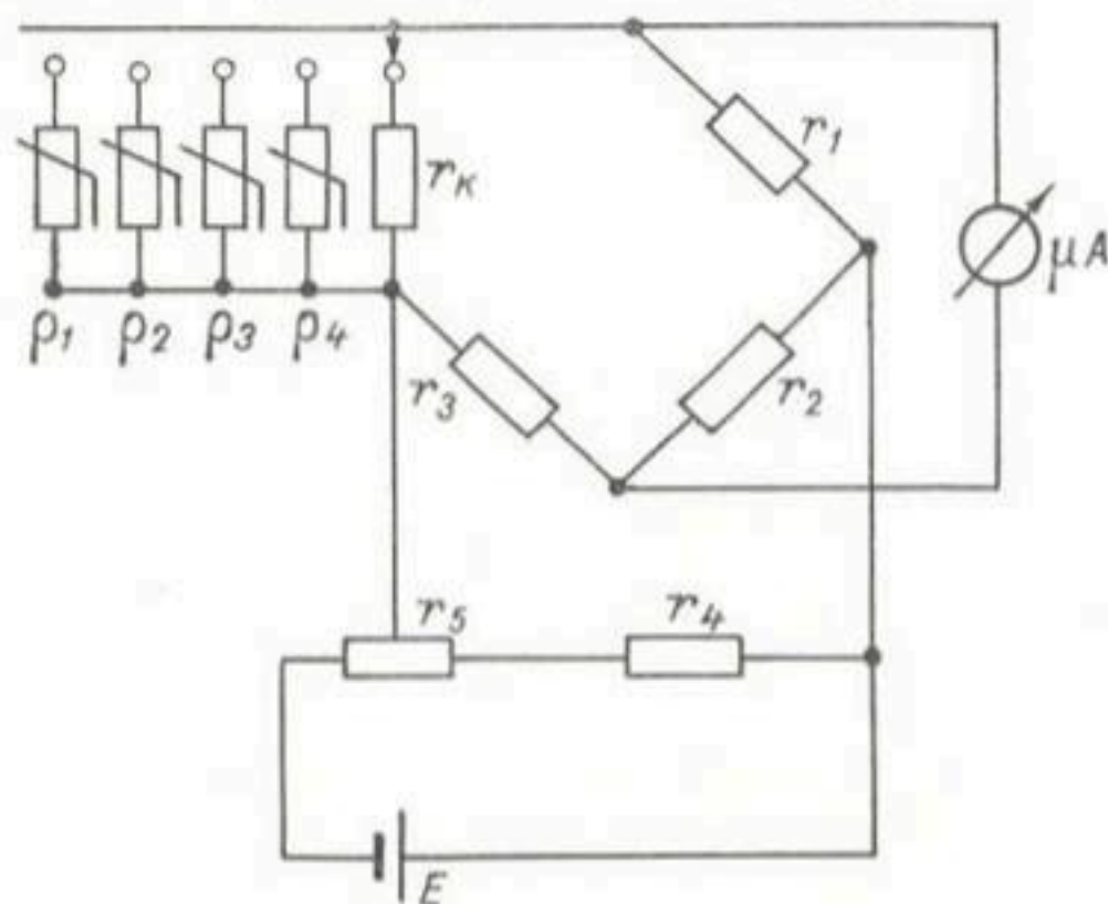
Рис. 4. Схема микроэлектротермометра.
