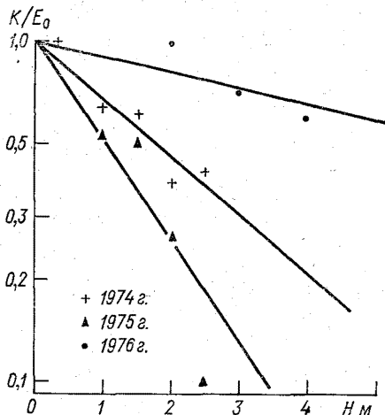
Рис. 2.6. Ход отношения подпитки активного слоя почвы K к оптимальному водопотреблению E_0 для орошаемого поля капусты в совхозе «Петровский» Челябинской области.
