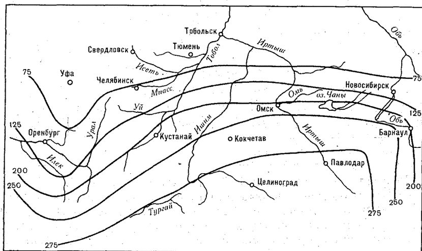
Рис. 4.5. Схематическая карта среднееголетних значений недостатка водопотребления M за период вегетации яровой пшеницы (мм).
