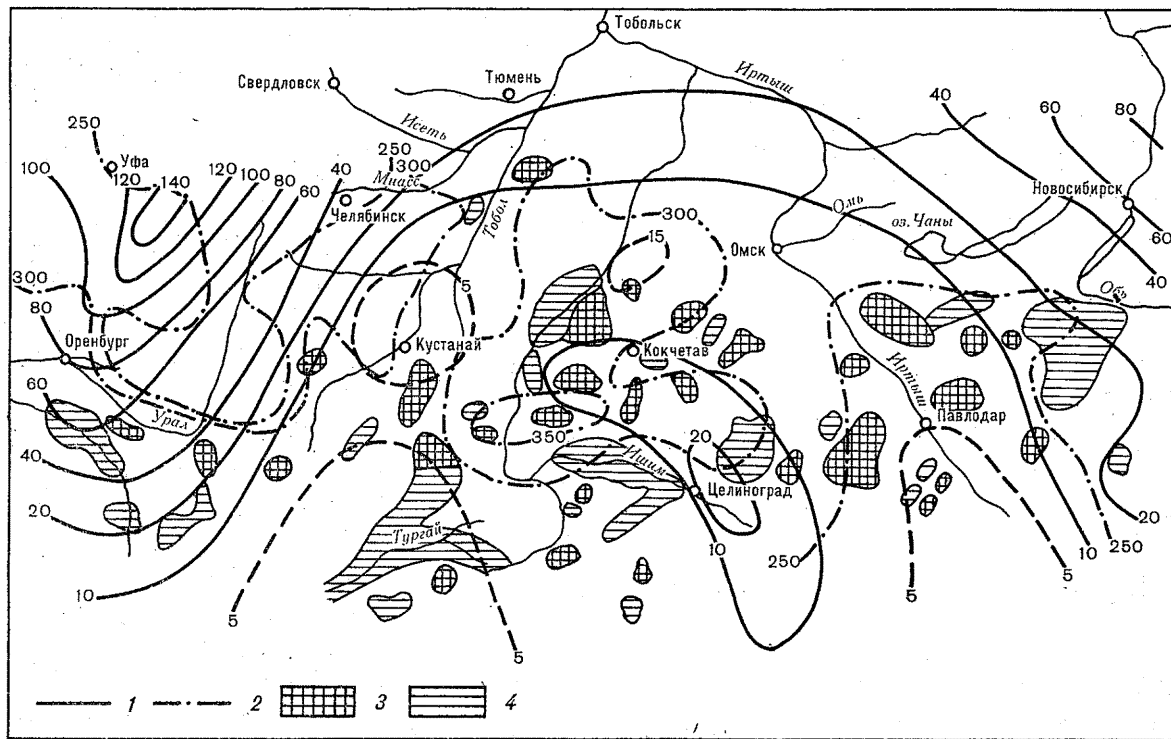
Рис. 3.10. Схематическая карта мелиоративного районирования для лиманного орошения в степной и лесостепной зонах Среднего региона СССР (составлена Н. А. Мосенко и Н. Н. Логиновой).
