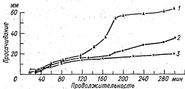
Рис. 3.4. Интегральные кривые впитывания воды в мерзлую почву. 1 — целина (1954 г.), 2 — зять (1954 г.), 3 — целина (1955 г.).
