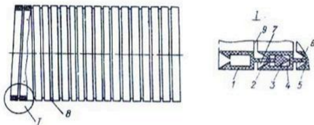
Рис. 6. Дренажная труба: 1 - виток пластмассовой ленты; 2 - отверстие; 3 - язычок; 4 - прорез; 5 - скосы; 6, 7 - кольцевые полости; 8 - кольцевая щель; 9 - внутренняя полость дренажной трубы.
