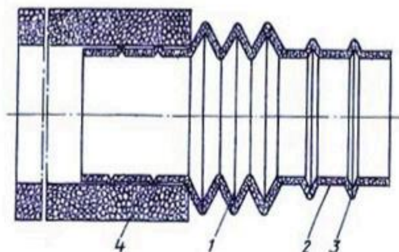
Рис. 19. Эластичное соединительное звено.
