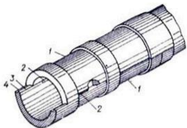
Рис. 27. Гончарная дренажная труба по патенту США № 3563039.
