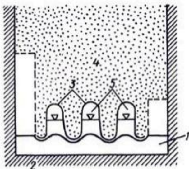
Рис. 4I. Устройство для дренирования связных грунтов: 1 - разбитый фильтрующий элемент; 2 - грунт не нарушенной структуры; 3 - профилированное покрытие-свод; 4 - обратная засыпка; 5 - полость дренажного устройства для транспорта воды.
