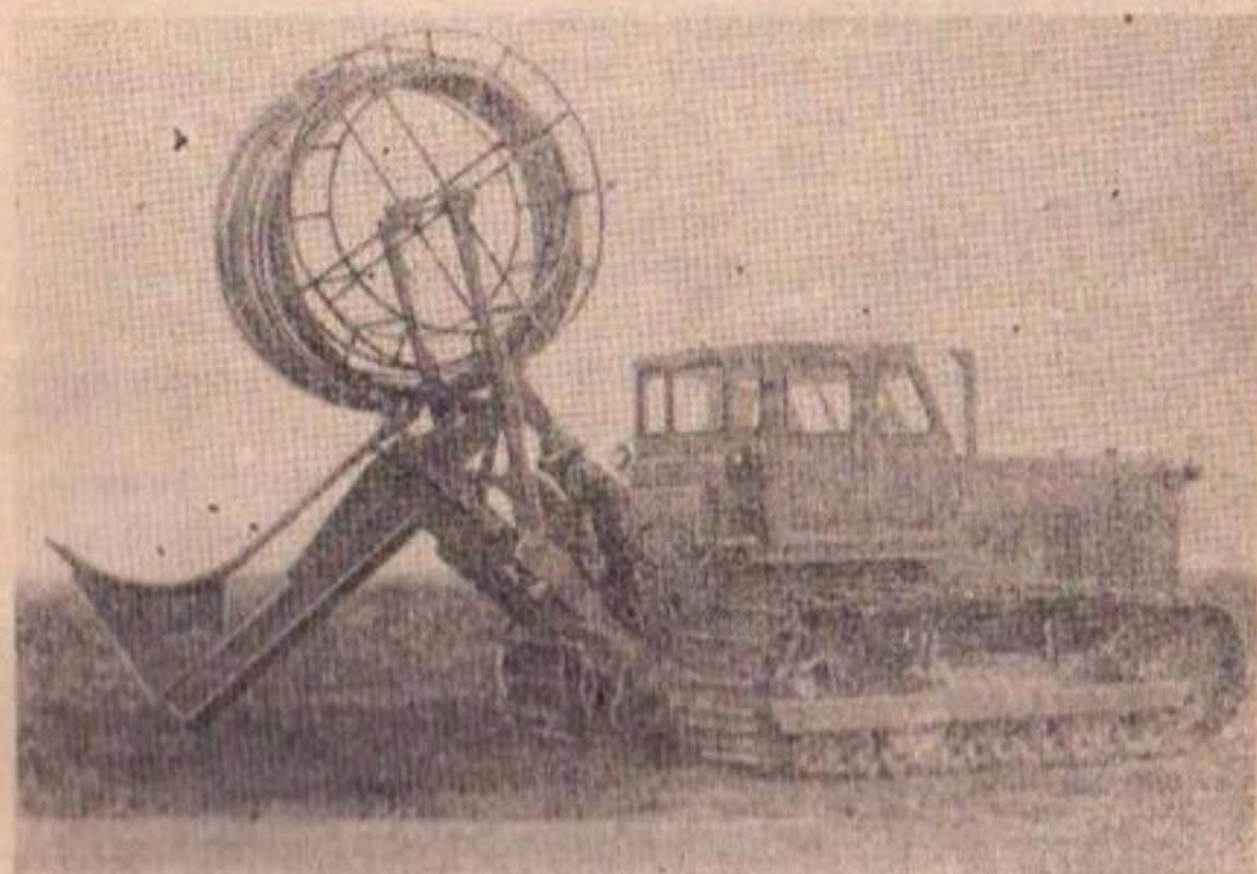
Рис. 22 Дреноукладчик ДПБН-1,8 для укладки готовых пластмассовых труб
