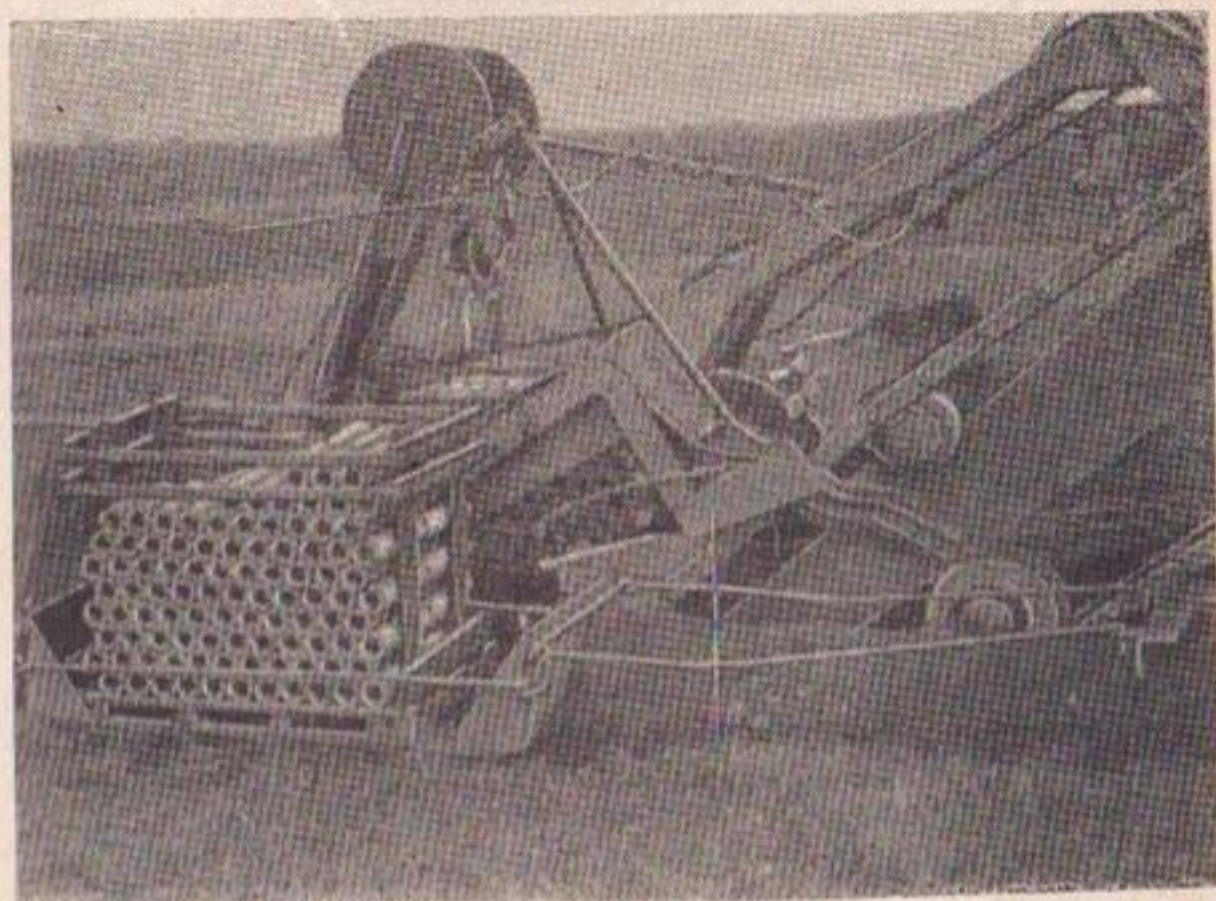
Р и с. 26. Транспортировка керамических труб за дрепоукладчиком
