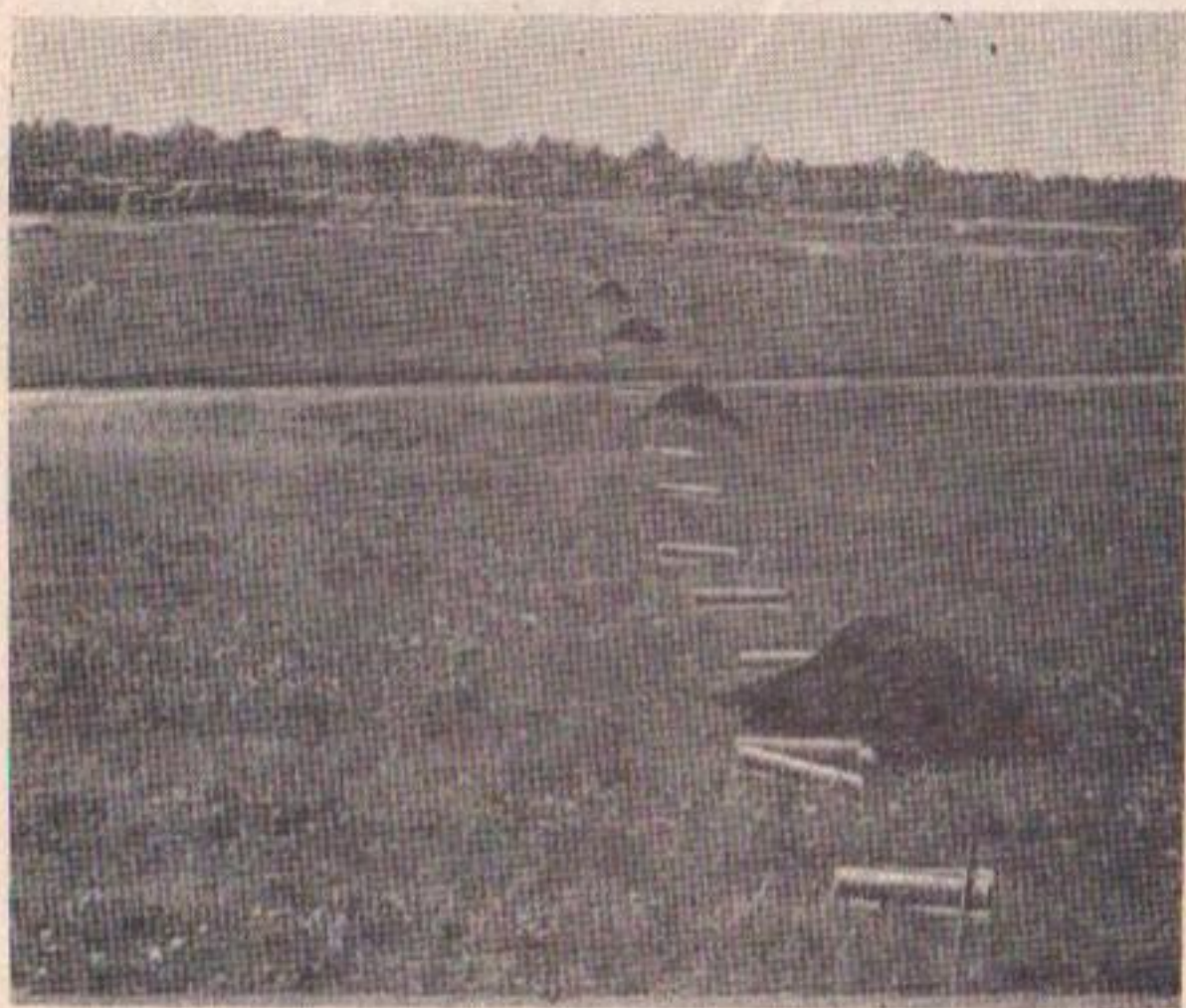
Р и с. 25. Раскладка керамических труб вдоль трассы кучками
