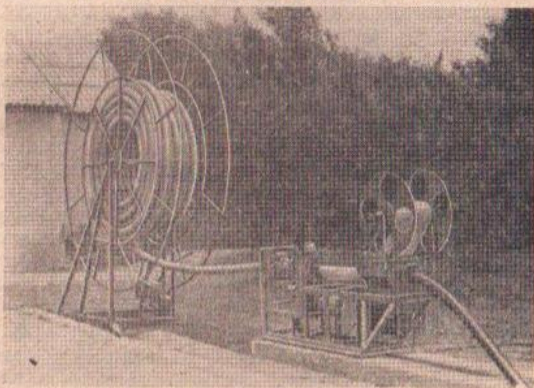
Рис. 11. Обмоточное устройство
