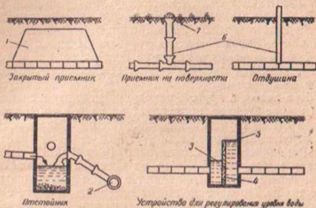
Рис. 10. Специальные устройства на дренажной сети: 1 — пористая засыпка; 2 — выпускная дрена; 3 — нижний уровень воды; 4 — перегородка; 5 — верхний уровень воды; 6 — металлическая труба или дрена со втулочным соединением (конец одной трубы входит в раструб на конце другой трубы); 7 — защитная решетка
