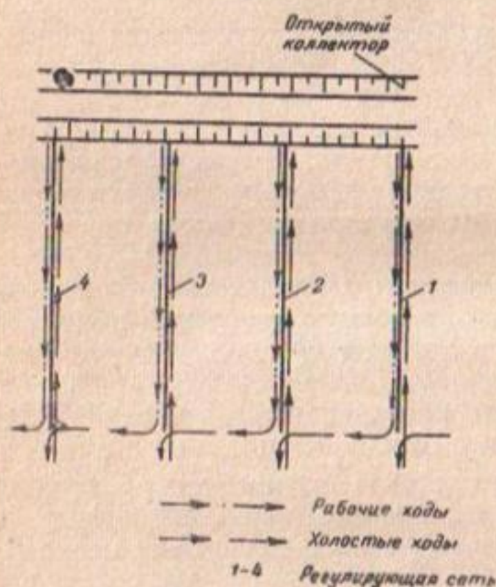
Р и с. 28. Схема движения дренажной машины БДМ-300
