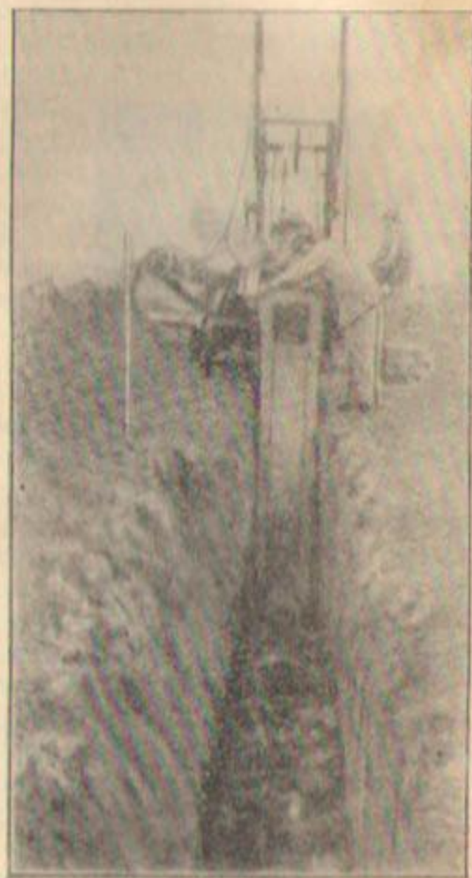
Рис. 148. Канавокопатель на тракторной тяге, прокладывающий траншею глубиной 1,8 м в песчаной почве.
