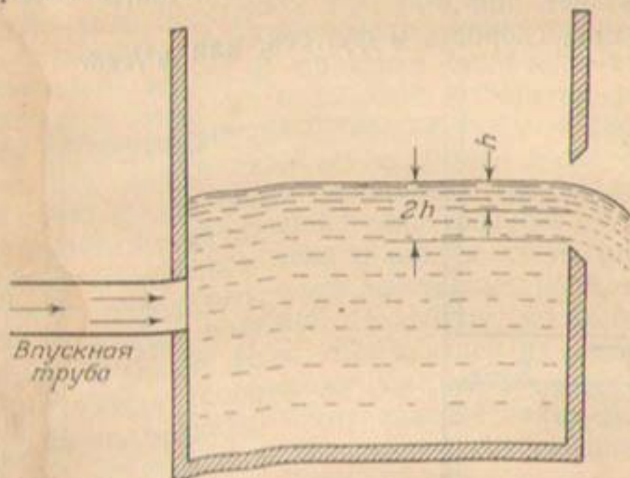
Рис. 12. Истечение воды через частично заполненное отверстие аналогично истечению через водослив.
