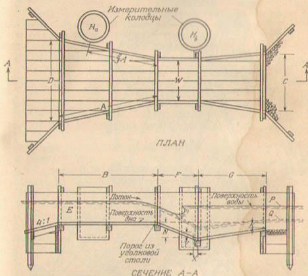
Рис. 22. План и продольный разрез водомера Паршалла. Размеры даны в табл. 3.
