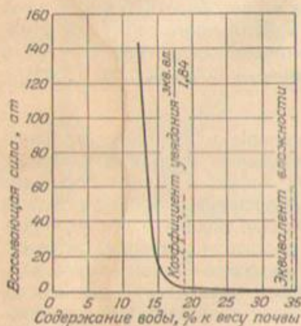
Рис. 153. Кривая всасывающей силы, удерживающей воду в илесто-глинистом суглинке при разных величинах влажности.
