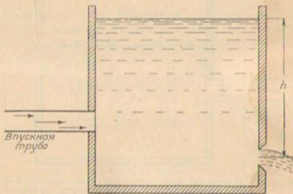
Рис. 11. Истечение воды через отверстие под напором.
