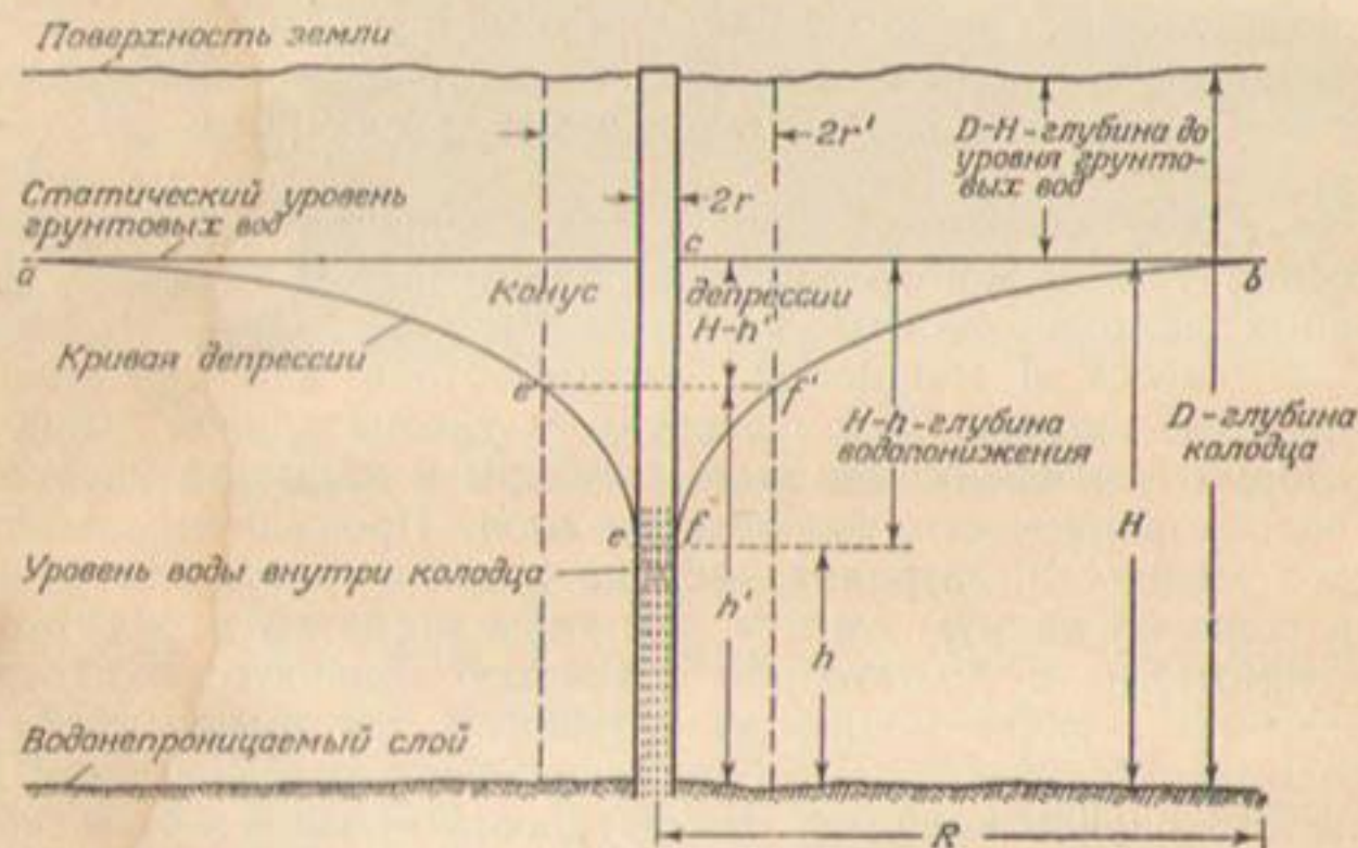
Р и с. 62. Вертикальный разрез типового оросительного колодца в безнапорных грунтовых водах (масштаб не соблюден).
