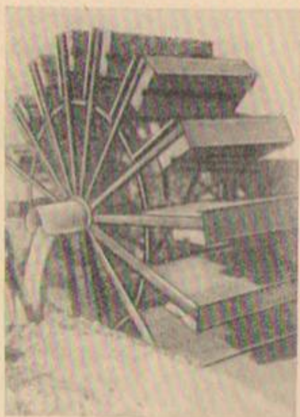
Р и с. 49. Стальное водоналивное колесо диаметром 6,6 м поднимает воду (42 л/сек) в канаву, расположенную на 3,4 м выше.
