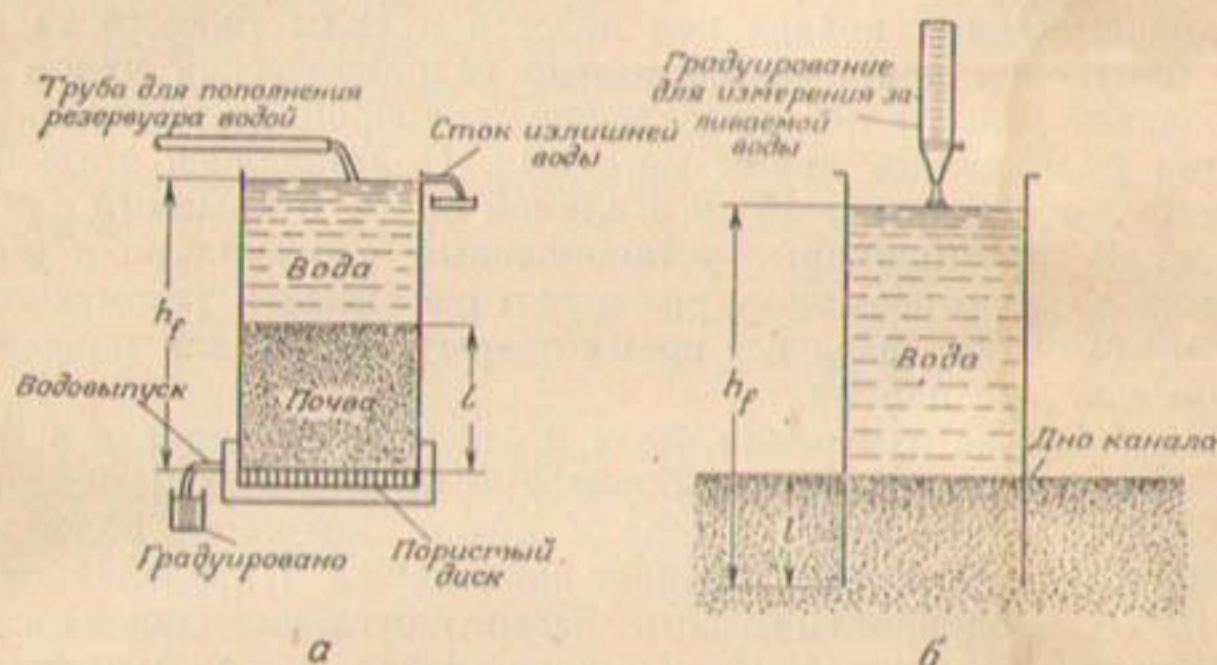
Рис. 132. Пермеаметры постоянного напора.
