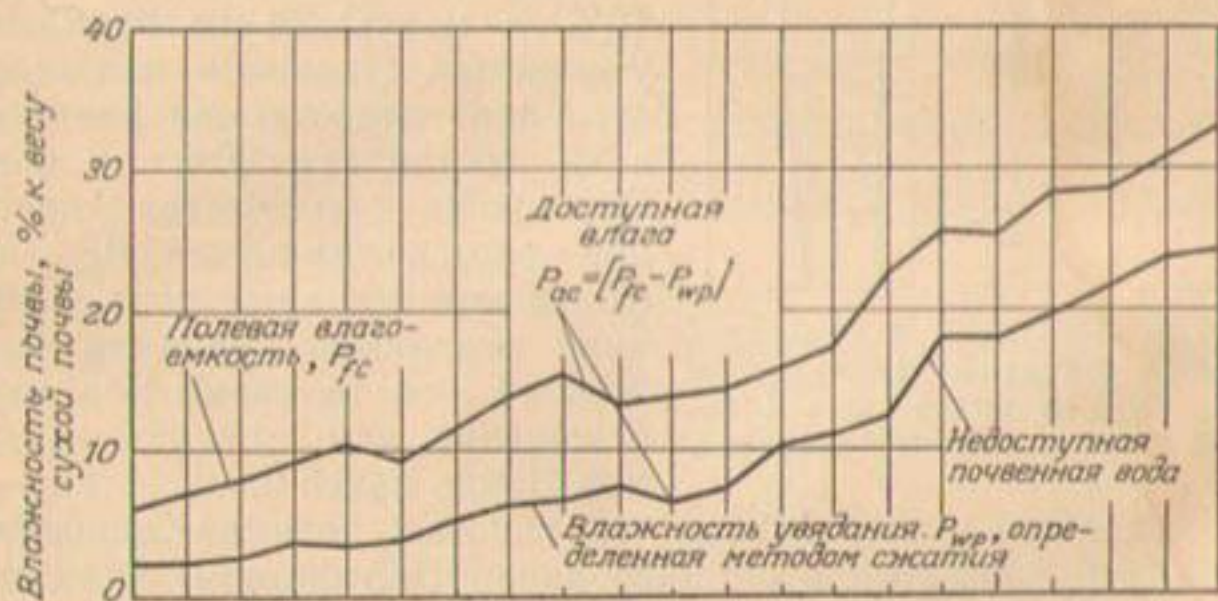
Рис. 122. Полевая влагоемкость, влажность увядания и доступная влага почвы в 21 пункте штата Южная Каролина.
