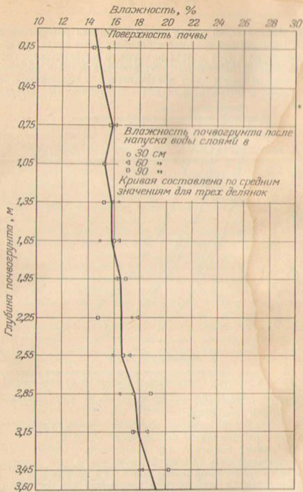
Р и с. 108. График распределения влажности в почвогрунте через 68 дней после полива с поправками на разнообразие механического состава почвогрунта, что дает представление о распределении, которое могло бы быть в почве с однородным механическим составом.
