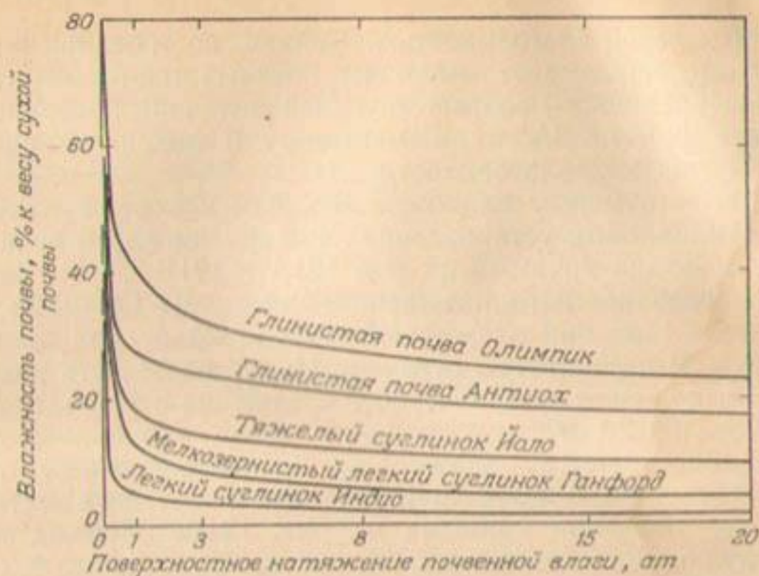
Рис. 121А. Поверхностное натяжение почвенной влаги в пределах 20 ат при различных величинах влажности для 5 видов почв Калифорнии.
