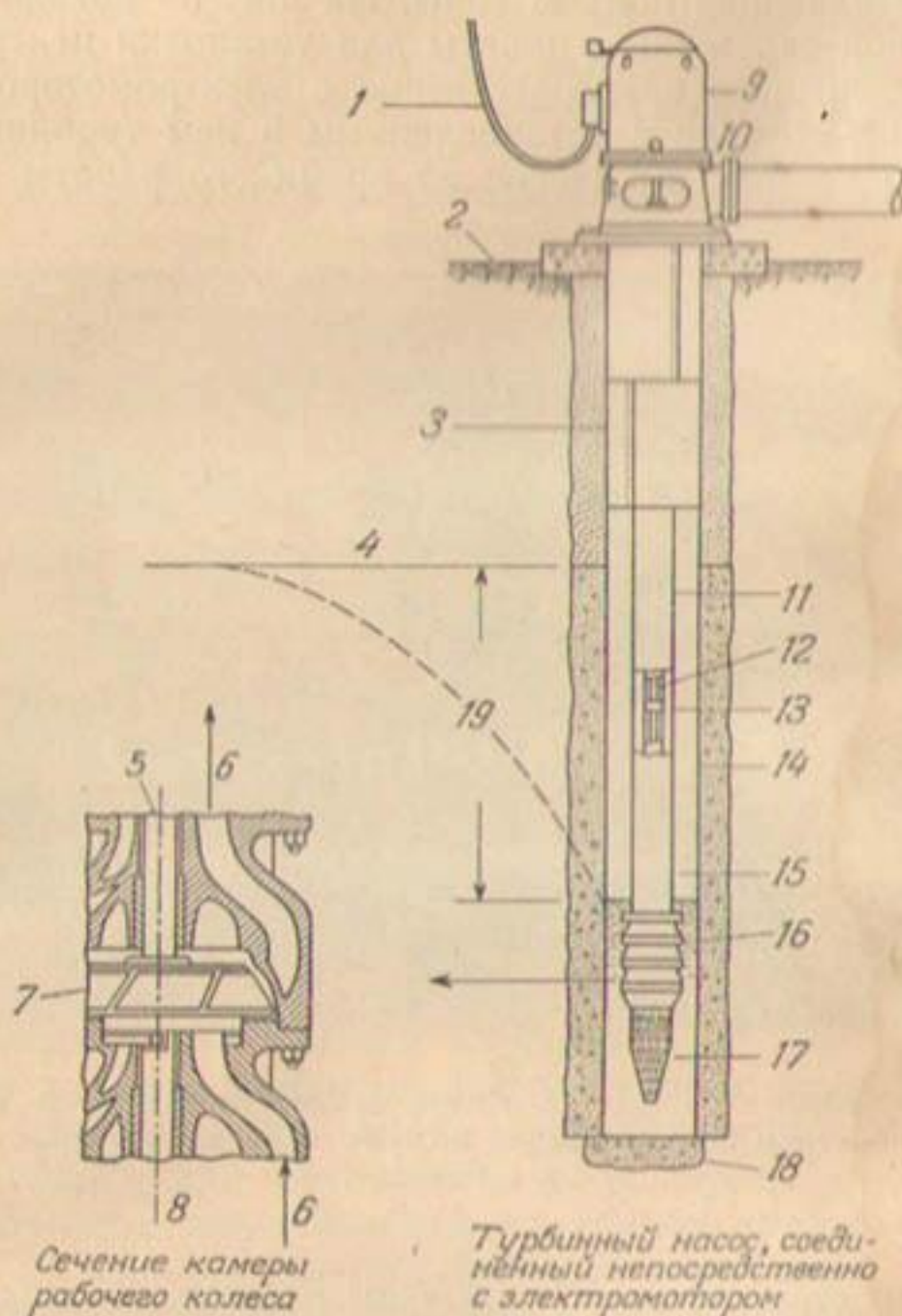
Р и с. 60. Схема установки турбинного насоса в глубоком колодце.
