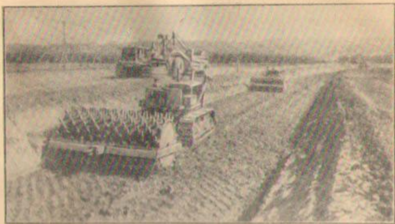
Р и с. 90. Тяжелый кулачковый каток. Применяется для уплотнения грунта в каналах, что увеличивает противифльтрационные свойства грунта, уменьшает опасность размыва и задерживает произрастание сорняков.
