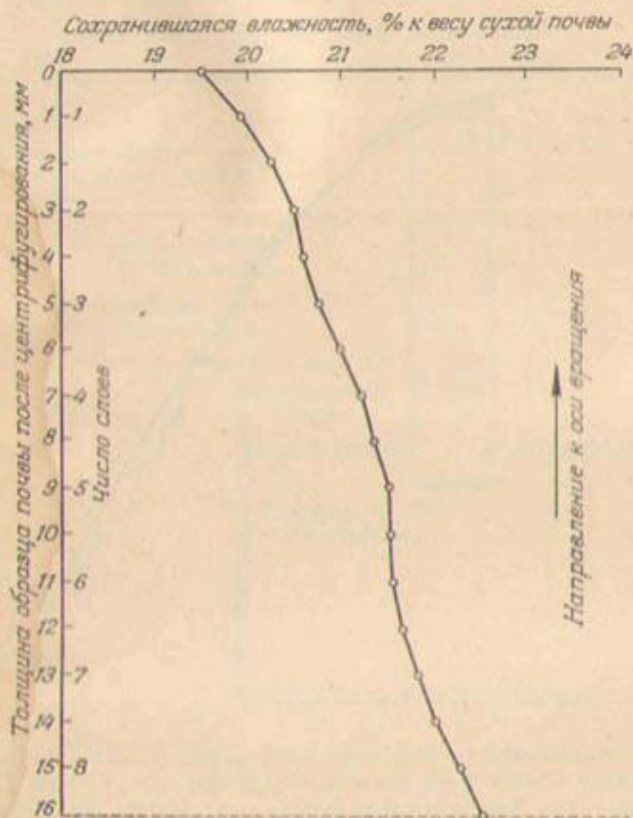
Рис. 107. Распределение влажности в 60-граммовой пробе тяжелого суглинка Йоло после действия на нее в течение получаса центробежной силы, в тысячу раз превышающей силу тяжести.
