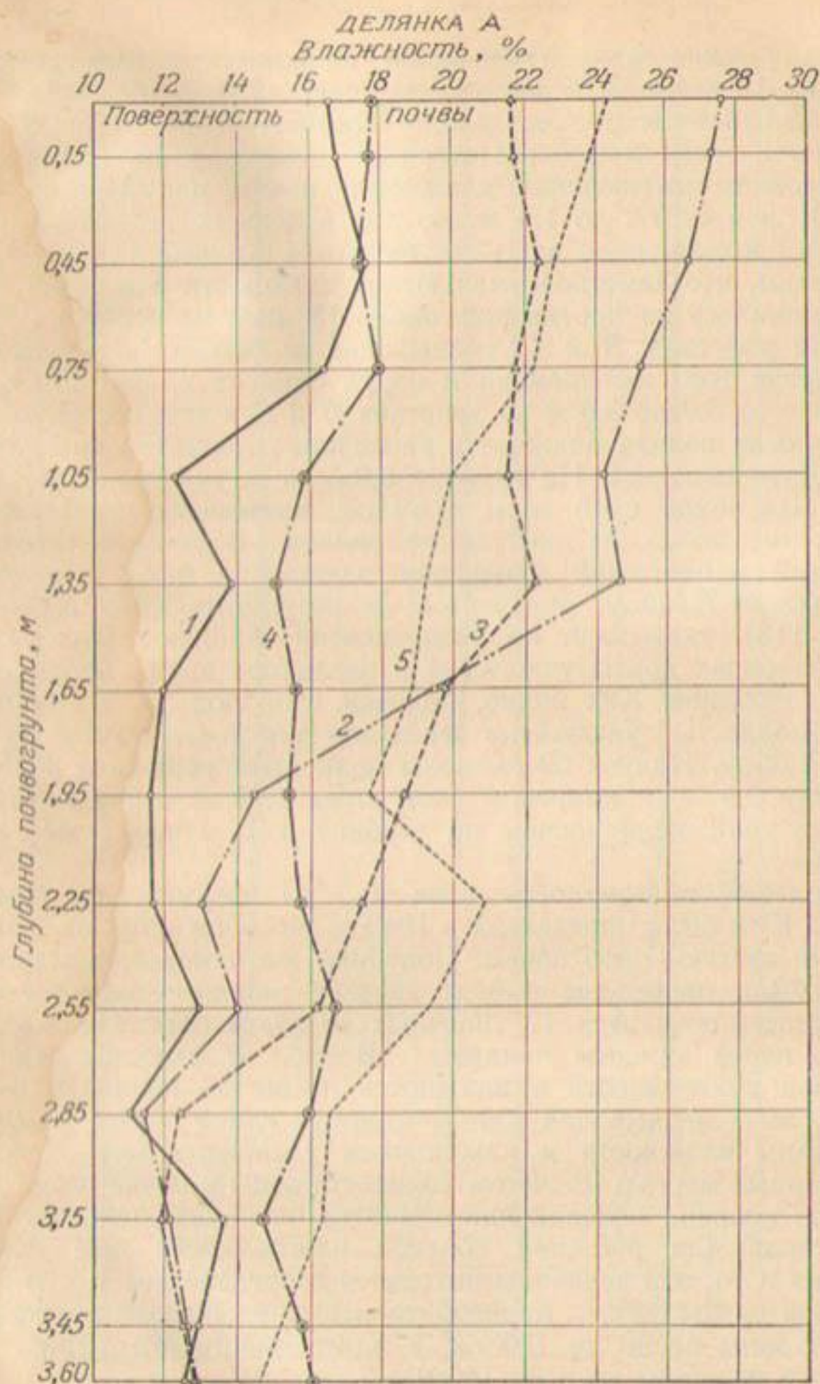
Р и с. 118. Распределение влаги в почве в различные периоды после полива слоем 30 см.
