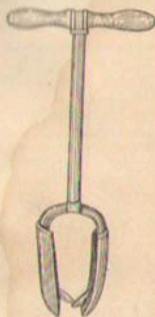
Рис. 111. Почвенный бур, применяемый для бурения ям под столбы. Подобными бурами малого диаметра пользуются для исследования распределения оросительной воды в почве.
