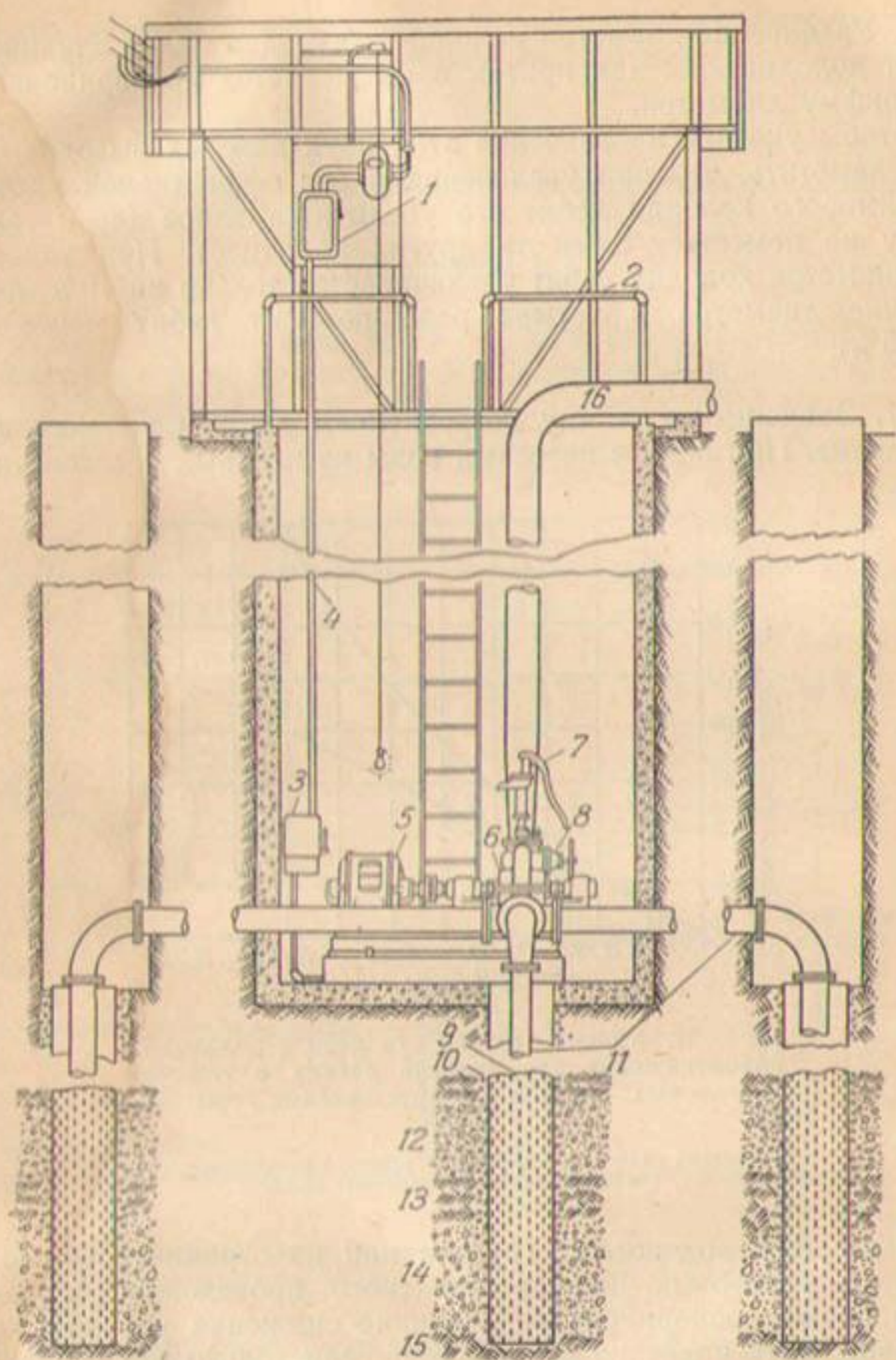
Р и с. 64. Горизонтальный центробежный насос, установленный в шахте и непосредственно соединенный с электромотором; насос выкачивает воду одновременно из трех колодцев.
