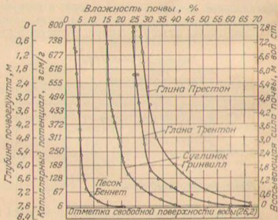
Рис. 137. Капиллярная влагоемкость при состоянии равновесия с грунтовой водой; показана для почв 4 типов (по опытам Ричардса).
