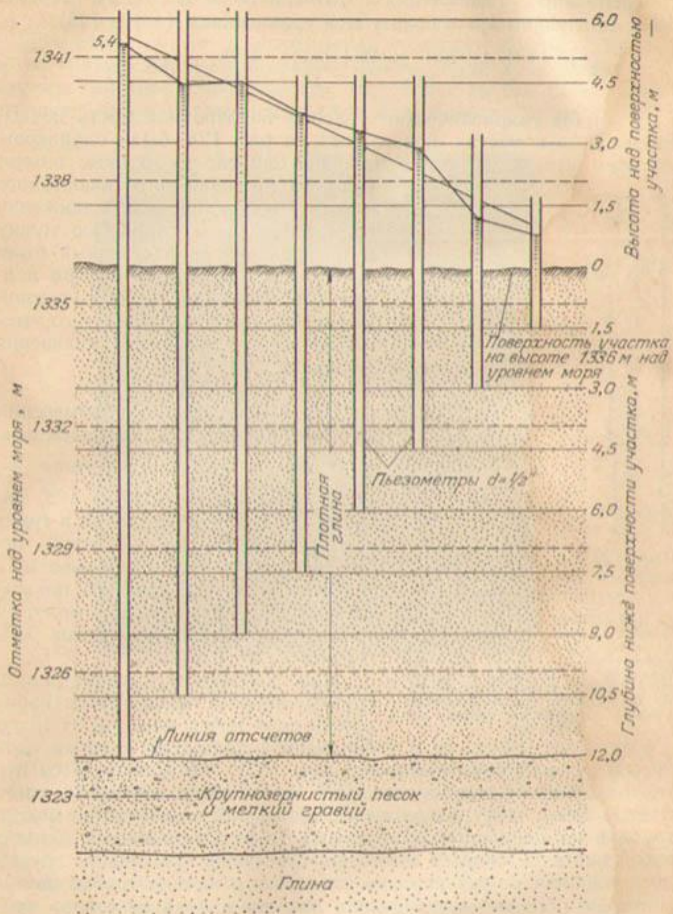
Р и с. 128. Схема определения среднего напора давления, построенная на основе результатов 24 измерений на 8 глубинах глинистого грунта, подстилаемого артезианским водоносным слоем.
