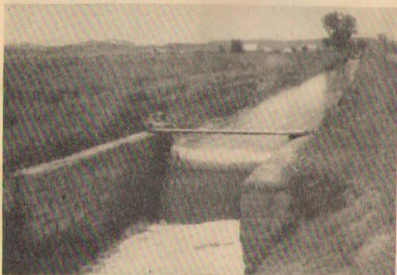
Рис. 44. Каменный перепад с длинным водобоем ниже перепада, уменьшающим размыв. Перепад пригоден для малых каналов и при небольшой высоте падения.
