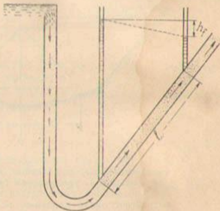
Рис. 125. Схема измерения гидравлического уклона.
