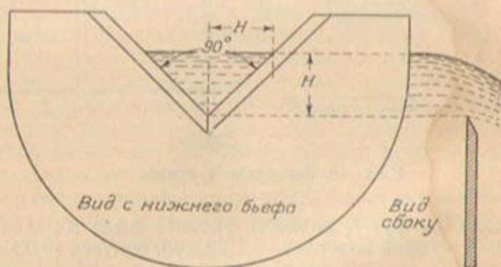
Рис. 15. Треугольный водослив с углом выреза 90°.
