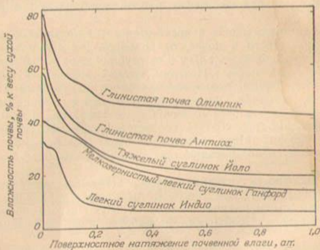
Рис. 121В. Поверхностное натяжение почвенной влаги в пределах 1 ат при различных значениях влажности для 5 видов почв Калифорнии.
