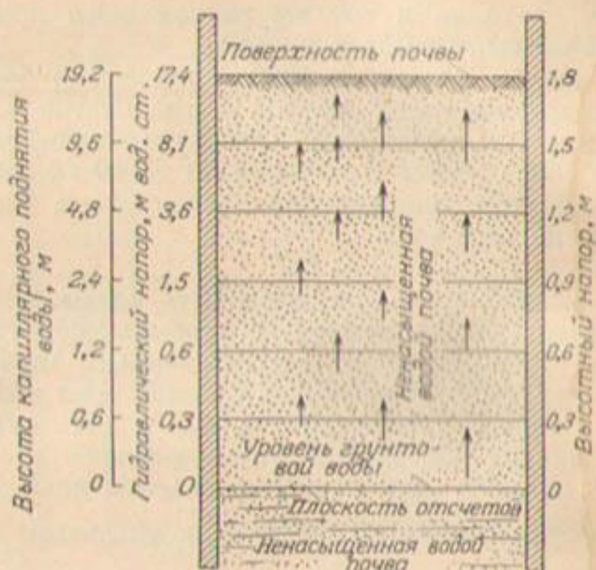
Рис. 136. Восходящий ток капиллярной воды, вызванный быстро увеличивающимся гидравлическим напором.
