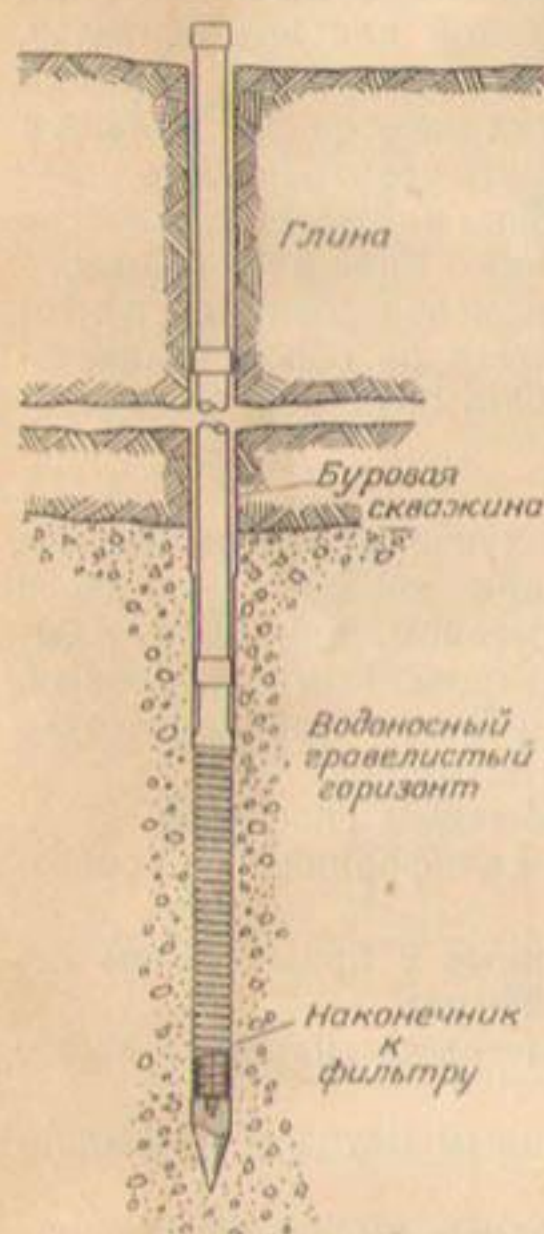
Р и с. 58. Вертикальное сечение колодца, сооруженного с помощью ударного инструмента.
