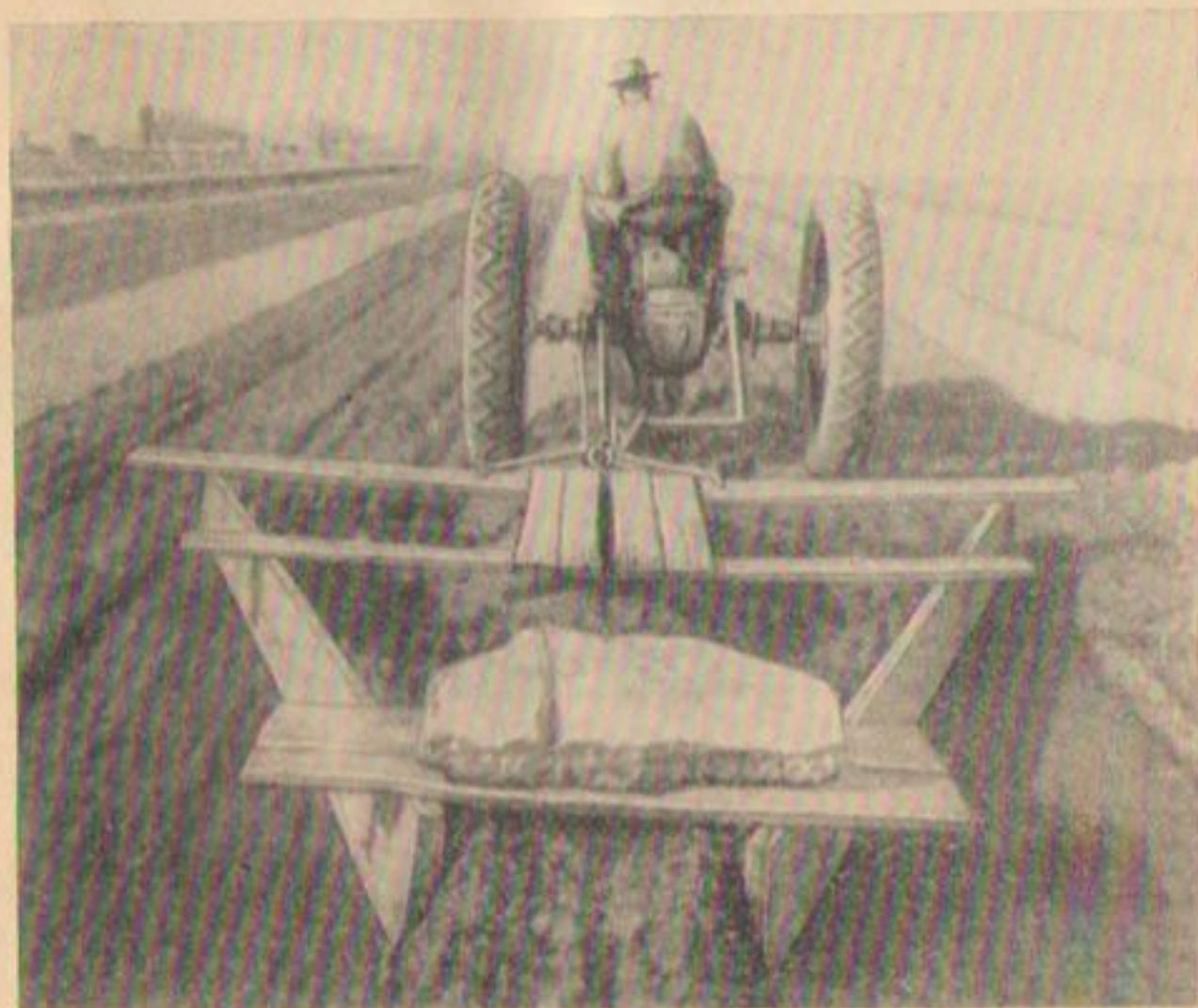
Рис. 87. Устройство валиков, ограничивающих поливные полосы.
