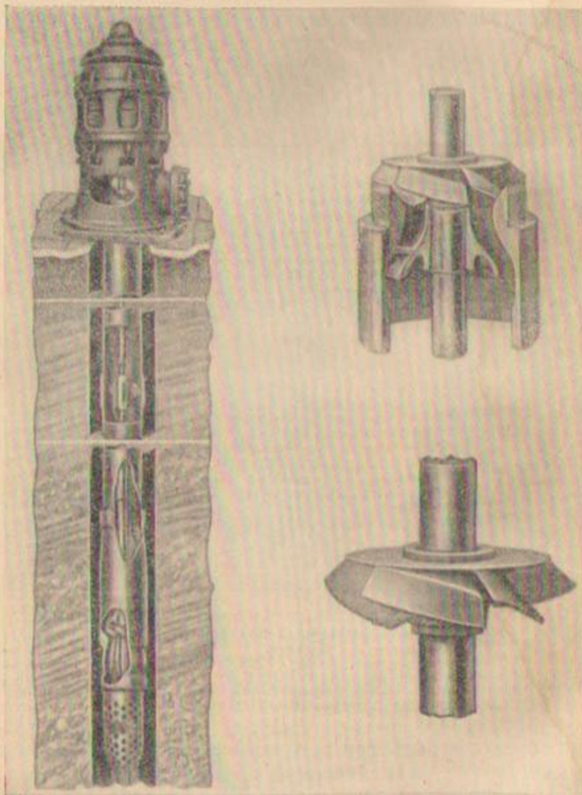
Рис. 55. Продольный разрез турбинного насоса с мотором, детали камеры и рабочее колесо, насаженные на вал.
