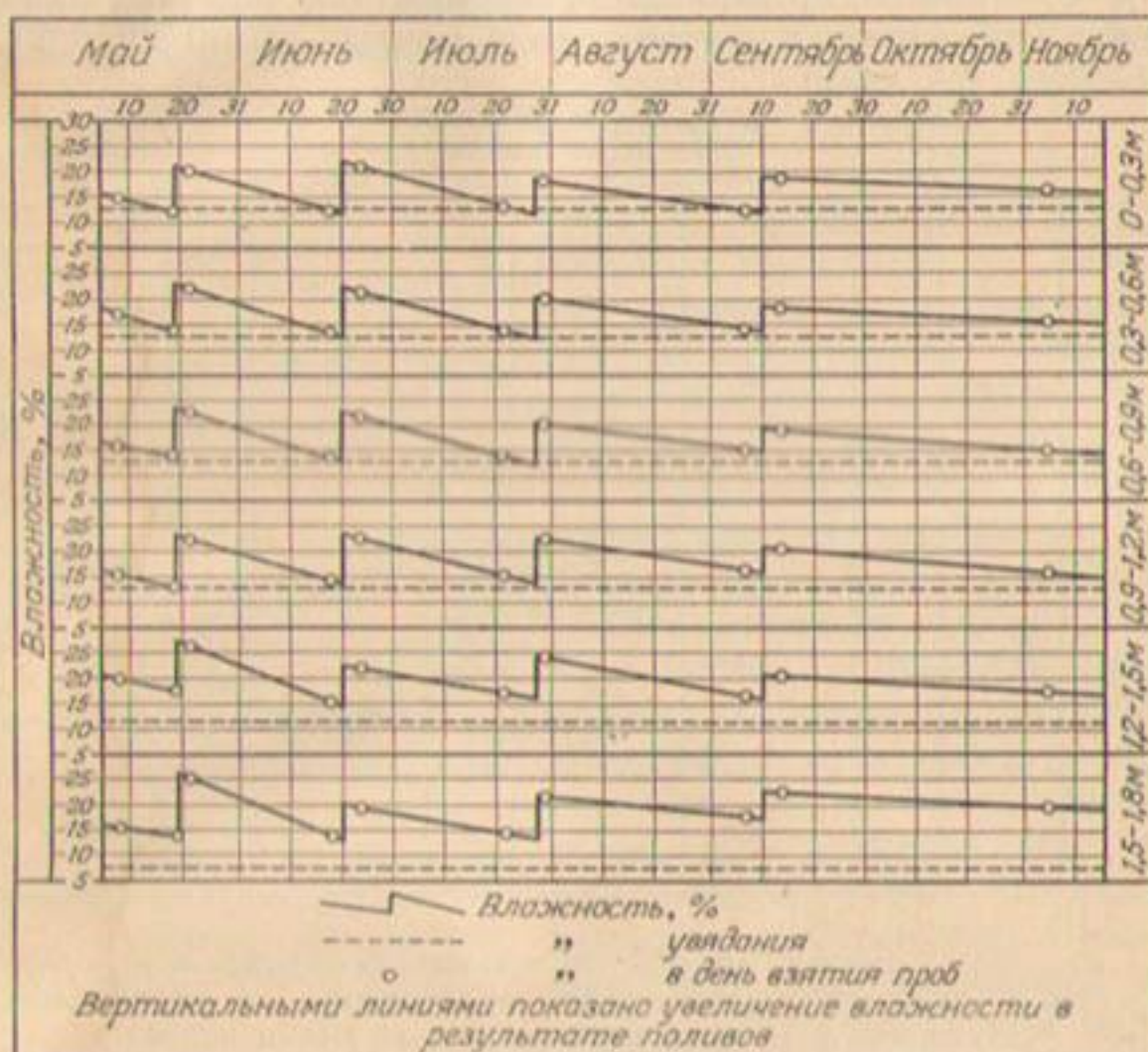
Рис. 155. Графики сезонных изменений влажности почвы на поле под люцерной.
