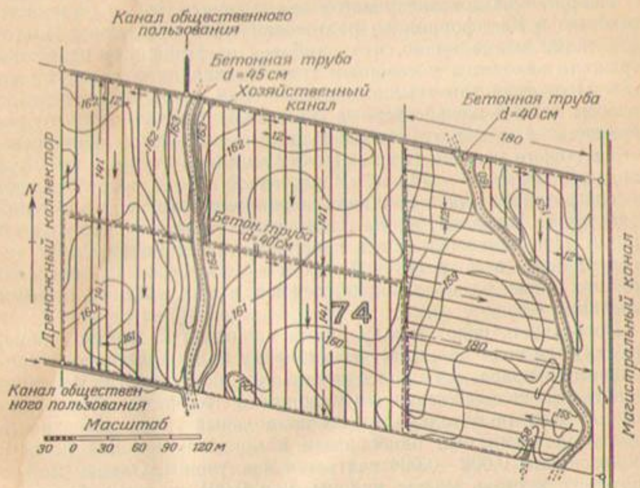
Р и с. 68В. План расположения полос, ограниченных по сторонам валиками, и каналы для подачи воды.
