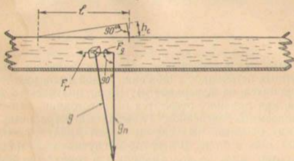
Рис. 29. Схема действия силы тяжести на единицу массы. Составляющая этой силы, параллельная поверхности воды, является движущей силой, заставляющей воду течь в канале.
