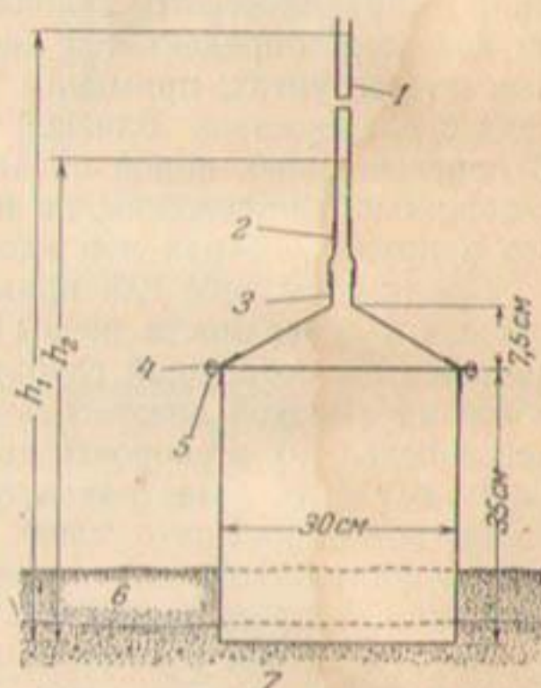
Рис. 133. Пермеаметр переменного напора.
