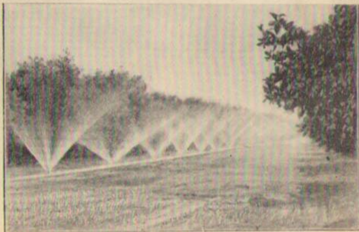
Рис. 169. Переносный трубопровод с неподвижными насадками с круговым разбрызгиванием для орошения цитрусового сада.
