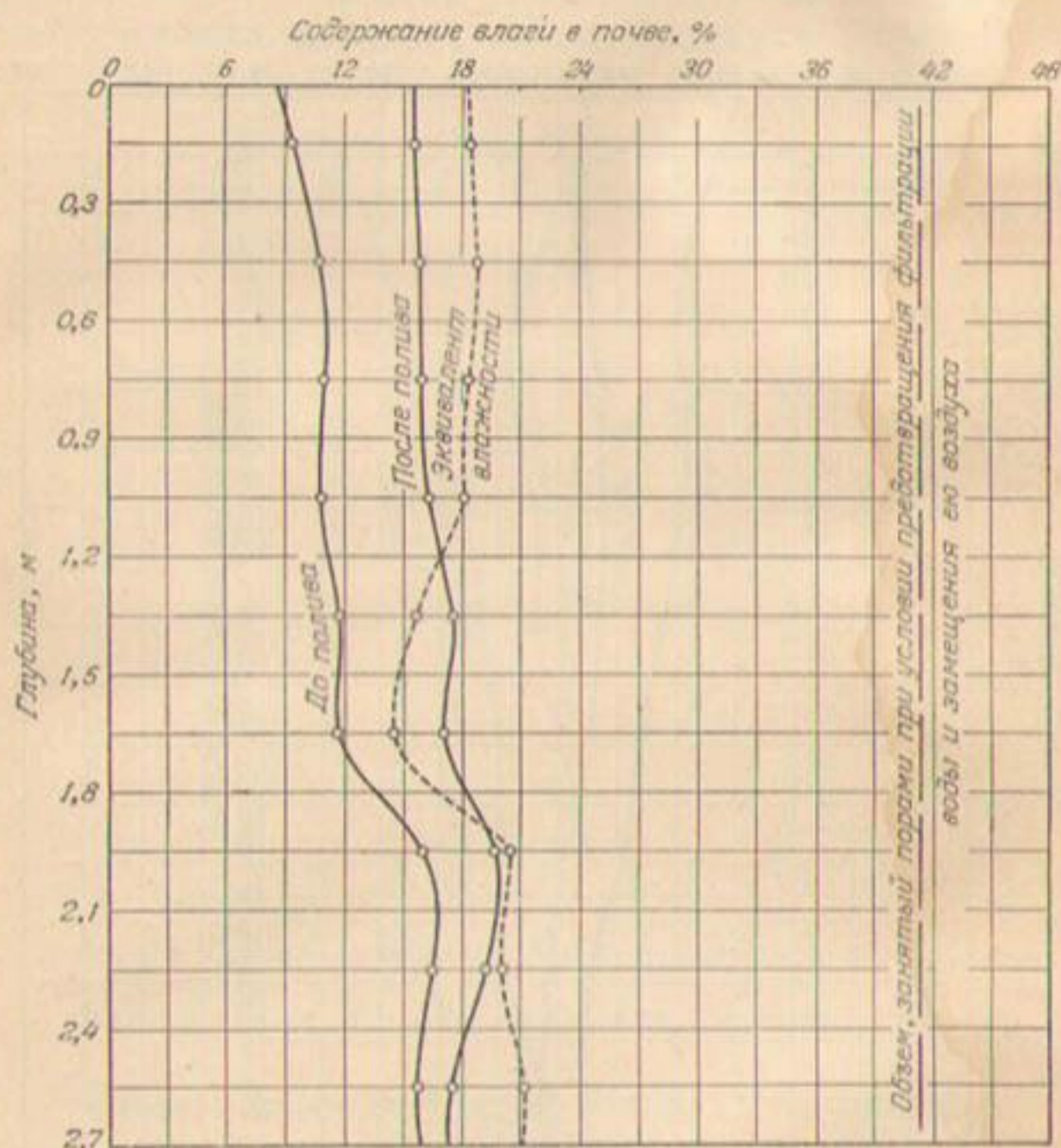
Рис. 113. Графики, показывающие содержание воды в почве до и после полива, эквивалент влажности и объем пор в илисто-суглинистых почвах, подстилаемых тонким песчанистым суглинком. Каждая кривая построена по средним значениям 68 проб.
