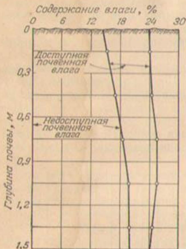
Рис. 123. Доступная и недоступная влага в верхнем 1,5-метровом слое одного из видов почв Калифорнии, по определению Эдлефсена.
