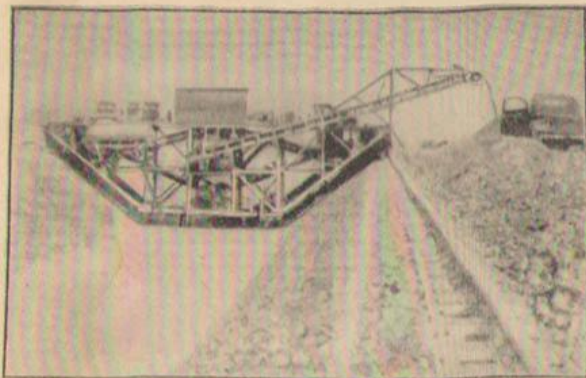
Рис. 40. Машина для облицовки и отделки поверхности канала.
