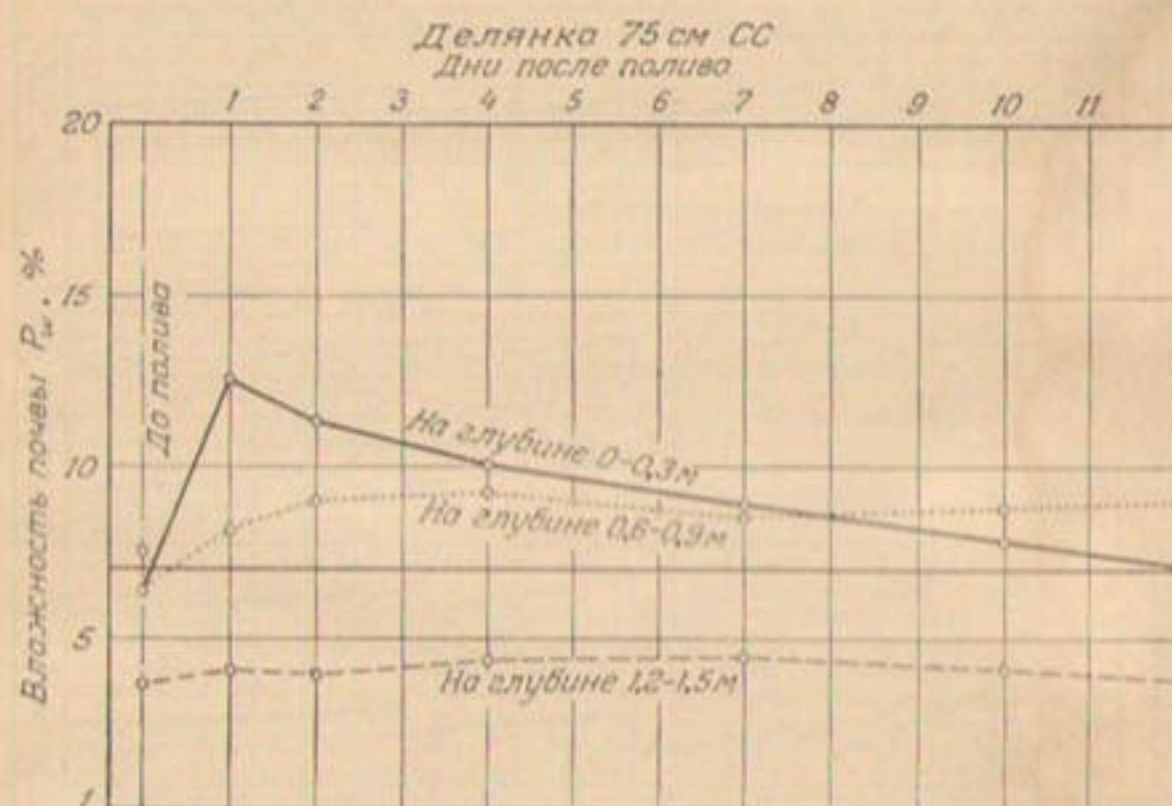
Рис. 154. Графики увеличения влажности почвы вследствие поливов люцерны, подвергшейся культивации, и уменьшения влажности в течение первых 10 дней после полива.
