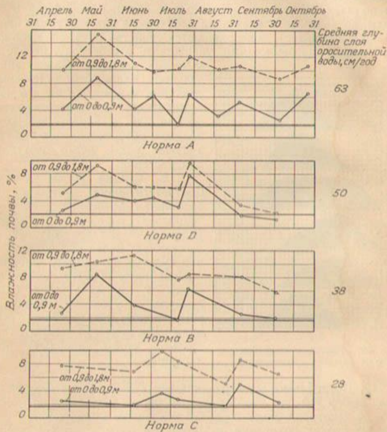
Рис. 156. Влажность почвы в плодовом саду в зависимости от количества воды, расходуемой для полива. Влажность длительного увядания на глубине от 0 до 90 см показана сплошными горизонтальными линиями.
