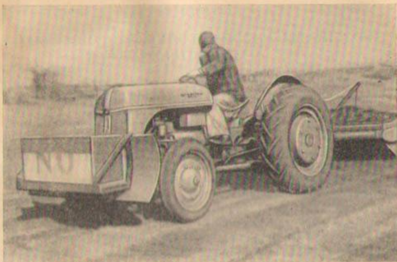
Р и с. 84. Сельскохозяйственный трактор и небольшой скрепер, применяемые для планировки участка. Ящик впереди трактора обеспечивает большую нагрузку на передние колеса, что облегчает заполнение скрепера грунтом.
