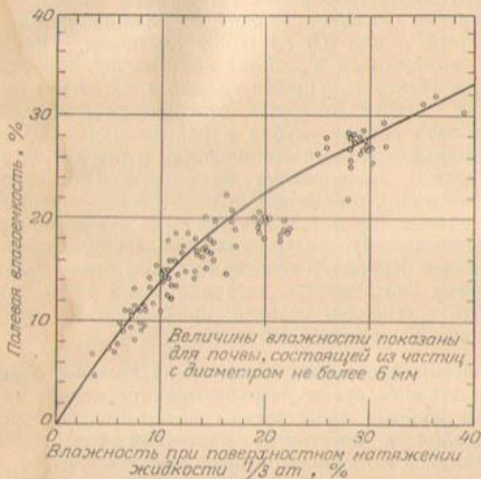
Рис. 120. Зависимость между полевой влагоемкостью почвы и ее влажностью при величине поверхностного натяжения жидкости \frac{1}{3} ат.
