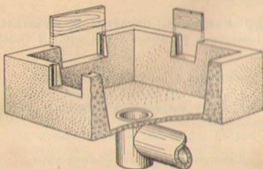
Р и с. 27. Водосливной ящик для пропорционального деления воды.
