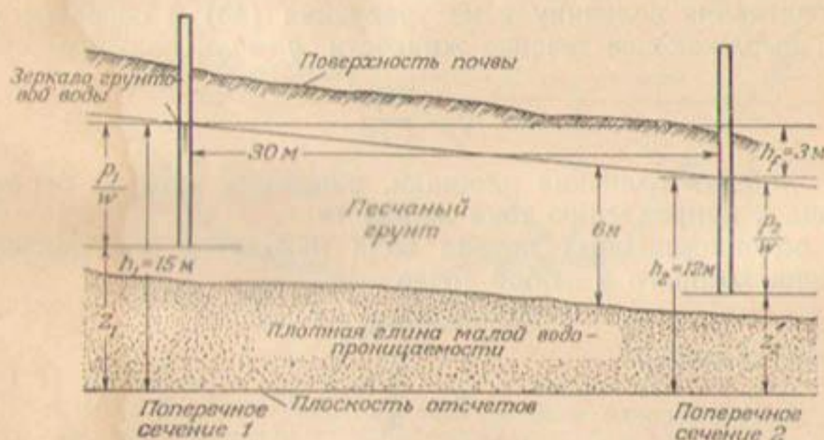
Рис. 127. Ток свободной грунтовой воды в насыщенном водой песчаном грунте, подстилаемом плотной глиной.
