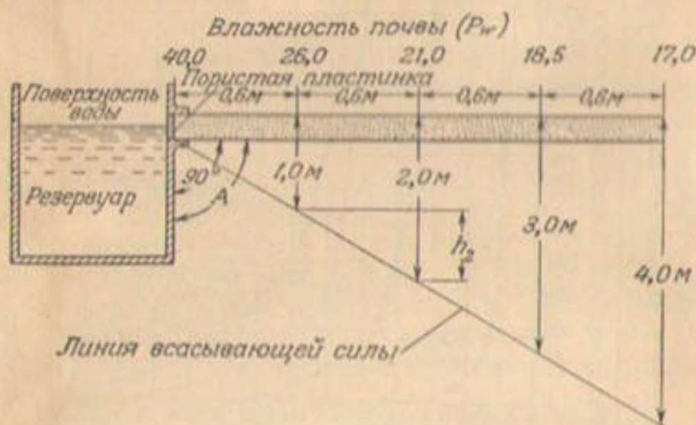
Рис. 138. Установившийся ток капиллярной воды в горизонтальной трубке небольшого диаметра, заполненной почвой с влажностью 40% у левого конца и 17% у правого.
