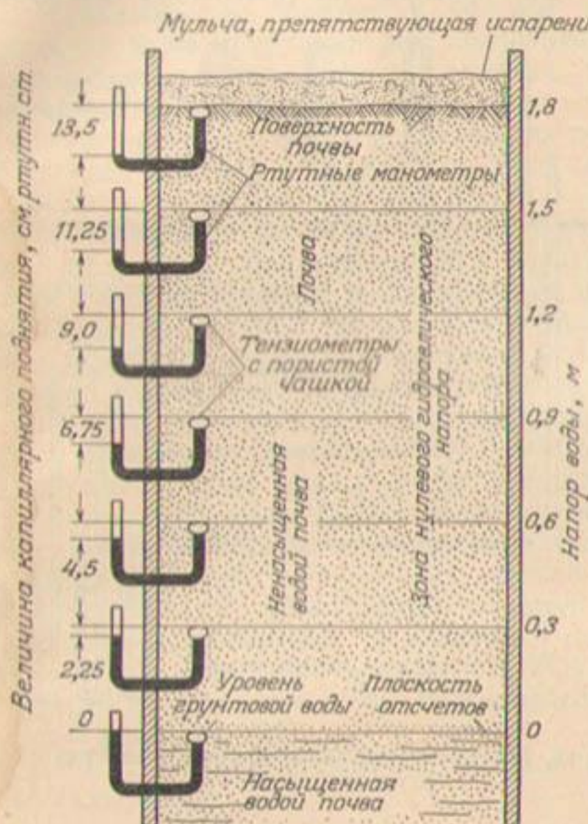
Рис. 135. Схема тока капиллярной воды, находящейся выше насыщенной водой почвы, и положения уровня грунтовой воды в зоне одинаковых гидравлических напоров. Вода в почве находится в состоянии покоя.
