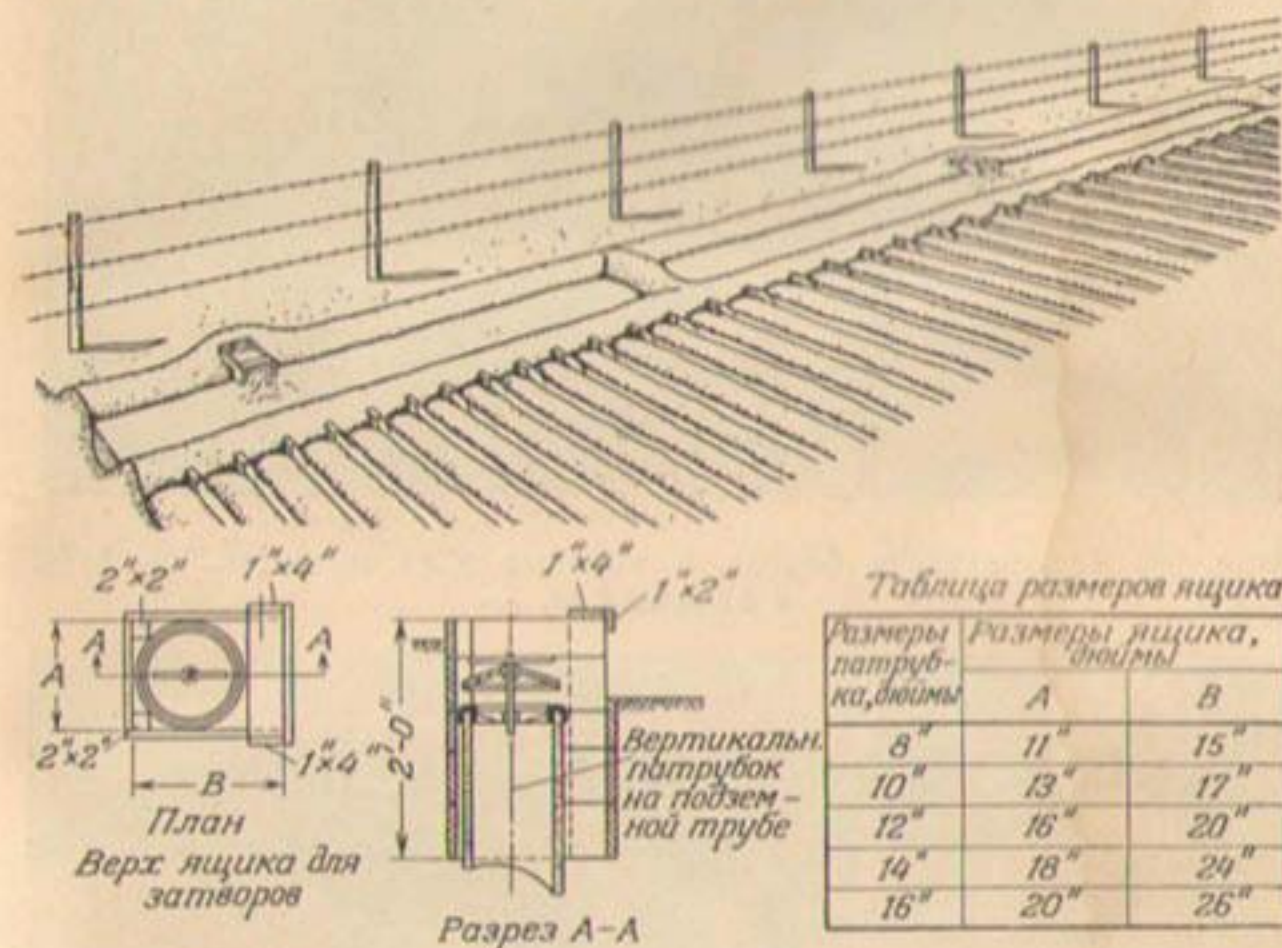
Рис. 98. Подача воды в каналы с применением подземной системы труб с задвижками на вертикальных патрубках. С помощью передвижных ящиков в устье патрубков устраняется размыв вокруг задвижек на песчаных почвах, и вода направляется в оросительные каналы.
