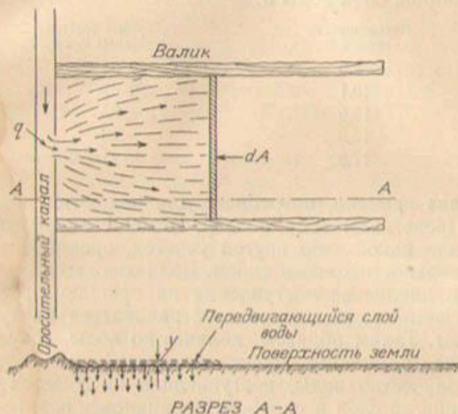
Рис. 70. Схема подачи оросительной воды на полосу. Показано продвижение воды на бесконечно малую площадку dA в бесконечно малое время dt , а также фильтрация воды в почву в верхней части полосы.
