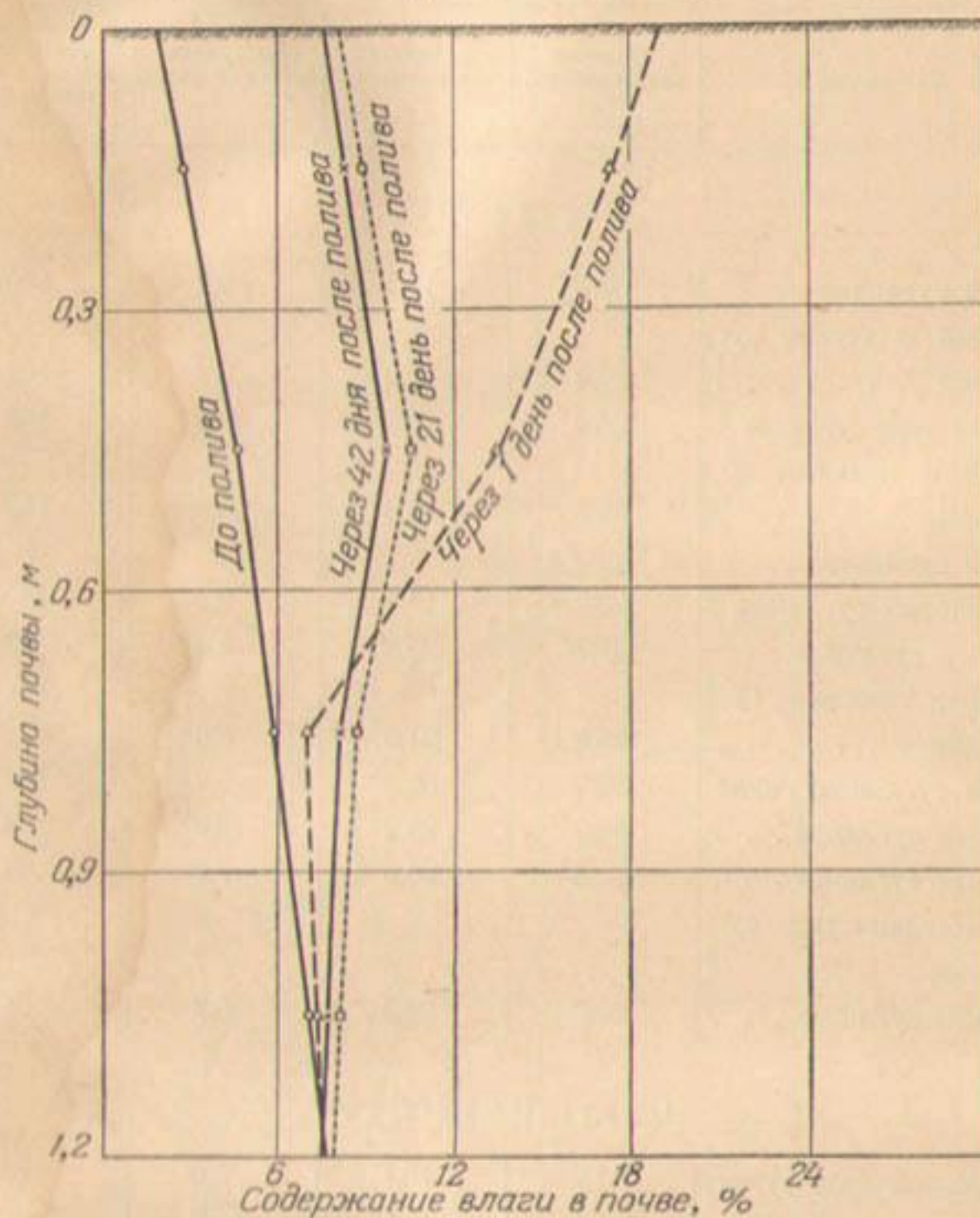
Рис. 119. Распределение влаги в почве до полива и в различные периоды после полива (в районе Якима штата Вашингтон).
