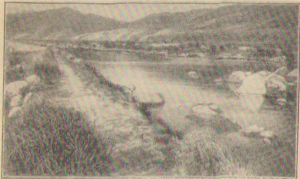
Р и с. 10. Дамба, построенная насыпкой грунта на глыбы камня в ложе реки, замедляет течение и способствует образованию лиманов, простирающихся от гребня одной дамбы до другой, расположенной выше по течению.
