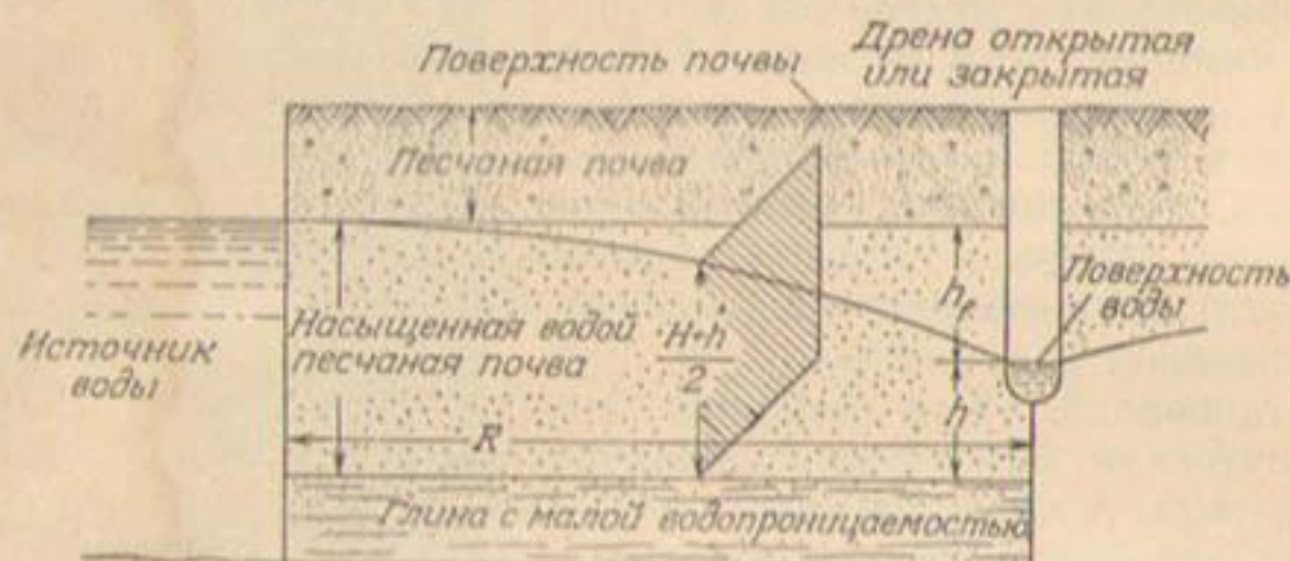
Рис. 150. Схема прямолинейных токов грунтовых вод в направлении к дренам с расстоянием между ними 2R . Уровень грунтовых вод находится на H-h выше горизонта воды в дренах, проложенных в песчаной почве, подстилаемой глиной.
