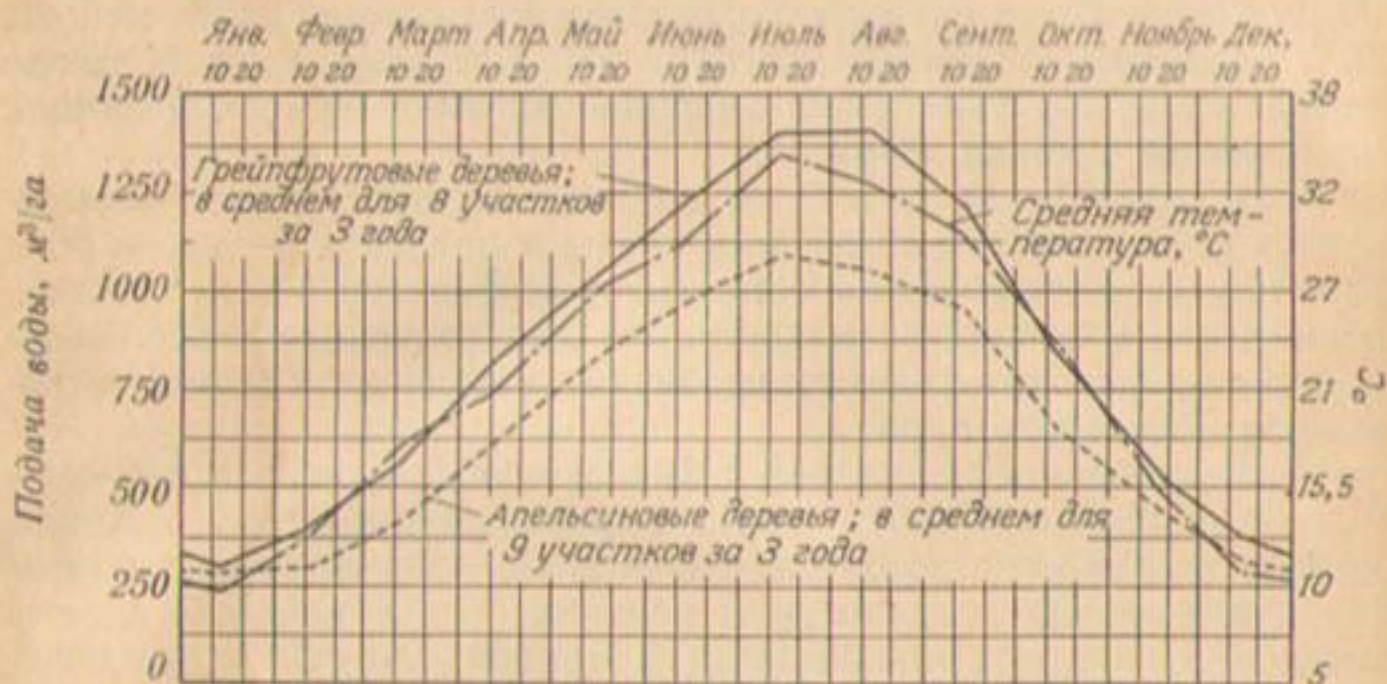
Рис. 176. Количество воды в \text{м}^3/\text{га} , потребляемой апельсиновыми и грейпфрутовыми деревьями при поливах с 30-дневными интервалами. Среднемесячные температуры в период проведения опытов.
