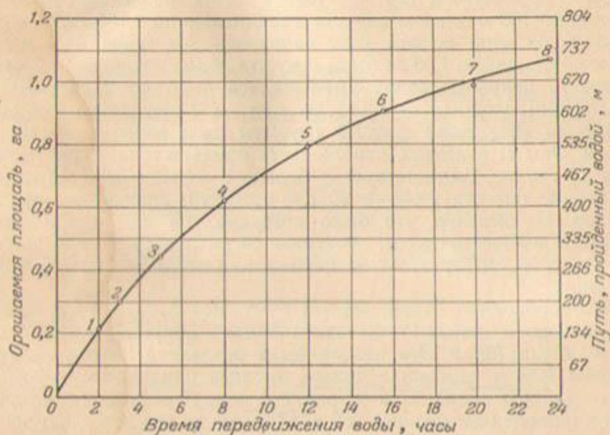
Рис. 72. Зависимость пути, пройденного водой, от времени ее передвижения по полосе шириной 15 м при постоянном расходе 64,5 л/сек.
