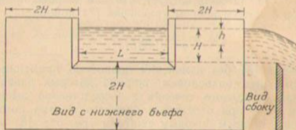
Рис. 13. Прямоугольный водослив с полным боковым сжатием.
