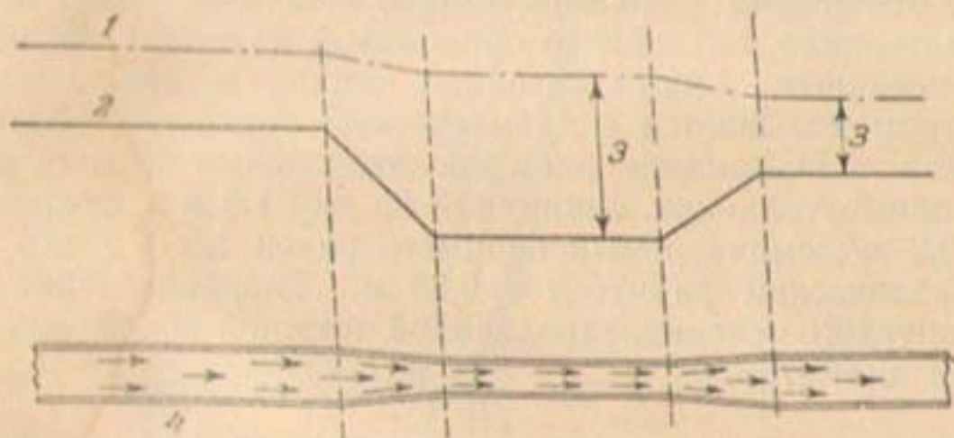
Рис. 33. Уклон линии градиента энергии, всегда направленный в сторону течения воды.
