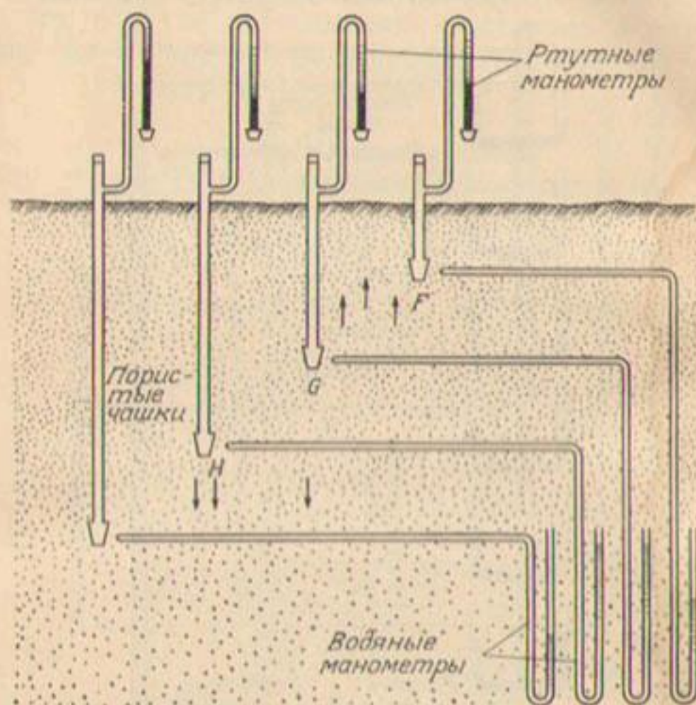
Рис. 134. Установка тензиометра с применением ртутных манометров.
