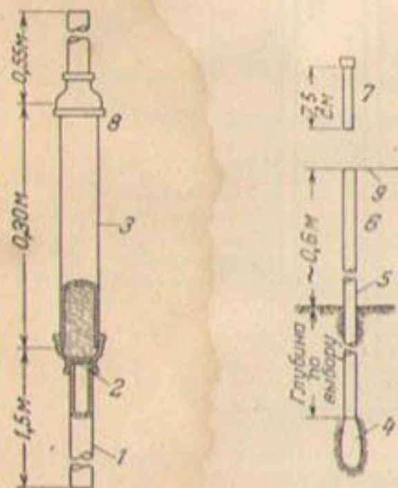
Рис. 129. Детали пьезометра и молота для забивания трубок пьезометра в грунт.
