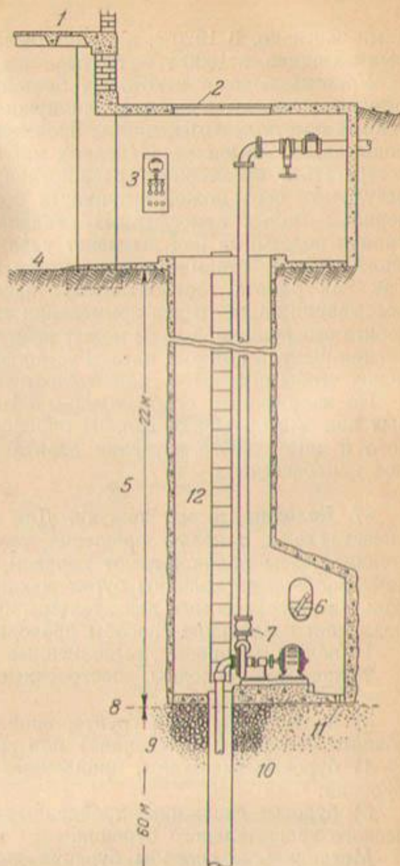
Р и с. 59. Центробежный насос с электромотором. Установка находится в копаном колодце; вода выкачивается из бурового колодца.
