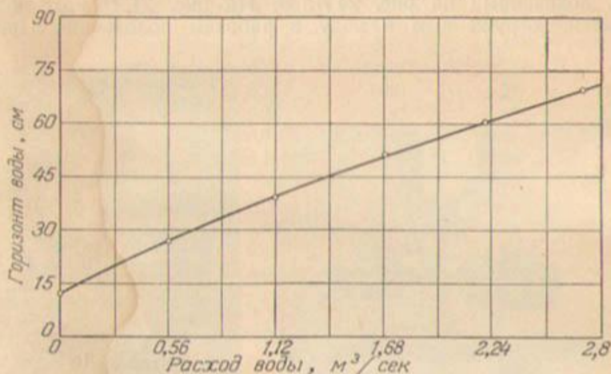
Рис. 25. Кривая расхода воды в оросительном канале.
