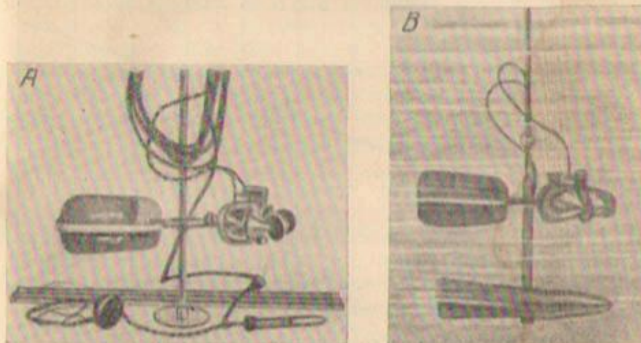
Р и с. 24. А — гидрометрическая вертушка системы Лейд, подвешенная на стержне с круглым опорным диском; В — гидрометрическая вертушка системы Герли в работе.
