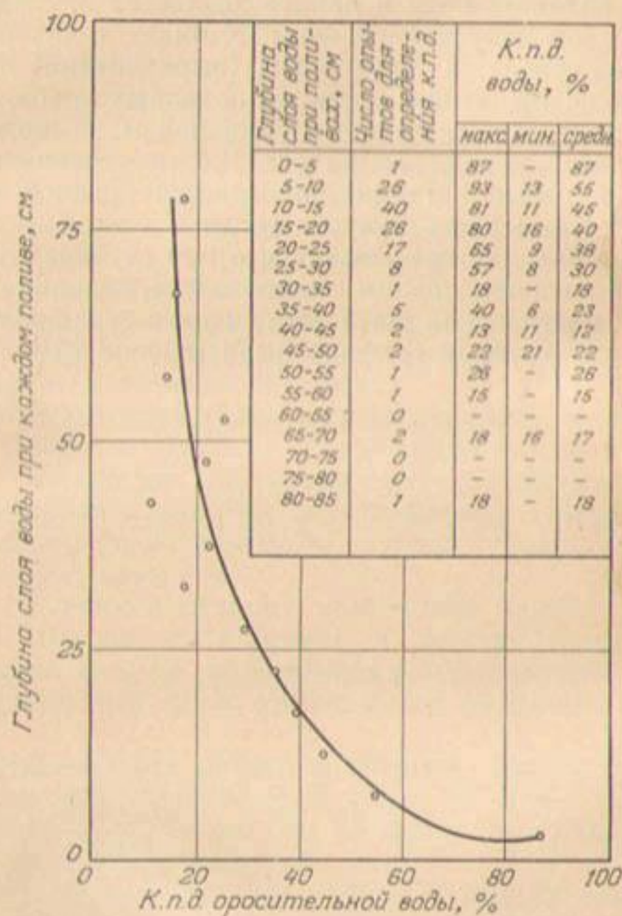
Р и с. 124. Зависимость величины к. п. д. от высоты слоя оросительной воды при каждом поливе.
