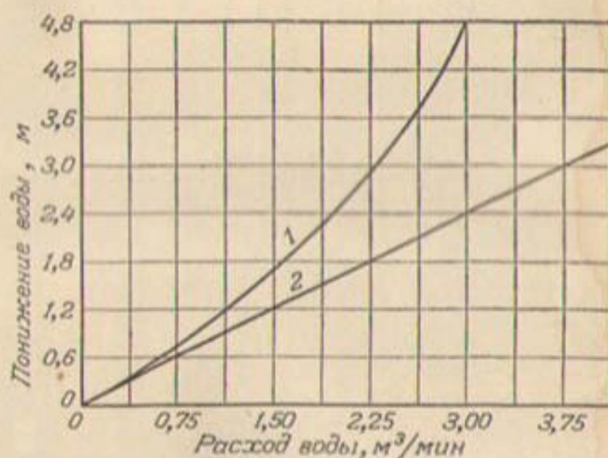
Рис. 63. Кривые зависимости дебита колодца от водопонижения для условий легких и тяжелых водоносных грунтов и в артезианских грунтовых водах.
