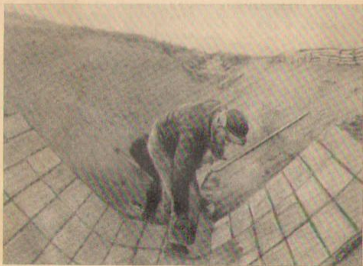
Р и с. 37. Облицовка канала бетонными плитами (размер 20 \times 60 \text{ см} ), соединяемыми в шпунт.
