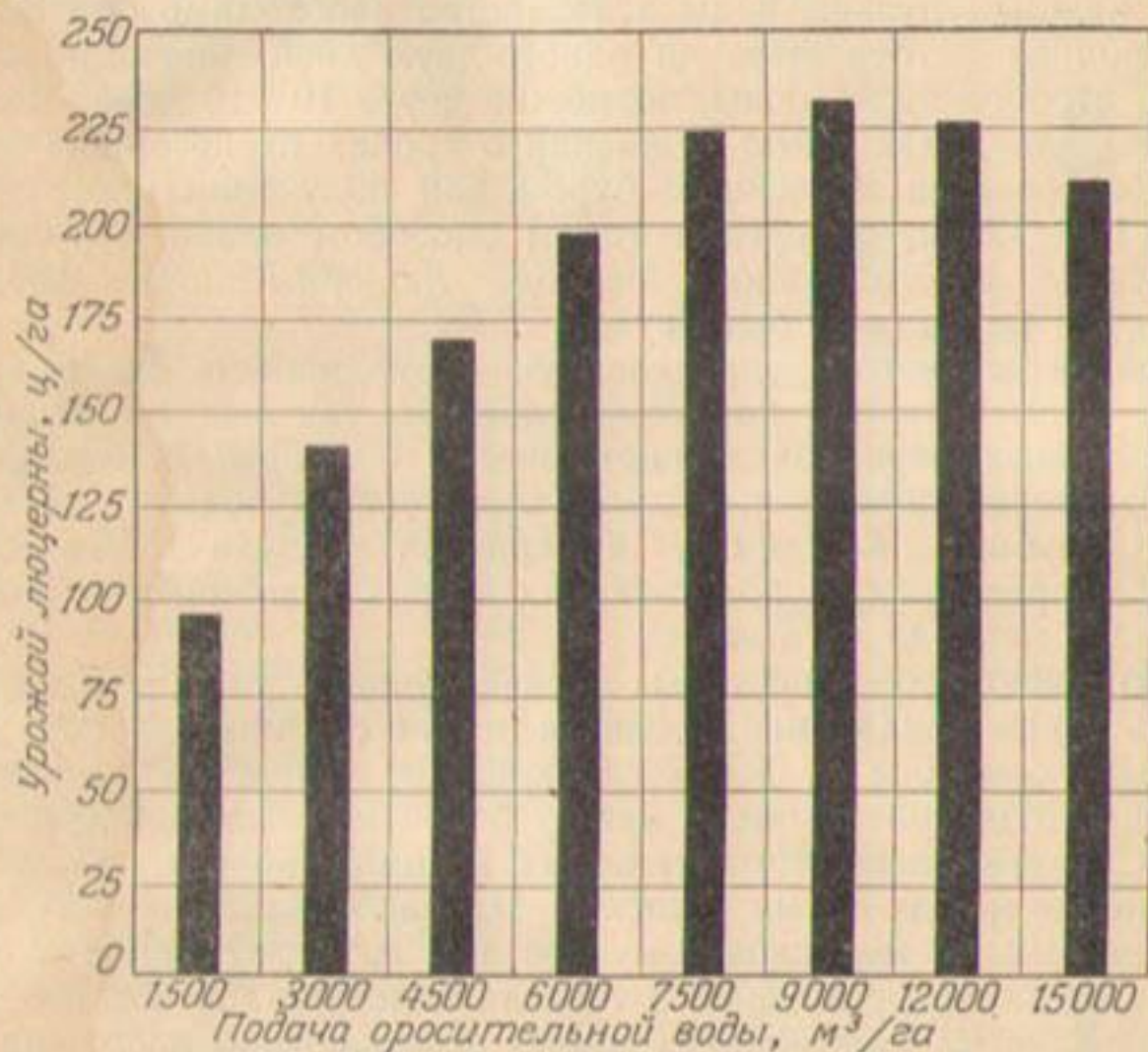
Рис. 165. Диаграмма, показывающая результаты опытов, проведенных на ферме университета в Калифорнии в 1910—1915 гг., по определению необходимой нормы воды для поливов люцерны. Наилучшие урожаи были получены при подаче на поле воды от 7500 до 9000 м³/га.
