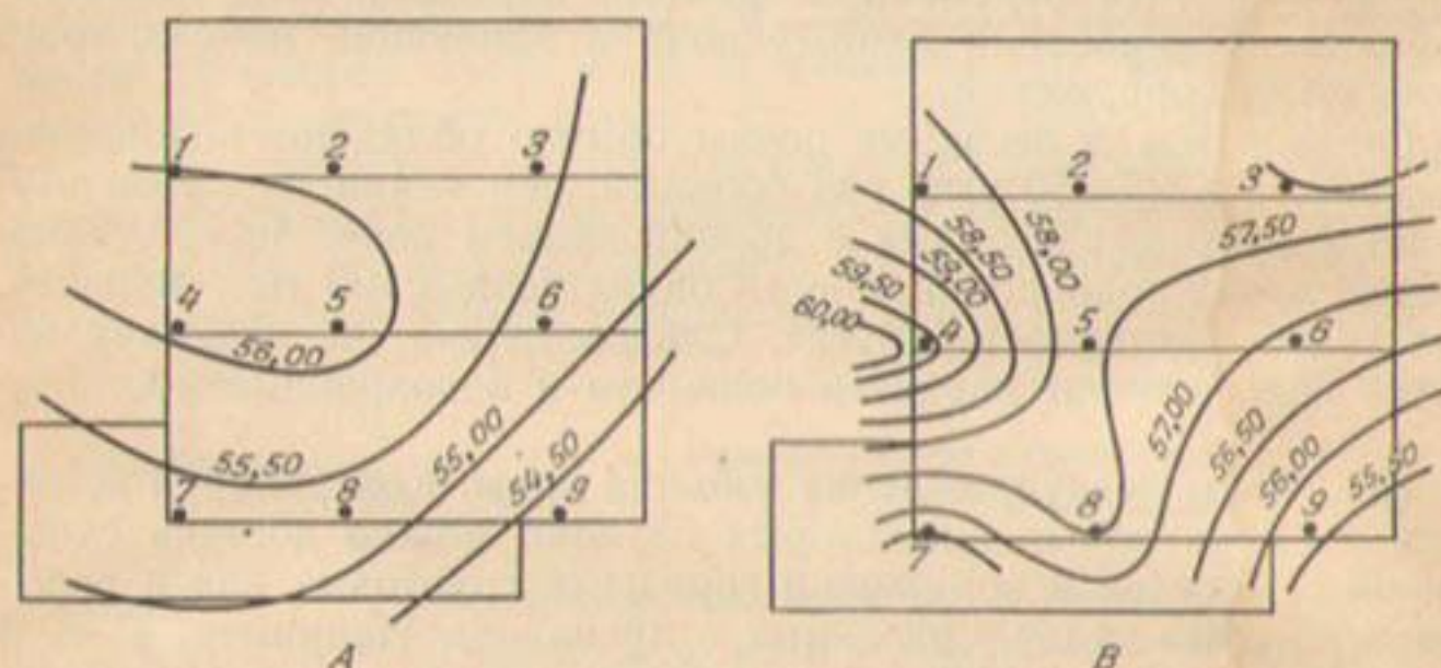
Р и с. 144. Уровень грунтовых вод на опытном поле.
