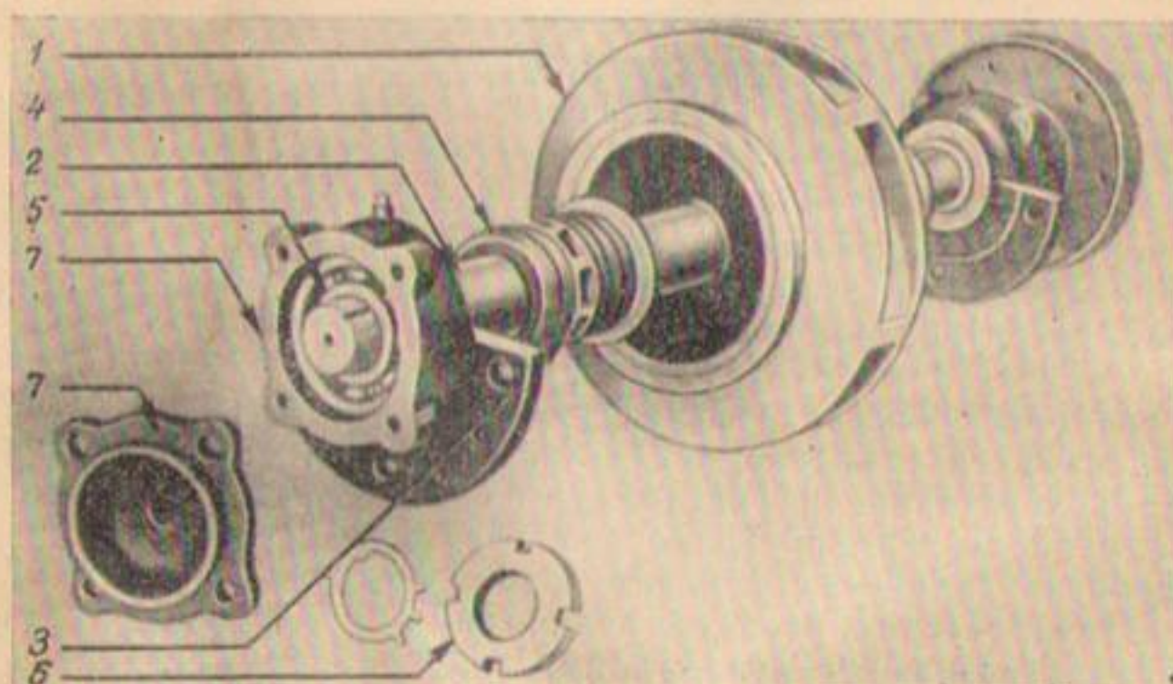
Р и с. 52. Рабочее колесо и вал насоса.
