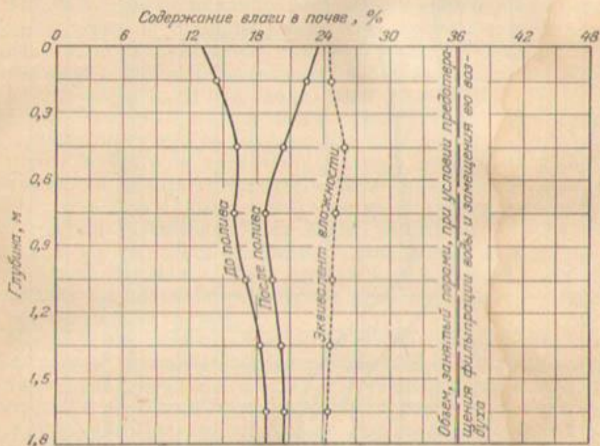
Рис. 115. Графики содержания воды до и после полива, эквивалент влажности и объем пор в тяжелых суглинистых почвах. Каждая кривая построена по средним значениям 148 проб.
