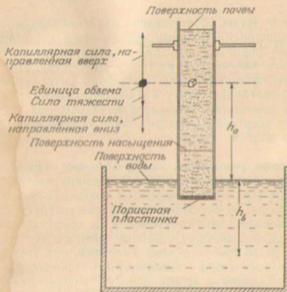
Рис. 105. Схема, показывающая равенство вертикальных сил, действующих на воду в любой единице объема почвы, в которой капиллярная вода находится в равновесии с грунтовой водой.
