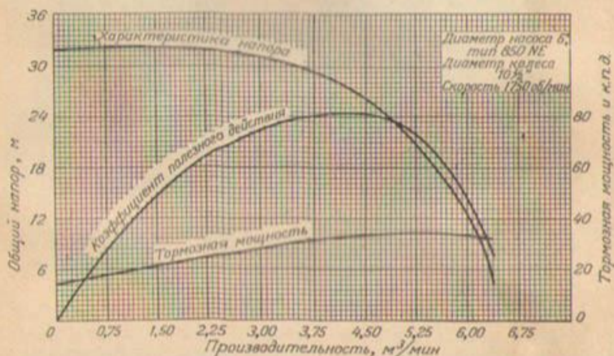
Рис. 50. Кривые характеристики насоса, построенные по опытным данным.
