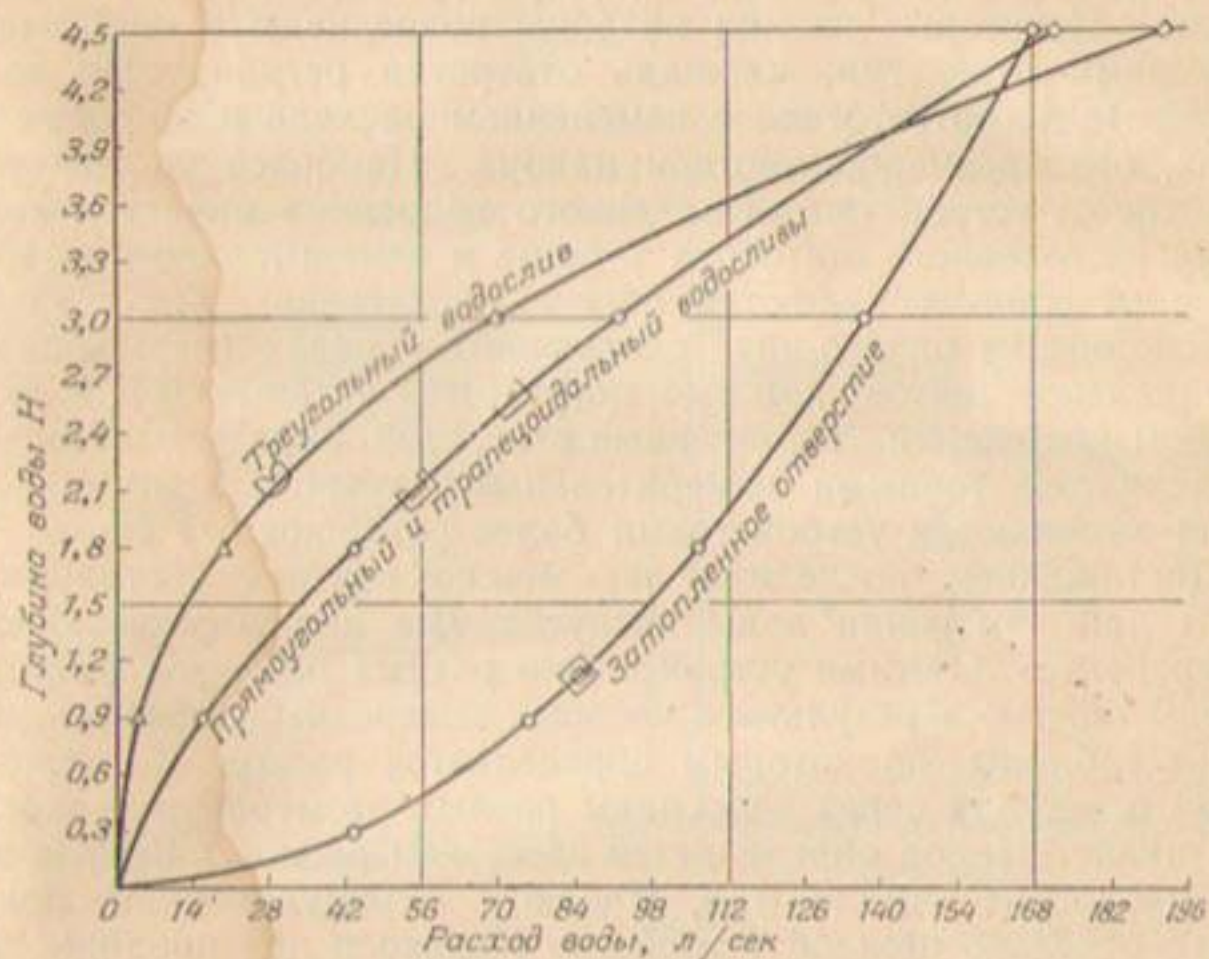
Рис. 17. Кривые, показывающие зависимость расхода воды (в л/сек) от глубины воды над порогом водослива (в дм) для 1-футового прямоугольного водослива с боковым сжатием, для 1-футового трапециoidalного водослива, для водослива с треугольным вырезом (угол 90^\circ ) и для затопленного отверстия с площадью сечения 0,09 \text{ м}^2 .
