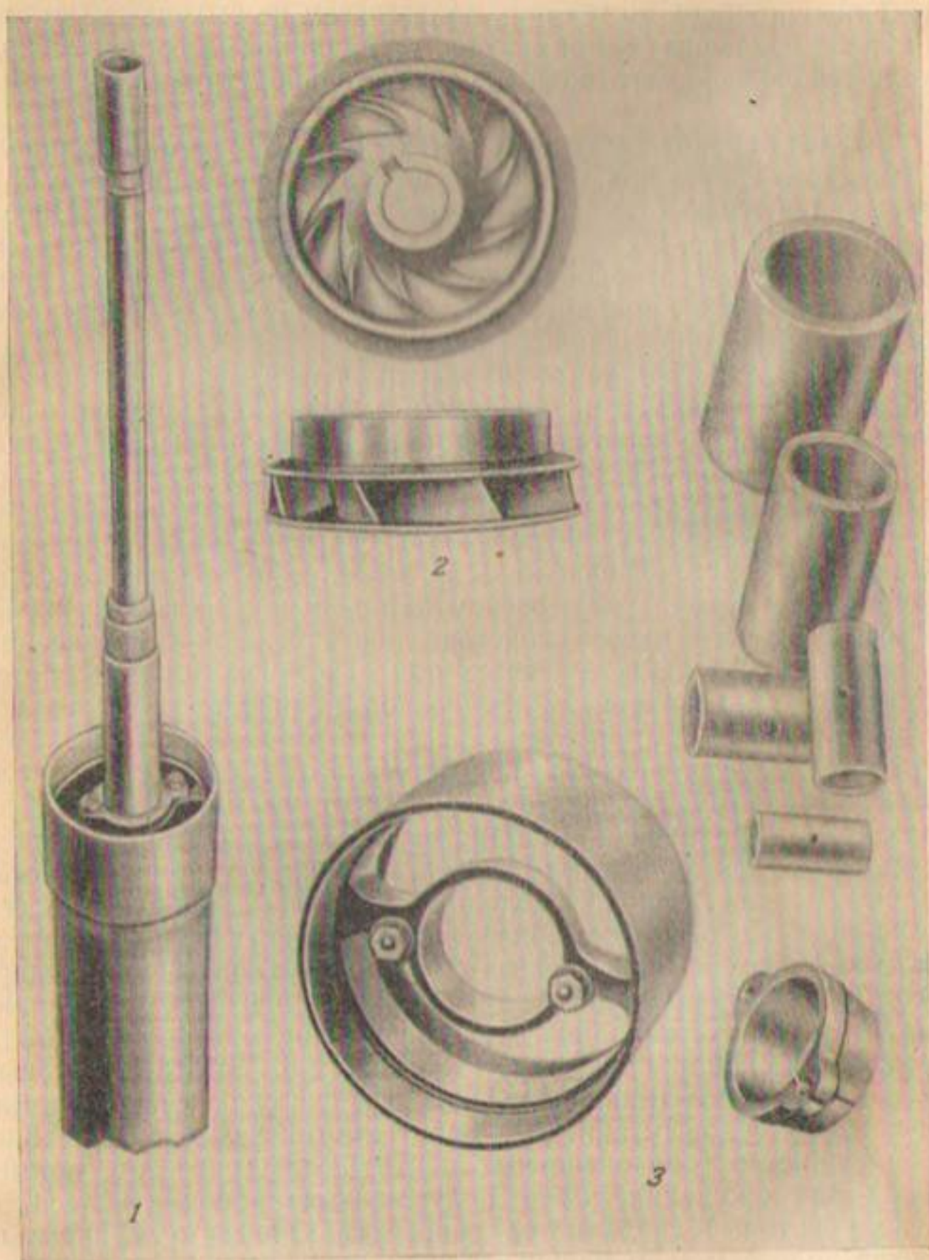
Р и с. 54. Отдельные части глубоководного турбинного насоса. 1 — общий вид насоса; 2 — рабочее колесо; 3 — спайдер насоса и соединительные муфты вала.
