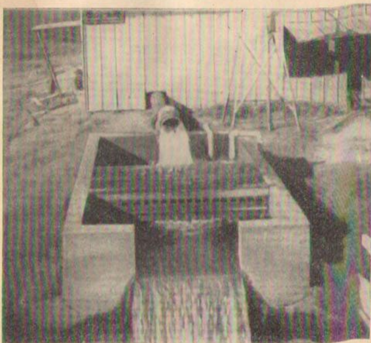
Рис. 66. Насосная установка. Вода поднимается насосом на 60 см выше, чем нужно. Успокоительный бассейн с тремя перегородками, действующий весьма эффективно.
