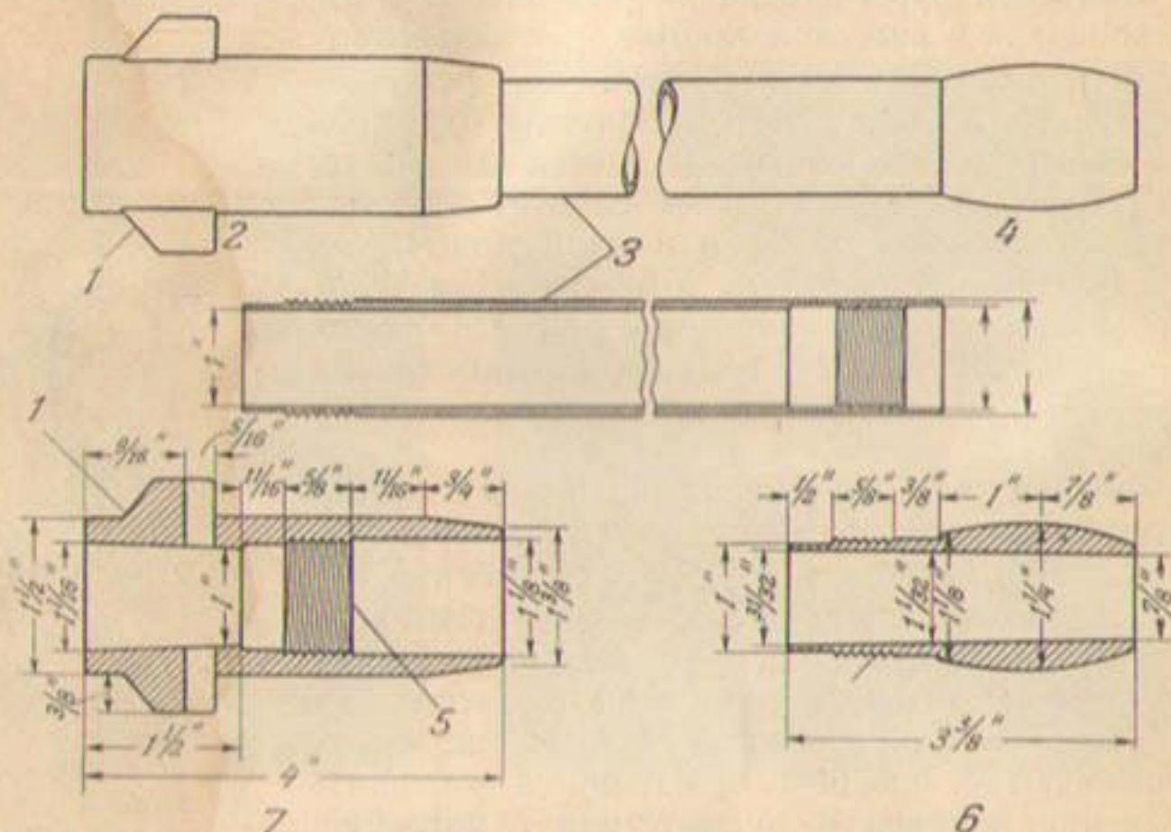
Рис. 112. Детали трубчатого бура.
