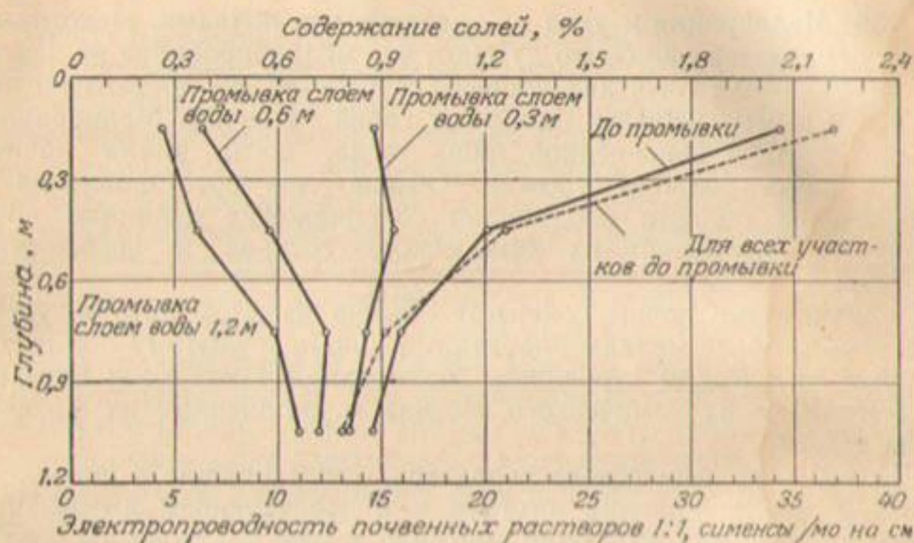
Рис. 142. Распределение солей в почве по глубине до и после ее промывки. Показаны результаты 3 промывок разными количествами воды
