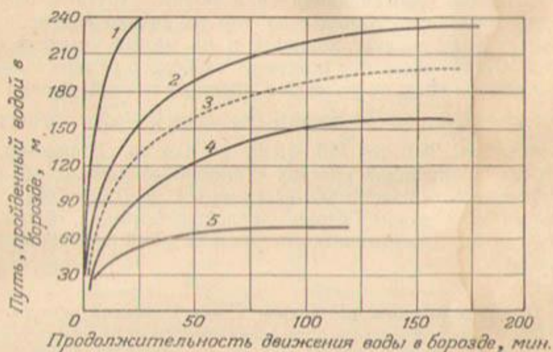
Рис. 73. Скорость передвижения воды при различных ее расходах на некоторой типичной почве при постоянном уклоне борозды.
