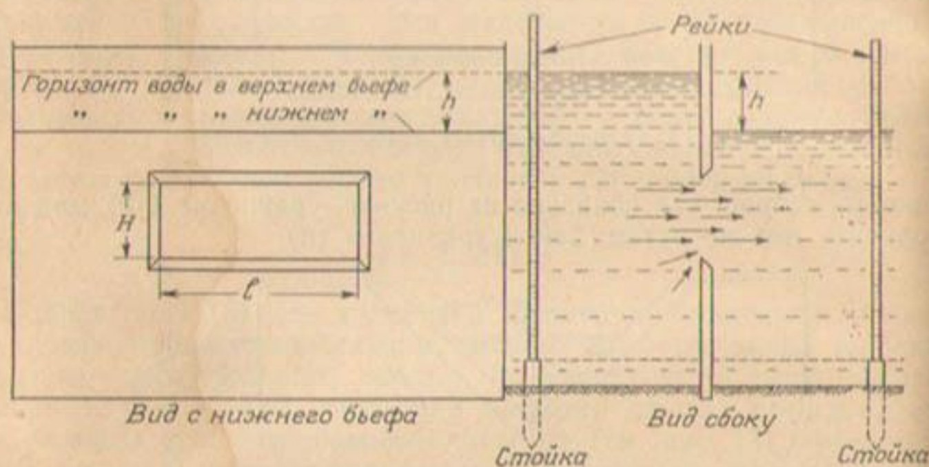
Р и с. 16. Затопленное отверстие.
