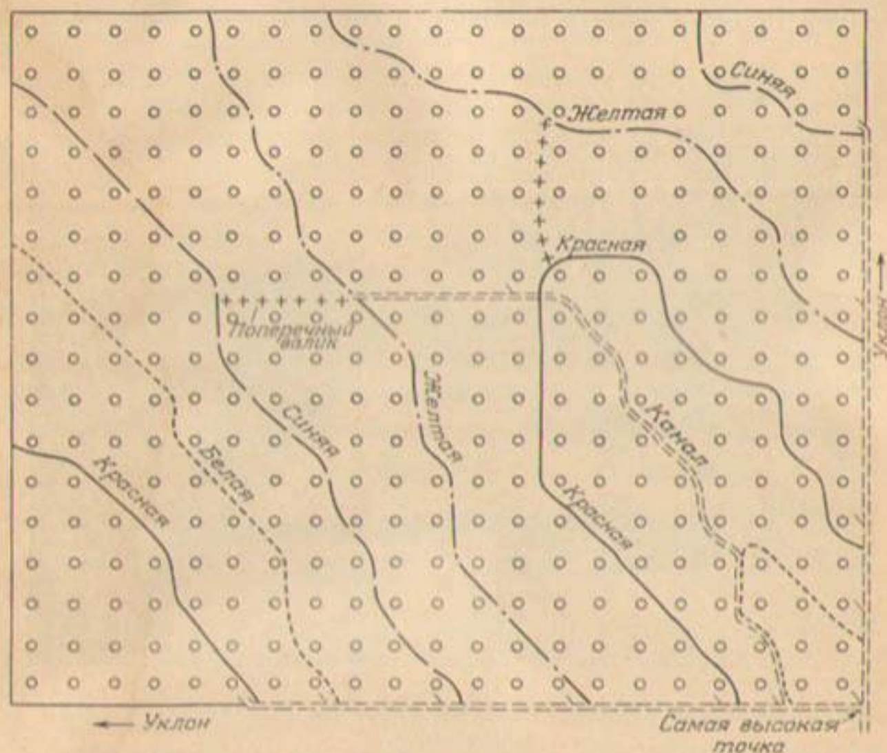
Рис. 174. План поливов фруктового сада затоплением чеков, расположенных по горизонталям на суглинистой почве, с расходом воды 3,4 \text{ м}^3/\text{мин} . На одной площадке посажено не более 40 деревьев. Горизонтالي рельефа отмечены на деревьях разным цветом — красным, белым, синим и желтым.
