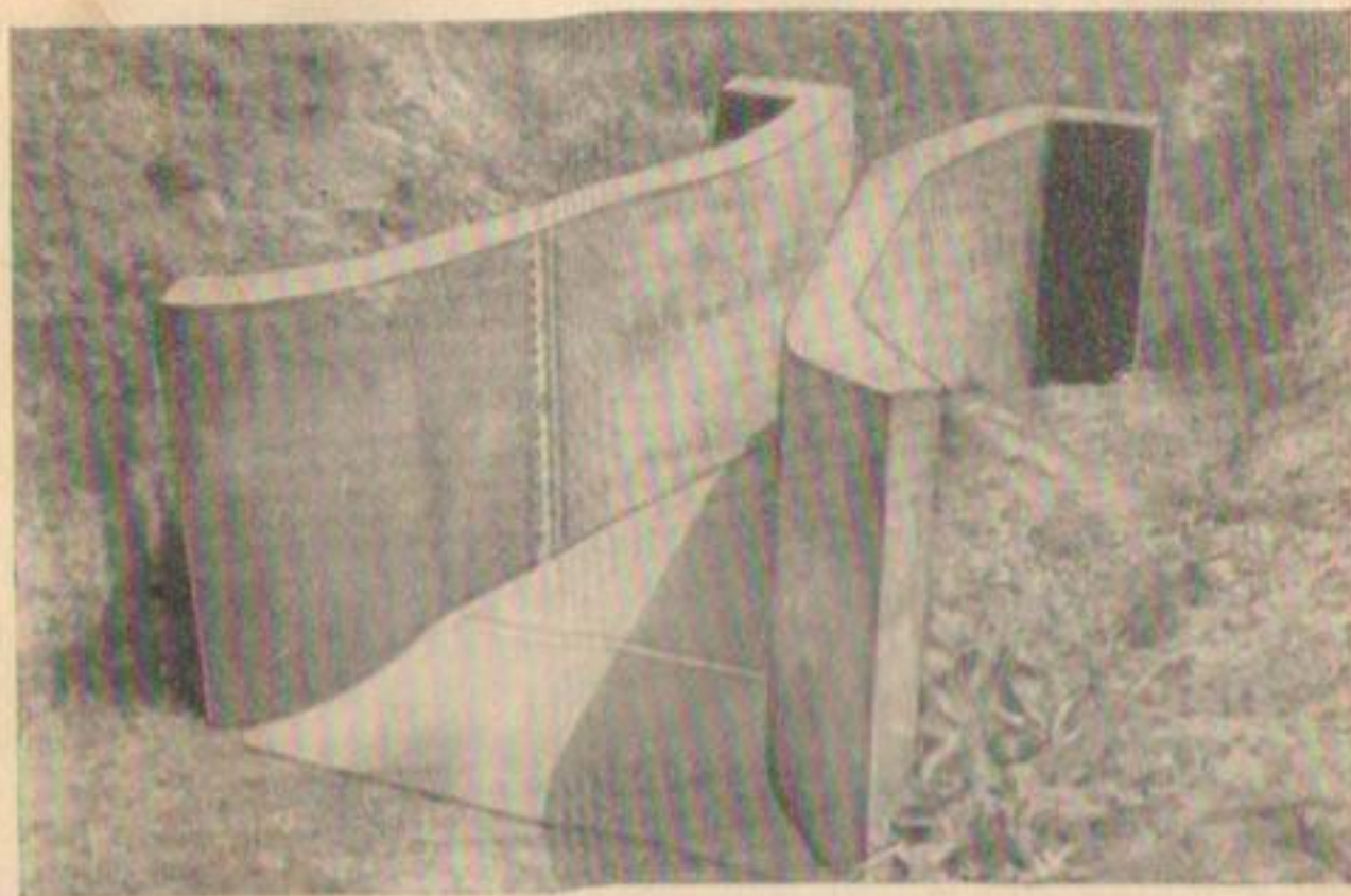
Р и с. 20. Девятидюймовый водомер Паршалла с измерительной рейкой. Стальной лист толщиной 1" у верхнего конца на пороге и у нижнего конца сооружения дает возможность точно установить дно на требуемом уровне.
