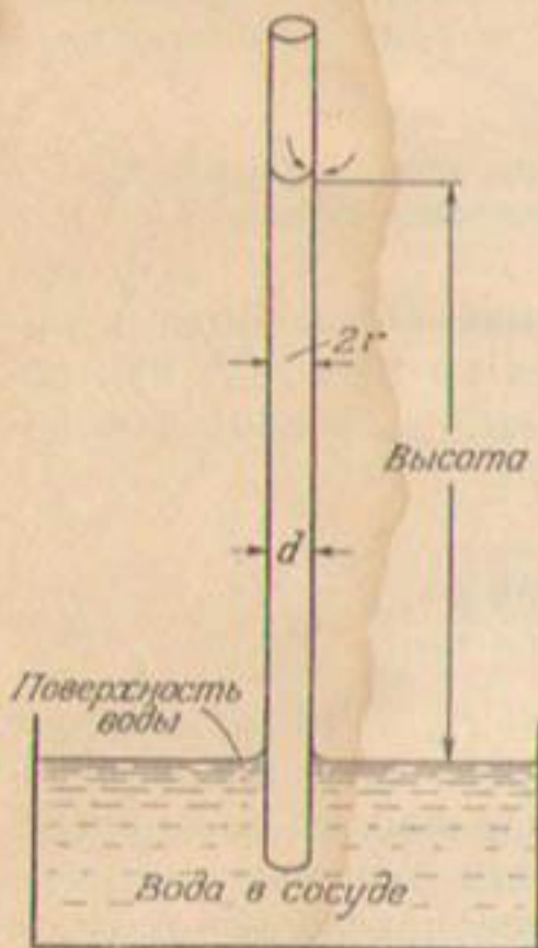
Рис. 104. Схема, показывающая подъем воды в капиллярной трубке над поверхностью воды в сосуде под действием поверхностного натяжения.
