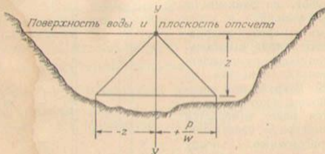
Рис. 126. Схема расположения области одинаковых гидравлических напоров (эквипотенциалей) в водоеме (в пруде или в озере). С увеличением глубины воды напор от высоты положения уменьшается в той же степени, с какой возрастает напор давления, вследствие чего сумма этих двух напоров постоянна.
