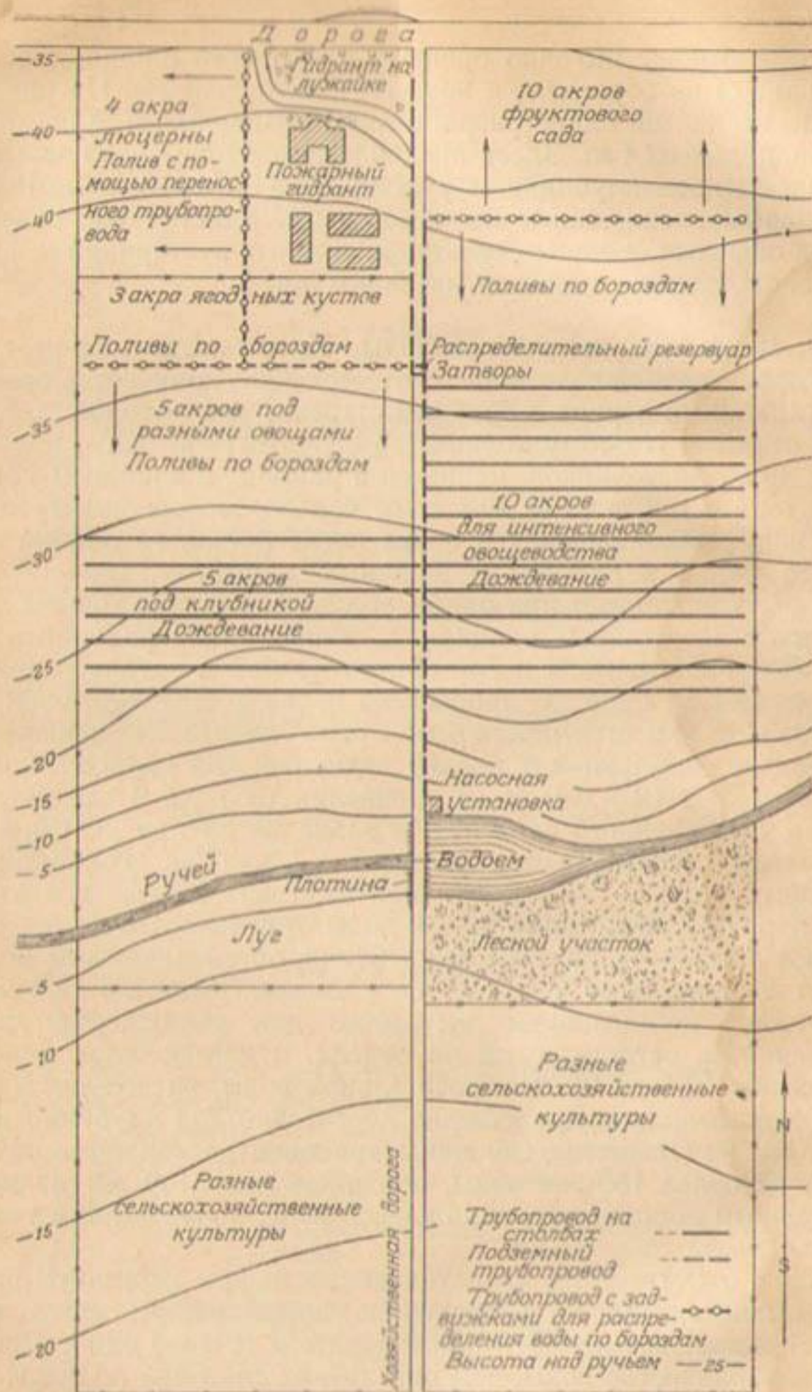
Р и с. 180. Типовой план фермерского хозяйства с площадью в 80 акров (32,4 га) в районах с влажным климатом. Оросительная вода подается насосом из водоема на участки и распределяется на них дождеванием или по бороздам.
