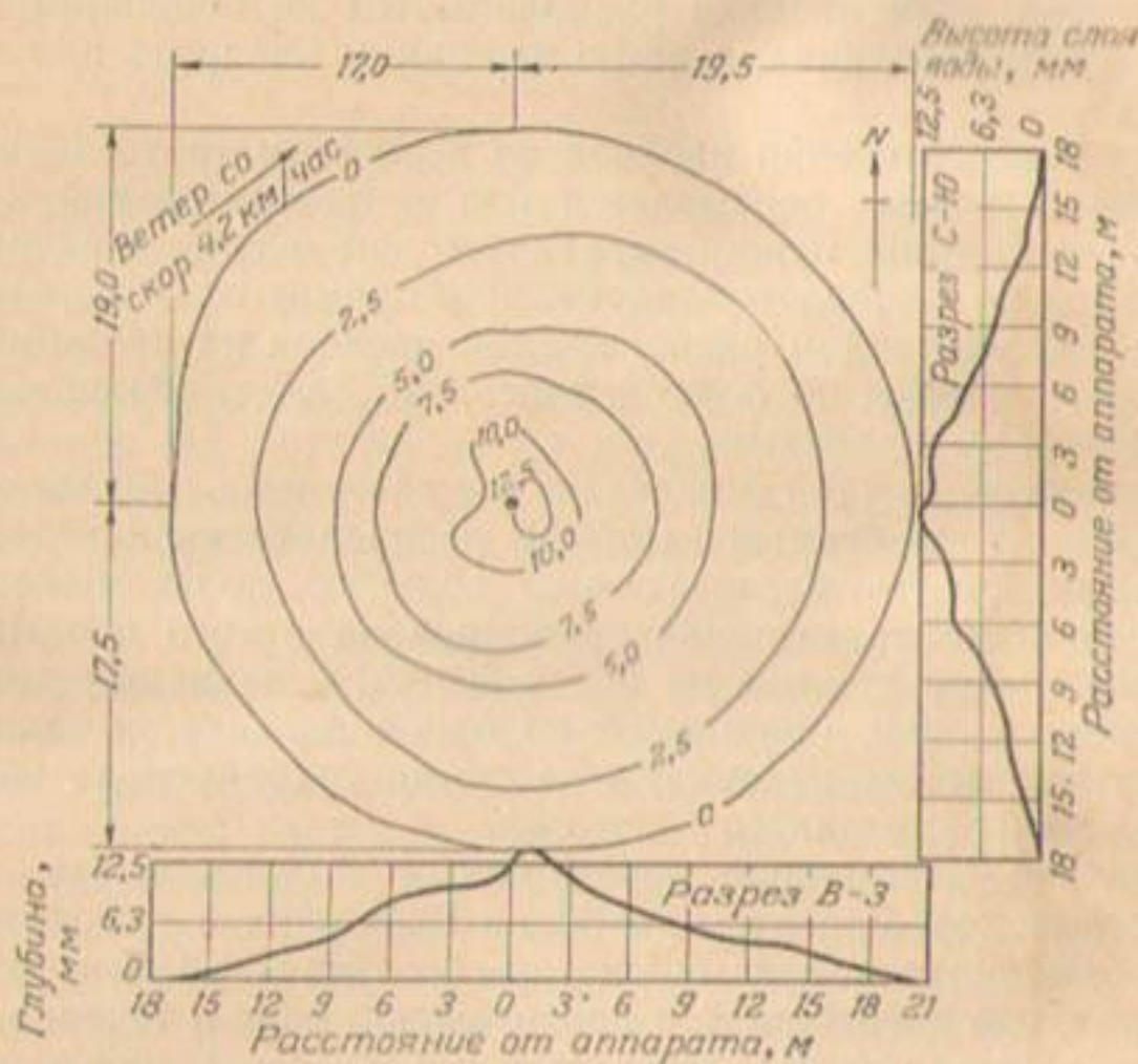
Рис. 83. Схема распределения воды дальноструйным дождевальным аппаратом (марки С-3): диаметры сопел — 6,3 мм и 5,6 мм; напор — 2,8 \text{ кг/см}^2 , расход — 75 \text{ л/мин} .
