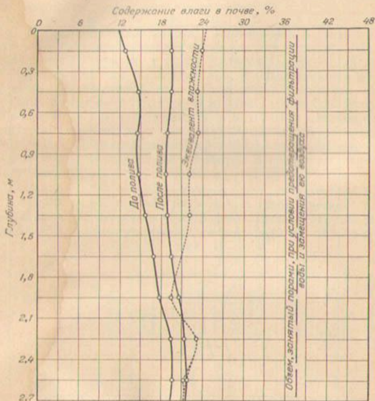
Рис. 114. Графики, показывающие содержание воды до и после полива, эквивалент влажности и объем пор в илисто-суглинистых почвах. Каждая кривая построена по средним значениям 87 проб.
