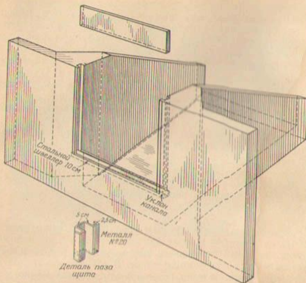
Р и с. 94. Бетонный регулятор с деревянным узким щитом.
