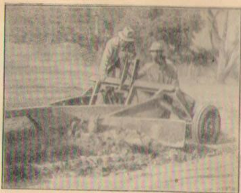
Р и с. 88. Моторизованный канавкопатель для рытья и отделки канала перед его облицовкой.
