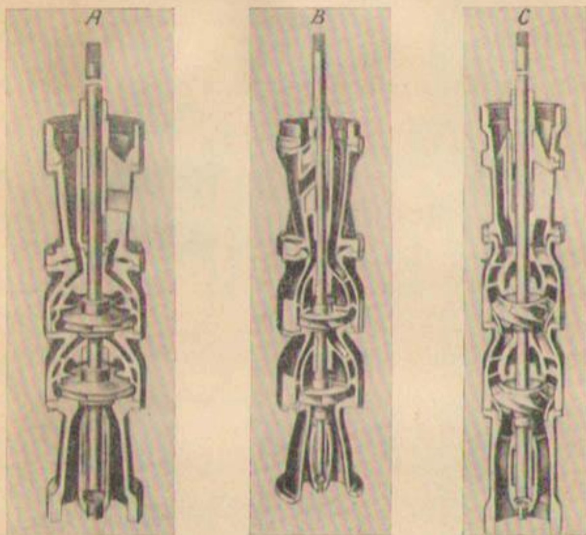
Рис. 56. Разрезы глубоководных двухступенчатых турбинных насосов.
