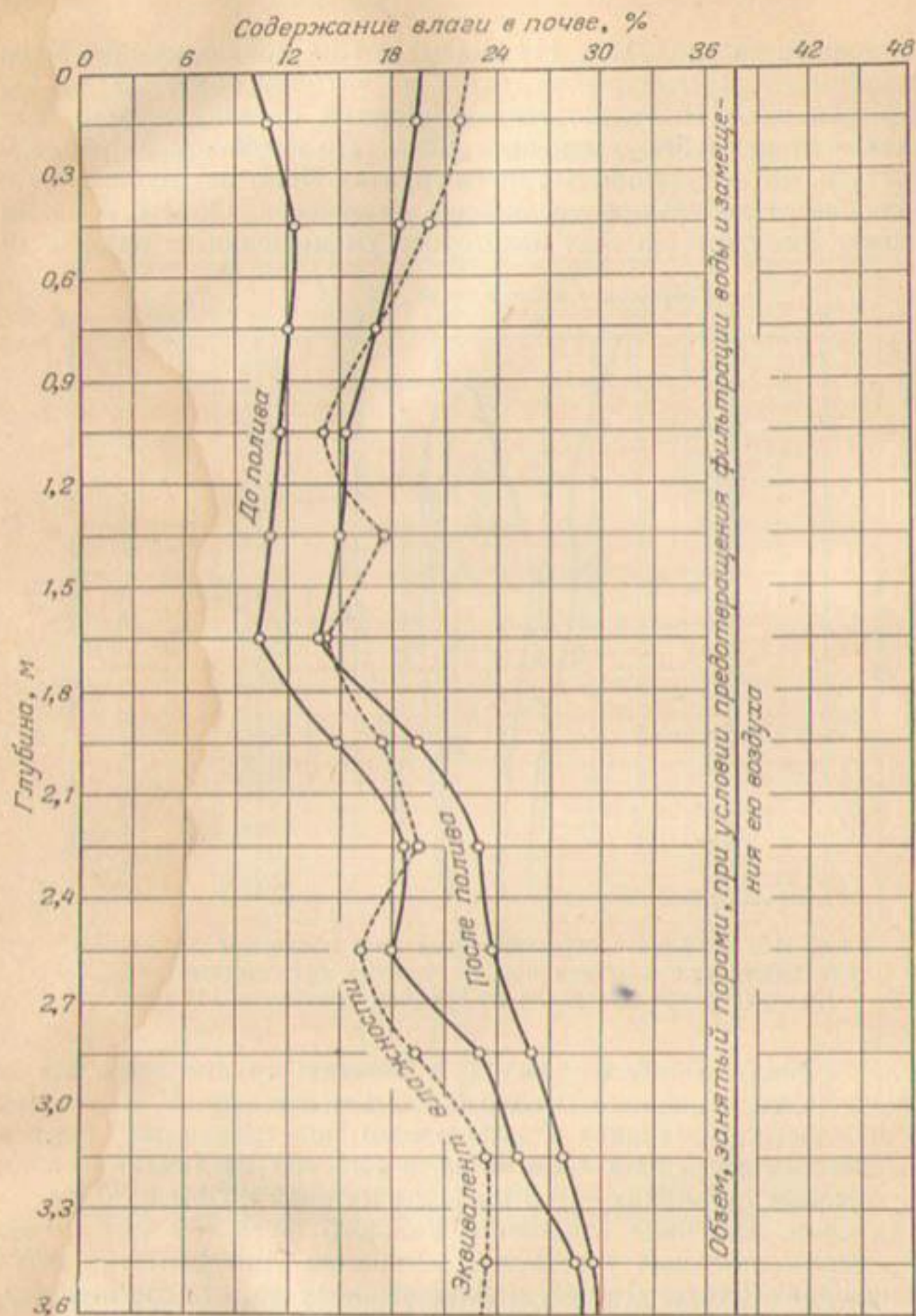
Рис. 116. Графики, показывающие содержание воды и объем пор в суглинистых почвах Йоло. Каждая кривая построена по средним значениям для 6 участков за 3 года, а также по средним значениям 147 проб.
