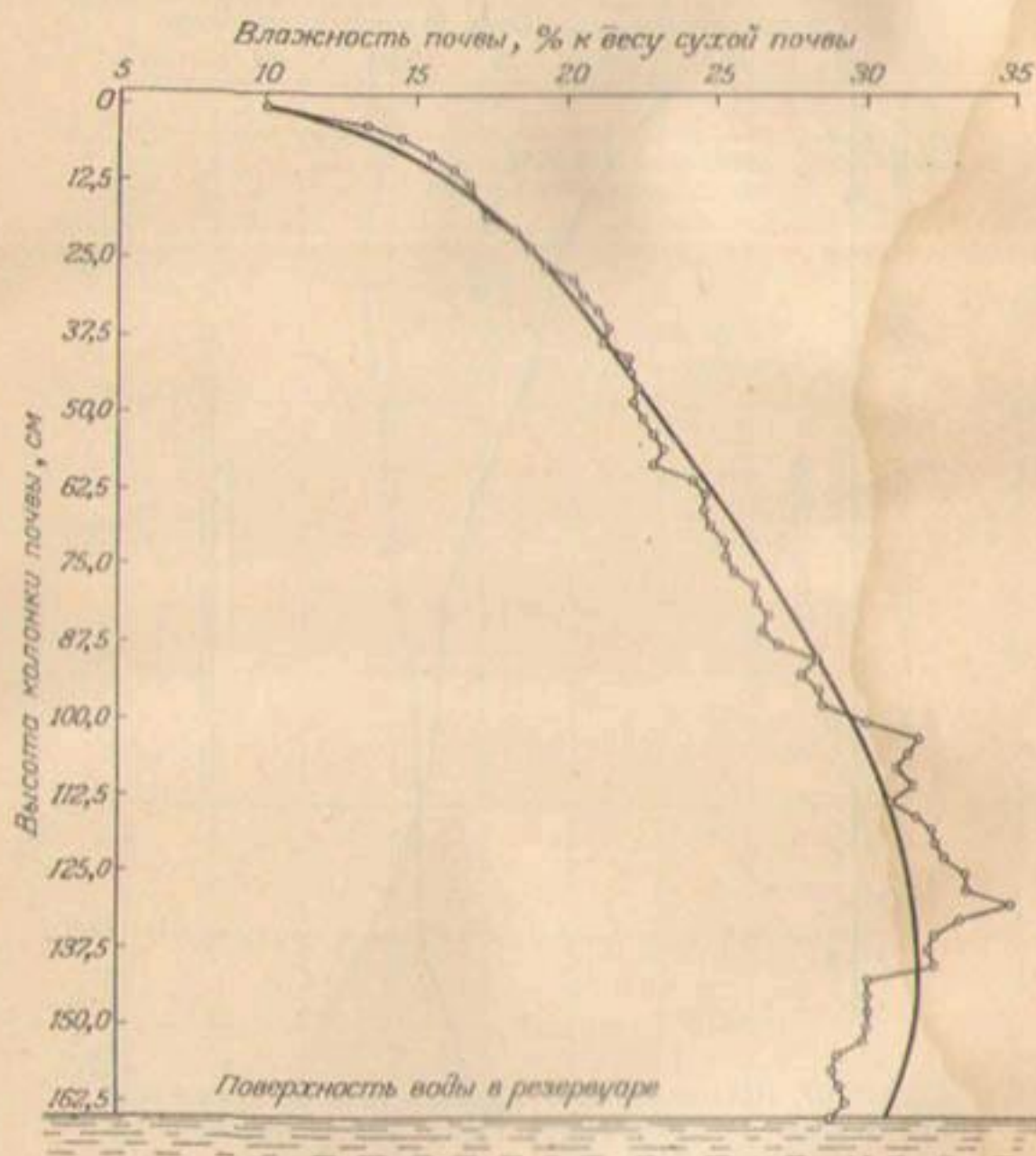
Рис. 106. Распределение капиллярной воды в вертикальной колонке вулканической почвы после 46 дней соприкосновения с водой в резервуаре.
