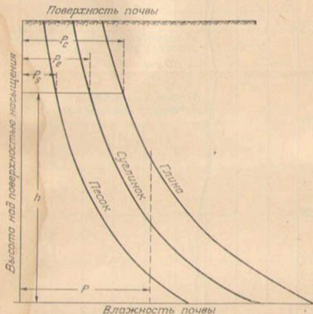
Рис. 109. Кривые, показывающие вероятное распределение капиллярной влаги в почвах различного механического состава в состоянии равновесия.
