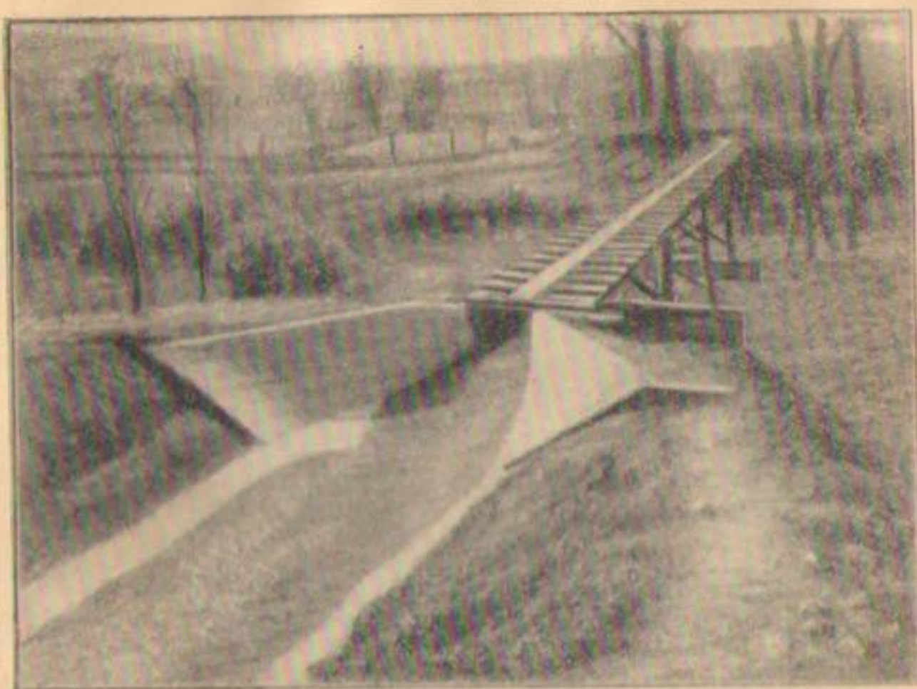
Р и с. 42. Небольшой акведук над оврагом, давший возможность спрямить канал и уменьшить его длину на 500 м.
