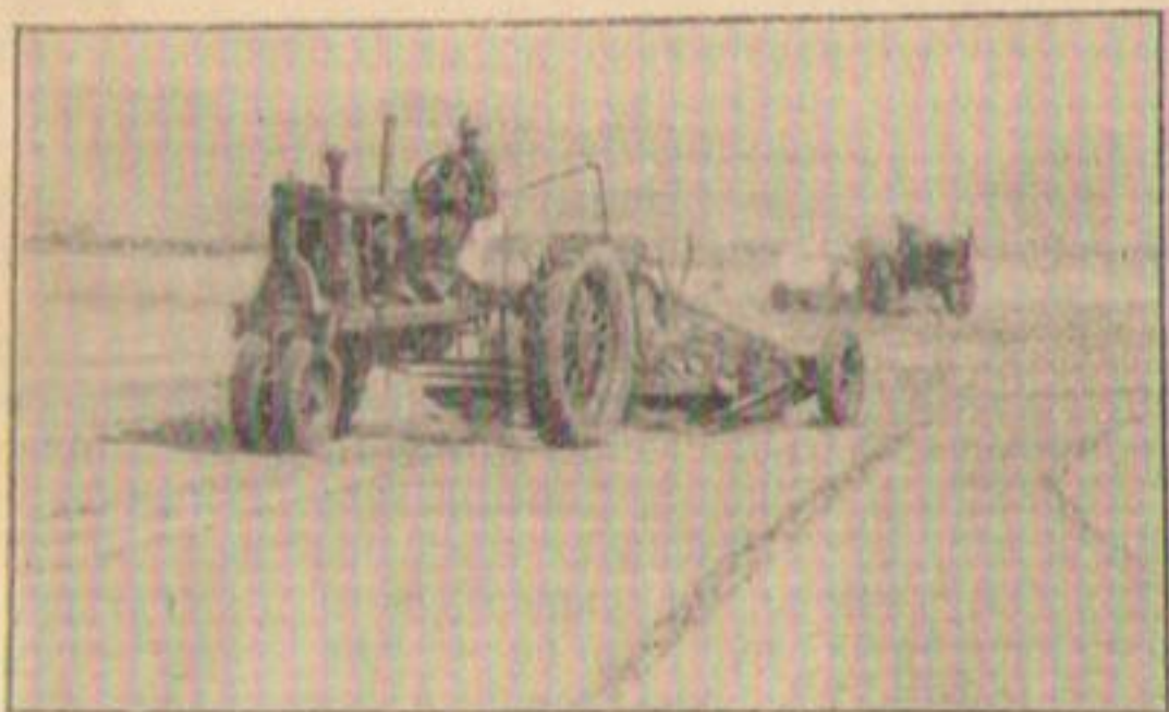
Р и с. 85. Планировщик марки Фресно на резиновых шинах, перемещающий снятый грунт на большое расстояние. Окончательная планировка производится волокушей.
