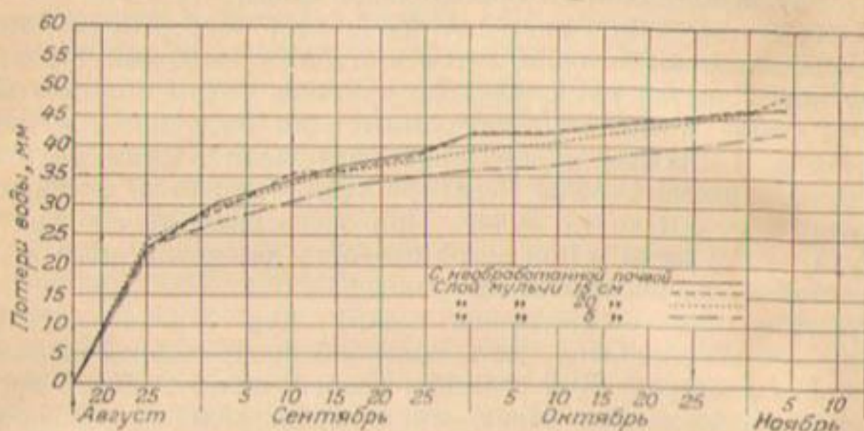
Р и с. 158. Потери воды на испарение с открытой поверхности почвы в сосудах.
