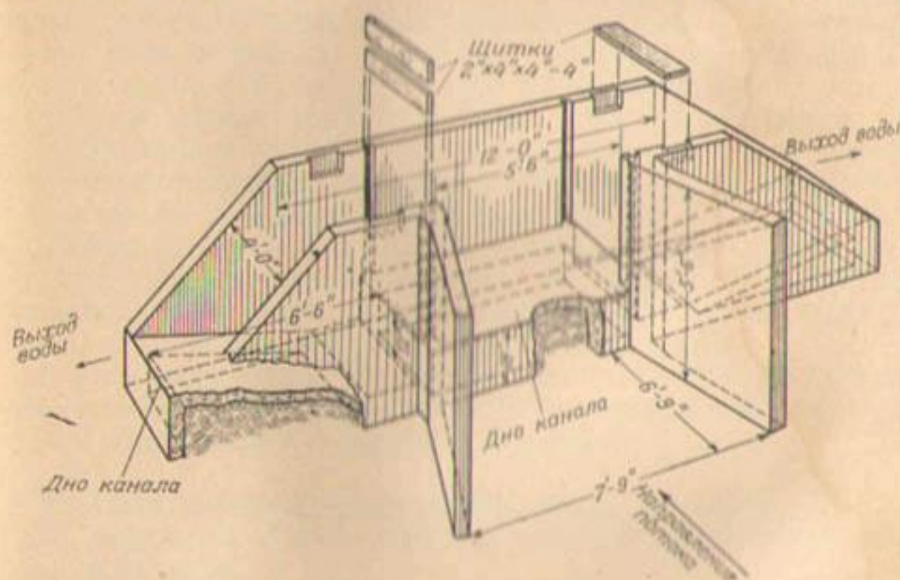
Р и с. 28. Бетонный ящик-вододелитель.
