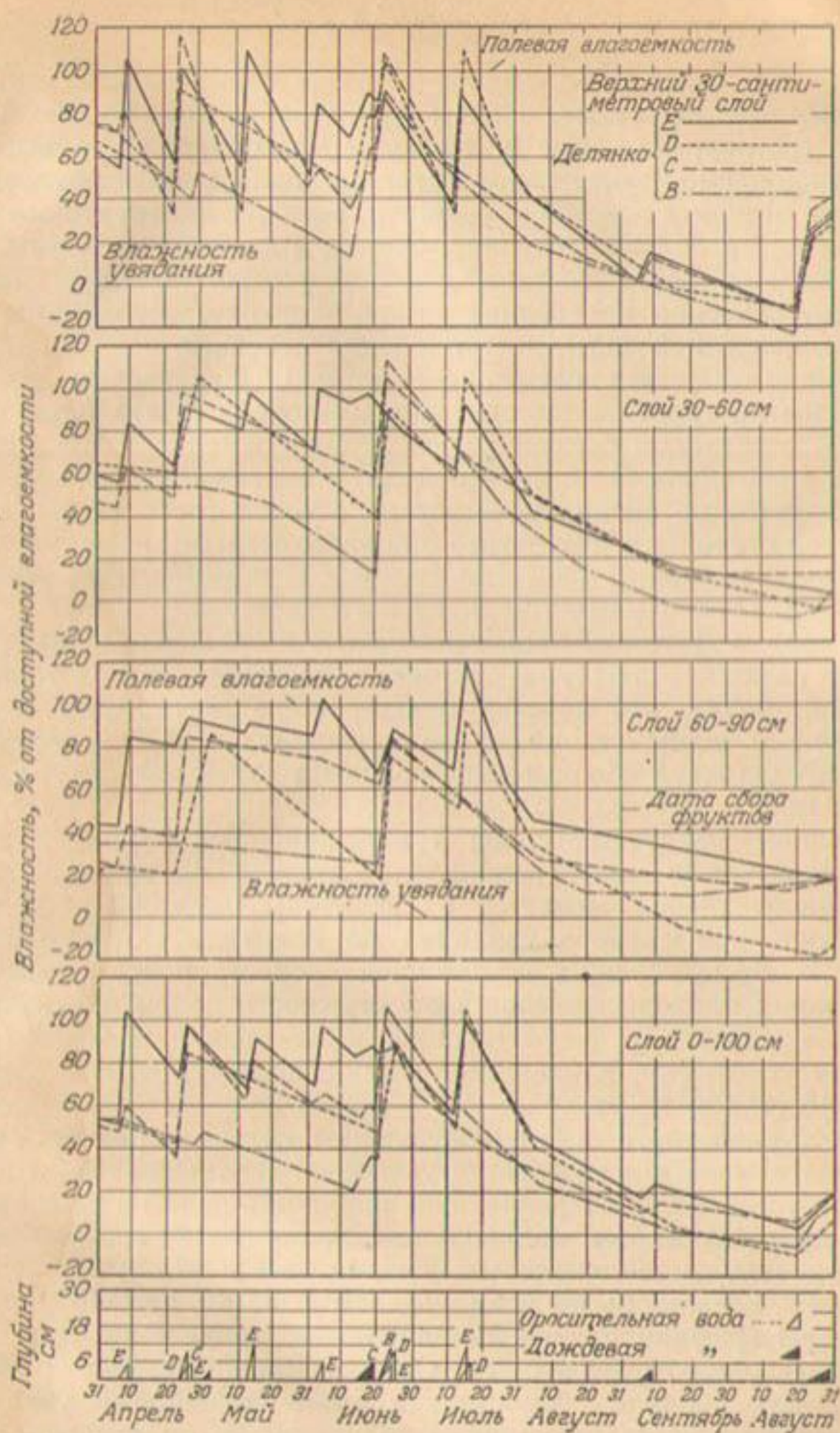
Р и с. 175. Графики почвенной влажности в процентах от доступной влагоемкости почвы в каждом из трех верхних слоев по 30 см, а также средняя влажность в верхнем 30-сантиметровом слое почвы. Показаны количества осадков и оросительной воды, использованной для полива фруктового сада. Вершины углов соответствуют глубине слоя оросительной или дождевой воды, поступившей на поле. Внизу показаны периоды поливов.
