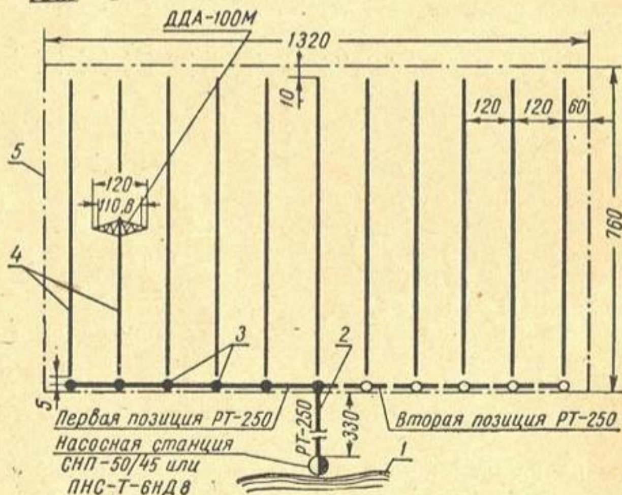
Рис. 10. Схемы орошения участков с помощью дождевального агрегата ДДА-100М:
