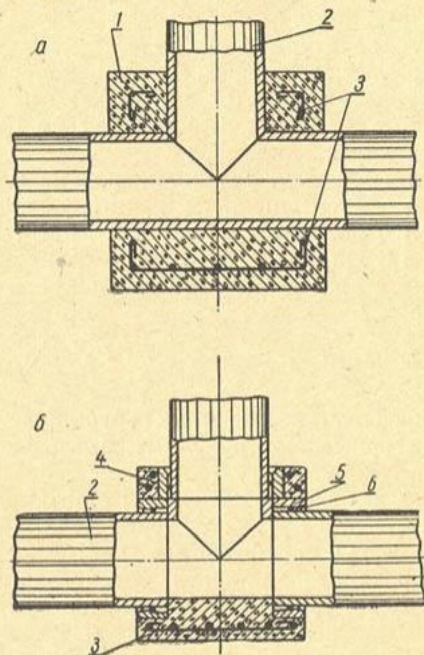
Рис. 54. Железобетонный тройник: а — монолитный; б — сборный; 1 — монолитная железобетонная тумба; 2 — асбестоцементная труба; 3 — стержневая арматура; 4 — сборная железобетонная фасонная часть; 5 — асбестоцементная полумуфта; 6 — уплотняющее резиновое кольцо.
