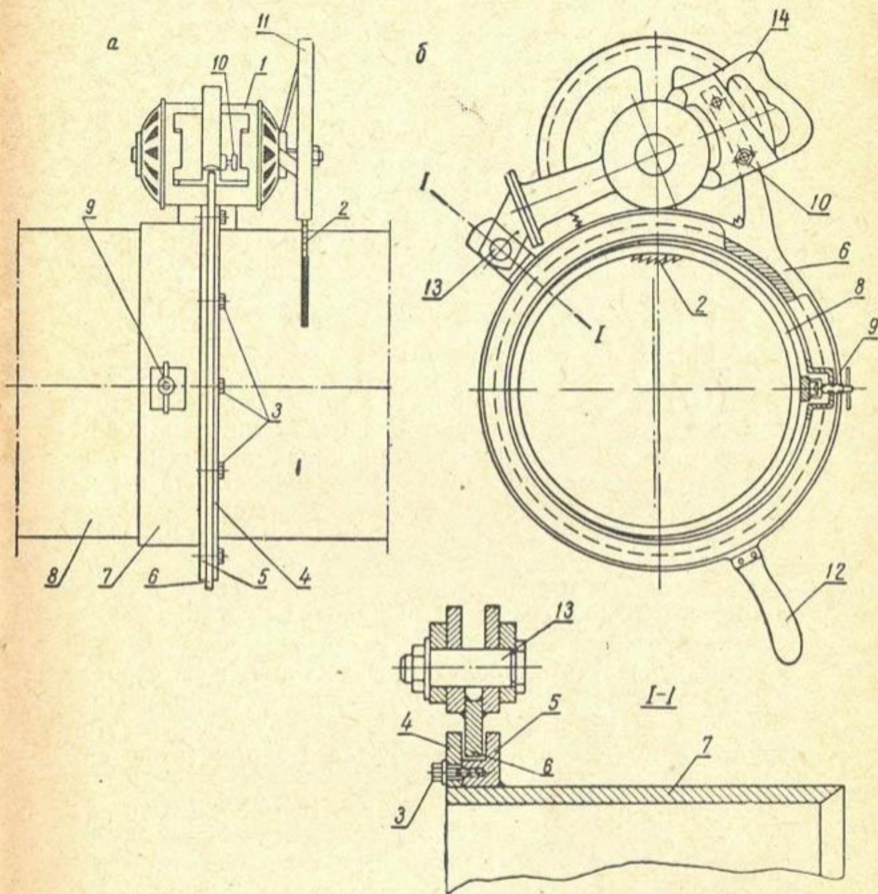
Рис. 17. Схема установки для резки полиэтиленовых труб: а — общий вид; б — вид с торца трубы (рабочее положение); 1 — электродвигатель; 2 — циркулярная пила; 3 — болты; 4, 5 — кольца; 6 — диск; 7 — патрубок; 8 — полиэтиленовая труба; 9 — винтовой упор; 10 — стопор; 11 — кожух для пилы; 12, 14 — ручки; 13 — шарнир.
