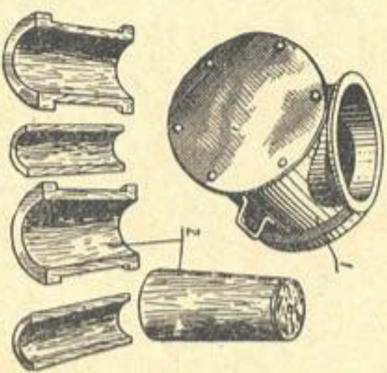
Рис. 55. Разборная опалубка: 1 — металлическая разъемная форма; 2 — деревянный сердечник.
