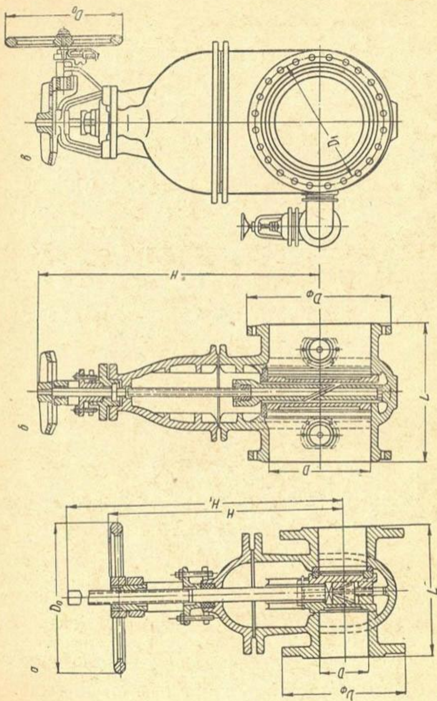
Рис. 56. Параллельные чугунные задвижки: а — с выдвижным шпинделем; б — с неподвижным шпинделем; в — с ободом и зубчатой передачей.
