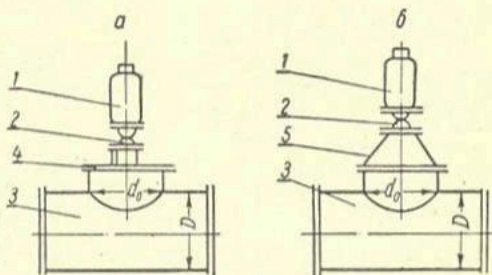
Рис. 58. Схема установки вантузов на подземных трубопроводах:
