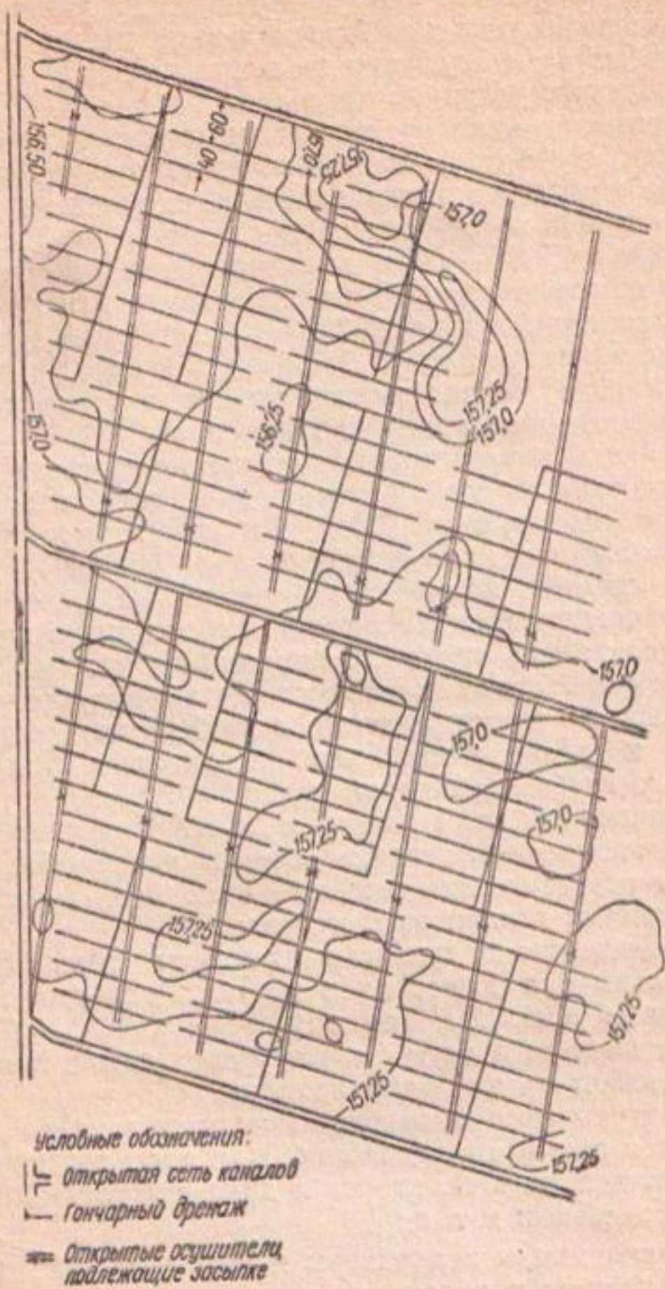
Рис. 2 Схема переустройства открытой сети на закрытый дренаж.
