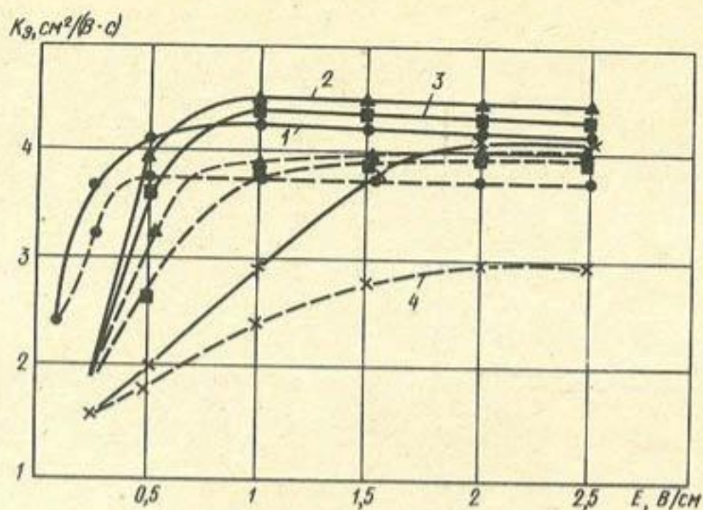
Зависимость коэффициента электроосмоса K_3 от градиента напряжения электрического поля E постоянного и пульсирующего токов для глин различного состава 1 — каолинитовая глина; 2 — гидрослюдистая глина; 3 — монтмориллонитовая глина; 4 — гидрослюдисто-каолинитовая глина; — при наложении поля постоянного тока; - - - при наложении поля пульсирующего тока
