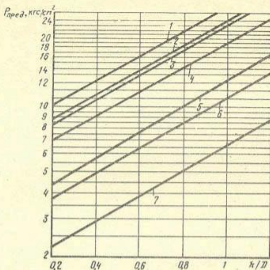
Рис. 1. Зависимость предельной нагрузки P_{\text{пред}} от относительной высоты балластной призмы из материалов, укрепленных вяжущими
