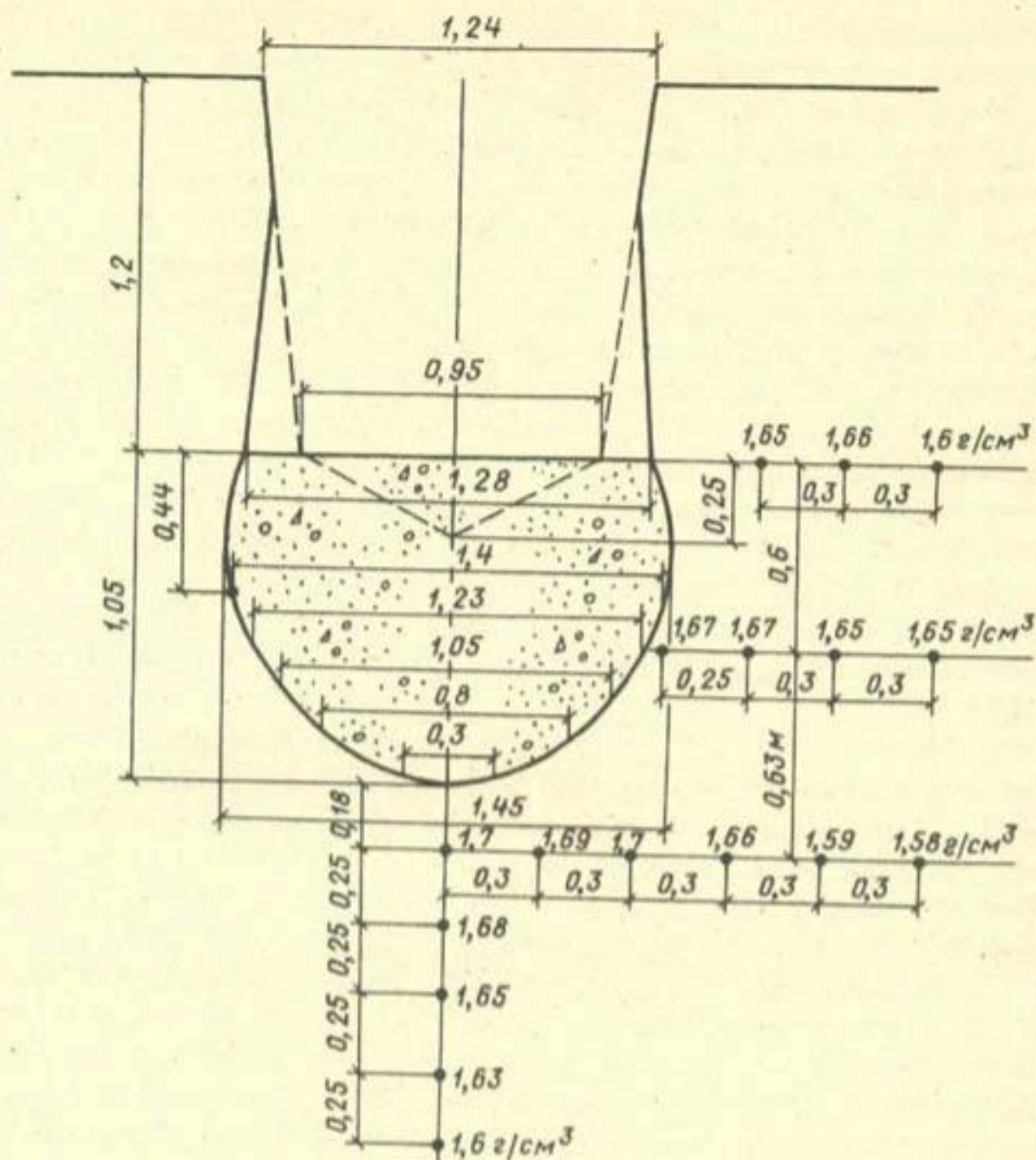
Поперечный разрез котлована № 4 с щебеночной подушкой и схема расположения проб грунтов по определению их объемной массы ( V_{\text{щебня}} = 1,5 \text{ м}^3 )
