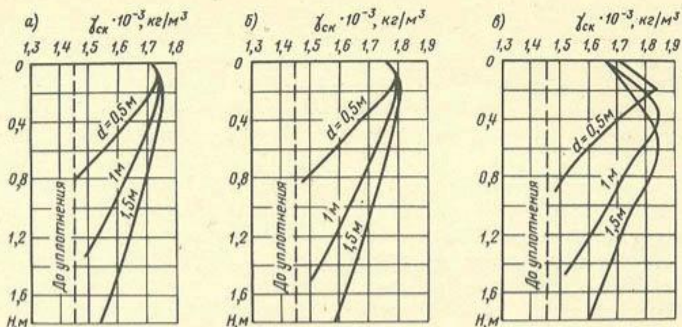
Рис. 2. Изменение плотности грунтов по глубине в зависимости от площади трамбовок и удельных импульсов
