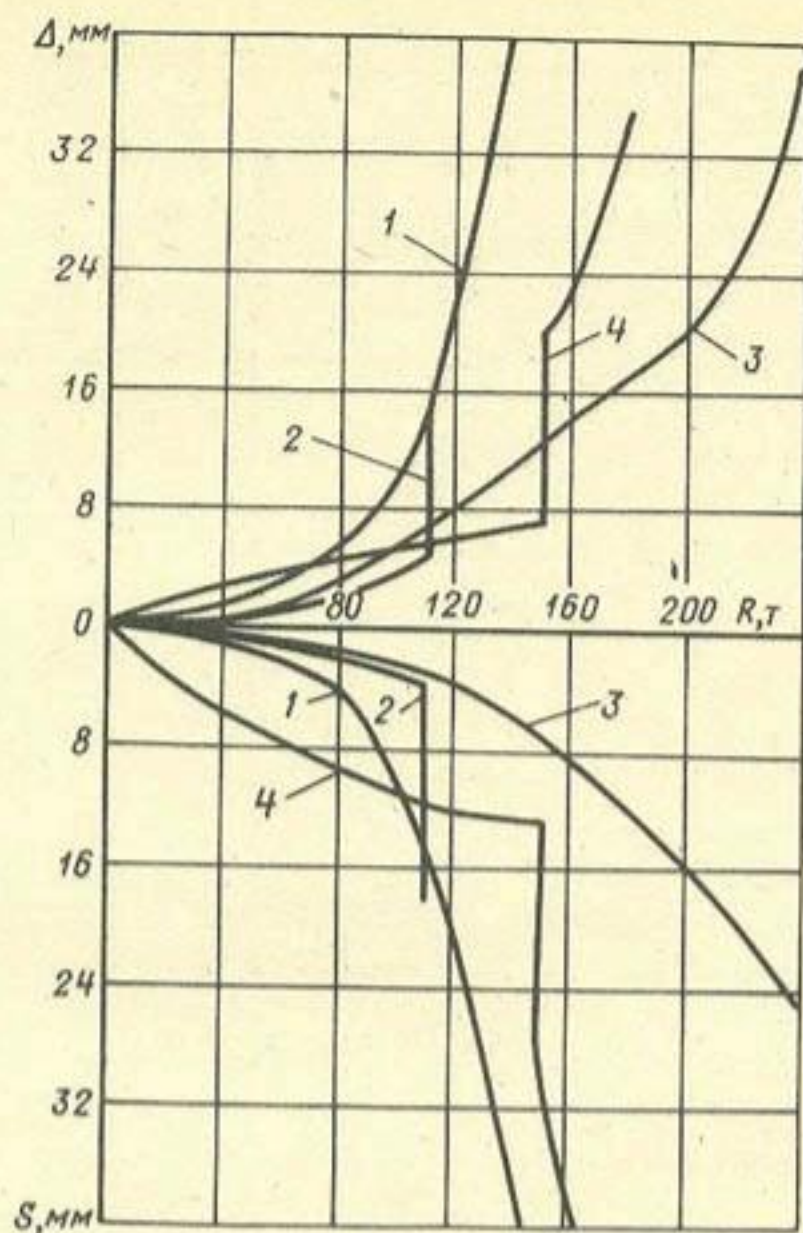
Рис. 2. Зависимость вертикальных и горизонтальных перемещений от наклонной нагрузки R 1 - сваи № 13-16; 2 - сваи № 5-8; 3 - сваи № 29-32; 4 - сваи № 21-24
