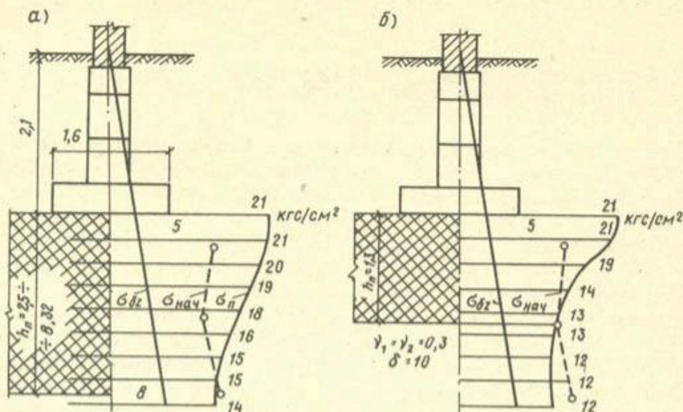
Схемы к расчету глубины уплотнения основания по моделям а — однородной среды; б — двухслойной среды
