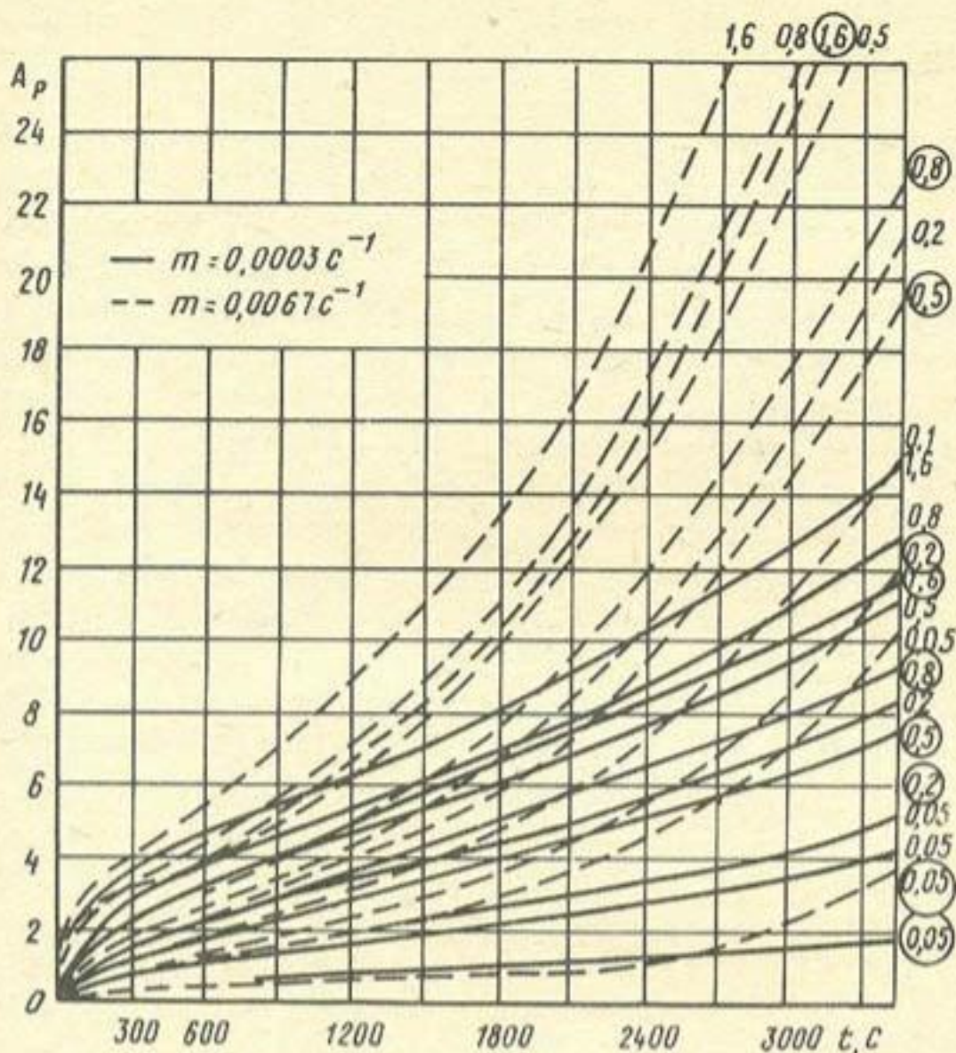
Рис. 2. Номограмма для определения значения A_p при различных грунтах, режимах инъекции и радиусах скважин r_o (в кружках даны значения W , мм/с, при r_o = 60 мм, без кружков — значения W при r_o = 20 мм)
