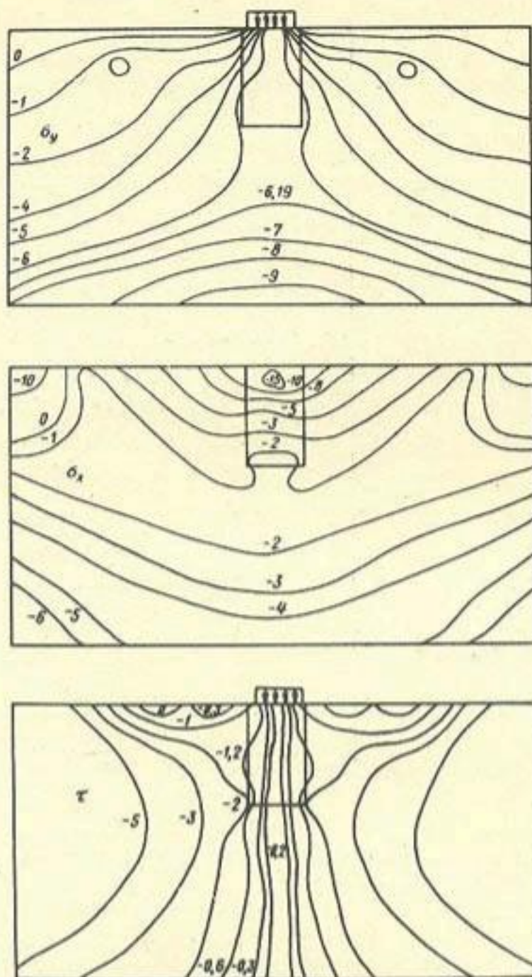
Линии равных напряжений: изобары \sigma_y ; распоры \sigma_x ; сдвиги \tau
