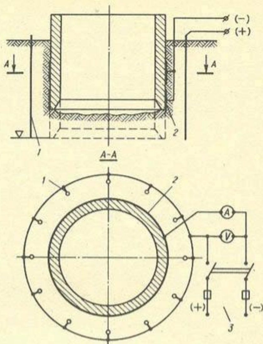
Схема размещения электродов
