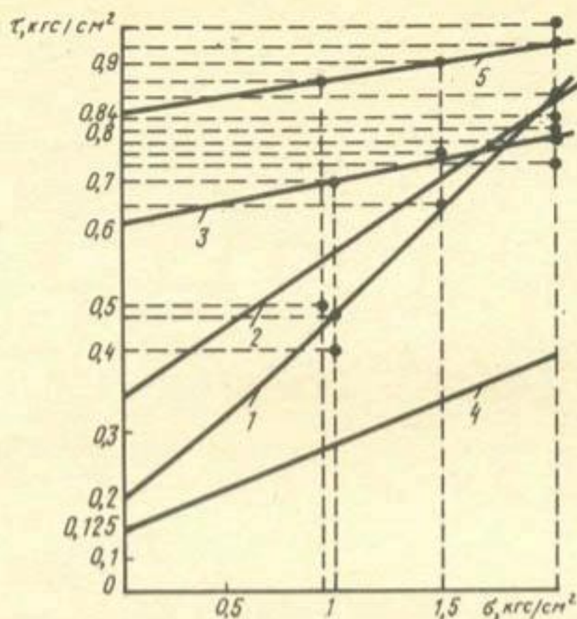
Рис. 2. Испытания грунтов на сдвиг 1 — незакрепленный грунт нарушенной структуры; 2 — закрепленный грунт нарушенной структуры через 7 дней; 3 — то же, через 28 дней; 4 — незакрепленный грунт природного сложения; 5 — закрепленный грунт в полевых условиях
