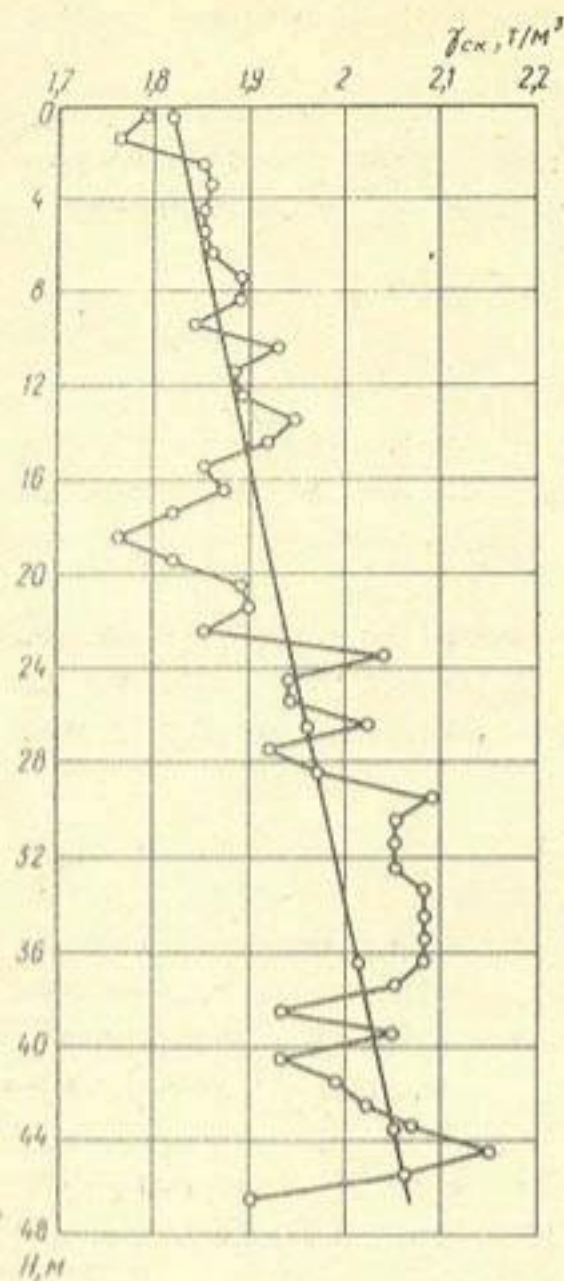
Рис. 1. Изменение объемной массы грунта по глубине опытной взрывонабросной плотины на р. Бурлык
