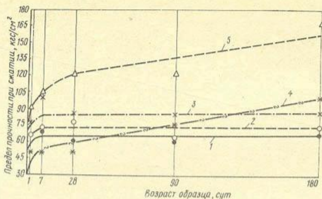
Рис. 1. Зависимость предела прочности при сжатии образцов песка, мела, глины от влияния среды 1 – песок в среде с pH = 1,1 ; 2 – песок в среде с pH = 11 ; 3 – песок в воде; 4 – мел в воде; 5 – глина в воде
