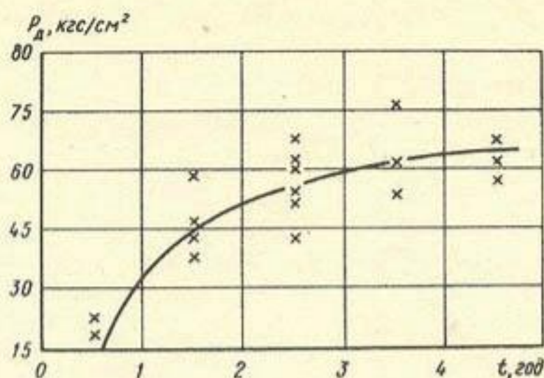
Рис. 1. Характер изменения сопротивления динамическому зондированию
