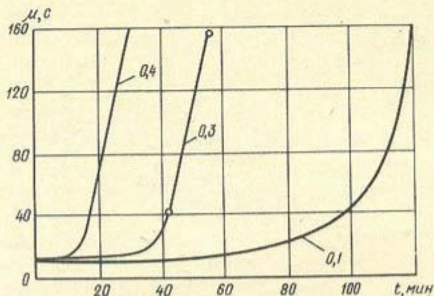
Рис. 1. Изменение вязкости \mu во времени для закрепляющей смеси на основе концентрированной ФРЭС (ФРЭС:Ф:ЕН) = 1:0,7:Х при добавлении различных количеств едкого натра в объемных отношениях (температура среды 18°C)
