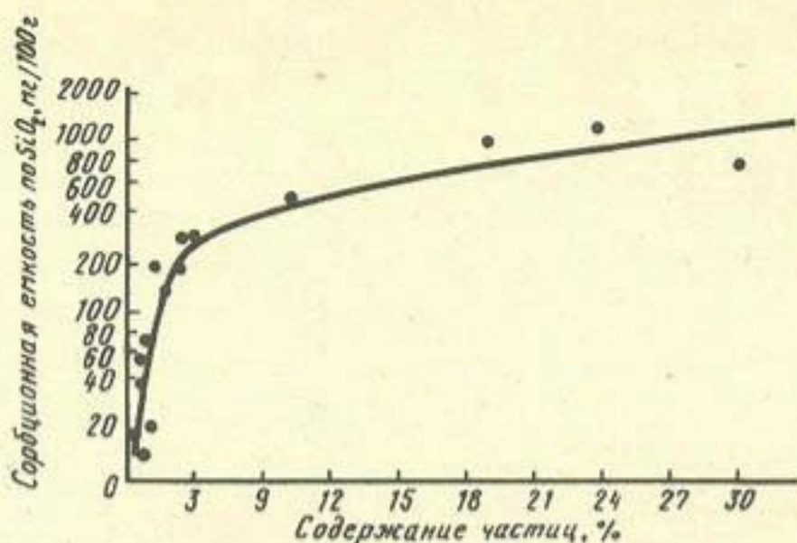
Зависимость сорбции \text{SiO}_2 от содержания частиц размером < 0,01 мм
