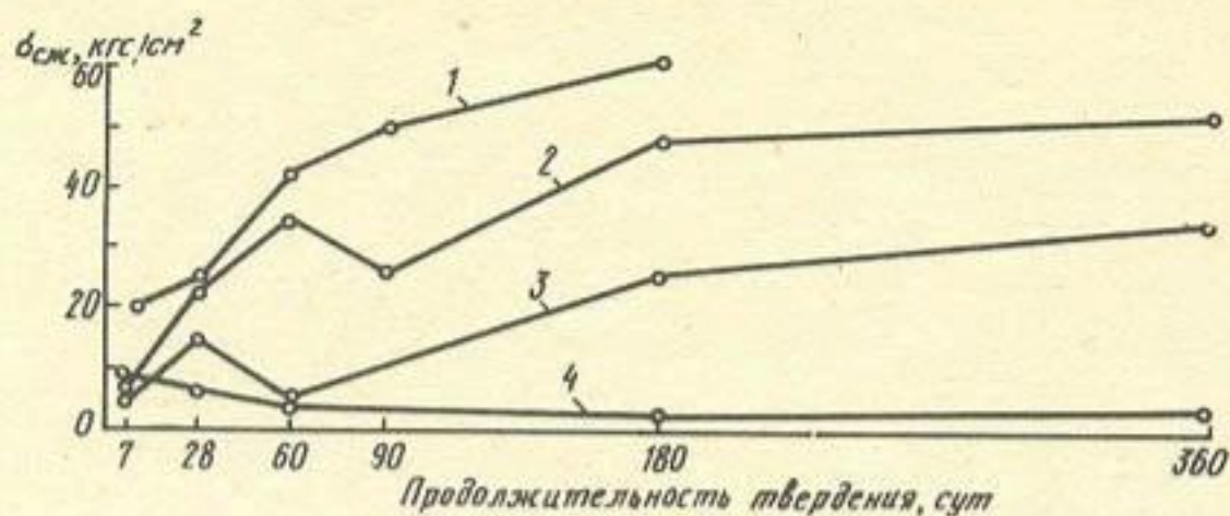
Рис. 1. Изменение прочности исследуемых зологрунтов во времени
