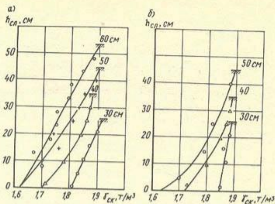
Рис. 1. Изменение плотности грунта по глубине при укатке автоскрепером за четыре прохода (а), и за шесть проходов (б). Цифрами на кривых обозначена исходная толщина слоя
