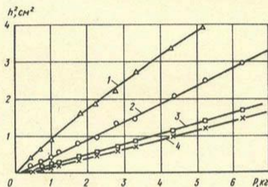
Рис. 2. Изменение удельного сопротивления пенетрации намытого песчаного грунта в зависимости от его возраста 1 — свеженамытый грунт; 2 — t = 1,5 г; 3 — t = 3,5 г.; 4 — t = 4 г.
