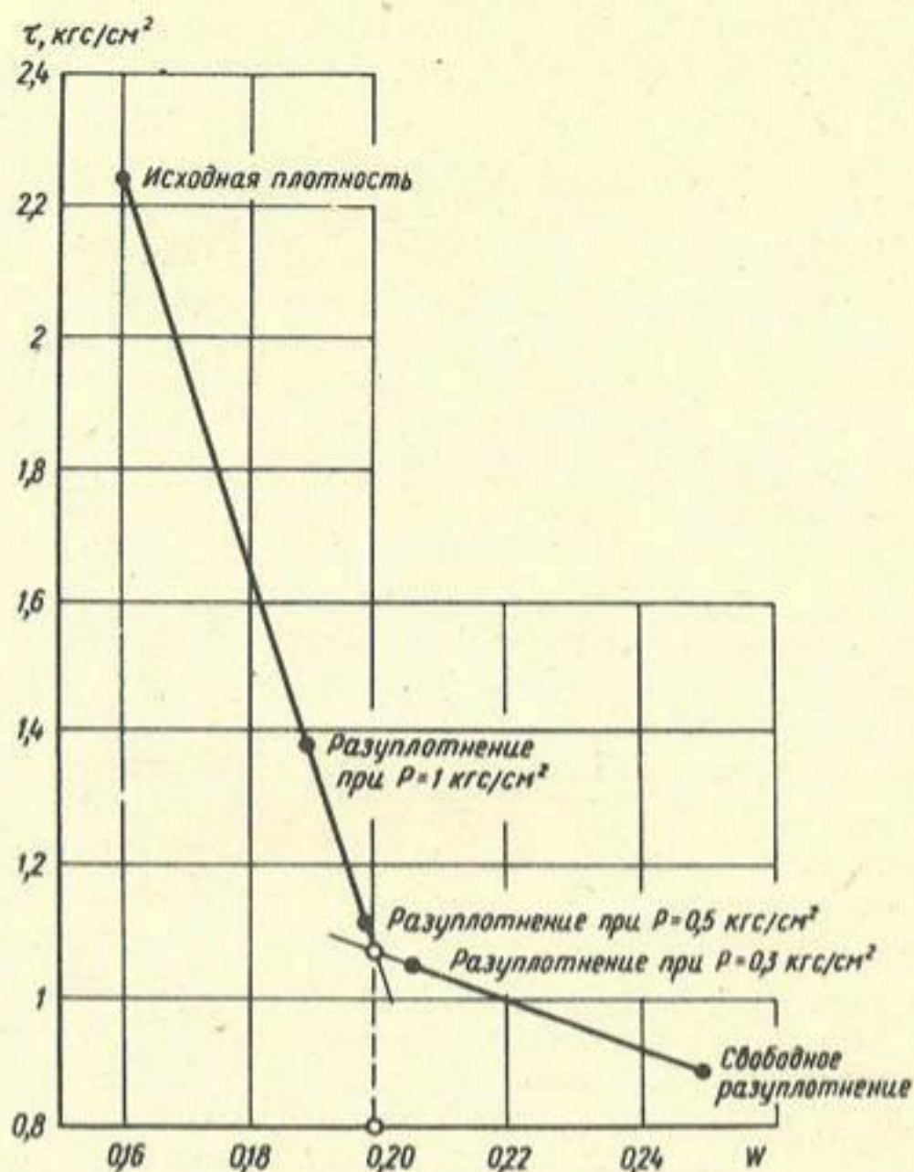
Рис. 2. Изменение сдвигающих усилий в зависимости от степени влажности при разуплотнении
