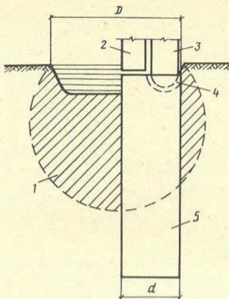
Рис. 1 Конструктивная схема короткой буронабивной сваи с уплотненным ядром
