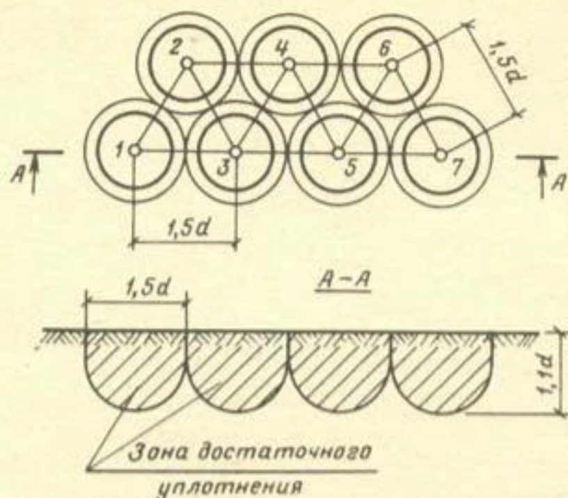
Технологическая схема прерывистого поверхностного уплотнения
