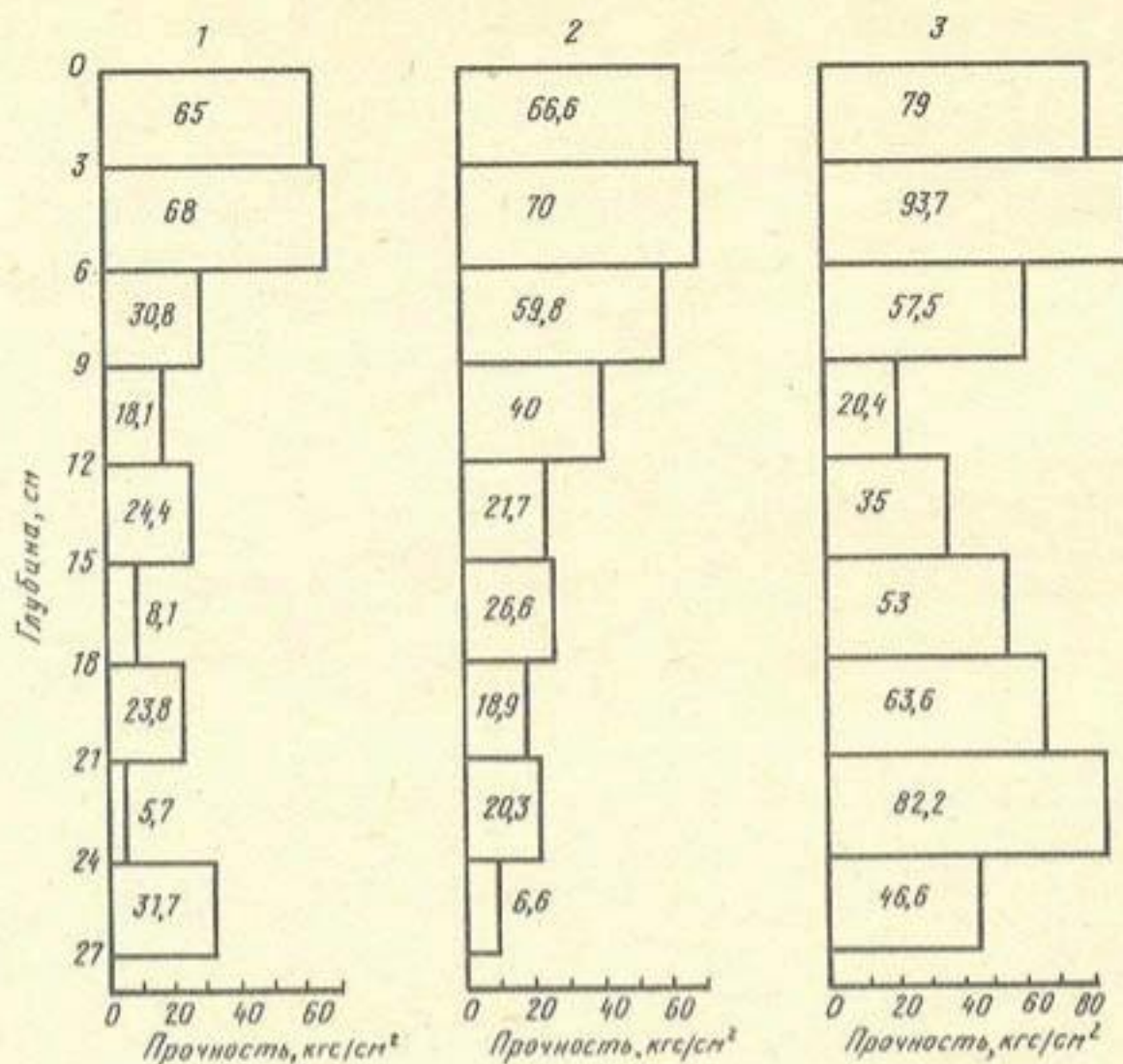
Прочность цилиндрических образцов по высоте при пропитке сверху 1, 2, 3 – номера образцов
