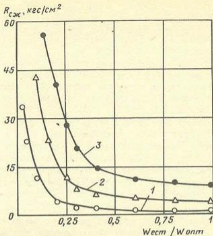
Рис. 1. Зависимость предела прочности R_{сж} при сжатии образцов укрепленного грунта от его относительной влажности W_{ест}/W_{опт} 1 - песок; 2 - суглинок легкий пылеватый; 3 - суглинок тяжелый
