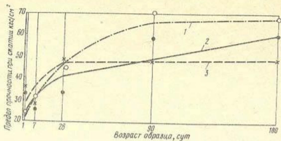
Рис. 2. Зависимость предела прочности при сжатии образцов грунта с опытного участка ИнгуриГЭС от влияния среды
