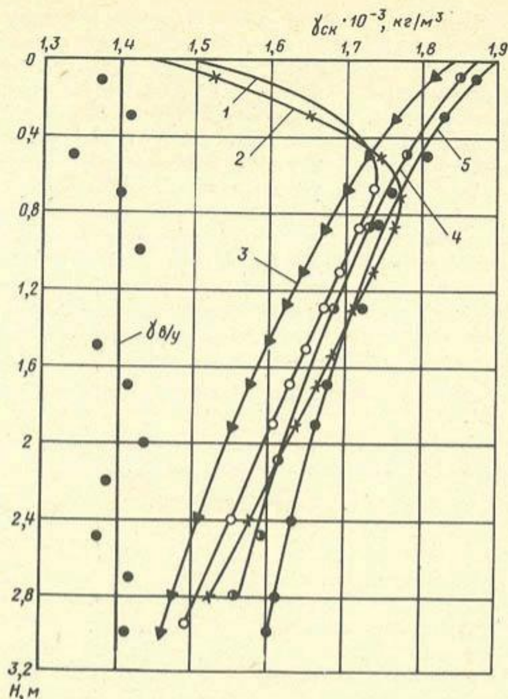
Рис. 1. Зависимость качества уплотнения \gamma_{ск} от сохранения удельного импульса i_{уд} в цикле заданного числа ударов ( n = 8 ) по одному следу 1 и 2 — i_{уд} = \text{const} ; 3–5 — i_{уд} \neq \text{const} ; \gamma_{ск} — плотность грунтов природного сложения (среднее значение по глубине)
