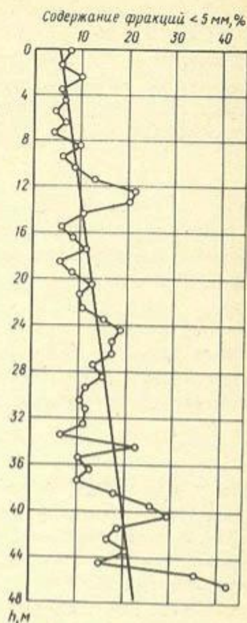
Рис. 2. Изменение содержания мелкозернистой фракции по глубине опытной взрывонабросной плотины на р. Бурлык
