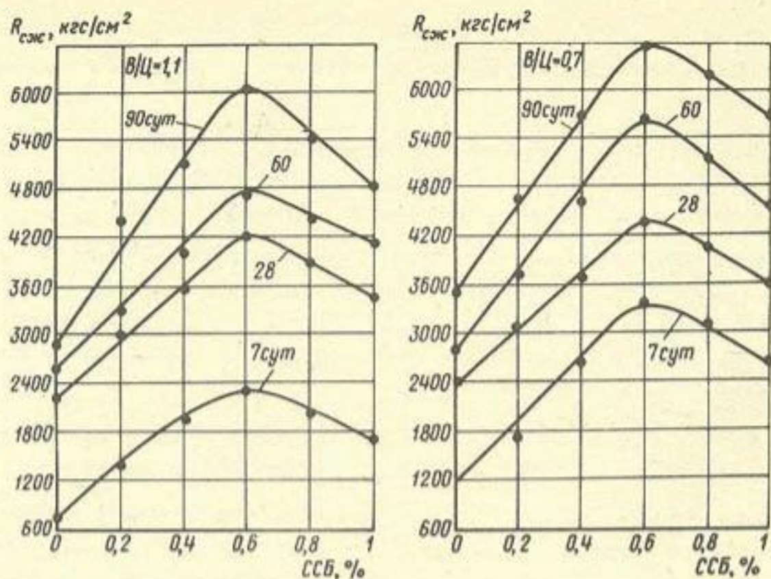
Зависимость прочностных характеристик от содержания ССБ в цементационном растворе при различном возрасте твердения
