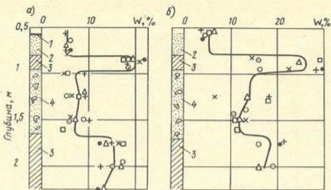
Рис. 1. Распределение влажности грунта W по глубине под гидроизоляционным покрытием (а) и за его пределами (б)
