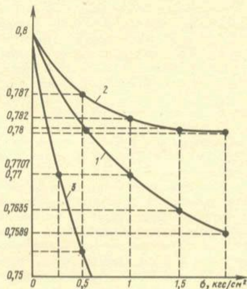
Рис. 1. Компрессионные испытания грунтов
