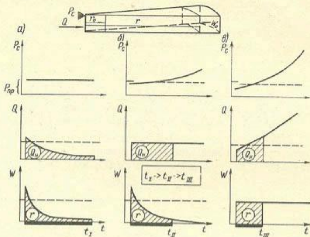
Рис. 1. Характер изменения во времени параметров различных режимов нагнетания а — при постоянном давлении нагнетания p_c ; б — при постоянном расходе раствора Q ; в — при постоянной скорости распространения раствора W
