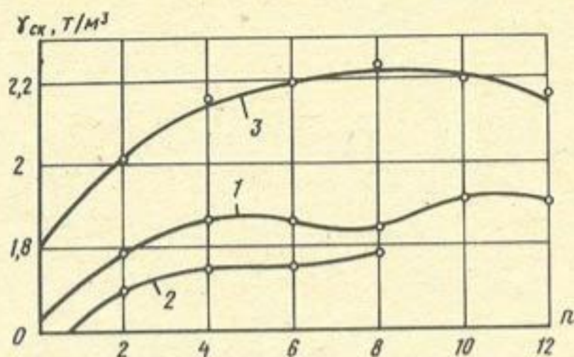
Рис. 2. Изменение плотности грунта \gamma_{ск} в зависимости от числа проходов катка n
