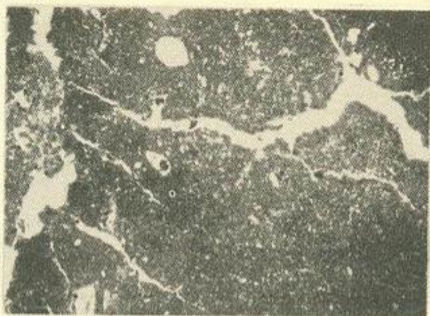
Рис. 1. Шлиф закрепленного силикатизацией лёсса (увеличено в 60 раз)
