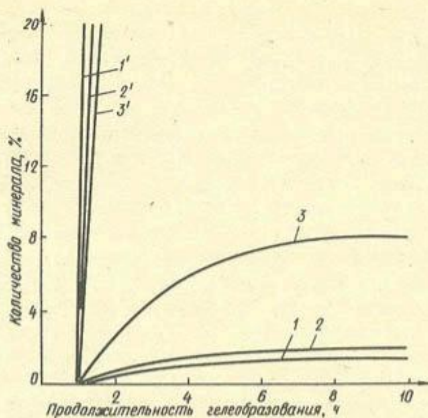
Рис. 1. Влияние глинистых минералов на гелеобразование карбамидной смолы 1, 2 и 3 — каолинит, монтмориллонит и нонтронит с содержанием карбонатов соответственно 3,8; 2 и 1,5%; 1', 2' и 3' — те же минералы, отмытые от карбонатов
