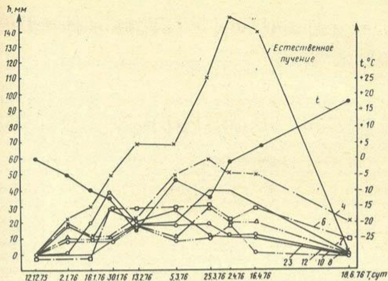
Рис. 2. Изменение величины пучения грунта катодной зоны во времени 2, 4, 6, 8, 10, 12, 23 — номера контрольных точек в зоне укрепленного грунта согласно схеме, показанной на рис. 1
