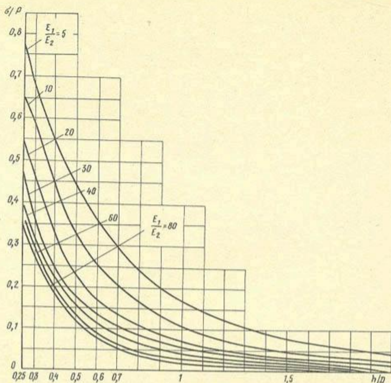
Рис. 2. Вертикальные напряжения на площадке земляного полотна при различных значениях E_1/E_2 или n/D
