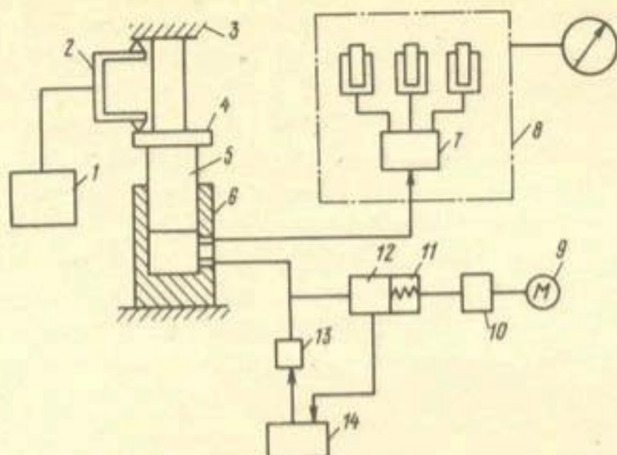
Автоматическая установка для исследования ползучести закрепленного грунта
