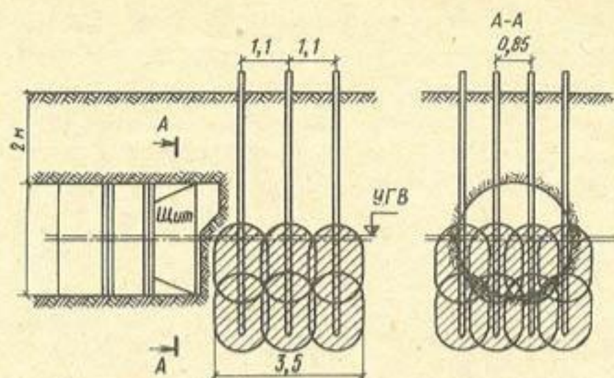
Рис. 2. Схема закрепления грунта с поверхности
