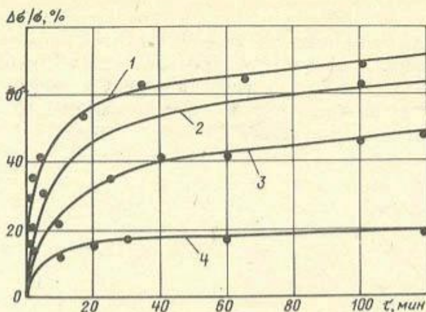
Релаксация напряжений в песчаном грунте, укрепленном различными способами 1 — 5% эмульгированного битума; 2 — 5% эмульгированного битума + 5% цемента; 3 — то же, 10% цемента; 4 — 10% цемента
