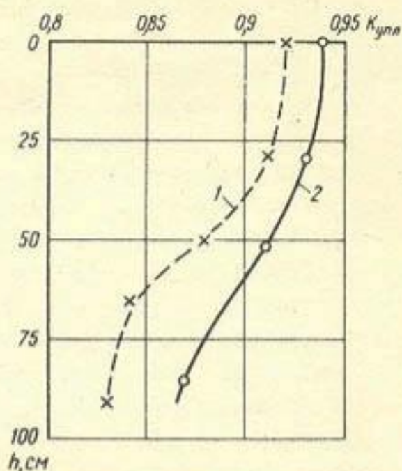
Распределение плотности грунта в траншейной неуплотненной засыпке (1) и после пролива водой (2)
