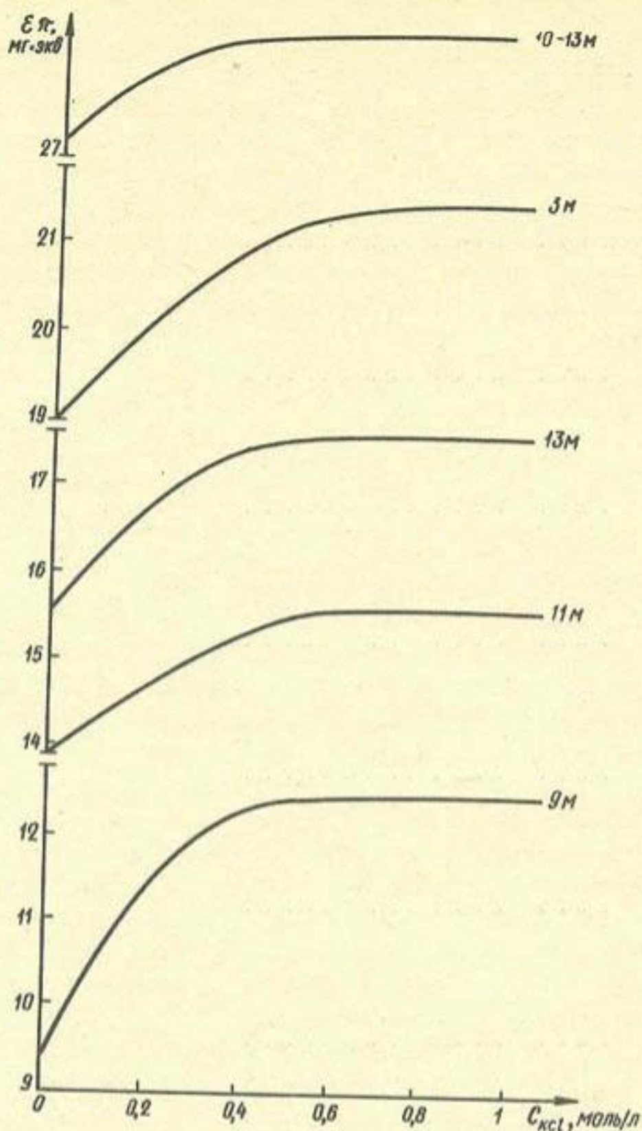
Зависимость емкости поглощения грунта от концентрации хлористого калия в 1 н. растворе NaOH
