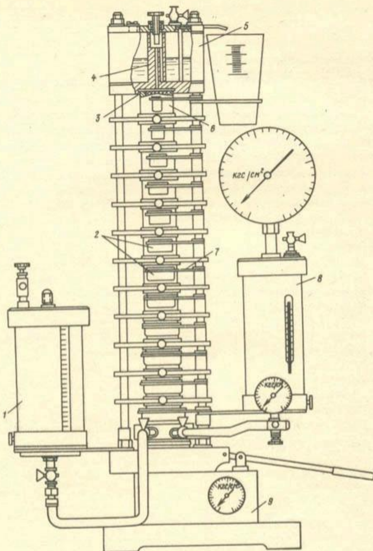
Устройство для лабораторного закрепления грунтов
