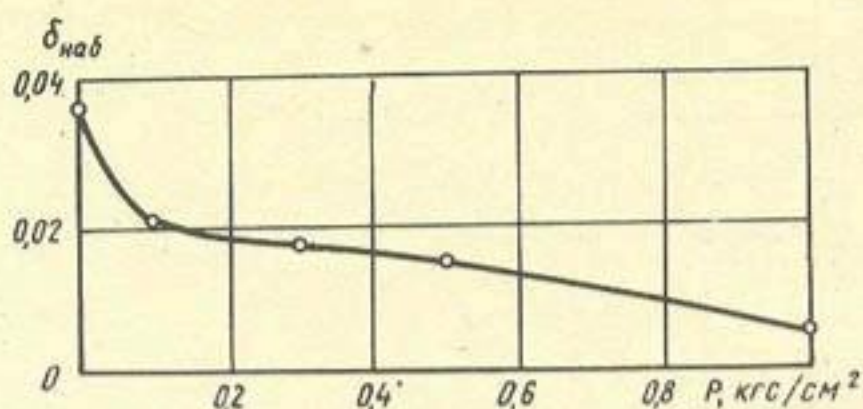
Рис. 1. Зависимость относительного разуплотнения от вертикальной пригрузки
