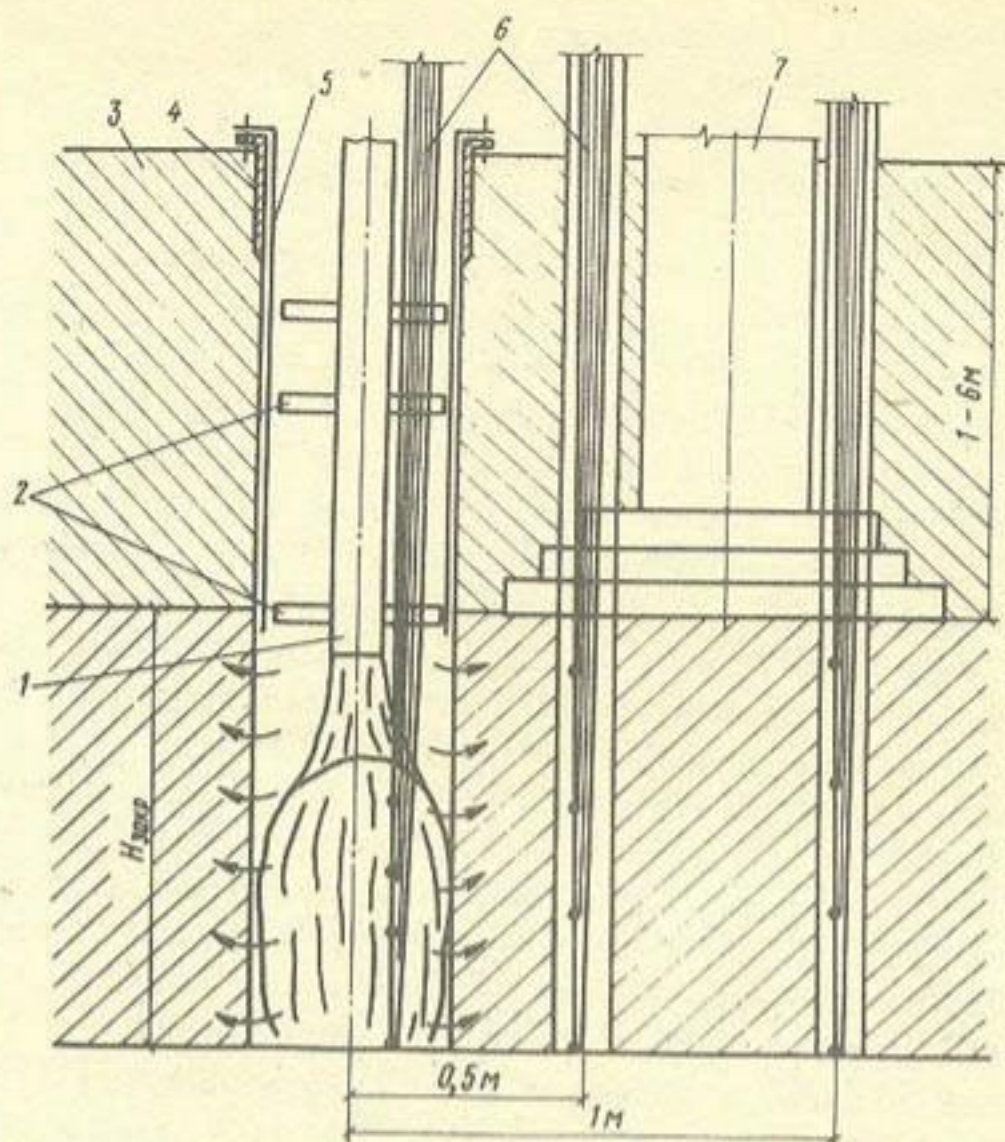
Схема закрепления основания существующего здания
