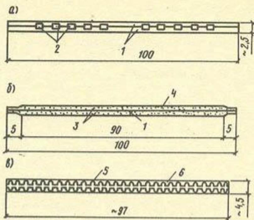
Экспериментальные конструкции вертикальных дрен
