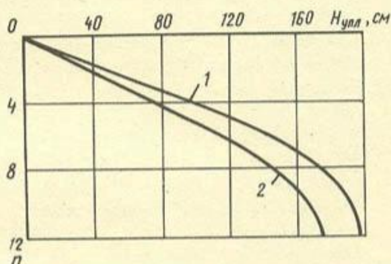
Рис. 2. Изменение глубины уплотнения H_{упл} для суглинка (1) и супеси (2) при \gamma_{ск} > 1,6 \text{ т/м}^3 в зависимости от числа ударов n
