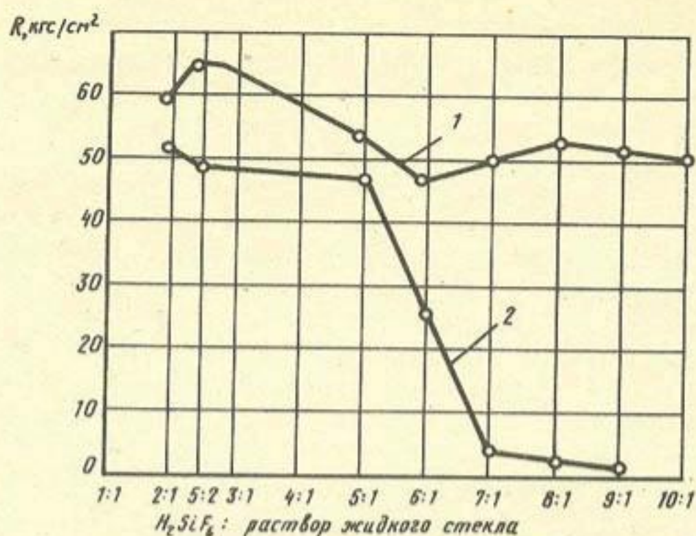
Зависимость предела прочности образцов при сжатии от объемного соотношения между H_2SiF_6 и раствором жидкого стекла 1 — сухие образцы; 2 — через 1 мес хранения в воде
