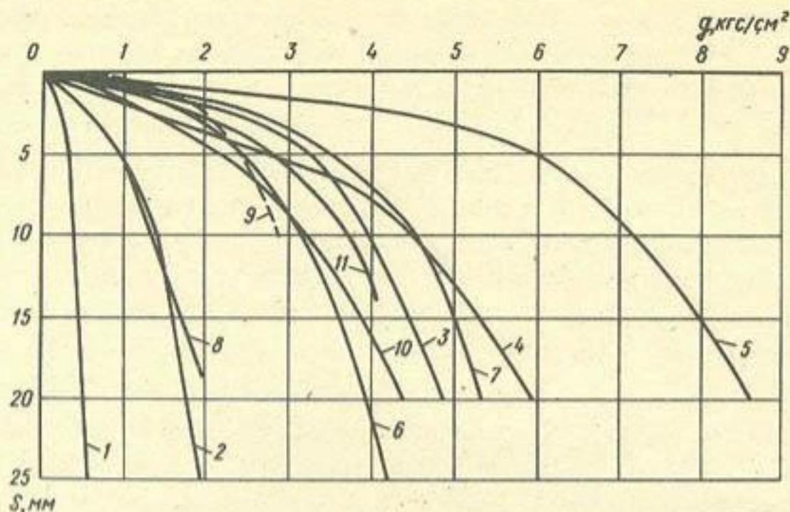
Рис. 2. Зависимость горизонтальных перемещений верха фундаментов S от приведенной величины горизонтальной нагрузки по боковой поверхности q 1, 8 — фундамент с откопанными боковыми стенками; 2–5 — q = 0, 2, 4 и 6 \text{ кгс/см}^2 ; 6–7 — q = 2-4 \text{ кгс/см}^2 ; 9–11 — q = 3,5 и 6 \text{ кгс/см}^2
