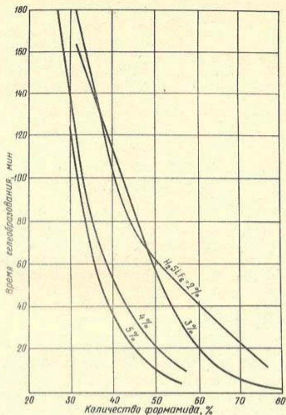
Влияние добавок H_2SiF_6 на продолжительность гелеобразования
