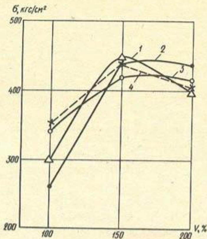
Рис. 2. Изменение прочности пластрасктора (смола ФРЭС + кероген 70) в зависимости от концентрации наполнителя по истечении 150 сут хранения в различных средах 1 — вода водопроводная; 2 — рН = 11; 3 — рН = 1,1; 4 — воздушно-влажное хранение
