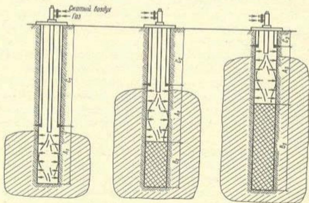
Рис. 2. Схема поэтапного обжига закрепляемой толщи
