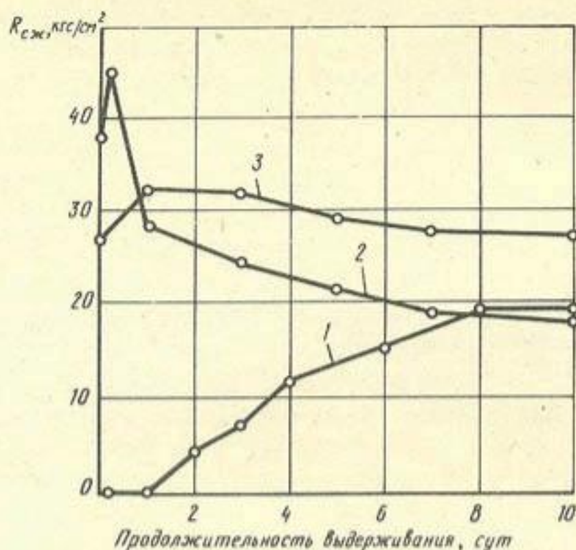
Рис. 2. Зависимость предела прочности при сжатии водонасыщенных образцов от продолжительности выдерживания до уплотнения зологрунтовой смеси различного состава 1 – без активизирующей добавки; 2 – с кремнефтористоводородной кислотой; 3 – с соляной кислотой
