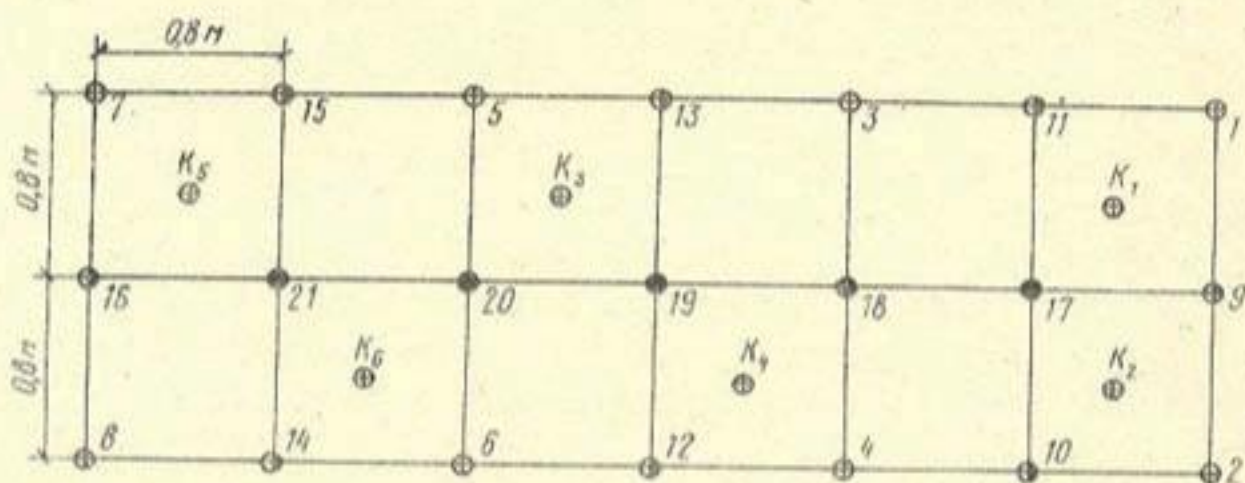
Рис. 3. План расположения инъекционных скважин опытно-производственного участка
