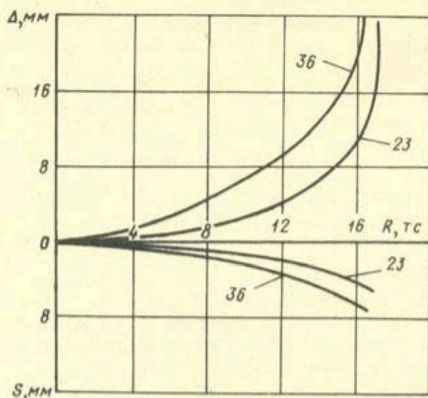
Зависимость вертикальных S и горизонтальных \Delta перемещений от комплексной нагрузки
