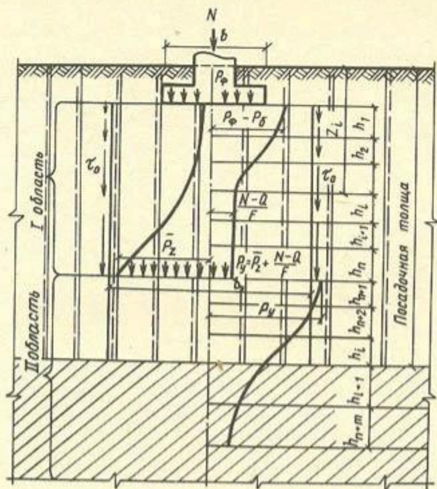
К расчету вертикальных давлений в массиве от веса сооружения и сил отрицательного сопротивления грунта
