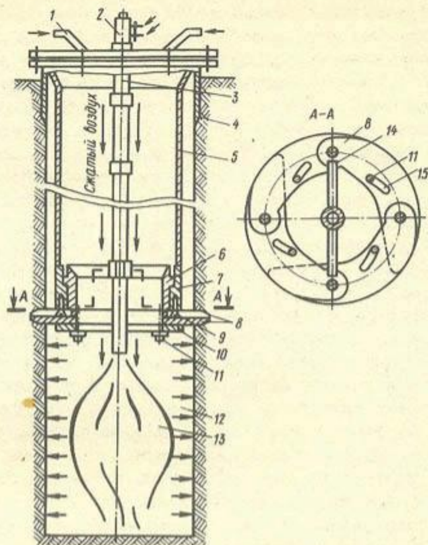
Рис. 1. Отсекатель рабочего объема скважины
