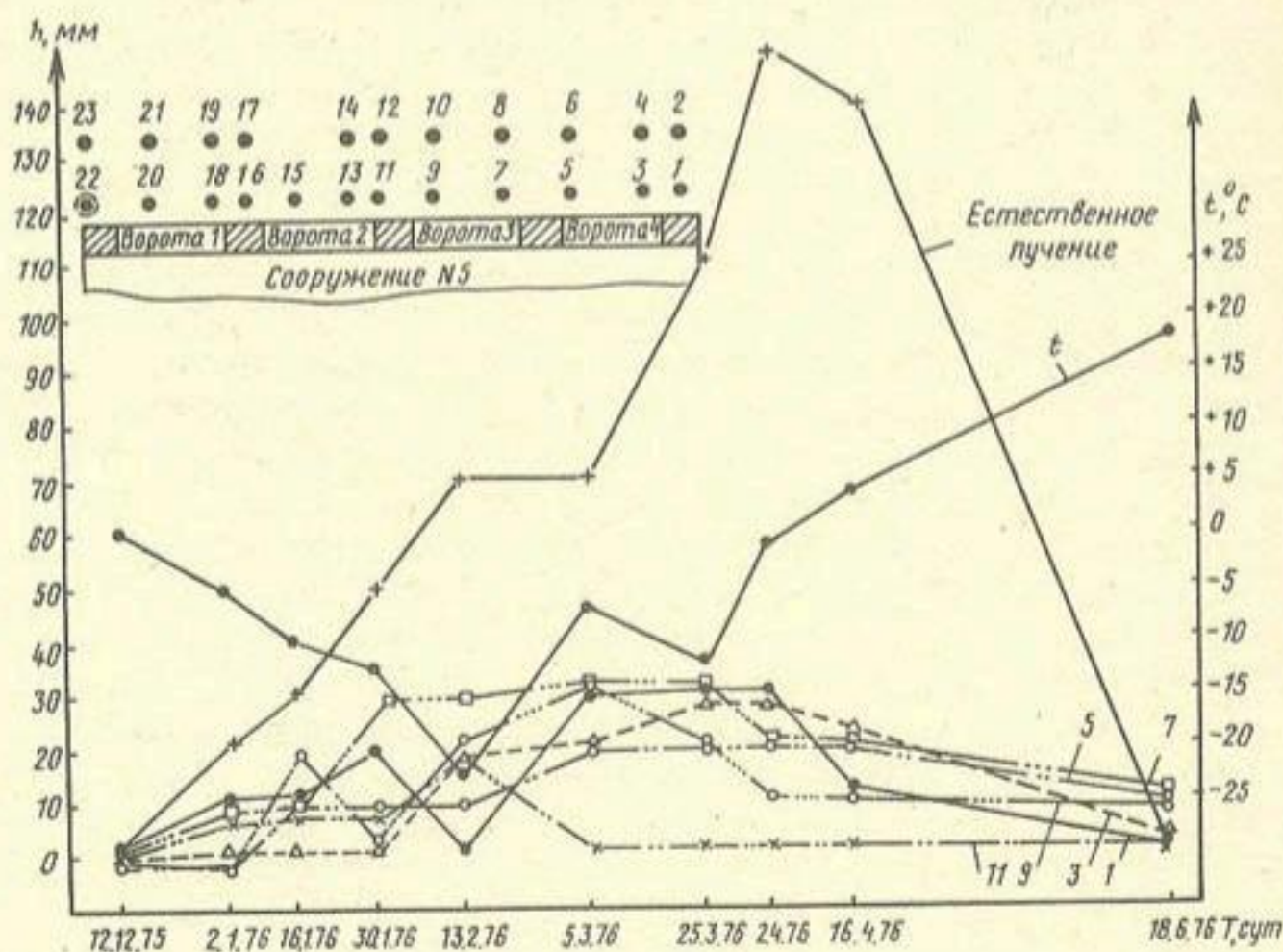
Рис. 1. Изменение величины пучения грунта анодной зоны во времени 1–23 – номера контрольных точек в зоне укрепленного грунта
