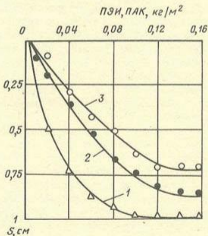
Рис. 2. Зависимость толщины S слоя грунта, укрепленного способом пропитки, от расхода комплексообразующих реагентов ПЭИ и ПАК 1 - песок; 2 - суглинок легкий пылеватый; 3 - суглинок тяжелый
