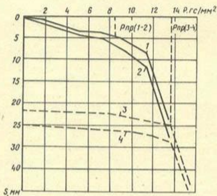
Рис. 2. Зависимость осадки от нагрузки 1-2 – первичное загрузке; 3-4 – повторное загрузке
