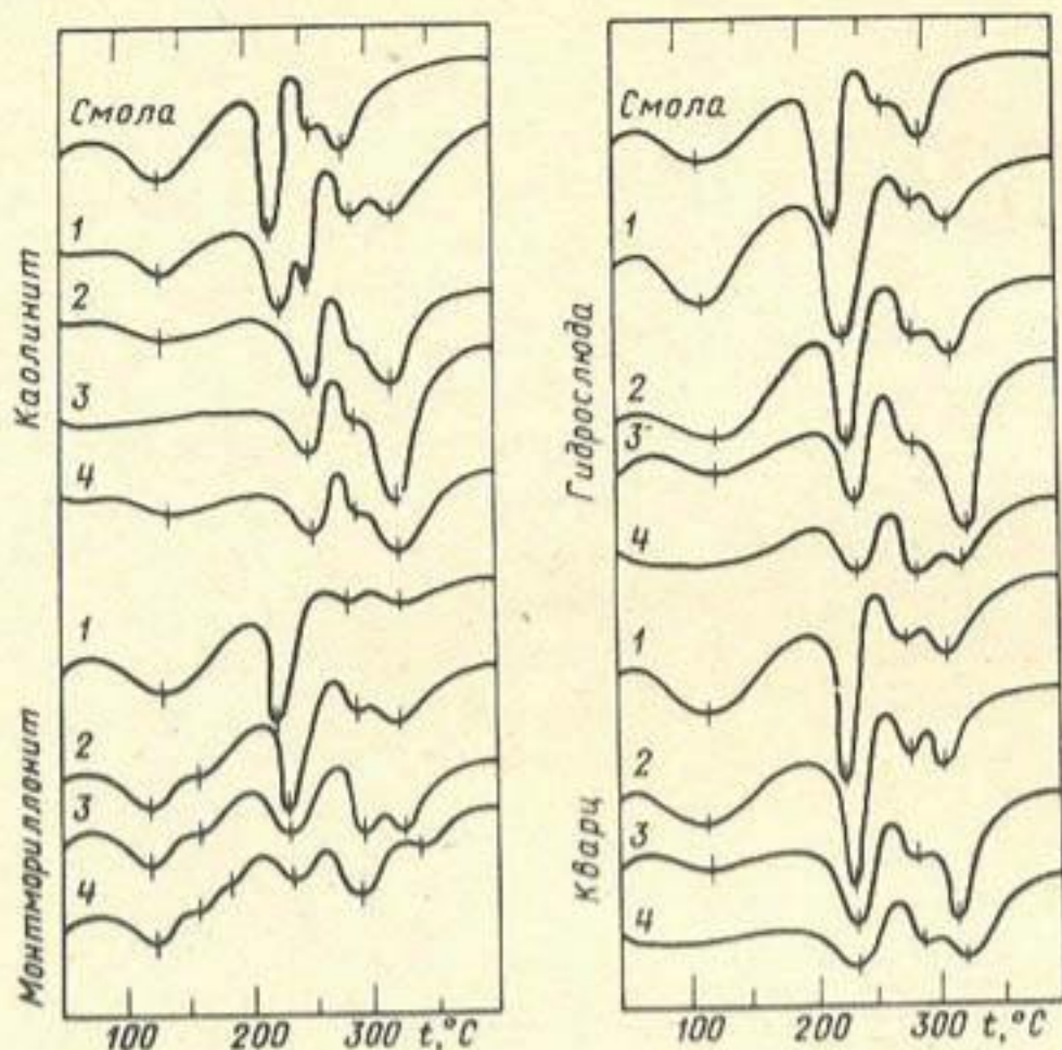
Рис. 2. Термограммы карбамидной смолы и ее композиций с минералами 1, 2, 3 и 4 — соотношение (по массе минерал: смола соответственно 5:95, 25:75, 50:50 и 75:25
