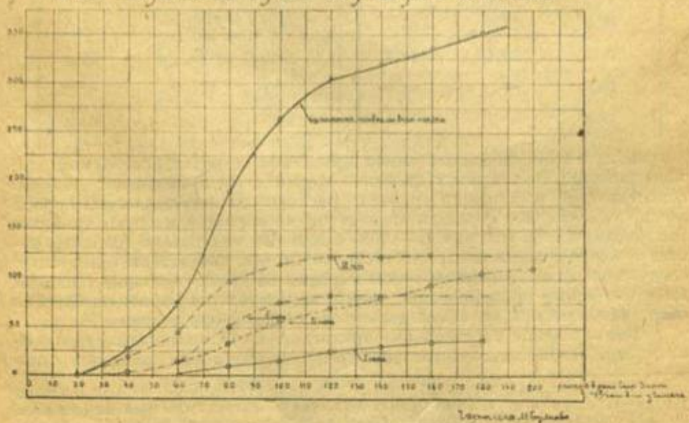
Кривые №1 зависимости числа действующих систем Нижне-Сыр-Дарьинского и Отырарского рай- онов от расхода в реке Сыр-Дарья по полям.
