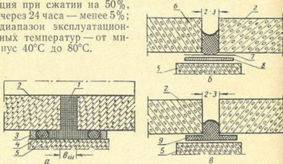
Рис. 12. Уплотнение швов в безраструбных лотках поронизолом, изолом или битумно-шлаковатной прокладкой:
