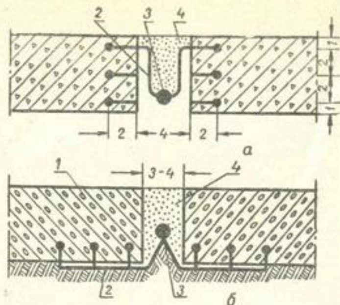
Рис. 22. Шпонка из профилированного полиэтилена в сборной (а) и моноклитной (б) облицовке каналов:
