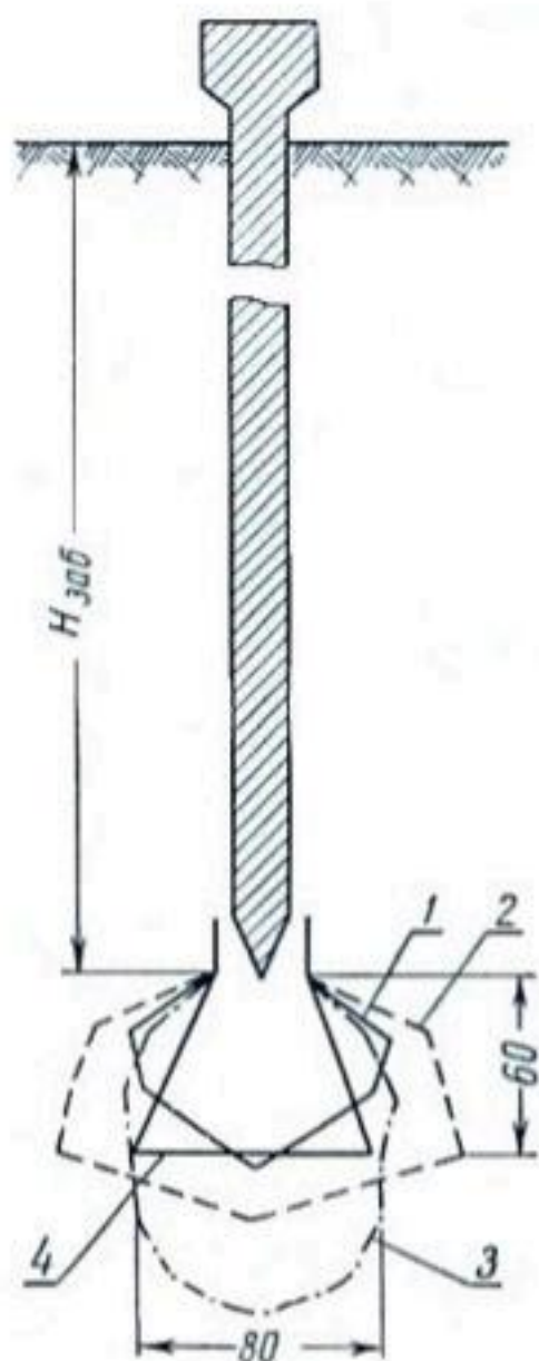
Рис. 27. Схема зон уплотнения сваями в совхозе № 28 с глубиной забивки: 1 — 2,5 м; 2 — 3,0 м; 3 — 3,5 м; 4 — расчетный контур уплотненного основания.
