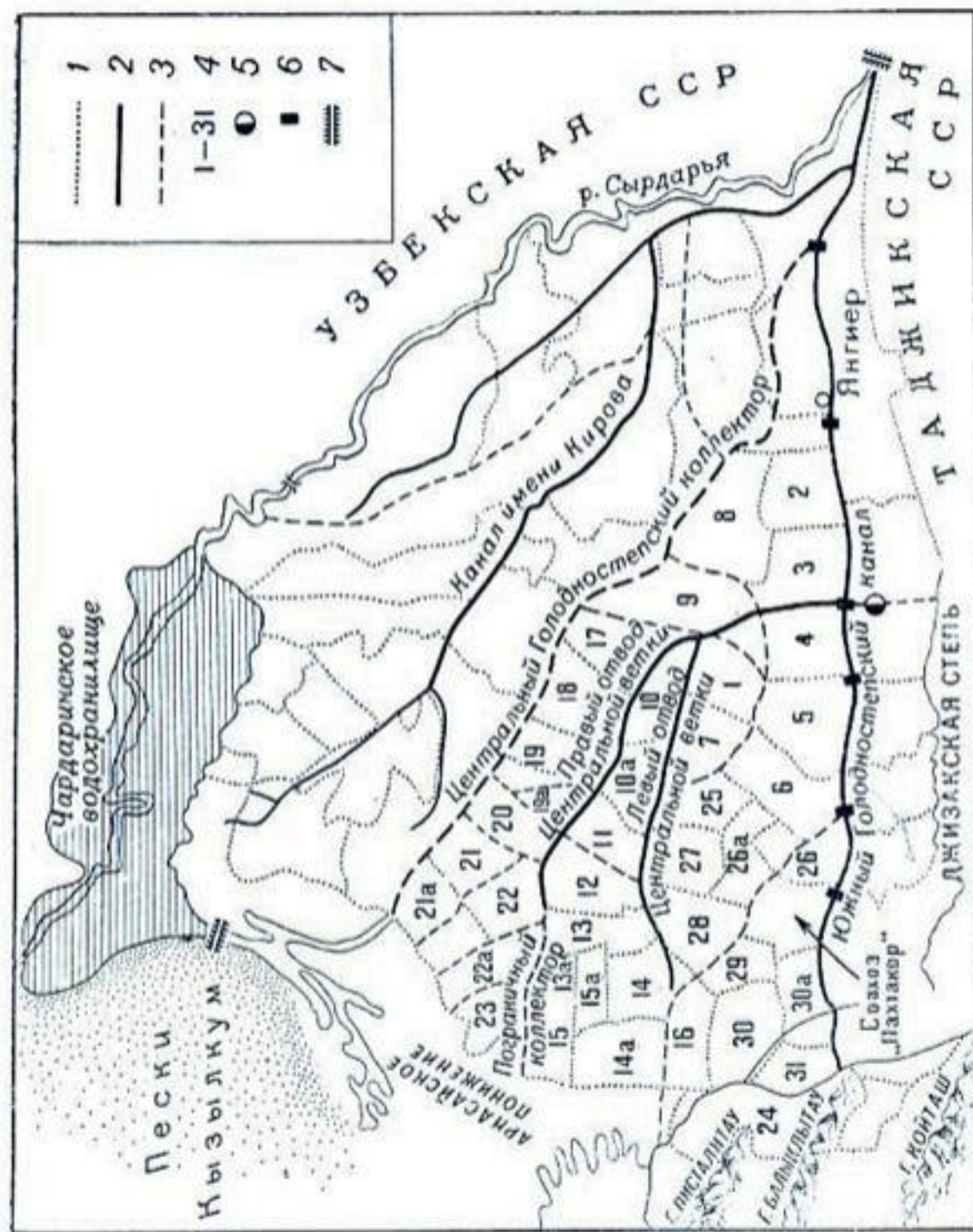
Рис. 1. Схема орошения и освоения Голодной степи: 1 — границы хозяйств; 2 — магистральные каналы; 3 — межхозяйственные коллекторы; 4 — номера совхозов; 5 — насосная станция; 6 — сооруженная; 7 — плотина.
