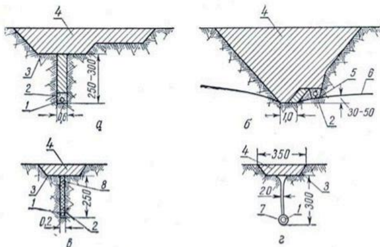
Рис. 42. Методы производства работ по горизонтальному дренажу: а — траншейным дрепоукладчиком; б — методом «полки»; в — щелевым дрепоукладчиком; г — бестраншейным дрепоукладчиком; 1 — дренажная труба; 2 — фильтровая обмотка; 3 — корыто; 4 — обратная засыпка; 5 — полка; 6 — кривая депрессии; 7 — фильтровая обмотка; 8 — замык щели.
