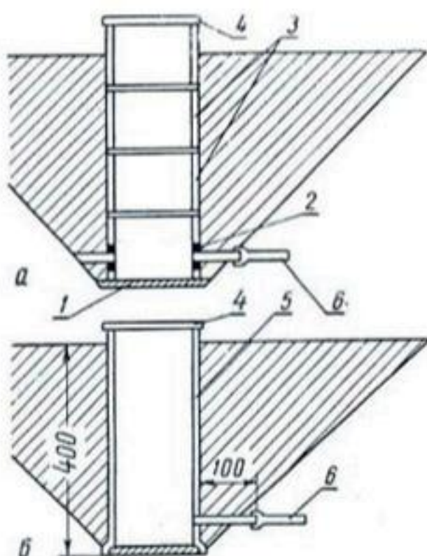
Рис. 52. Конструкция колодцев (размеры в см):
