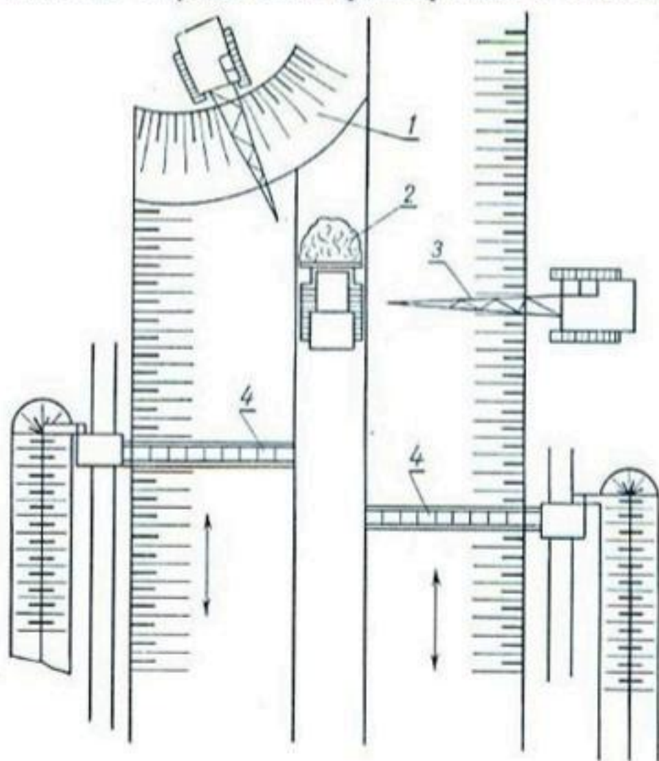
Рис. 19. Схема производства работ по подготовке каналов под облицовку с помощью машины ЭМ-201 налевой ветке ЮГК:
