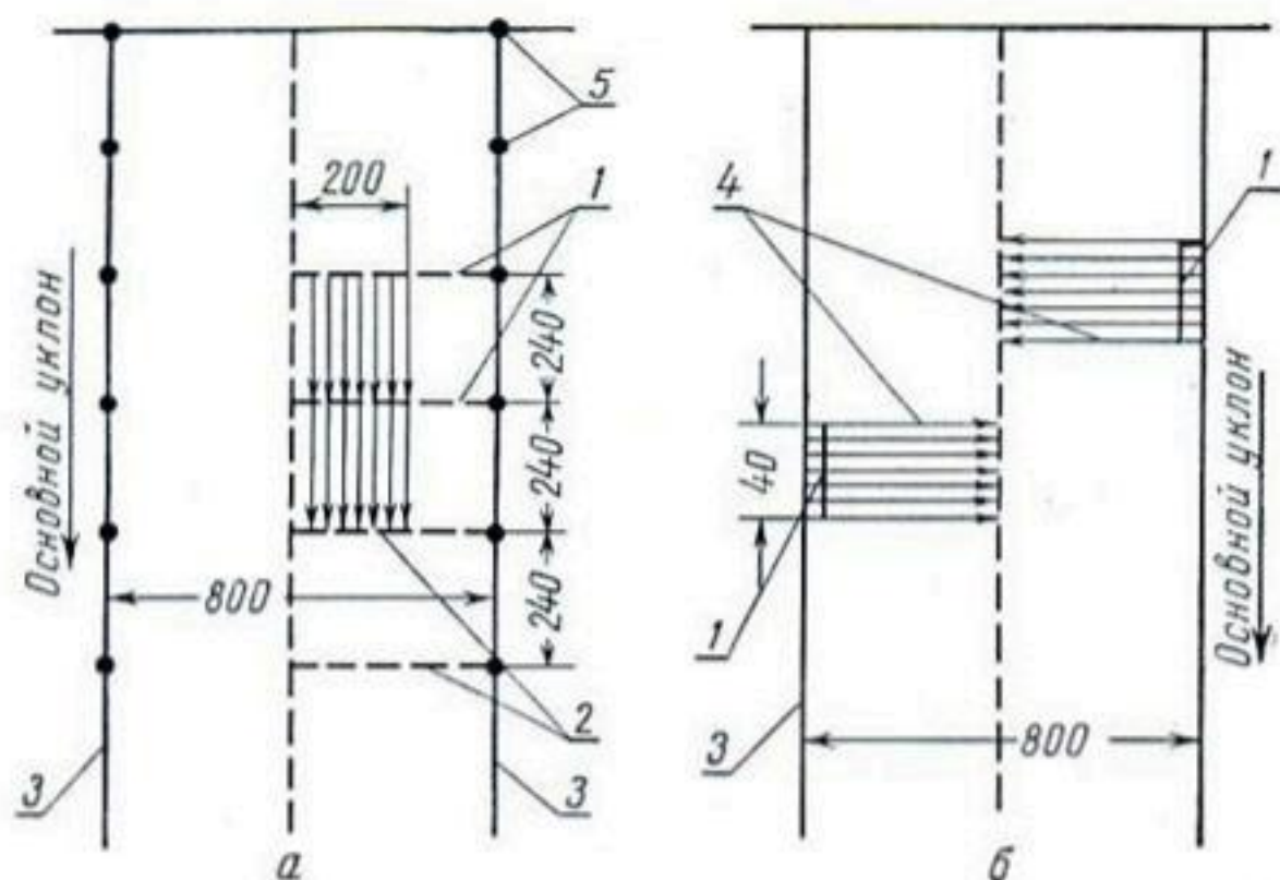
Рис. 35. Схема полива из гибких трубопроводов (размеры в м): а — продольная; б — поперечная; 1 — работающие трубопроводы; 2 — приготовленные к работе трубопроводы; 3 — участковые оросители; 4 — поливные борозды; 5 — водовыпуски.
