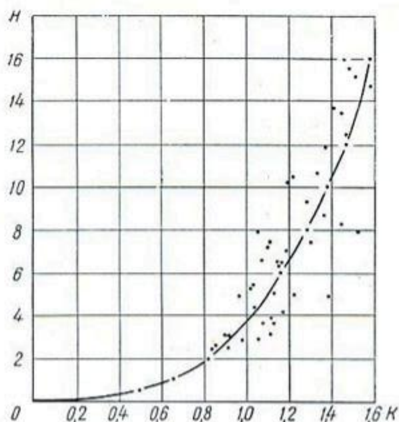
Рис. 38. Зависимость оросительных норм от уровня грунтовых вод.
