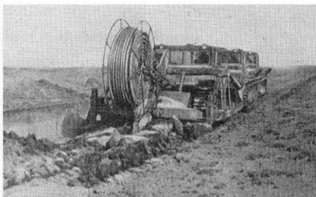
Рис. 43. Устройство дрены бестраншейным дренаукладчиком БДМ-300 на тяге трех тракторов ДЭТ-250.
