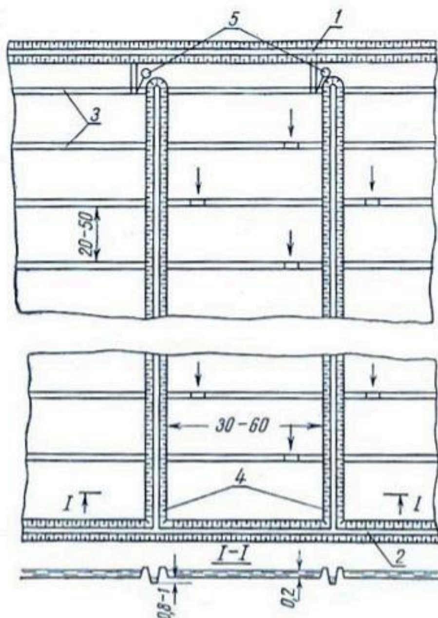
Рис. 60. Схема промывки по методу Голодностеп-строя с подачей воды по длине чеков на фоне временного дренажа (размеры в м):
