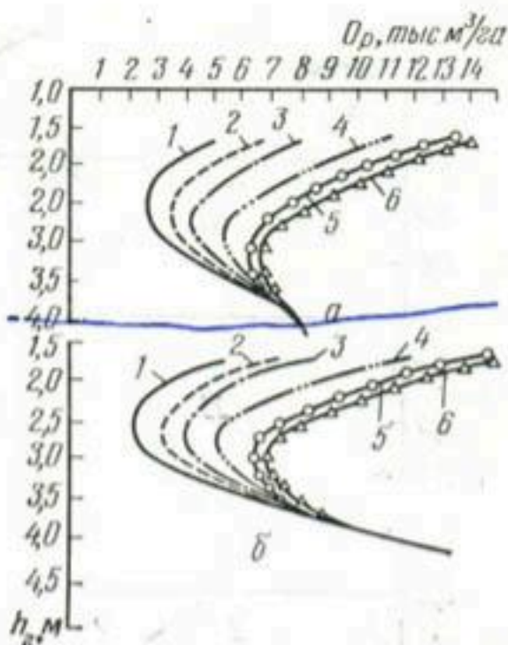
Рис. 41. Изменение суммарных расходов воды от глубины грунтовых вод для Голодной степи при различной минерализации грунтовых вод:
