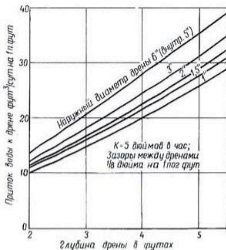
Рис. 138. Зависимость притока воды от диаметра дрена по данным Киркхема (1949, 1950).
