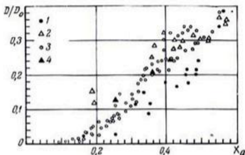
Рис. 206. Зависимость между отношением D/D_0 и долей наполненных воздухом пор x_a :
