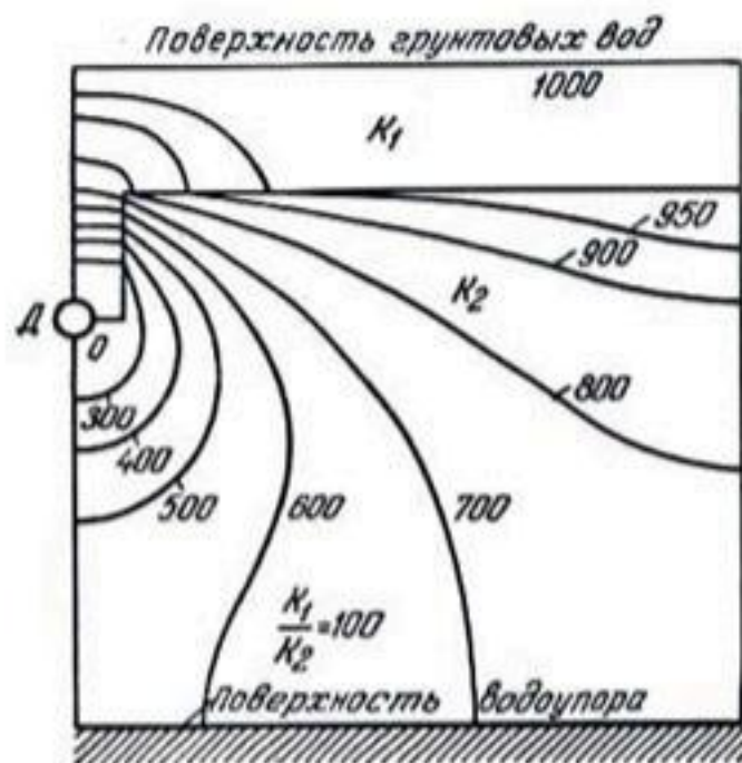
Рис. 86. Эквипотенциали для дренажной трубки в двухслойном подшертом грунте с коэффициентами фильтрации k_1 и k_2 , когда поверхностная почва с k_1 используется для обратной засыпки траншеи. Буквой Д обозначена дрена. По Лютину и Гаскеллу (1950).
