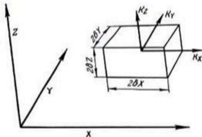
Рис. 32. Элементарный объем анизотропного гидравлического проводника, используемый при выводе уравнения непрерывности.
