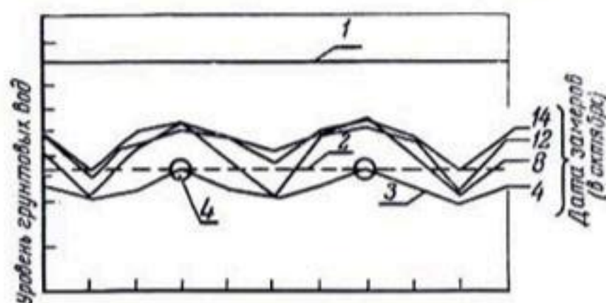
Рис. 233. Изменение уровня грунтовых вод в зависимости от времени подпочвенного орошения в органической почве. По Моррису (1949):
