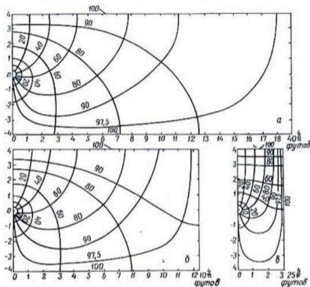
Рис. 126. Линии тока и эквипотенциали, построенные для потока скопившейся воды.
