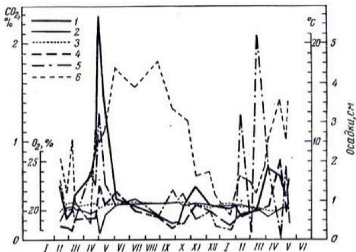
Рис. 205. Изменение содержания \text{CO}_2 и \text{O}_2 в течение года на глубине 15 см на участках, которые были засеяны пшеницей. По Расселу и Апплейярду (1913):
