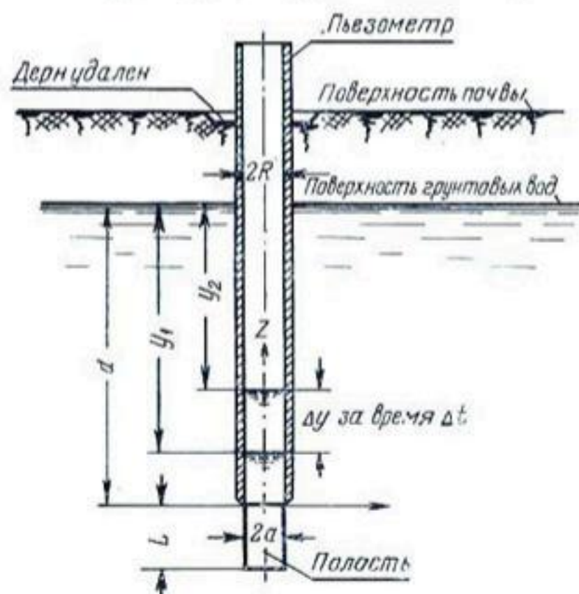
Рис. 195. Чертеж, служащий для разъяснения пьезометрического метода. По Лютину и Киркхену (1949).
