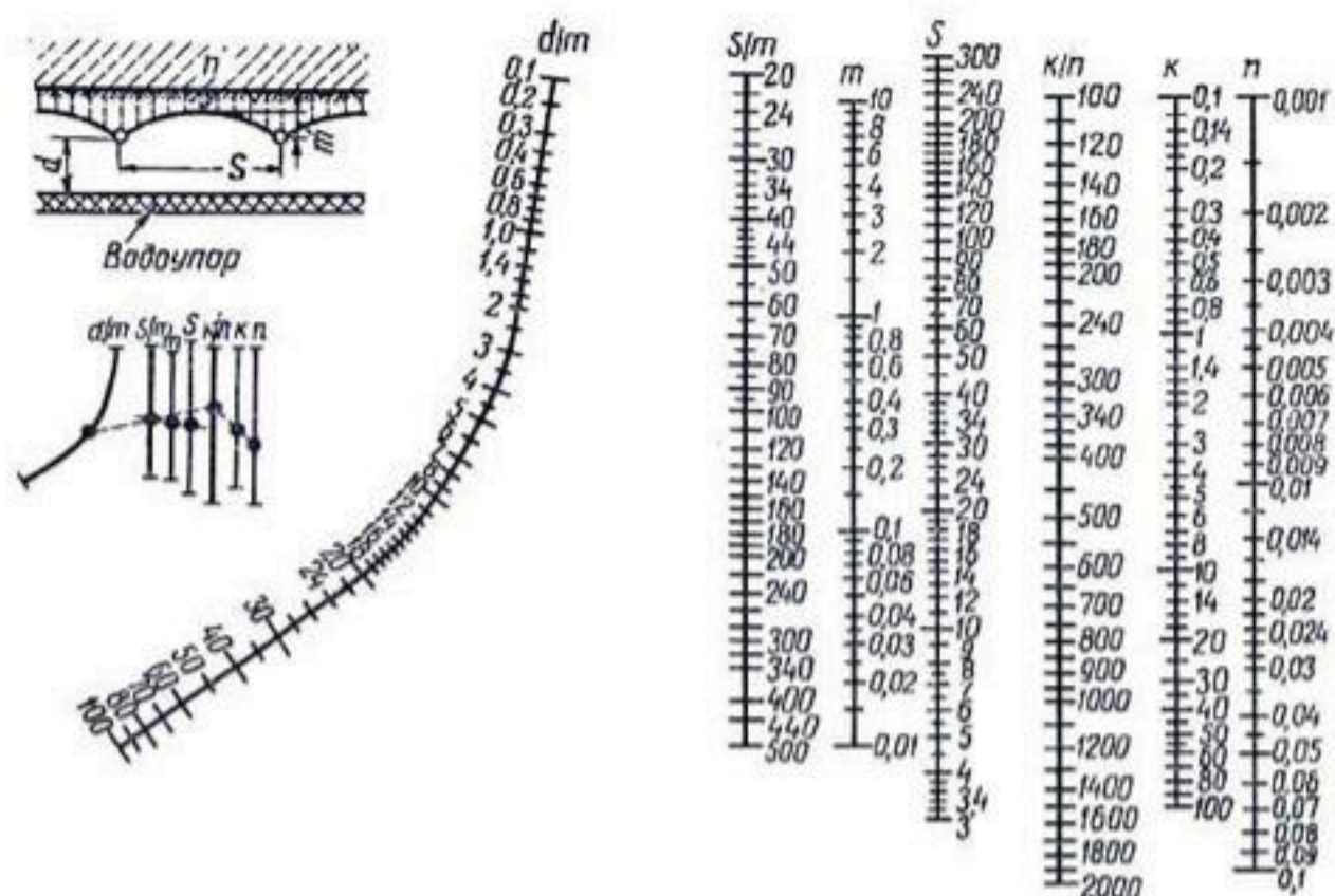
Рис. 36. Номограмма для определения расстояний между дренами при k/n \geq 100 (по Виссеру, 1954):
