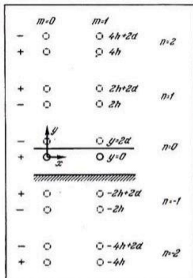
Рис. 79. Подобия, построенные для задачи, иллюстрируемой рисунком 78 (по Киркхему, 1949).
