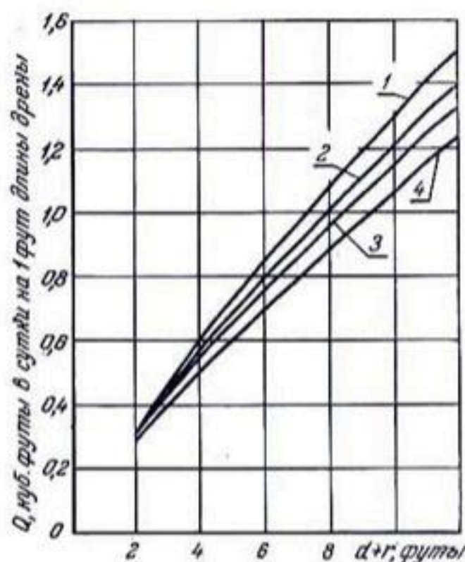
Рис. 74. Зависимость скорости просачивания воды Q в дренажную трубу в задаче, иллюстрируемой рисунком 72, от глубины залегания трубы (d+r) . Графики построены для различных диаметров труб. Труба в каждом случае работает полным сечением ( s=r ) без засасывания или подпора. Коэффициент фильтрации k=2,54 см/сутки. Диаметры труб: 1—30,5 см (12"); 2—20,3 см (8"); 3—15,2 см (6"); 4—10,2 см (4").
