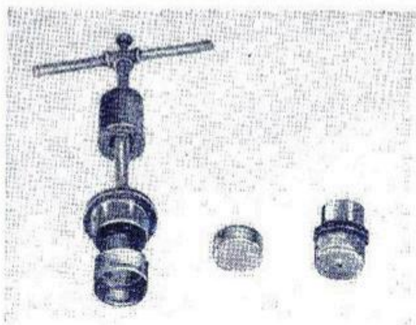
Рис. 182. Оборудова- ние для взятия почвен- ного монолита. По Лют- цу и др. (1947).
