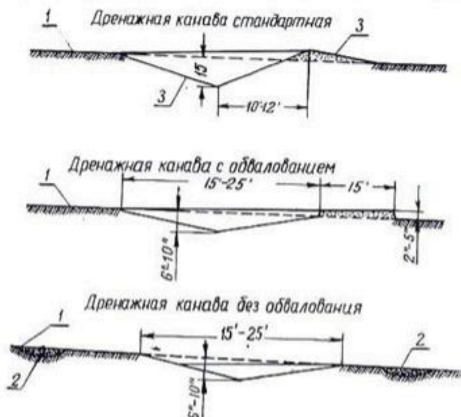
Рис. 167. Два типа стандартных дренажных террас (по Войта):
