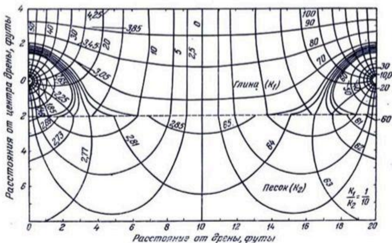
Рис. 84. Сетка токов, аналогичная схеме, изображенной на рисунке 83; разница заключается лишь в том, что песок и глина на этом рисунке поменялись местами. По Киркхему (1951).
