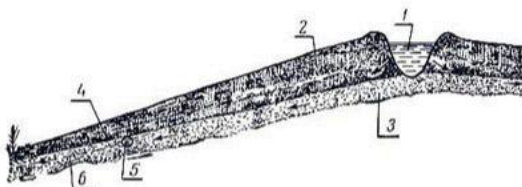
Рис. 156. Дрена, перехватывающая воду, которая фильтруется из канала:
