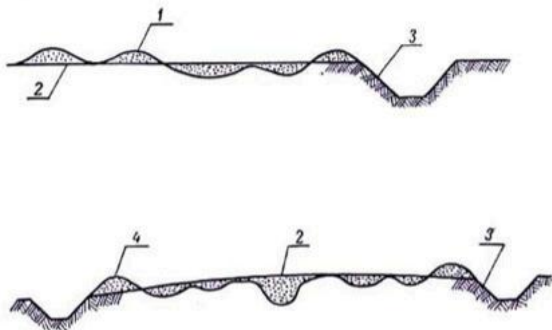
Рис. 165. Два вида планировки при устройстве поверхностного дренажа:
