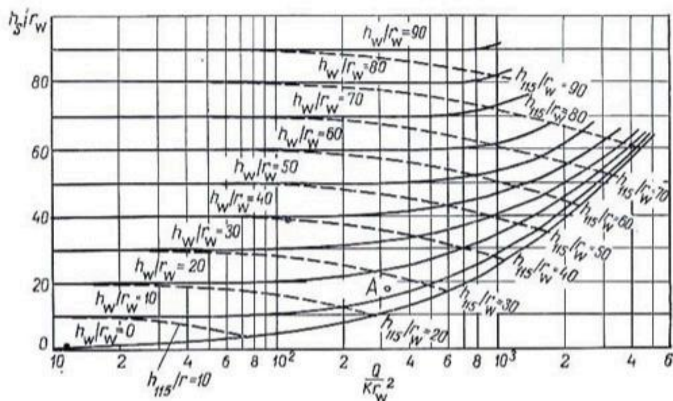
Рис. 98. Функциональная зависимость между расходом и геометрическими параметрами:
