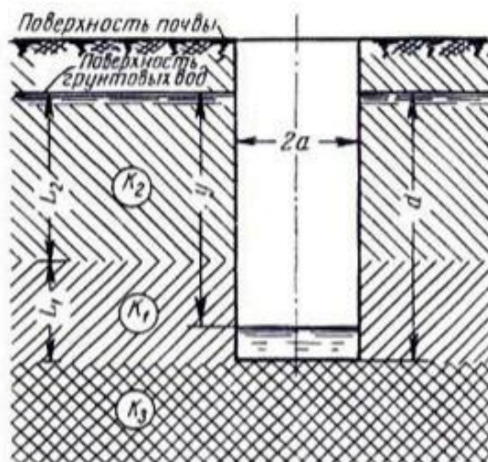
Рис. 192. Чертеж скважины, используемый при выводе формулы Хоугхаудта для слоистого грунта.
