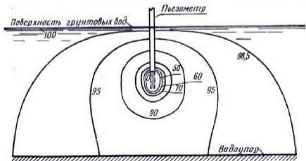
Рис. 197. Распределение гидравлического напора вокруг пьезометрической полости. По Лютину и Киркхему (1949).
