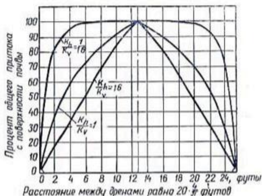
Рис. 128. Распределение притока в плоскости грунтовой воды в зависимости от величины отношения k_h/k_v для трех гидродинамических сеток, изображенных на рисунке 127.
