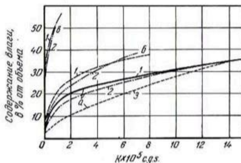
Рис. 24. Гидравлическая проводимость некоторых пористых материалов как функция содержания влаги:
