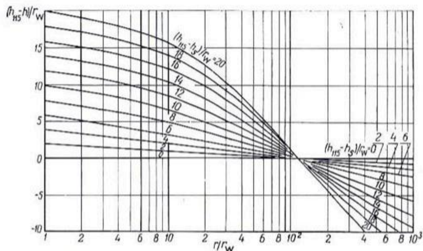
Рис. 100. Обобщенные кривые профиля свободной поверхности для колодцев в непiezометрическом бассейне грунтовых вод.
