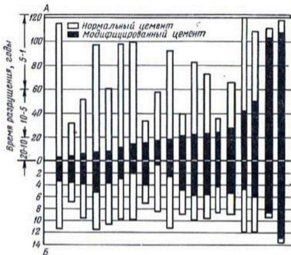
Рис. 148. Сравнение сульфатостойкости девятнадцати модифицированных и нормальных цементов одних и тех же заводов.
