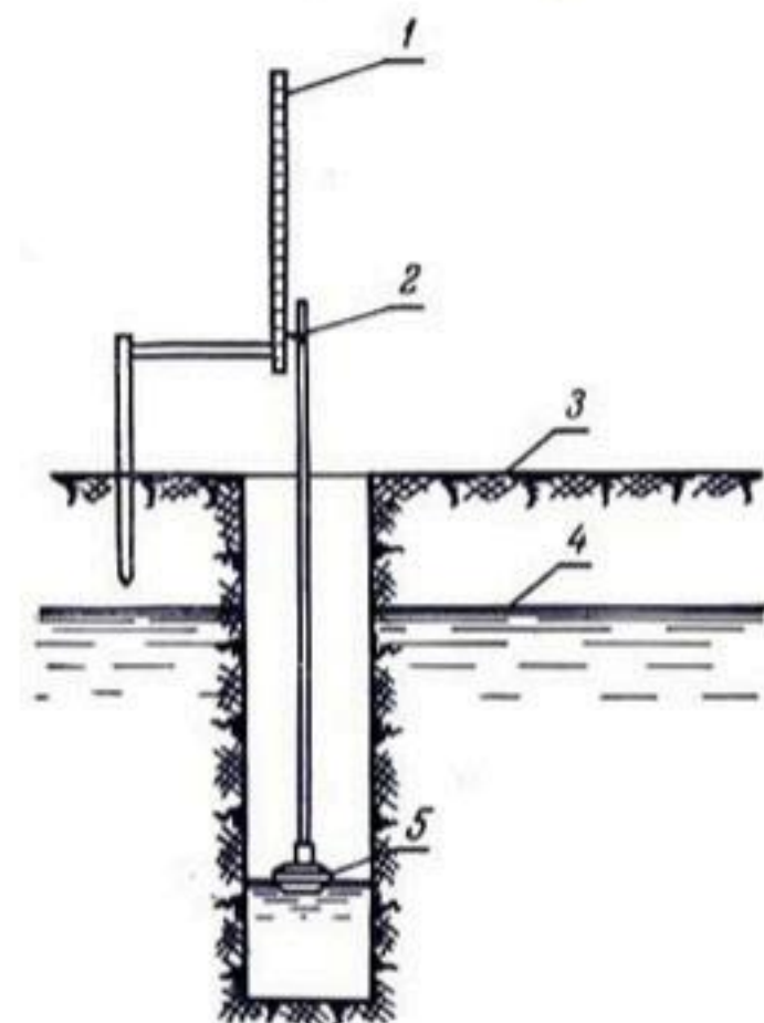
Рис. 186. Метод буровой скважины. На рисунке показано оборудование, которое было усовершенствовано Виссером и его помощниками для использования в Нидерландах:
