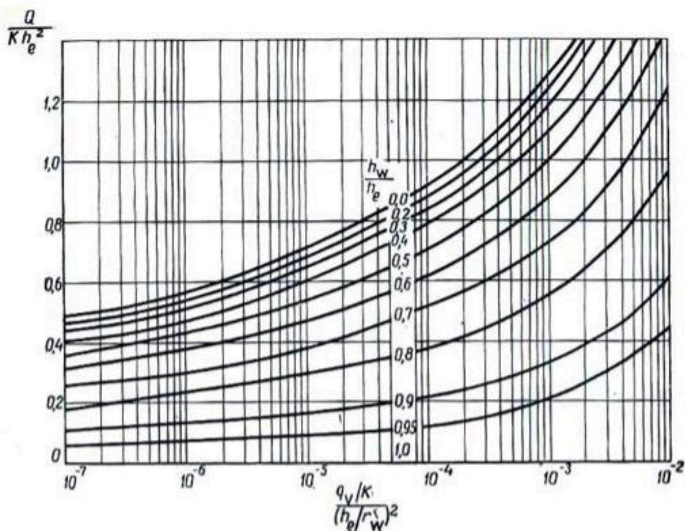
Рис. 102. Параметры расхода для вертикально пополняемого неограниченно- го грунтового потока. По вертикали — коэффициент колодца; по горизонтали — коэффициент пополнения.
