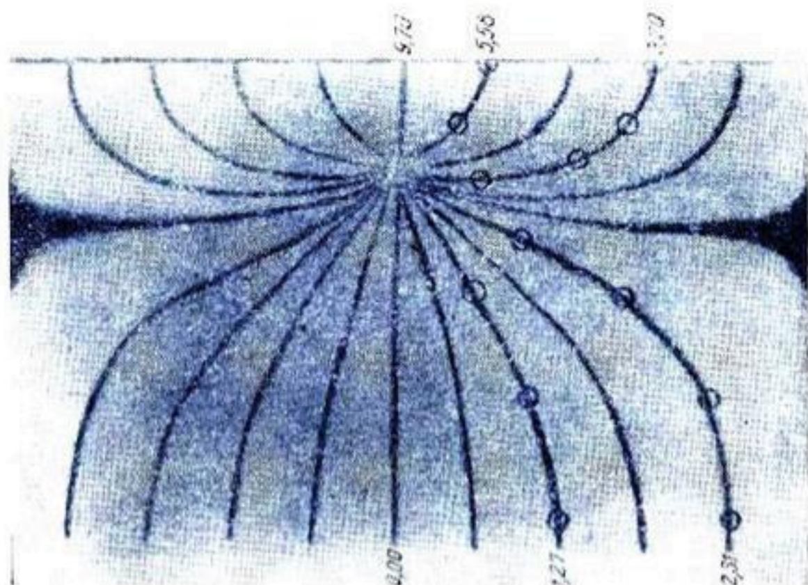
Рис. 90. Линии токов, полученные Хардингом и Будом (1942) в резервуаре с песком, сравниваются с теоретическими линиями тока (обведенные кружками), полученными Киркхеном (1945). На рисунке показано просачивание как скопившейся, так и артезианской воды в одну из трубок, находящихся на равном расстоянии друг от друга.
