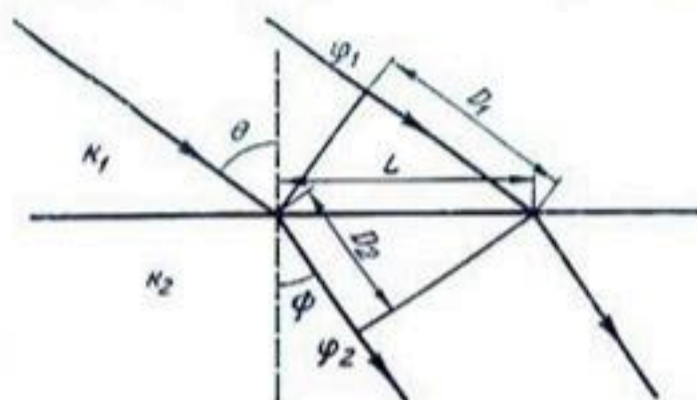
Рис. 31. Преломление линий тока на границе между двумя слоями грунта различной водопроницаемости k_1 и k_2 . Стрелки указывают направление линий тока. В изотропных почвах эквипотенциали \varphi_1 и \varphi_2 перпендикулярны линиям тока.
