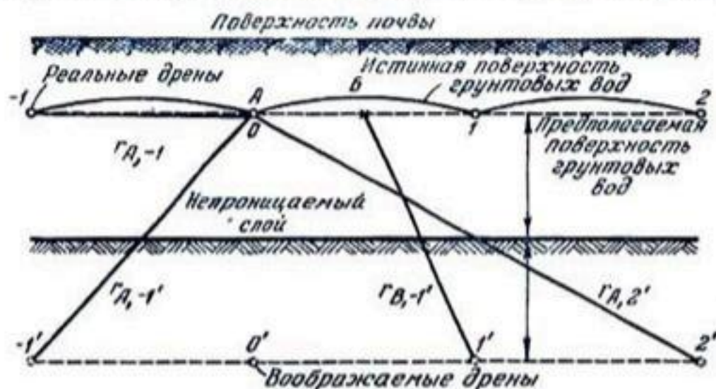
Рис. 34. Воображаемые дрены, создающие эффект непроницаемого слоя.
