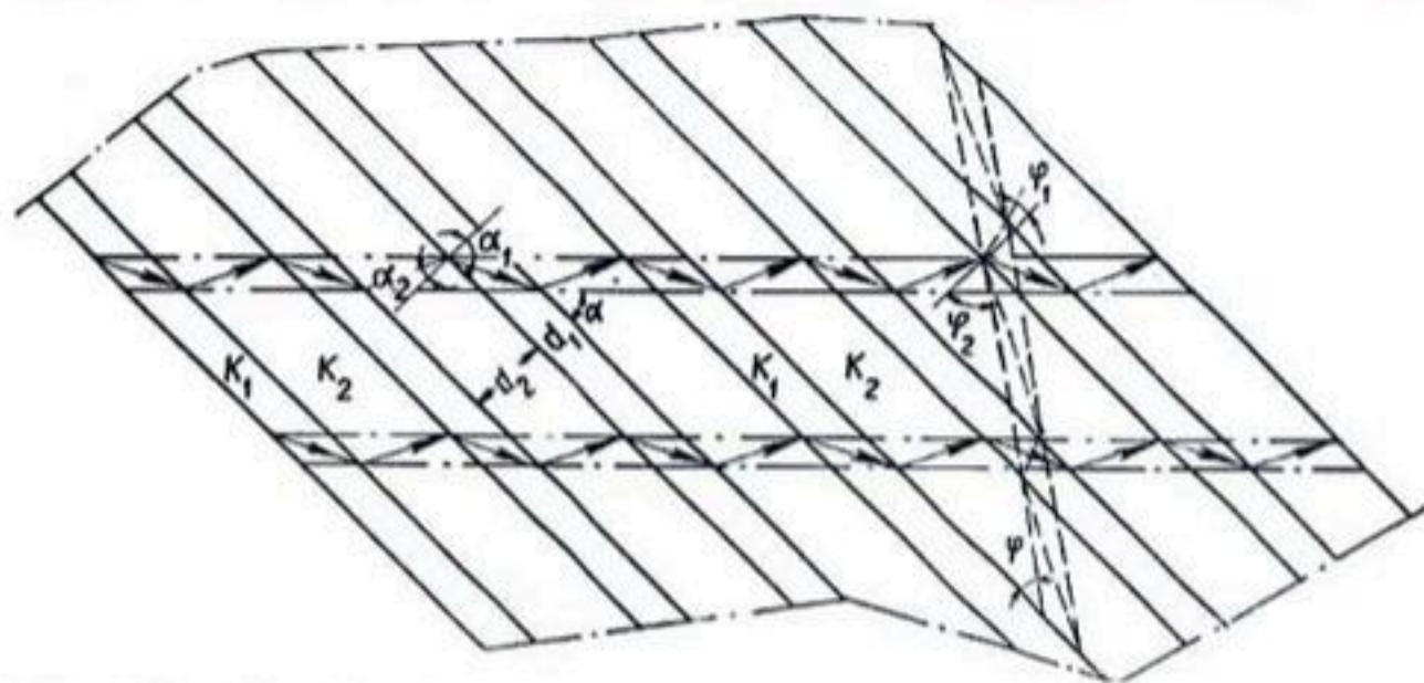
Рис. 117. Линейный поток через неоднородный грунт, состоящий из равномерно чередующихся однородных изотропных слоев, которые имеют неограниченную протяженность.
