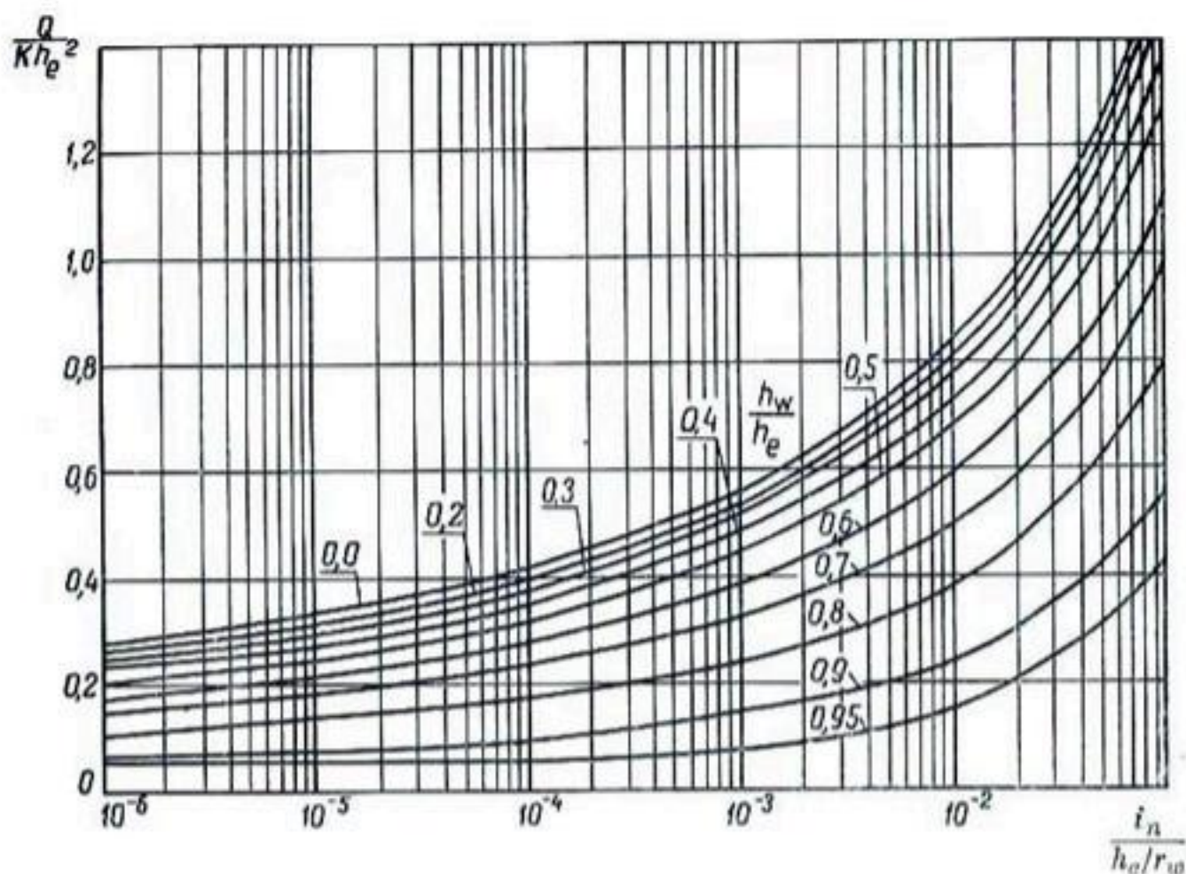
Рис. 101. Параметры расхода для «горизонтально пополняемого колодца» в неограниченной системе. По вертикали — коэффициент колодца; по горизонтали — коэффициент пополнения.
