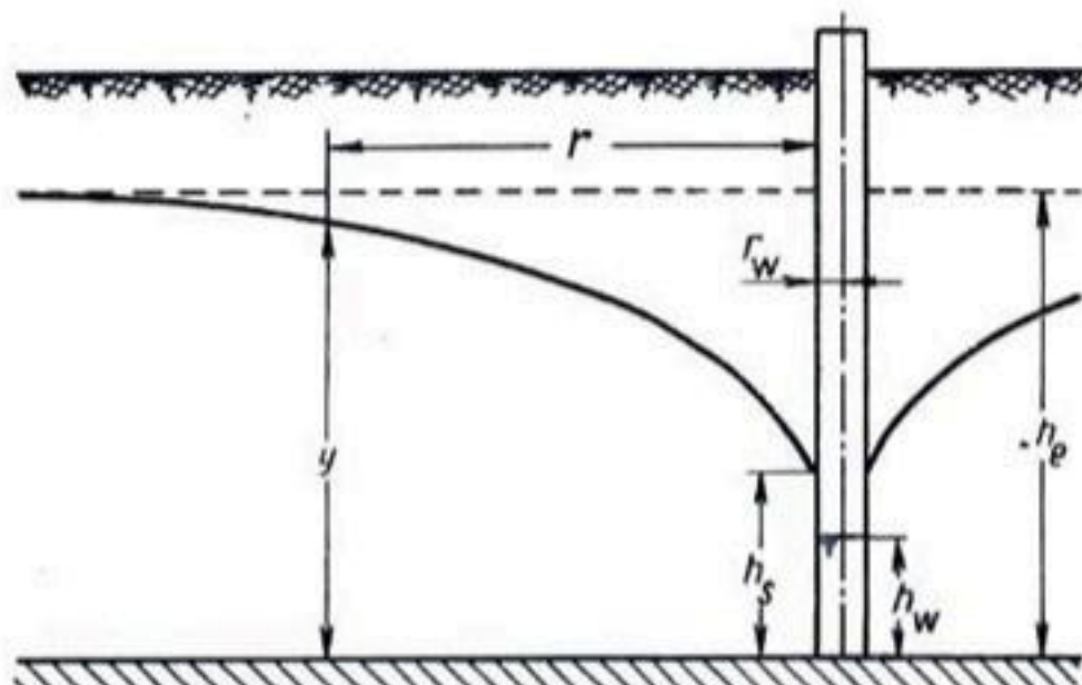
Рис. 97. Схема колодца в ненапорном бассейне грунтовых вод (показана и поверхность высачивания).
