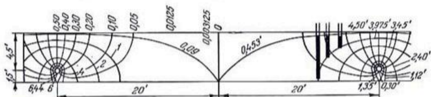
Рис. 80. Сетка токов для расположенных на одинаковом расстоянии дренажных трубок, работающих полным сечением. Эти трубки диаметром 18,3 см (0,60 фута) отстоят друг от друга на 12,2 м (40 футов), заглублены в водоносный слой на 1,22 м (4,5 фута) и находятся в затопленной почве, лежащей на непроницаемом слое, который расположен на глубине 1,83 м (6 футов). На левой половине рисунка эквипотенциали обозначены условными единицами 1, 2, 4, ... . На правой половине указан гидравлический напор относительно горизонтальной плоскости (в футах), проходящей через оси дрен. Пьезометры показывают напор воды 3,975 фута (1,21 м) на эквипотенциали 3,975 фута. Почва насыщена водой. Глубина слоя скопившейся воды бесконечно мала. Линии тока обозначены только на левой половине чертежа цифрами 0,50; 0,40; 0,30...; разность любых этих двух цифр дает значение той части полного расхода трубы, которая попадает в трубу между рассматриваемыми линиями тока. По Киркхему (1949).
