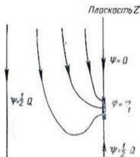
Рис. 130. Один из параллельных полосовых стоков, расположенных на равном расстоянии друг от друга в безграничной среде. По Энгелунду (1951).
