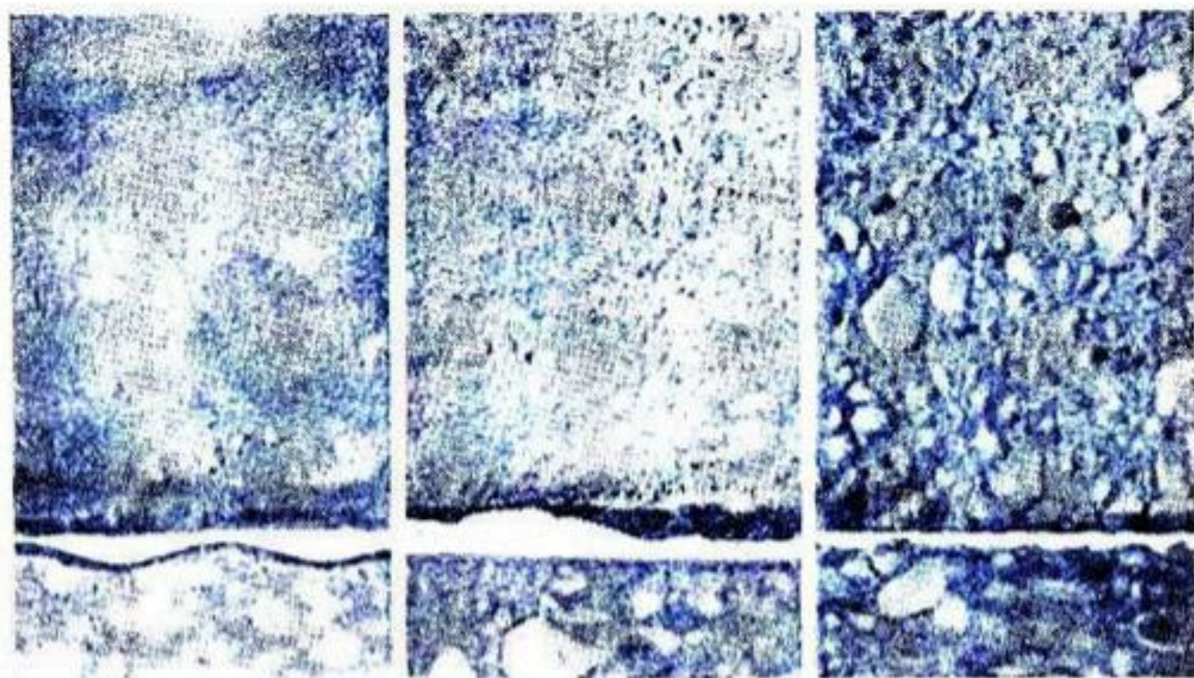
Рис. 146. Образцы из труб повышенного качества диаметром от 12 до 30 дюймов после 22-летней экспозиции. Слева направо:
