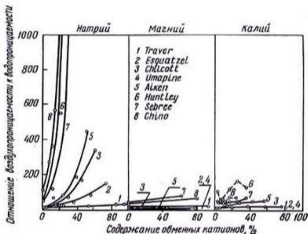
Рис. 177. Влияние обменного натрия, магния и калия на разрушение почвенной структуры, выраженное отношением воздухопроницаемости к водопроницаемости. По Бруксу и др. (1956).
