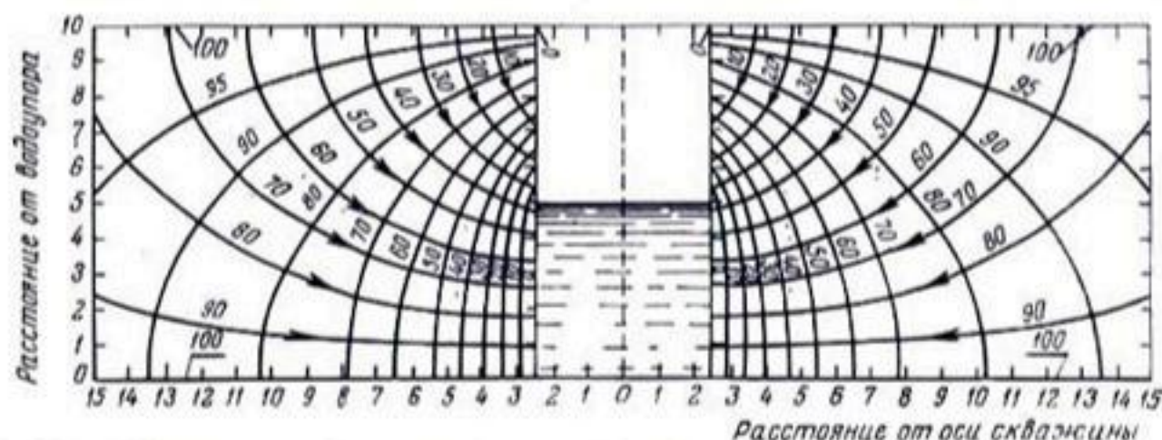
Рис. 190. Распределение напора вокруг скважины, наполовину заполненной водой (по Киркхему и ван Бейвелу, 1949).
