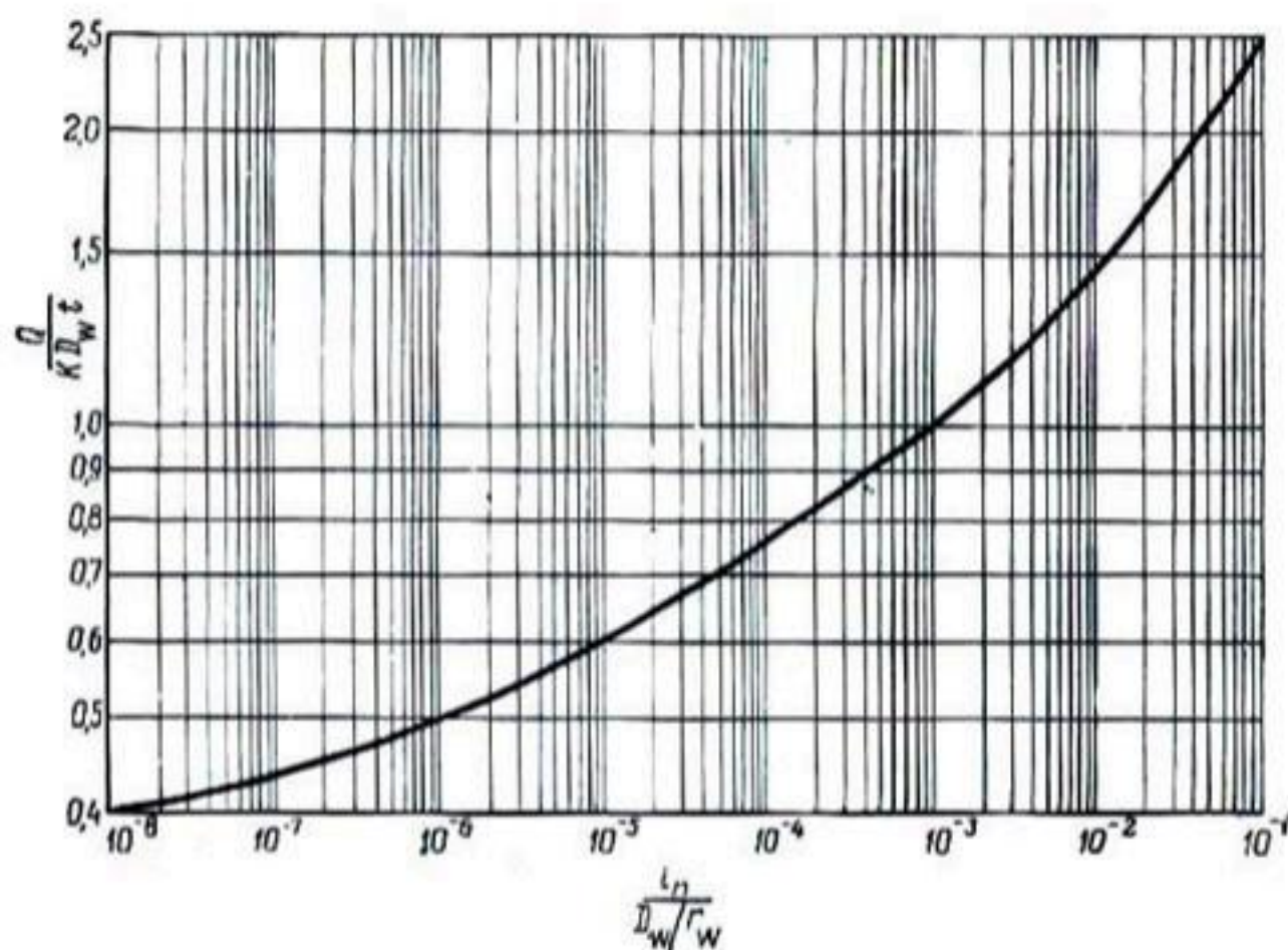
Рис. 104. Параметры расхода для горизонтально пополняемого артезианского колодца.
