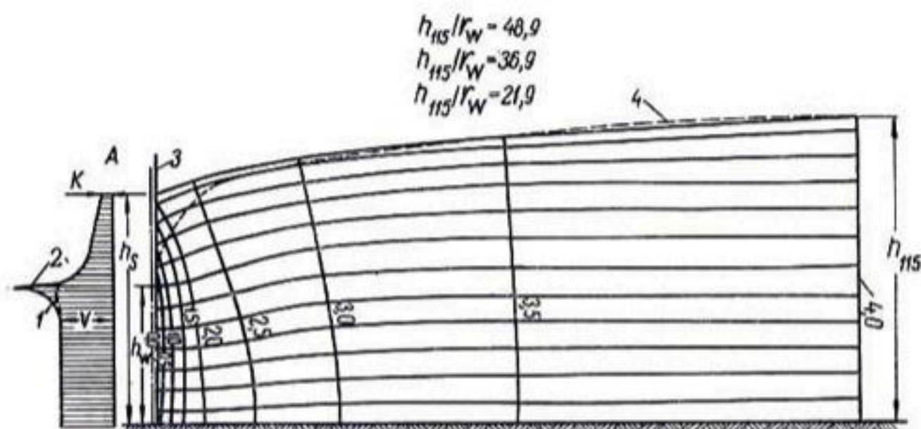
Рис. 99. Модель радиального потока к колодцу:
