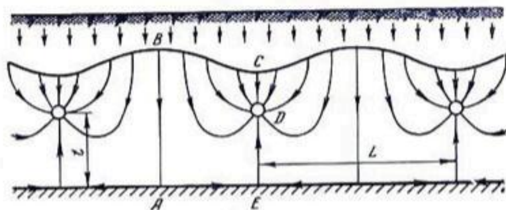
Рис. 43. Идеализованная модель потока при дренаже однородных почв.
