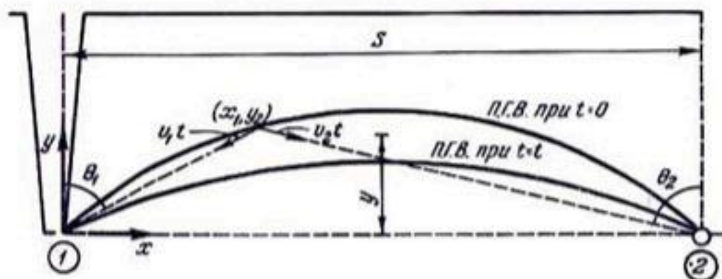
Рис. 41. Схема и обозначения, используемые при выводе уравнения Уолкера.
