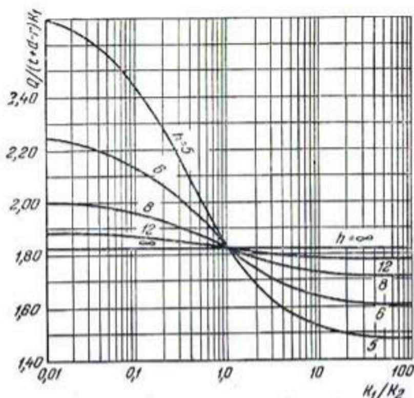
Рис. 85. Кривые зависимости величины Q/(t+d-r)k_1 от отношения k_1/k_2 ; если k_1 выражено в футах/сутки, а (t+d-r) — в футах, то фильтрационный расход на единицу длины дренажной трубки выражен в куб. футах/сутки на погон. фут. По Киркхему (1951).
