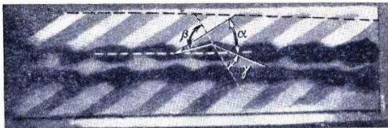
Рис. 118. Экспериментальное изучение потока через слоистый грунт. По Дахлеру (1933).
