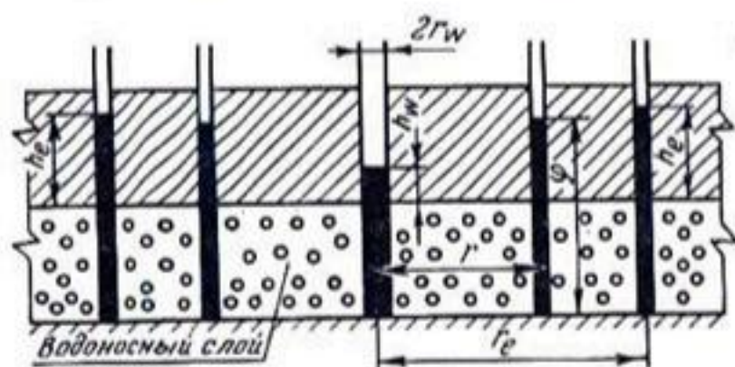
Рис. 71. Эскиз к задаче радиального потока в водоносном слое в направлении к цилиндрическому колодезю (решение этой задачи является основным для всех задач скопившейся воды).
