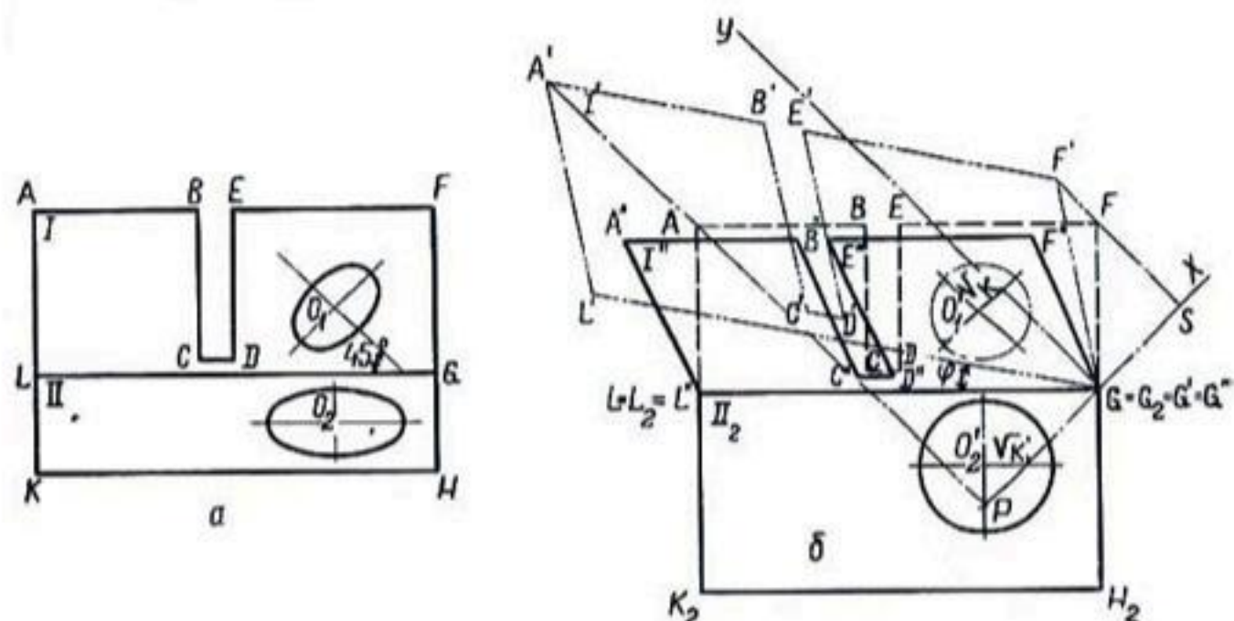
Рис. 121. Пример преобразования анизотропной двухслойной системы A в воображаемую изотропную двухслойную систему B .
