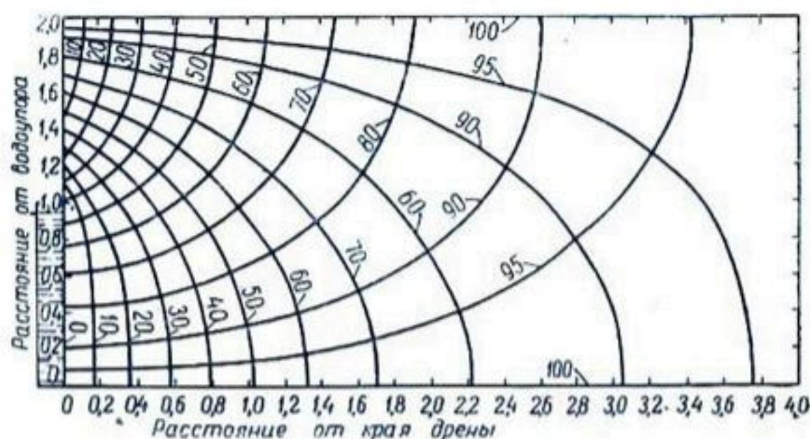
Рис. 93. Сетка токов для рисунка 92, когда уровень воды в дренах находится на расстоянии h/2 от поверхности почвы ( 2s=4h ). Сетка показана только между координатами x=0 и x=s . По Киркхему (1950b).
