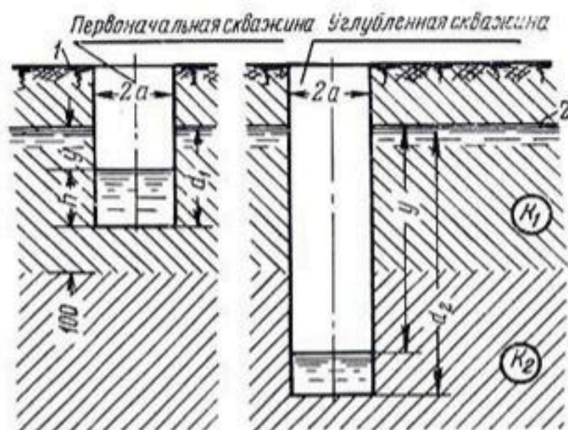
Рис. 193. Чертеж скважин, используемый Эрнстом при выводе формулы для слоистого грунта:
