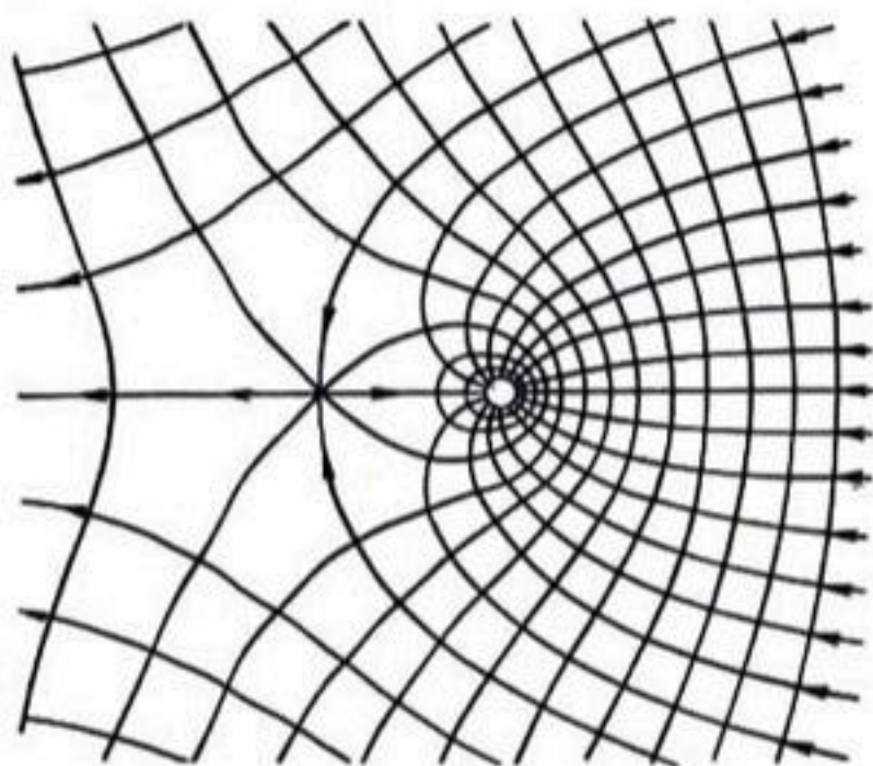
Рис. 108. Колодец в наклонном гидравлическом поле.
