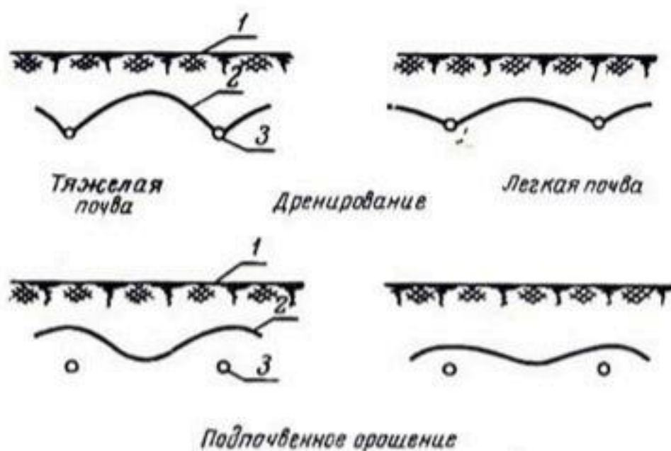
Рис. 232. Дренирование и подпочвенное орошение на малопроницаемых (тяжелых) и на хорошо проницаемых (легких) почвах:
