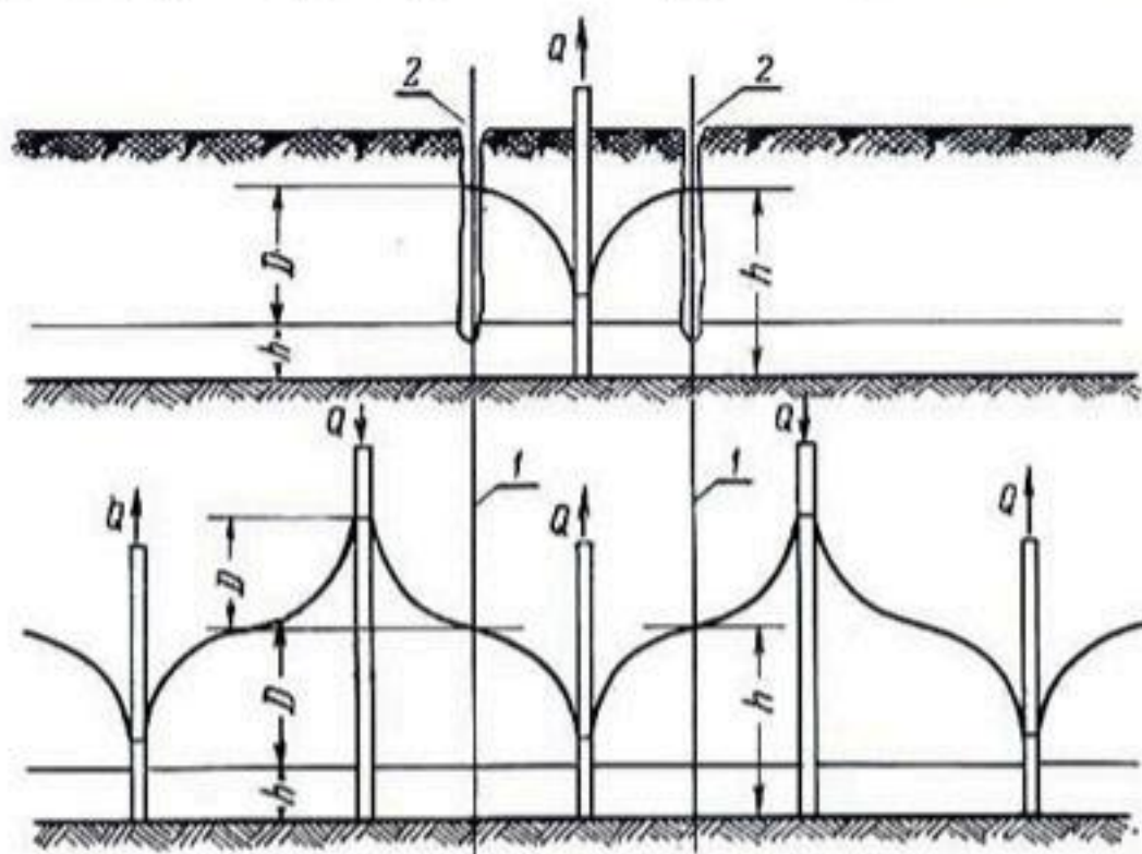
Рис. 112. Применение метода отражений к колодцу, находящемуся между двумя открытыми дренами: 1 — плоскость отражения 2 — открытая дрена.
