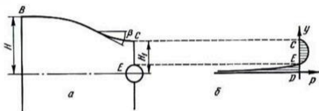
Рис. 64. Поверхность грунтовых вод (а) при d < d_0 и распределение давления (б) вдоль линии DEC .
