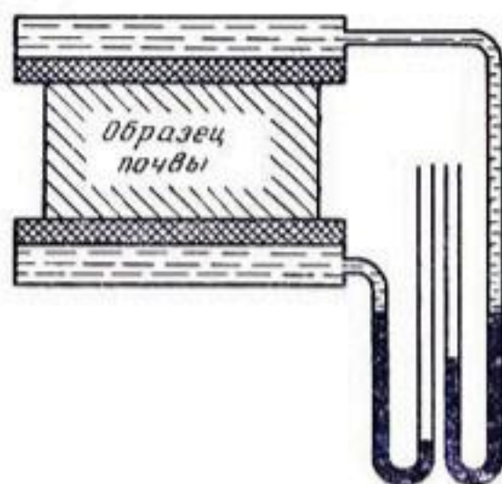
Рис. 22. Детали прибора для измерения гидравлической проводимости ненасыщенной почвы. Вода подается и извлекается под действием сосущей силы через ходы пористых пластинок.
