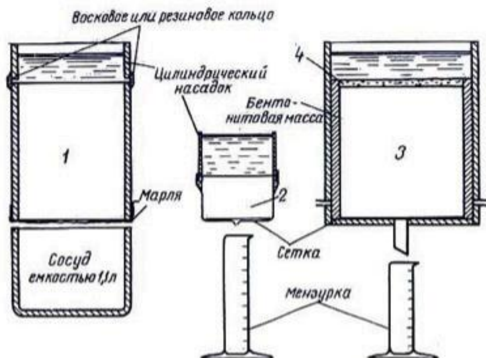
Рис. 184. Три метода монтирования и установки почвенных монолитов для определения проницаемости в лабораторных условиях:
