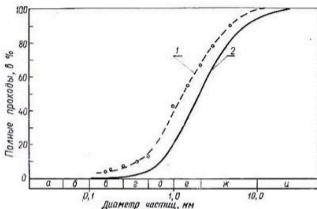
Рис. 154. Типичные гравийные фильтры, применявшиеся в долинах Импириал и Кочелла (штат Калифорния). Кривые гранулометрического состава фильтров:
