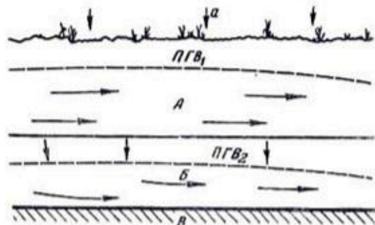
Рис. 30. Осадки a вызывают образование временной поверхности грунтовых вод ПГВ_1 в верхнем слое A , водопроницаемость которого больше, чем в нижнем слое B . В слое B может быть вторая поверхность грунтовых вод ПГВ_2 , которая иногда отходит от поверхности ПГВ_1 .
