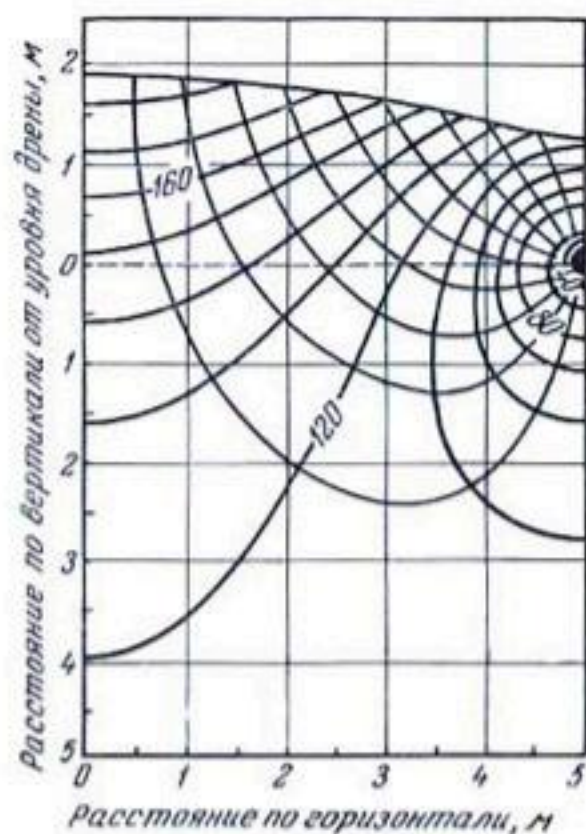
Рис. 45 и 46. Линии токов и эквипотенциали, полученные электромоде- лированием (по Чайлдсу).
