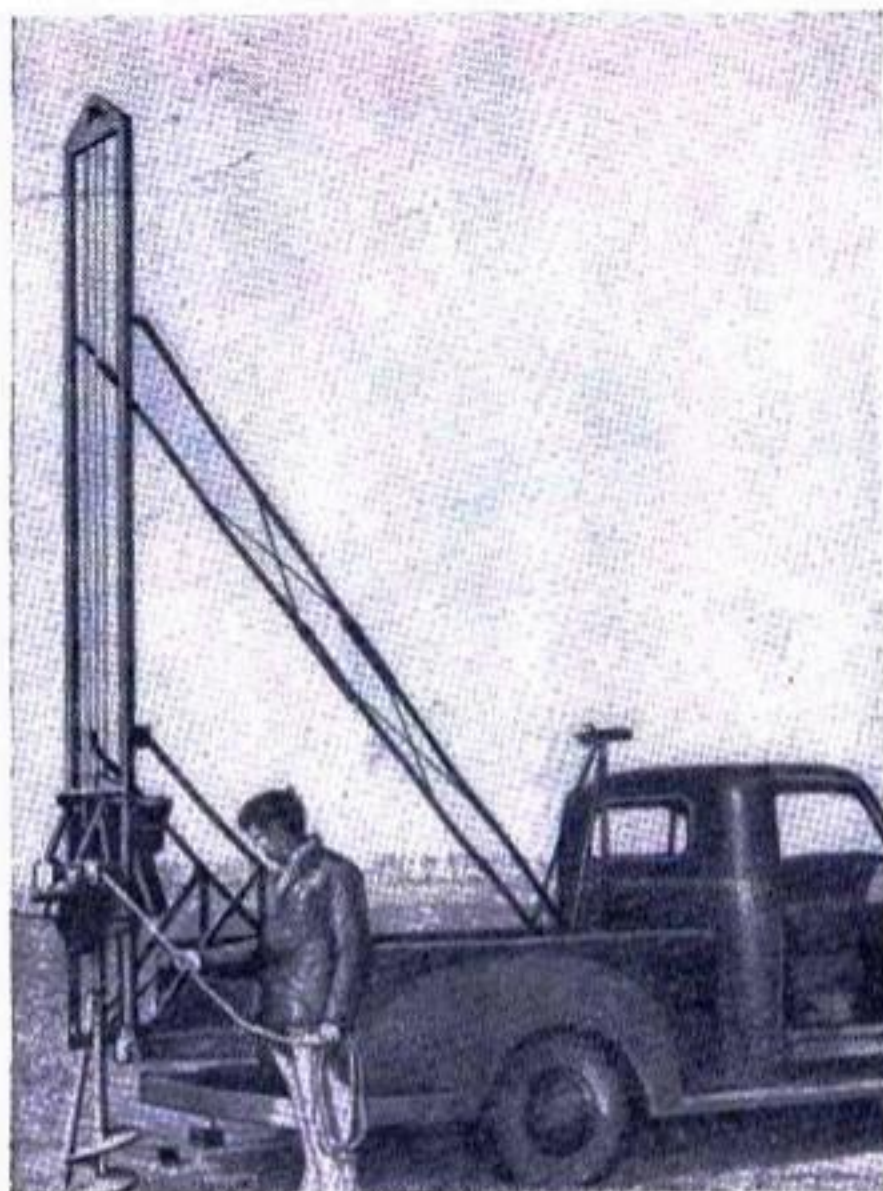
Рис. 200. Механический бур диаметром 305 мм, оборудованный двигателем мощностью 6 л. с. Бур имеет валы-удлинители, позволяющие брать образцы с глубины до 3 м.
