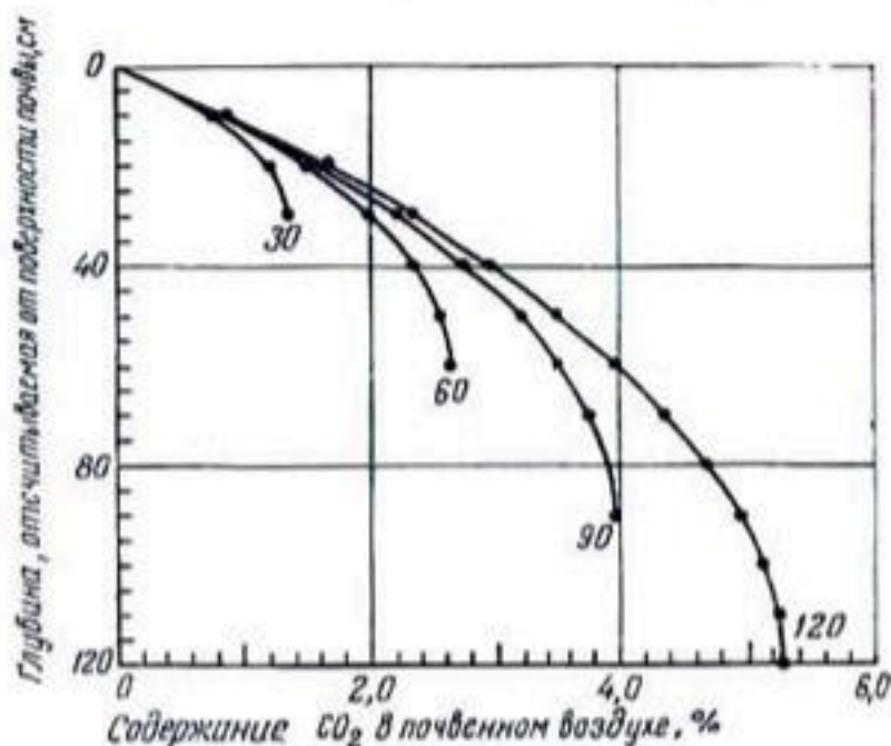
Рис. 207. Максимальное процентное содержание \text{CO}_2 на различных глубинах, подсчитанное по формуле p = p_0 - \alpha / (-Lz + z^2/2)^2 . По ван Бейвелу (1951).
