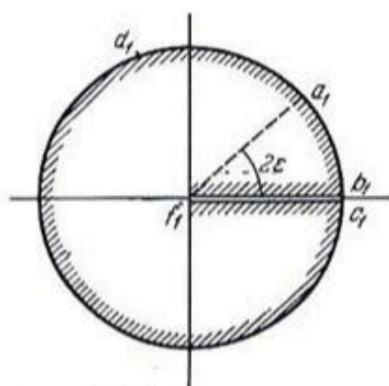
Рис. 60. Плоскость \omega_1 .
