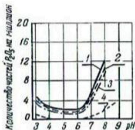
Рис. 222. Растворимость фосфора, добавляемого к хорошо дренируемой почве. По Локи, 1941 (цитируется по Мицуи, 1954):
