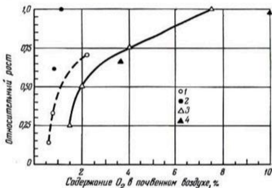
Рис. 204. Зависимость скорости роста различных видов растений от парциального давления кислорода при постоянной температуре. По Кэннону (1925): 1— Prozopis velutina , 20°; 2— Citrus sinensis , 27°; 3— Gossypium barbadense ; 4— Zea mays , 17°.
