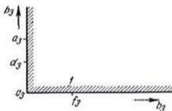
Рис. 62. Плоскость \omega_3 .
