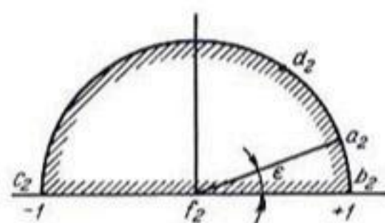
Рис. 61. Плоскость \omega_2 .
