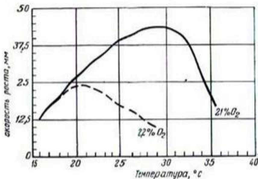
Рис. 203. Зависимость скорости роста корней хлопчатника от температуры (Кэнион, 1925).
