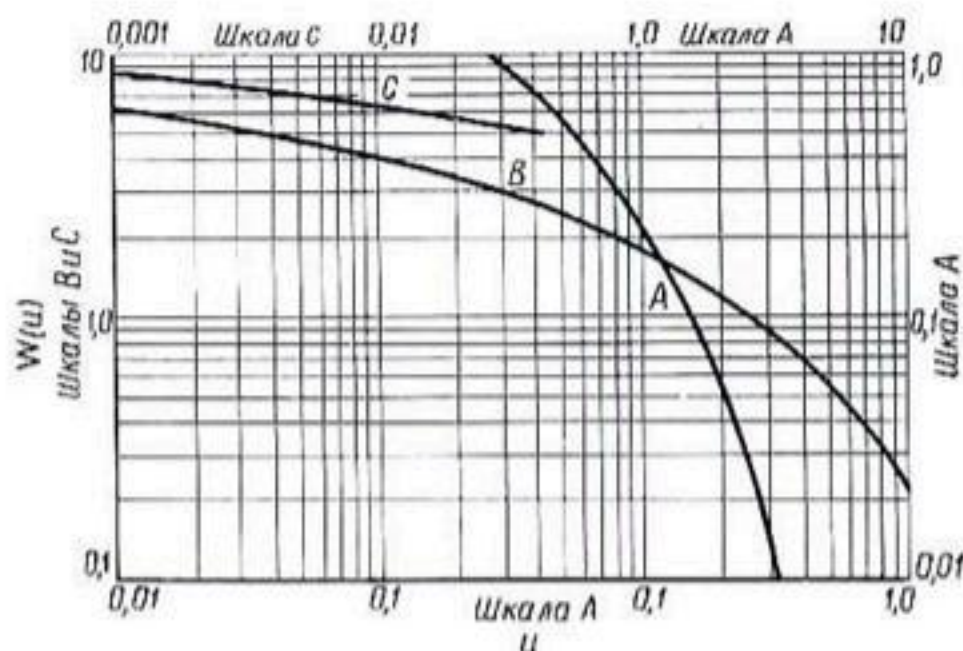
Рис. 105. Функция колодца.
