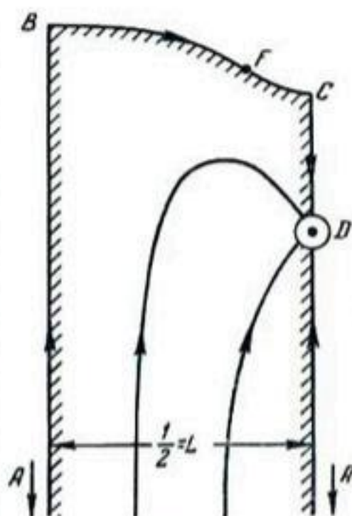
Рис. 57. Плоскость z .
