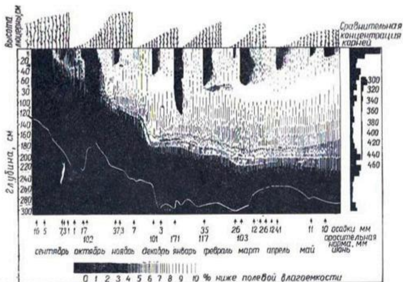
Рис. 231. На диаграмме показаны изменения влажности почвы, уровень грунтовых вод и толщина капиллярной каймы в период вегетации люцерны (Австралия). Указаны также количество осадков, поливная норма, высота стеблей люцерны и концентрация корней. Белая извилистая линия на черном фоне — поверхность грунтовых вод. По Весту (1933).
