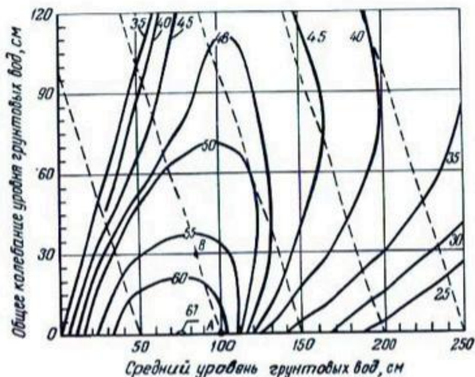
Рис. 215. Зависимость между урожаем ржи на песчаных почвах в 1949 г., средней глубиной уровня грунтовых вод и годовыми колебаниями этого уровня. Сплошные линии являются линиями одинаковых урожаев. Пунктирные линии связывают точки с одинаковым уровнем грунтовых вод (летом) и точки с различными уровнями (зимой). У точки A уровень 100 см является постоянным и летом, и зимой. В точке B средний уровень грунтовых вод равен 85 см, общее колебание составляет 30 см. Летом глубина равна 85 + 15 = 100 см, а зимой она составляет 85 - 15 = 70 см.
