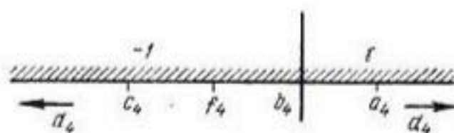
Рис. 63. Плоскость \zeta .
