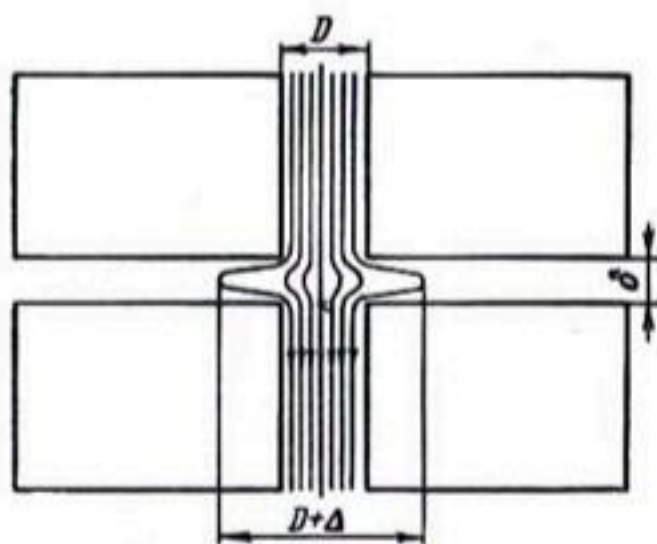
Рис. 21. Изображенное линиями тока движение через почвенные трещины показывает, что поперечные трещины являются малоэффективными в качестве проводников почвенной воды.
