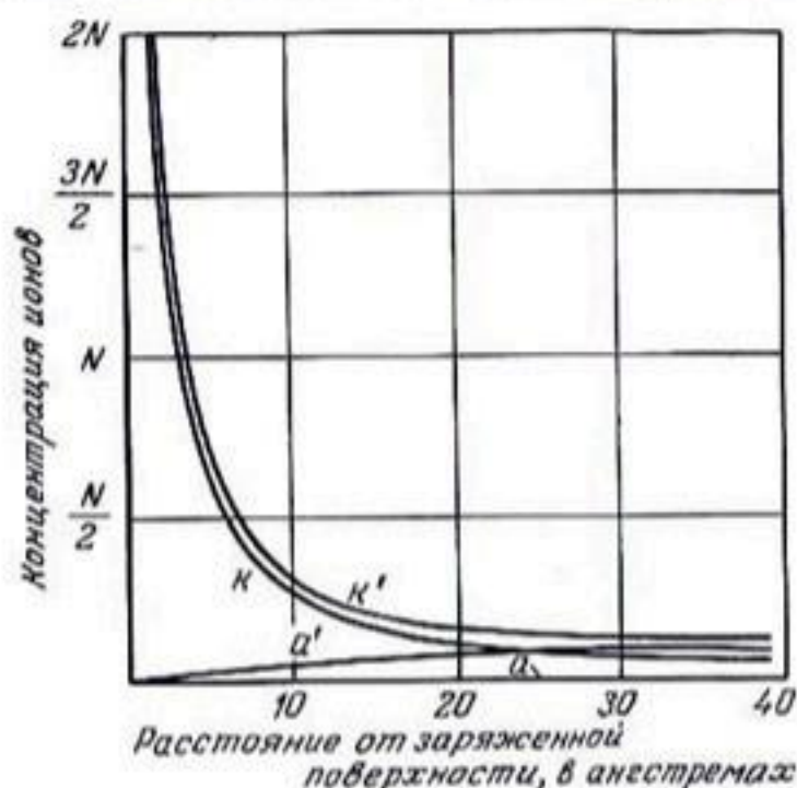
Рис. 7. Распределение ионов в слое Гу между двумя параллельными плоскостями монтмориллонитовых кристаллов с обменной базой 100 миллиэквивалентов на 100 г (расстояние между этими плоскостями 80 ангстрем). Так как слой является симметричным относительно средней плоскости, на чертеже показана только половина этого слоя. Кривая a , совпадающая с горизонтальной осью координат, показывает концентрацию анионов для пластинок, находящихся в растворе одновалентных ионов ( N/1000 ). Кривая k показывает концентрацию катионов. Кривые a' и k' построены для раствора одновалентных ионов ( N/10 ).
