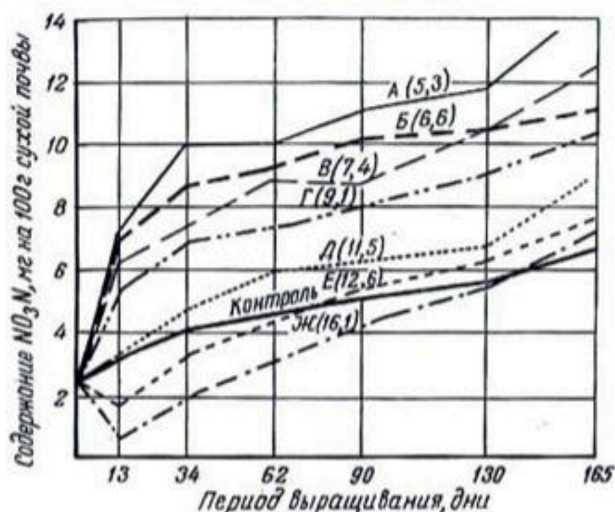
Рис. 220. Скорость минерализации органических веществ, добавляемых в хорошо дренируемую почву. Эта скорость характеризуется количеством освобожденного азота. По Шнори и Мицун, 1935 (цитируется по Мицун, 1954). Цифры в скобках обозначают отношение S/N .
