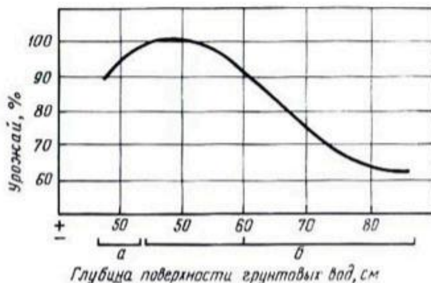
Рис. 235. Урожай гнацинта Невишность в зависимости от уровня грунтовых вод. По Главу (1938b): а — мелкий дюнный песок; б — крупный дюнный песок.
