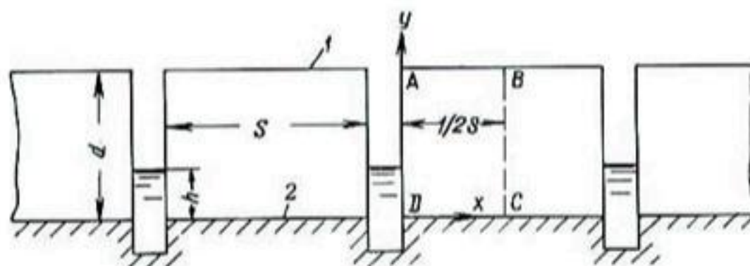
Рис. 125. Вертикальный разрез почвы, лежащей на непроницаемом слое и дренируемой канавами, расположенными на равном расстоянии друг от друга. По Киркхему (1950b): 1 — поверхность почвы; 2 — поверхность водоупора.
