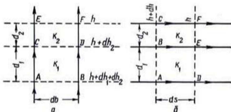
Рис. 115. Потенциальный поток в слоистом грунте: a — поток, перпендикулярный направлению слоистости; b — поток, параллельный направлению слоистости.
