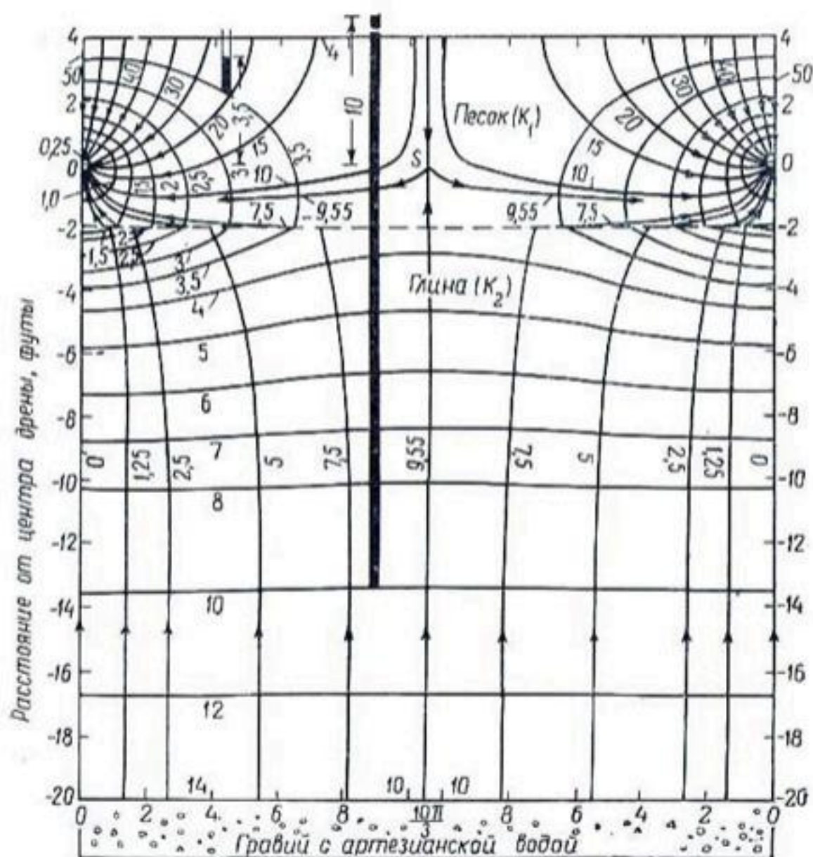
Рис. 91. Сетка токов в слоистом грунте (вверху — песок, внизу — глина и артезианский гравий). Прорыва артезианской воды на поверхность почвы нет, несмотря на то, что вода в пьезометре, доходящем до артезианского гравия, стоит на отметке 14 футов (4,3 м) выше труб, то есть на высоте 10 футов, считая от поверхности почвы. По Киркхему (1945).
