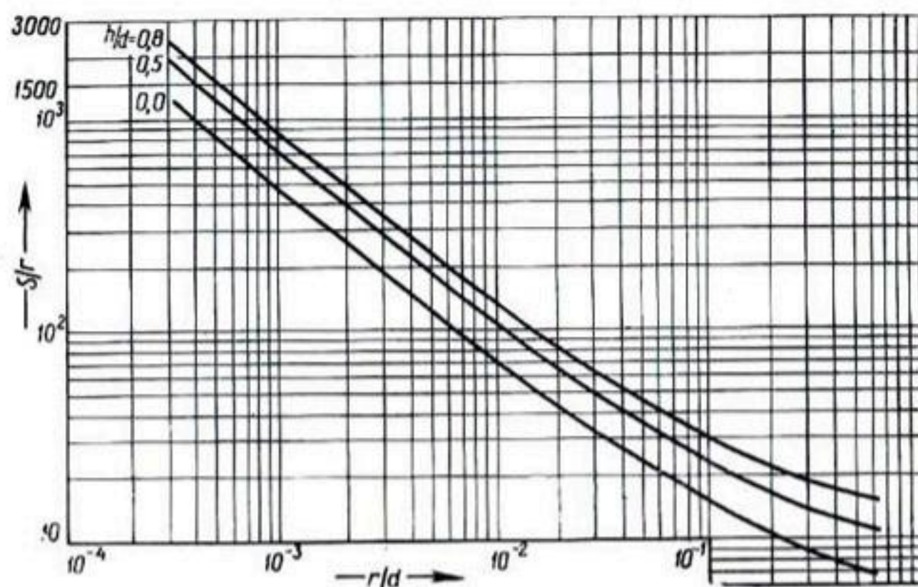
Рис. 133. Значения S/r в зависимости от r/d при h/d=0,8 ; 0,5 и 0,0; s=0 .
