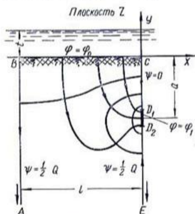
Рис. 129. Поток скопившейся воды к полосовому стоку, вокруг которого вычерчены эквипотенциалы, имеющие форму, близкую к эллиптической. По Энгелунду (1951).
