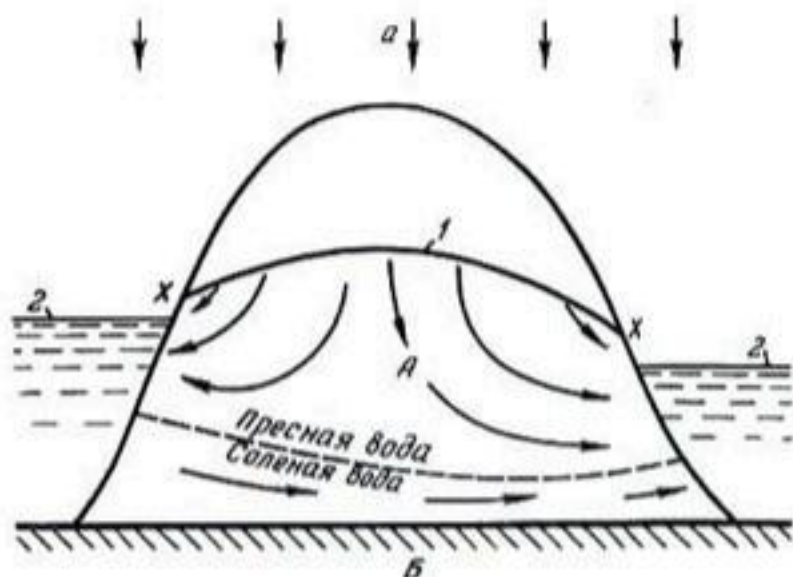
Рис. 29. Поверхность грунтовых вод в условиях устойчивых осадков a , когда пресные грунтовые воды оттесняют соленые грунтовые воды морского происхождения (линия Гибен-Герцберга):
