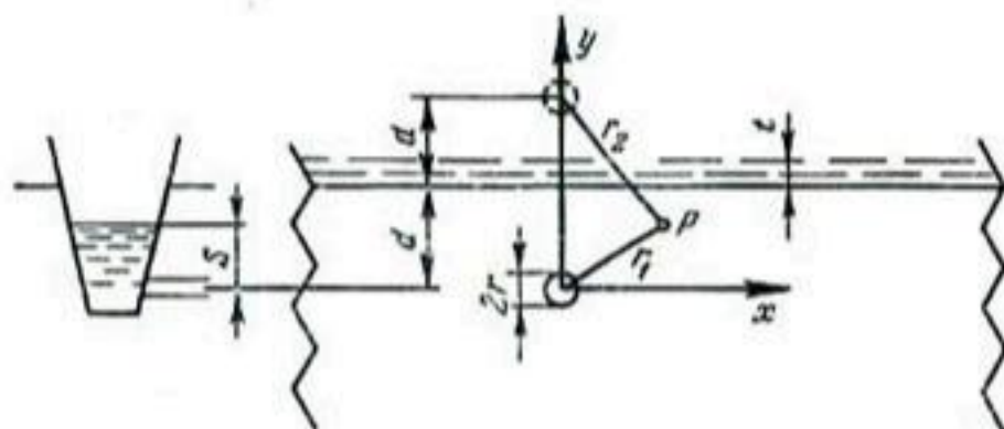
Рис. 72. Действительная и мнимая дренажные трубы при решении задачи скопившейся воды; непроницаемый слой, находящийся на большой глубине (здесь он не показан), не позволяет воде уходить из грунта, минуя дренажные трубы.
