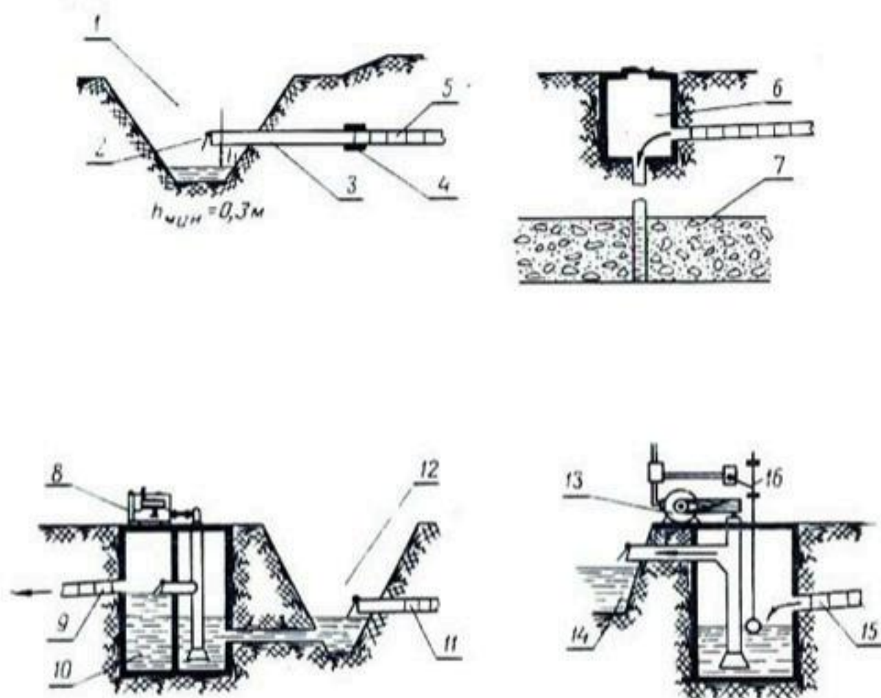
Рис. 137. Водовыпуски из гончарных дрен:
