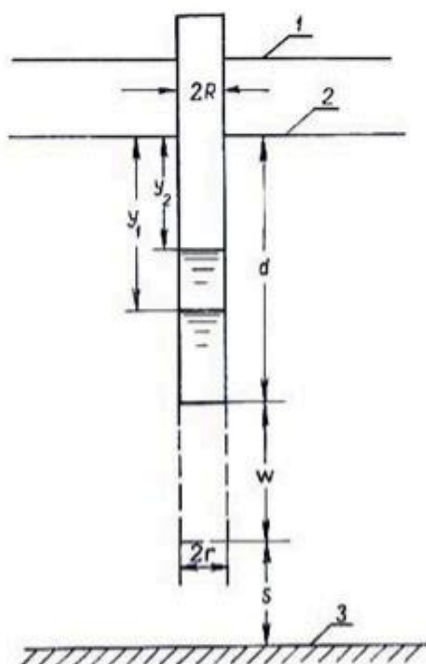
Рис. 131. Пьезометр в однородном грунте:
