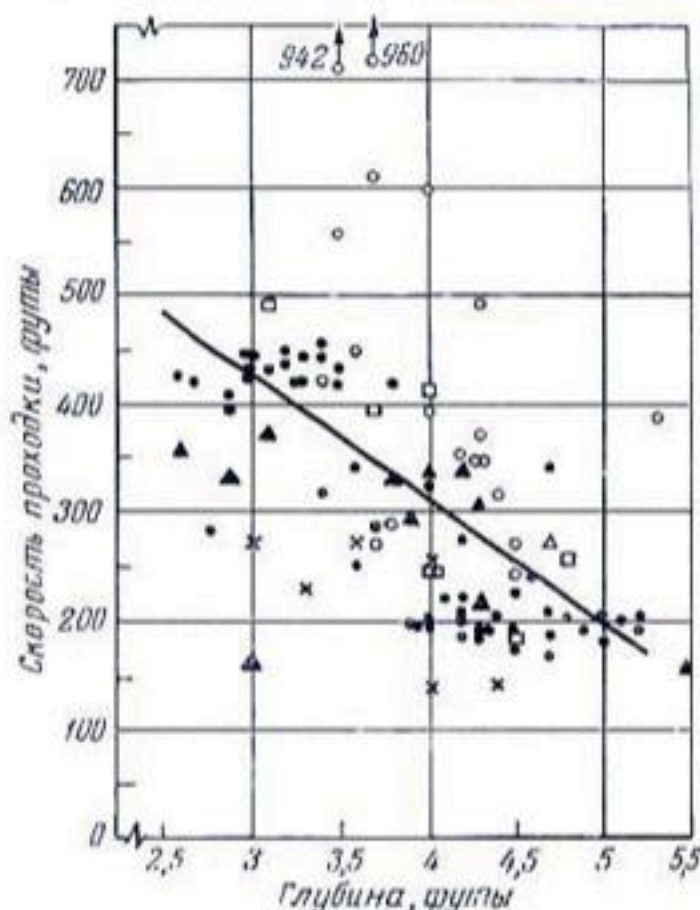
Рис. 142. Зависимость скорости проходки [фут/час] от глубины траншей. По данным Гича (1948), де Фриса (1951), Швэба и др. (1956). Разные обозначения точек на поле графика соответствуют разным машинам.
