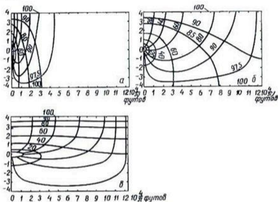
Рис. 127. Линии токов и эквипотенциали в анизотропном грунте, построенные для потока скопившейся воды в дренах эллиптической формы. Расстояние между дренами составляет 20 (4/π) футов (7,75 м). Непроницаемый слой находится в 8 футах (2,44 м), а центр гонимой дрены — в 4 футах (1,22 м) от поверхности почвы. Для графиков а, б и в отношение (k_h/k_v)^{1/2} = 1/4 , 1 и 4 соответственно.
