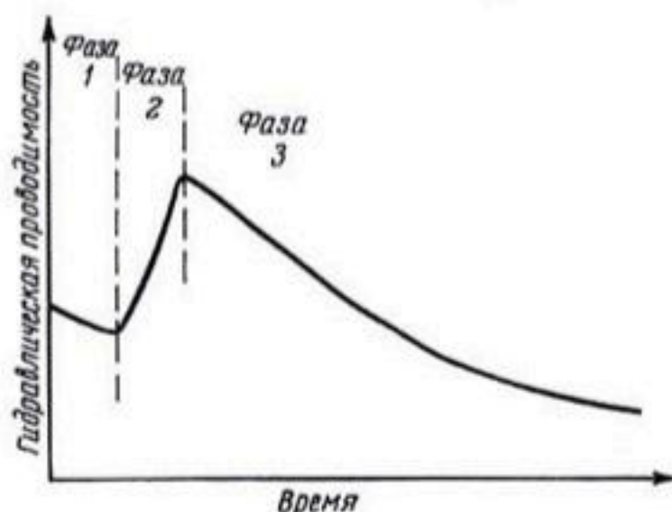
Рис. 179. Зависимость гидравлической проводимости почв от времени при их длительном затоплении. По Аллисону (1947).
