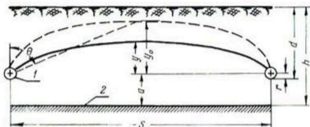
Рис. 172. Обозначение символов, используемых в формулах для определения расстояний между гончарными дренами:
