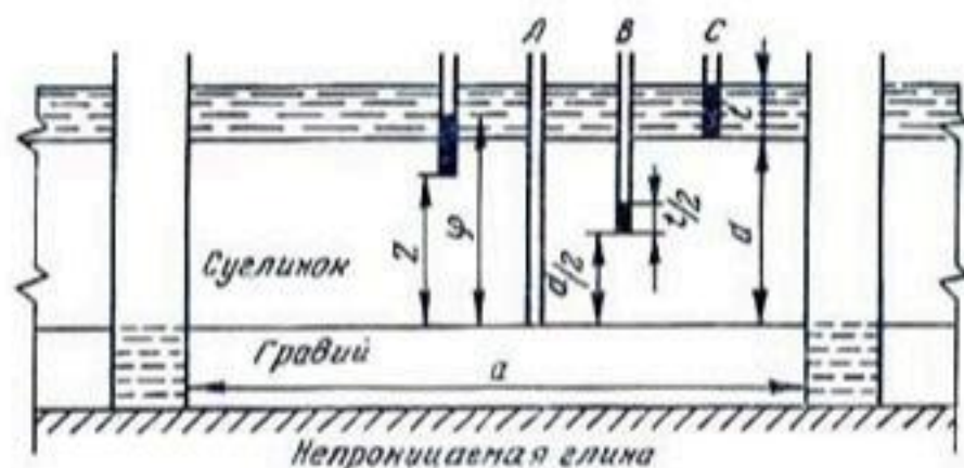
Рис. 70. Прямолинейное вертикальное просачивание воды в гравий, перерезанный дренажными каналами; пьезометры показывают давление воды и гидравлический напор.
