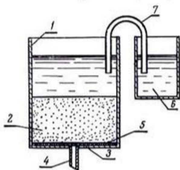
Рис. 185. Прибор для определения проницаемости образцов почв с нарушенной структурой. По Файерману (1944):
