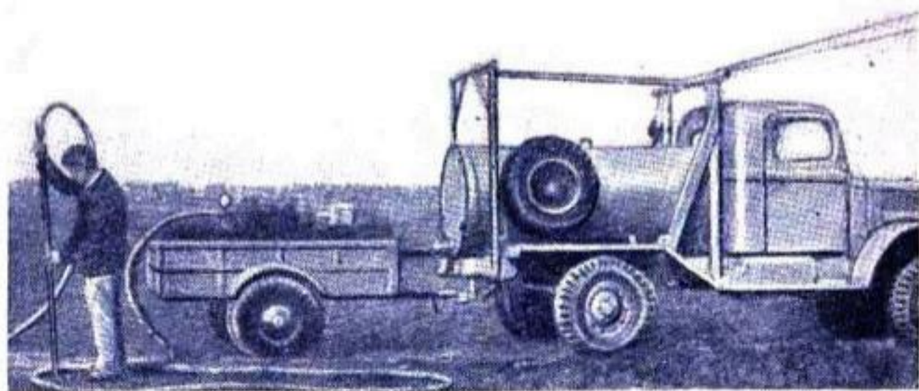
Рис. 201. Гидравлическое оборудование для установки в почву пьезометров диаметром 12,5 мм.
