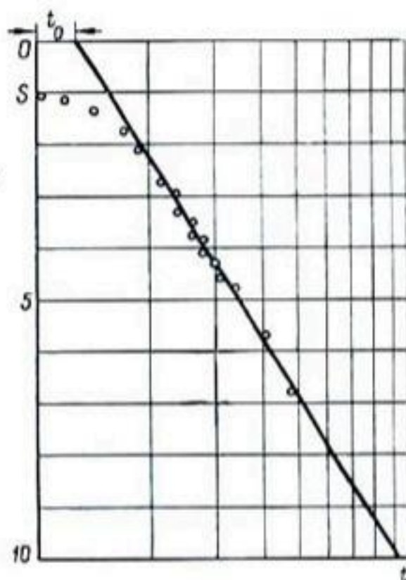
Рис. 107. Понижение в колодце как функция времени: s — понижение; t — время.
