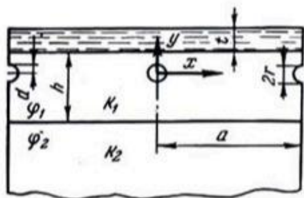
Рис. 82. На чертеже изображен ряд трубок, расположенных на одинаковом расстоянии друг от друга в грунте, состоящем из верхнего слоя с коэффициентом фильтрации k_1 и нижнего слоя с коэффициентом фильтрации k_2 .
