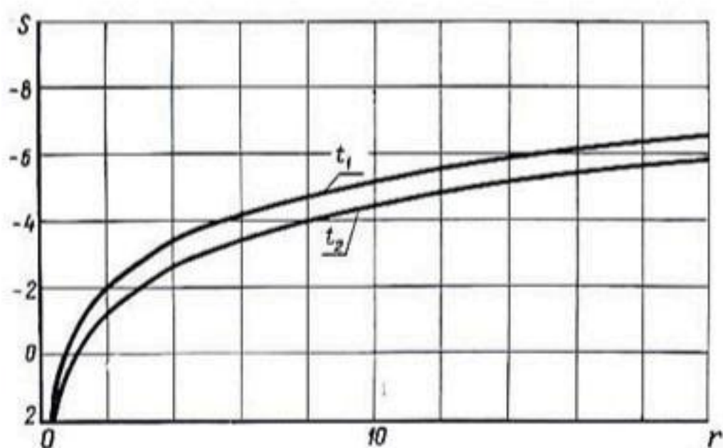
Рис. 106. Зависимость понижения от времени и расстояния от колодца:
