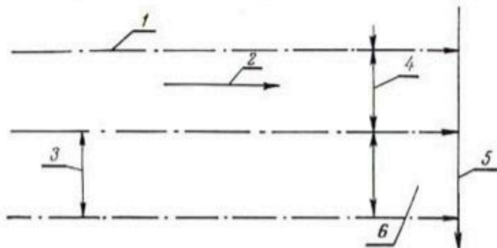
Рис. 170. Расположение каналов для регулирования уровня грунтовых вод (по Бошам):
