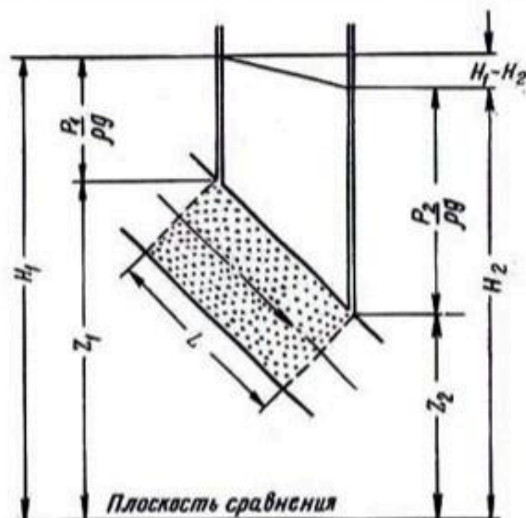
Рис. 175. Распределение гидравлического напора при однородном прямолинейном потоке в пористой среде. По Джекобу (1950).
