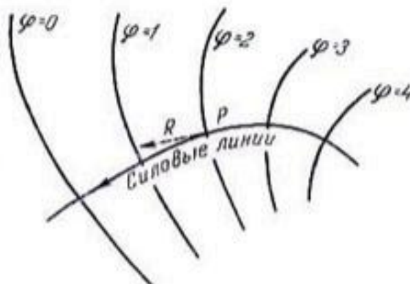
Рис. 17. На рисунке показано несколько эквипотенциалей, на основании которых могут быть получены силовые линии. R — направление равнодействующей силы в точке P , которое перпендикулярно к эквипотенциали, проходящей через эту точку.
