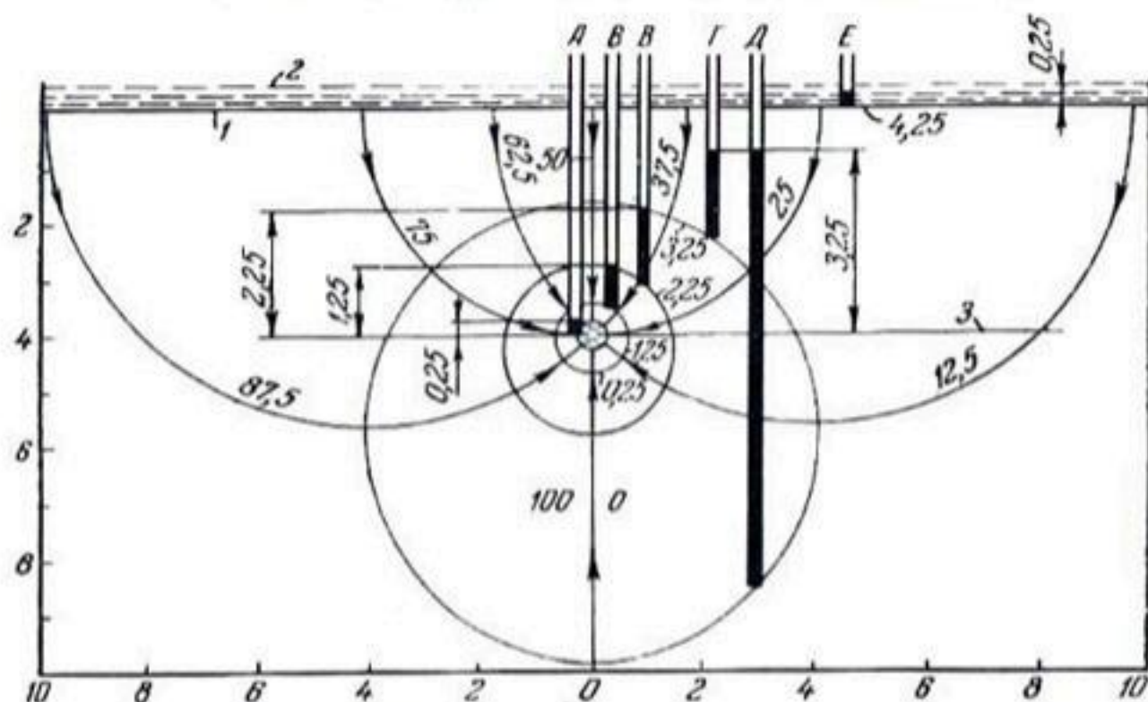
Рис. 77. Эквипотенциали и линии тока, построенные для дренажной трубы, проложенной в грунте, поверх которого находится скопившаяся вода. Грунт простирается неопределенно далеко как в горизонтальном, так и в вертикальном направлениях. Непроницаемый слой находится на большой глубине: 1 — поверхность грунта; 2 — скопившаяся вода; 3 — пьезометр; 4 — уровень отсчета.
