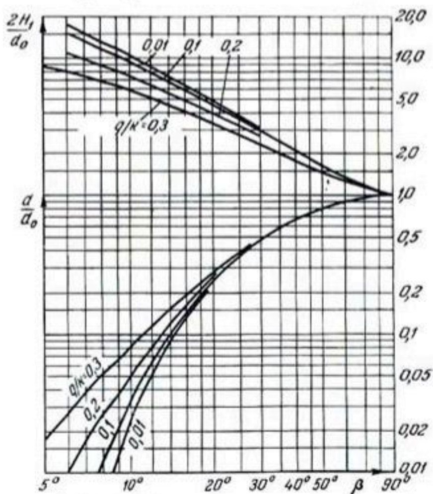
Рис. 68. \frac{d}{d_0} и \frac{2H_1}{d_0} как функции величин \beta и \frac{q}{k} .
