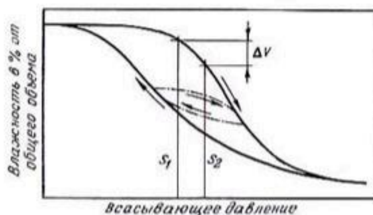
Рис. 5. Кривая влажности в несжимающейся почве. Стрелки показывают, происходит ли высыхание или увлажнение почвы. Штрих-пунктирной кривой показана петля внутреннего, или частичного, гистерезиса.
