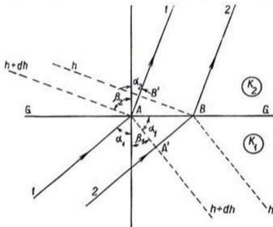
Рис. 120. Рефракция на границе двух однородных изотропных слоев с коэффициентами фильтрации k_1 и k_2 ( k_2 < k_1 ).
