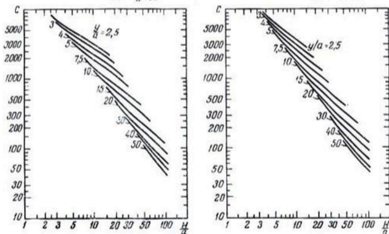
Рис. 188. Графики, облегчающие нахождение решения по формуле Эрнста (по Маасленду и Хаскью, 1957):
