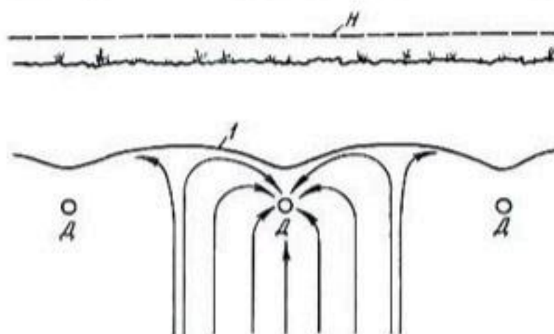
Рис. 27. Поверхность грунтовых вод I поддерживается на определенном уровне за счет артезианской воды с пьезометрической поверхностью H при наличии дренажной системы D .
