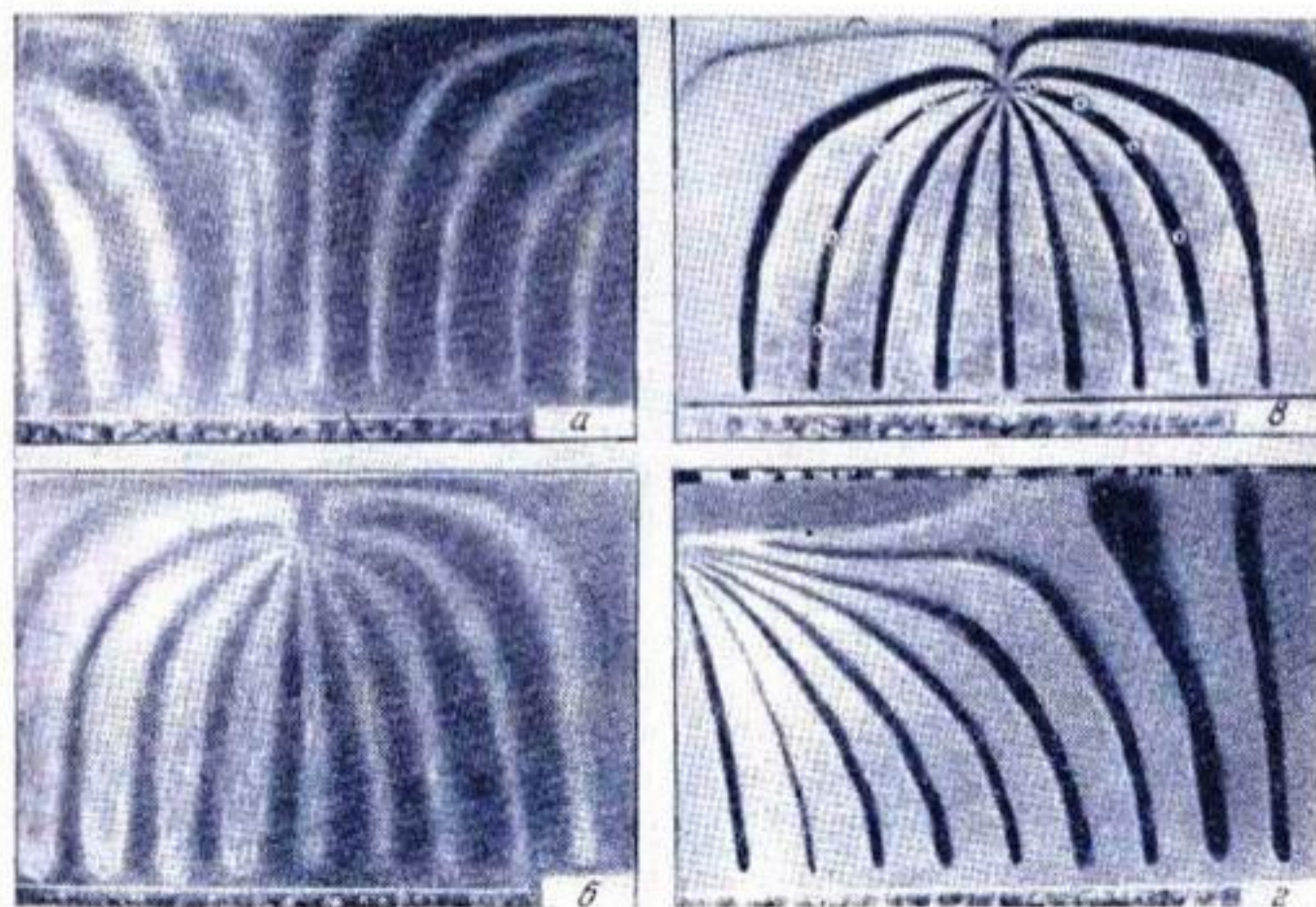
Рис. 89. Испытания на моделях в резервуаре с песком со стеклянной передней стенкой. Линии токов обусловлены артезианским давлением в водоносном пласте (галька ниже песка). По Киркхему (1940а).
