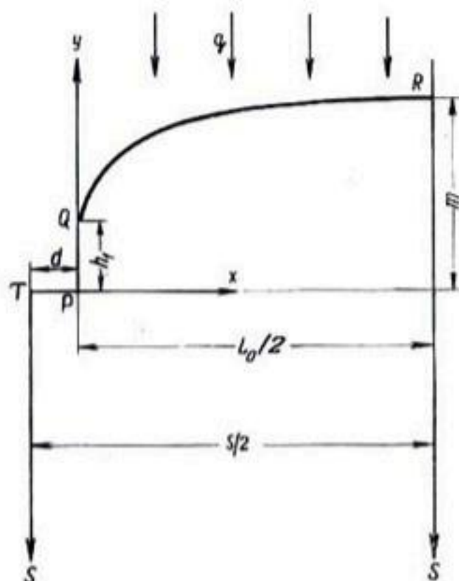
Рис. 124. Установившийся поток к открытым дренам прямоугольного сечения в среде, ограниченной с одной стороны. Непроницаемый слой находится ниже дрена на очень большой глубине или отсутствует совсем. Ширина траншей равна 2d . По ван Демтеру (1950).
