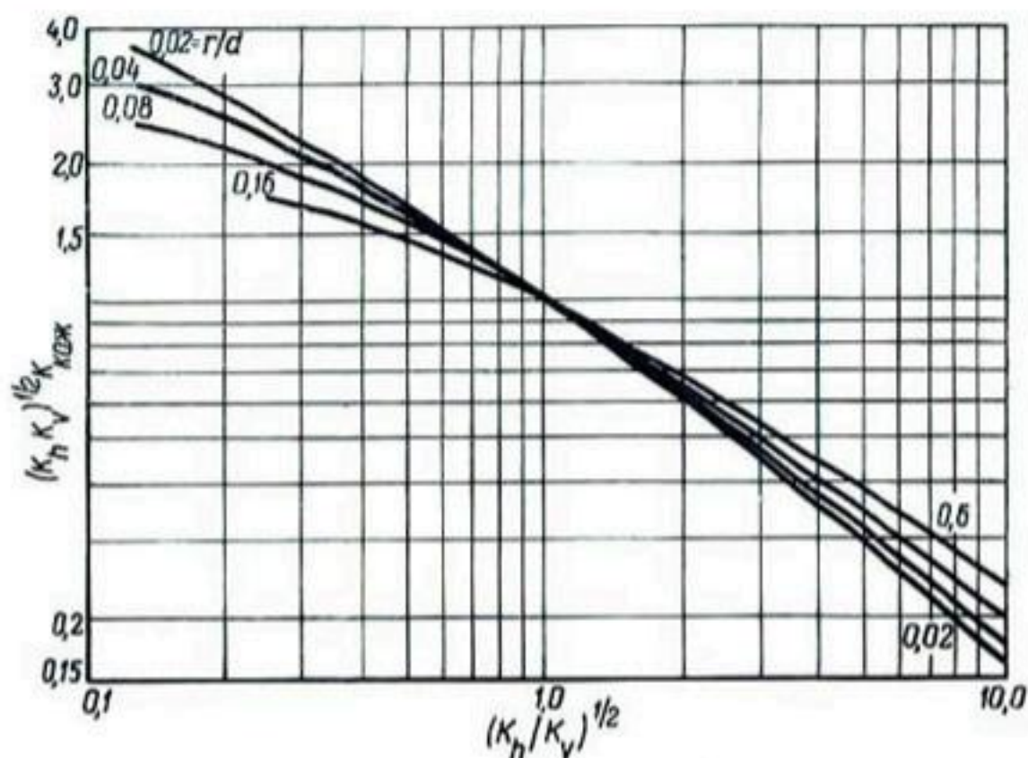
Рис. 134. Зависимость отношения (k_h k_v)^{1/2} / k_{каж} от величины (k_h / k_v)^{1/2} . Графики построены для буровых скважин, у которых отношение r/d равно 0,16; 0,08; 0,04; 0,02 ( h/d=0,5 , а s=0 ).
