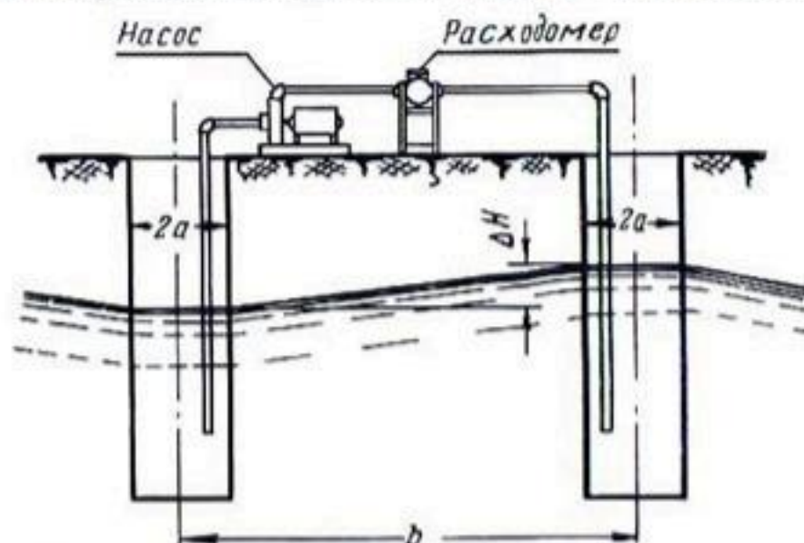
Рис. 194. Чертеж для разъяснения метода двух колодцев. По Чайлдсу и др. (1953).
