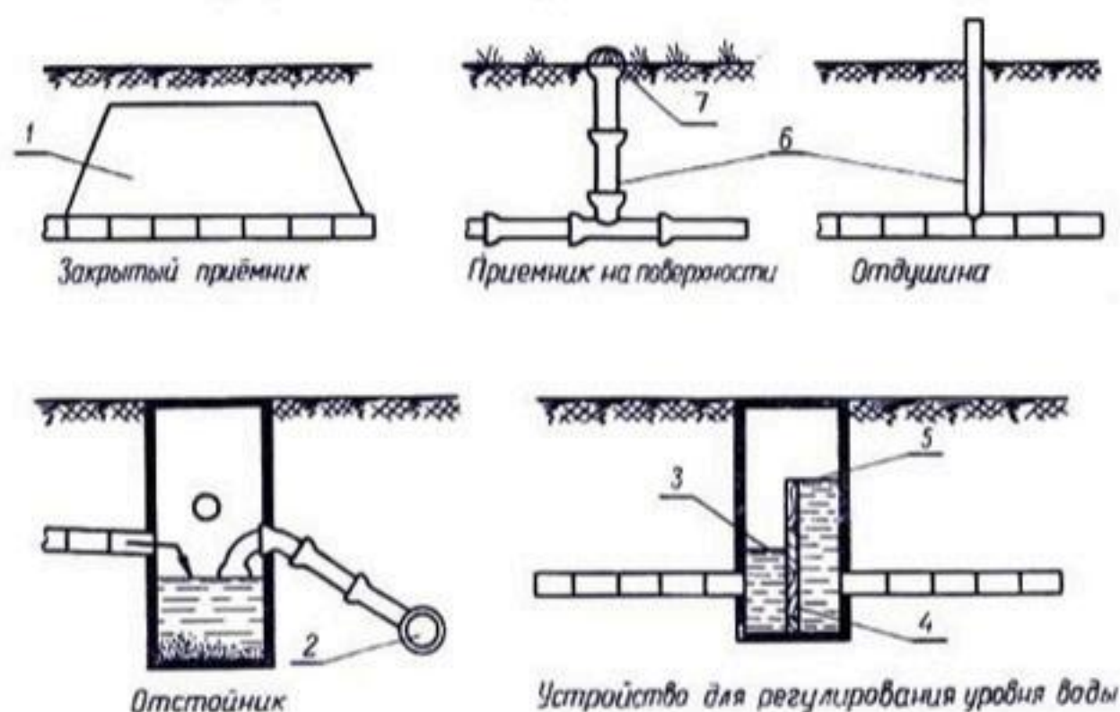
Рис. 141. Специальные устройства для гончарных дренажей:
