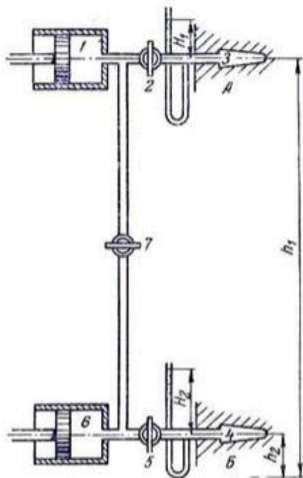
Рис. 18. Схема прибора для иллюстрации того, как измеряется гидравлический потенциал почвенной воды:
