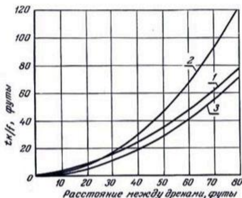
Рис. 42. Графики зависимости между tk/f и расстоянием между дренами, построенные по двум уравнениям Гловера и на основе приближенного решения Киркхема и Гаскелла (подсчитано для падения уровня грунтовых вод на один фут посередине между открытыми каналами глубиной 5 футов, доходящими до непроницаемого слоя):
