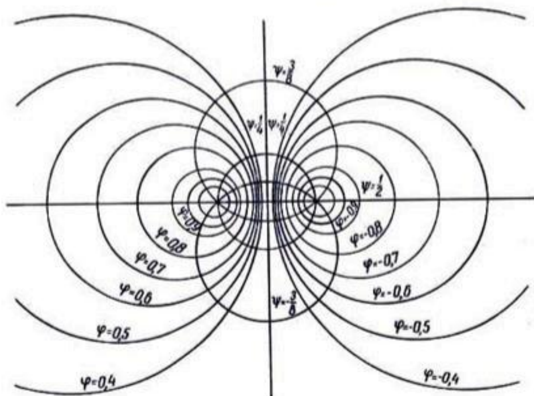
Рис. 109. Модель потока для колодцев пополнения и расхода.
