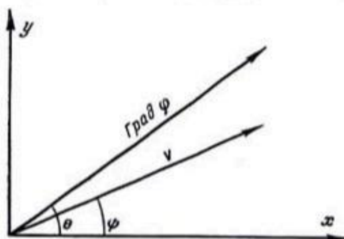
Рис. 20. Несовпадение направлений градиента потенциала и обусловленной им скорости потока в анизотропной среде.
