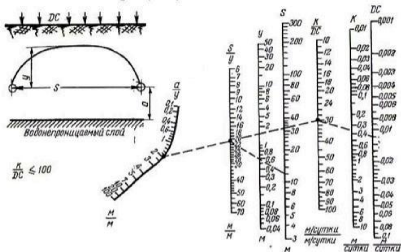
Рис. 173. Номограмма для определения расстояния между гончарными дренами при K/DC \leq 100 (по Виссеру). Под шкалами номограммы указаны размерности величин, отложенных на этих шкалах.
