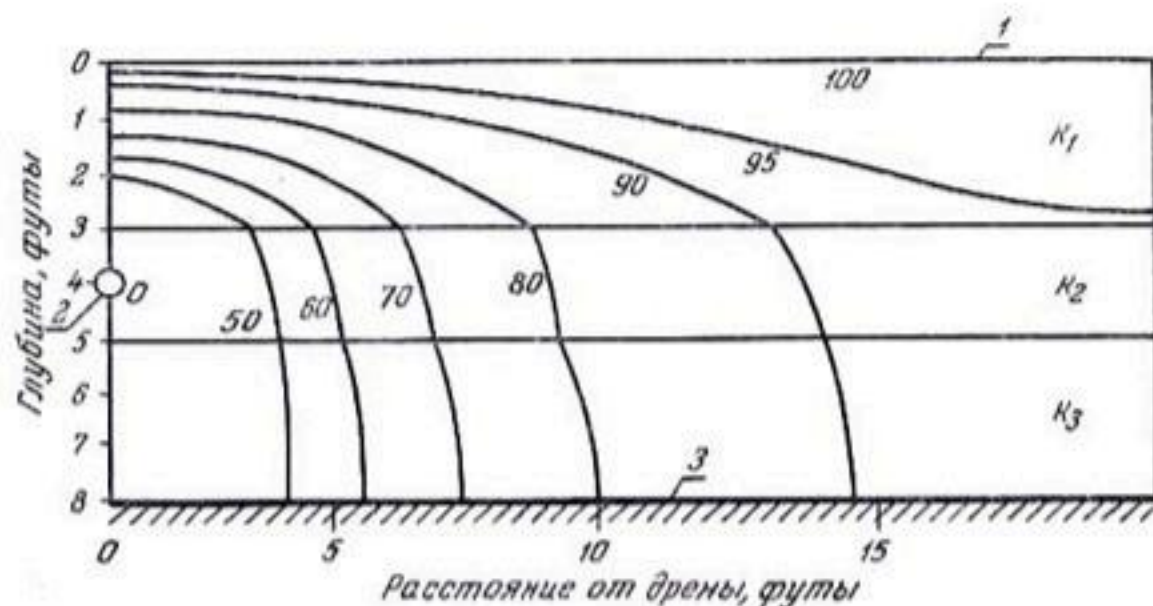
Рис. 87. Распределение гидравлического напора в трехслойном грунте при расположении дренажных труб в наиболее проницаемом слое с гидравлической проводимостью k_2 . Здесь k_1 = k_3 , а k_2 = 4k_1 . По Лютину (1953):
