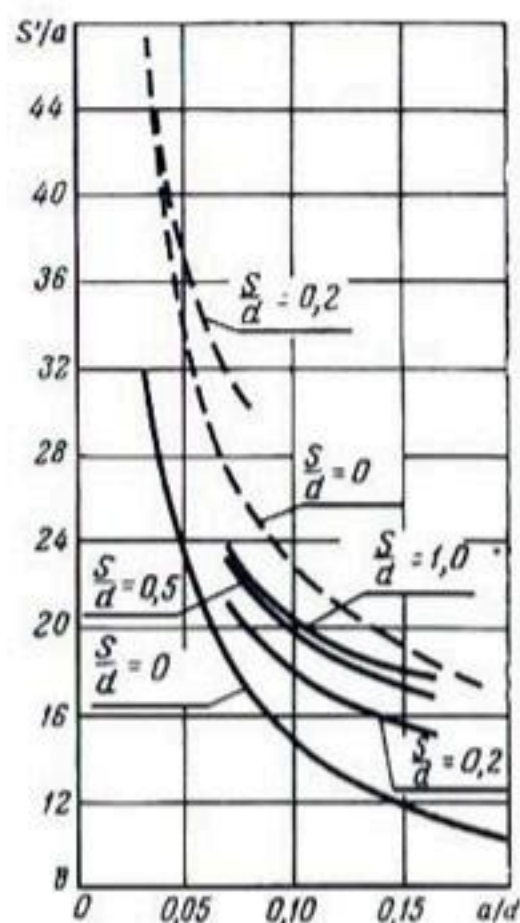
Рис. 191. Графики зависимости расстояния S' от отношения a/d , построенные для различных отношений s/d (по Киркхему и ван Гейвелу, 1949): пунктирные линии — скважина наполовину заполнена водой ( h=d/2 , t=0 ); сплошные линии — скважина пустая ( h=d , t=0 ).
