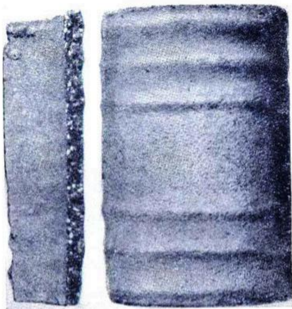
Рис. 149. Дренажная труба очень хорошего качества (диаметр трубы 15,2 см).
