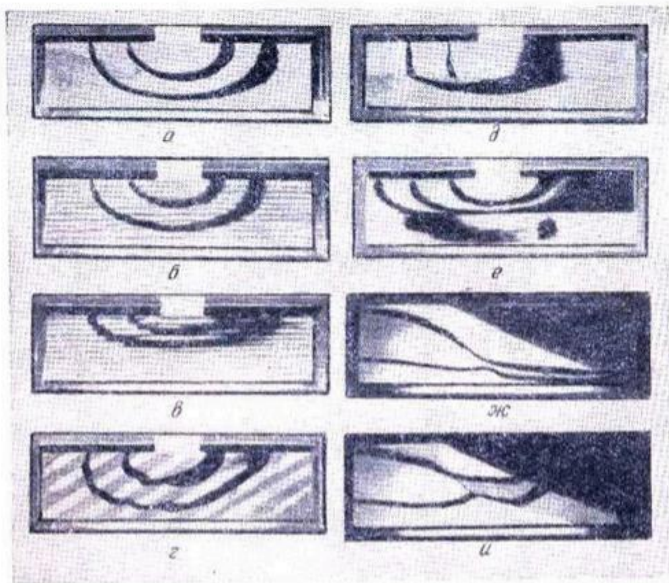
Рис. 119. Модельные испытания в песчаных лотках (по Шаффернаку, 1933): а — движение грунтовых вод в изотропном грунте у основания плотины; б — то же, что и а, но для равномерно перемежающихся слоев; в — то же, что и б, но при большом различии коэффициентов фильтрации слоев; г — асимметричные линии тока при негоризонтальном залегании слоев; д — движение воды у основания плотины в слабопроницаемом слое, лежащем на слое с большой проницаемостью; е — то же, что и д, но слои расположены в обратном порядке; ж — линии тока грунтовых вод в теле земной плотины (залегание слоев негоризонтальное); з — то же, что и ж, но при другом расположении слоев.
