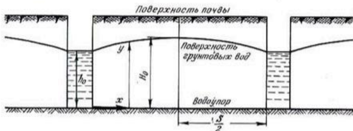
Рис. 33. Схема и обозначения, употребляемые при выводе эллиптического уравнения.
