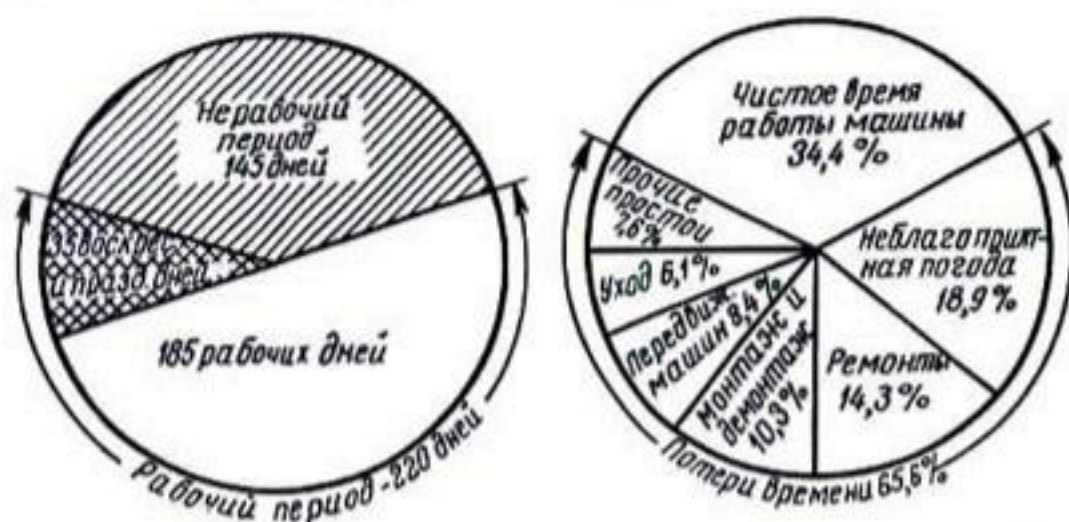
Рис. 143. Годовое использование и потери времени при эксплуатации тракторных машин, работающих в условиях штатов Айова и Миннесота. По данным Швэба и др. (1956).
