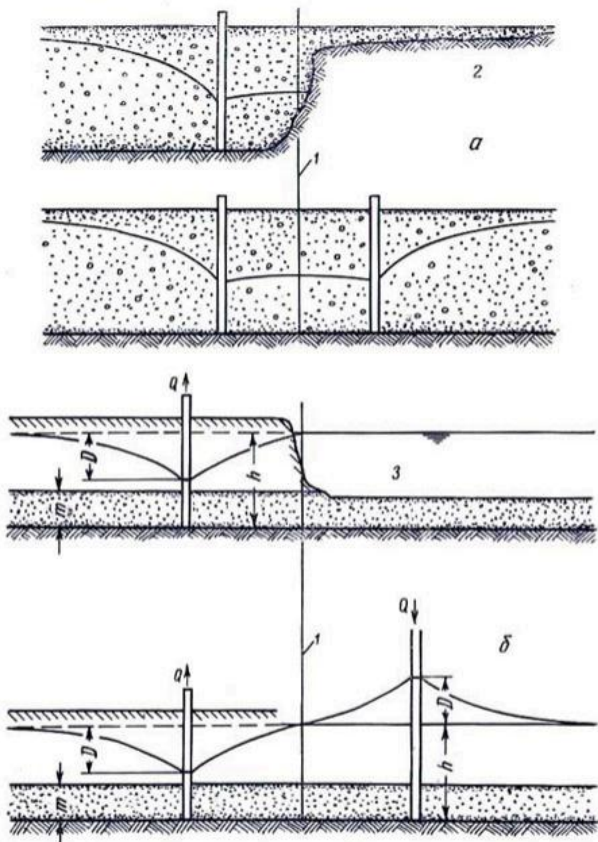
Рис. 111. Применение метода отражений:
