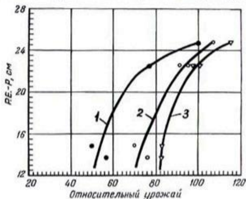
Рис. 216. Зависимость относительных урожаев яровых хлебных злаков от разности P. E. - P. , где P — осадки:
