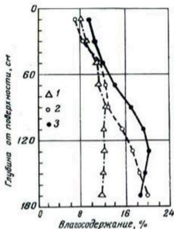
Рис. 210. Содержание влаги на различной глубине после уборки в сентябре 1949 г. люцерны (1), озимой (2) и яровой (3) пшеницы на участках с глинистой почвой, содержащей 20% частиц размером меньше 2 \mu . По Морелу и Ричеру (1953). Уменьшение содержания влаги на глубине ниже 130 см под яровой пшеницей объясняется уменьшением содержания глины.
