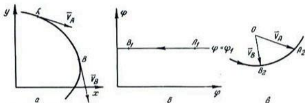
Рис. 55. Изображение плоскости z , плоскости w и годографа линии тока.
