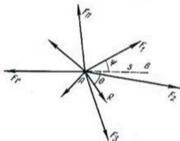
Рис. 16. Изображение сил, поясняющее обусловленный ими потенциал.
