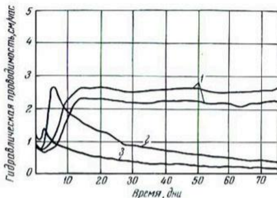
Рис. 180. Влияние микроорганизмов на гидравлическую проводимость суглинки при продолжительном затоплении. По Аллисону (1947):
