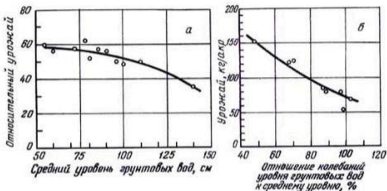
Рис. 217. Зависимость урожая земляники (кг/агр), полученного на песчаной почве, от положения поверхности грунтовых вод (по Виссеру, 1948): например, колебание уровня, равное 80%, означает, что средняя глубина h см уменьшается до 0,6 h см зимой и увеличивается до 1,4 h см летом; в большинстве случаев глубина h в опытах была приблизительно равна 70 см.
