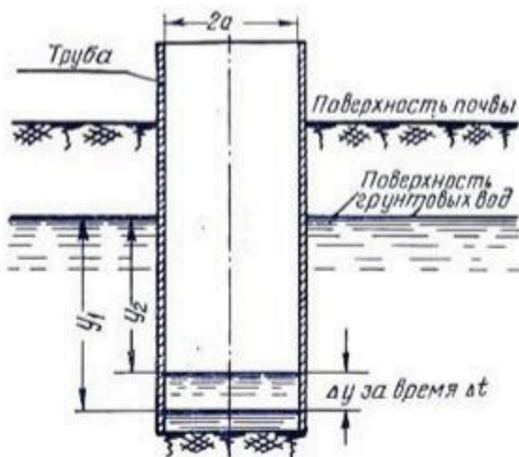
Рис. 198. Чертеж, служащий для объяснения трубчатого метода Киркхема. По Фриверту и Киркхему (1948).
