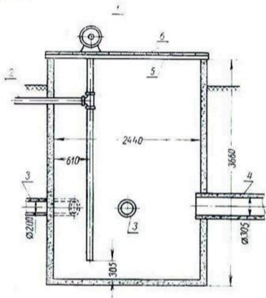
Рис. 161. Водовыпуск из дрен (долина Имбирнал):
