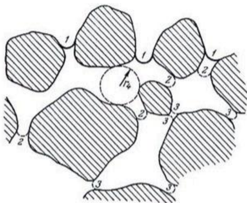
Рис. 4. Стадии изменения содержания влаги в несжимающейся почве. Положения водно-воздушной поверхности раздела, соответствующие каждой стадии, указаны цифрами.
