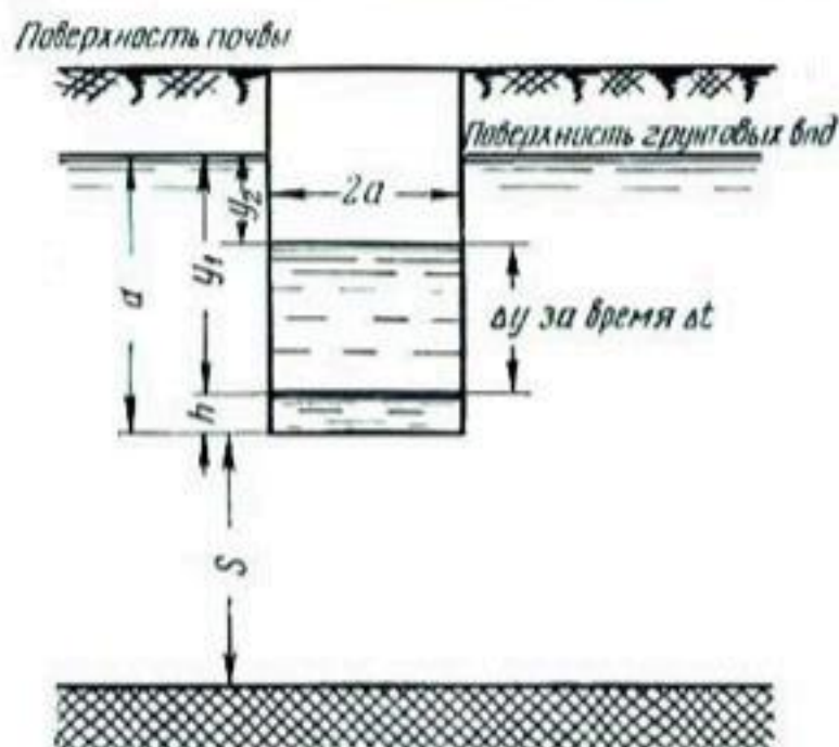
Рис. 187. Скважина в однородном грунте, не используемая при определении водопроницаемости.
