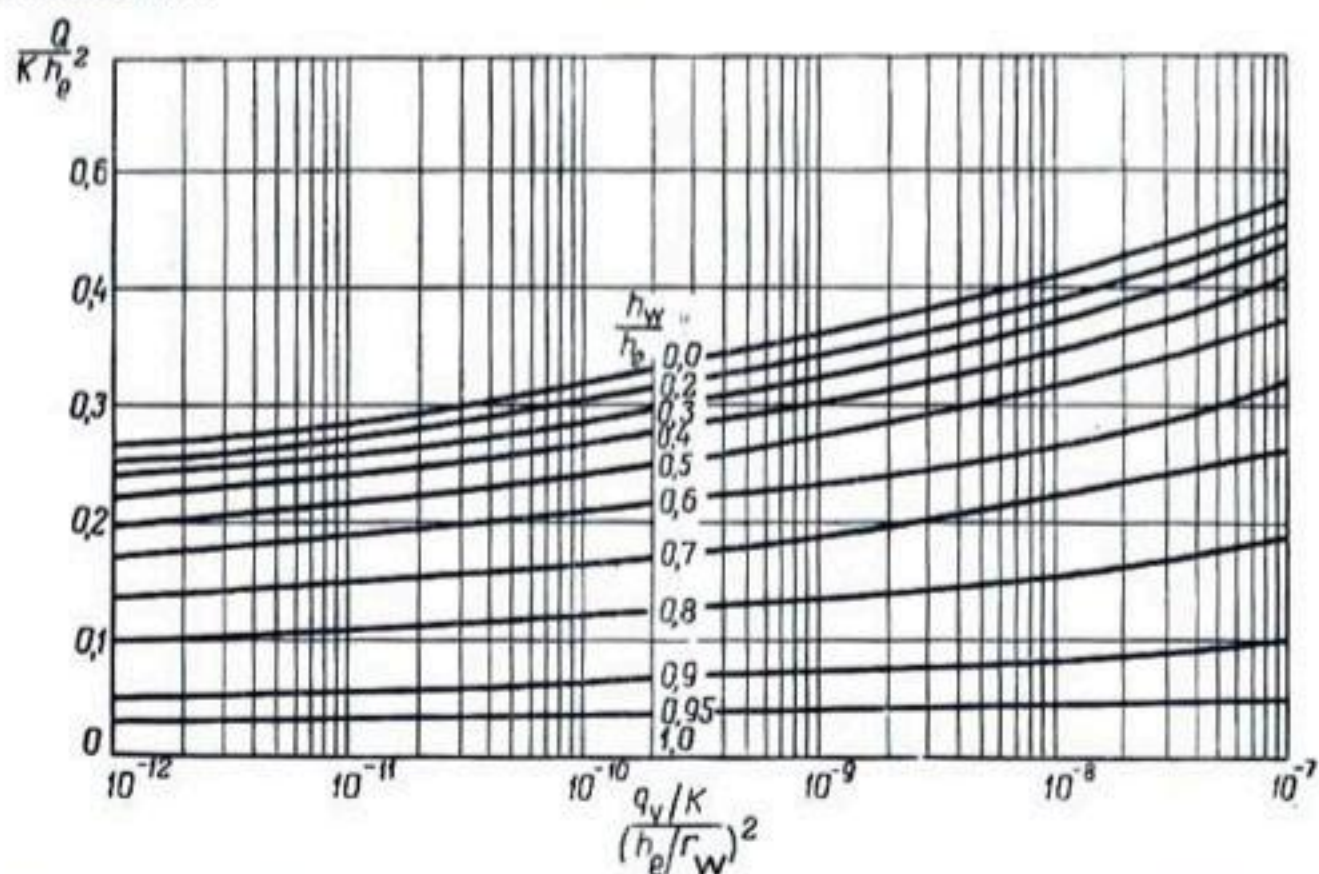
Рис. 103. Параметры расхода для вертикально пополняемого неограниченно- го грунтового потока (продолжение рис. 102 влево, масштаб по вертикаль- ной оси увеличен).
