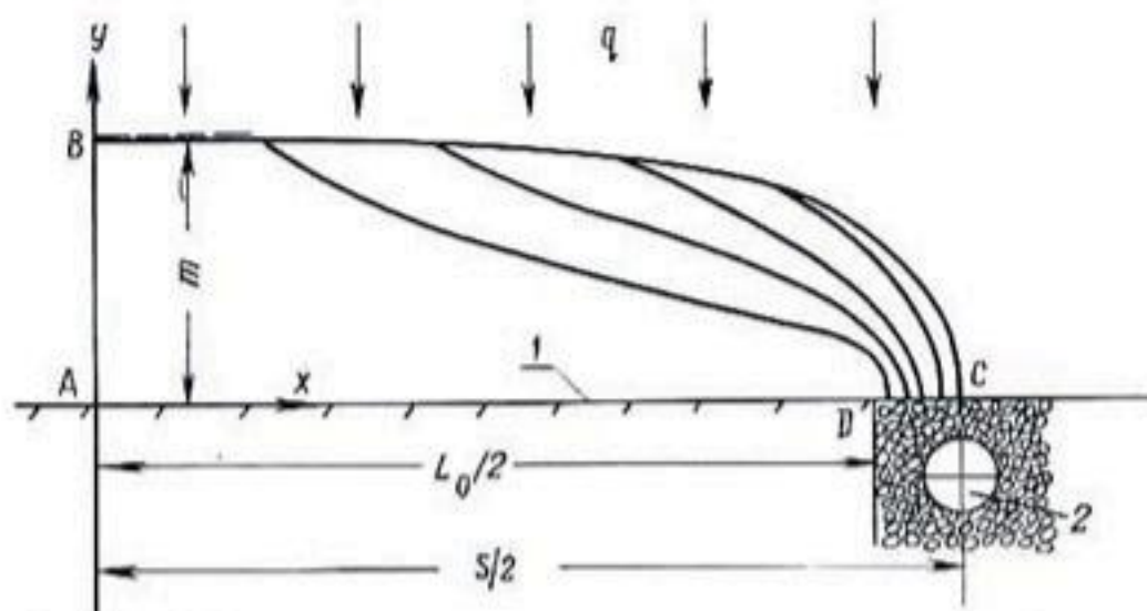
Рис. 123. Дрены, уложенные в непроницаемом слое. Равномерная инфильтрация q с поверхности почвы. По Энгелунду (1951):
