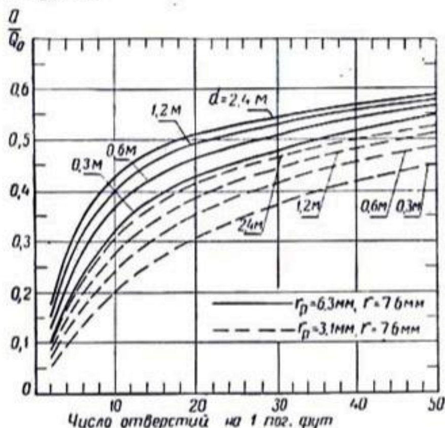
Рис. 140. Зависимость относительного притока от перфорации дренажных труб;
