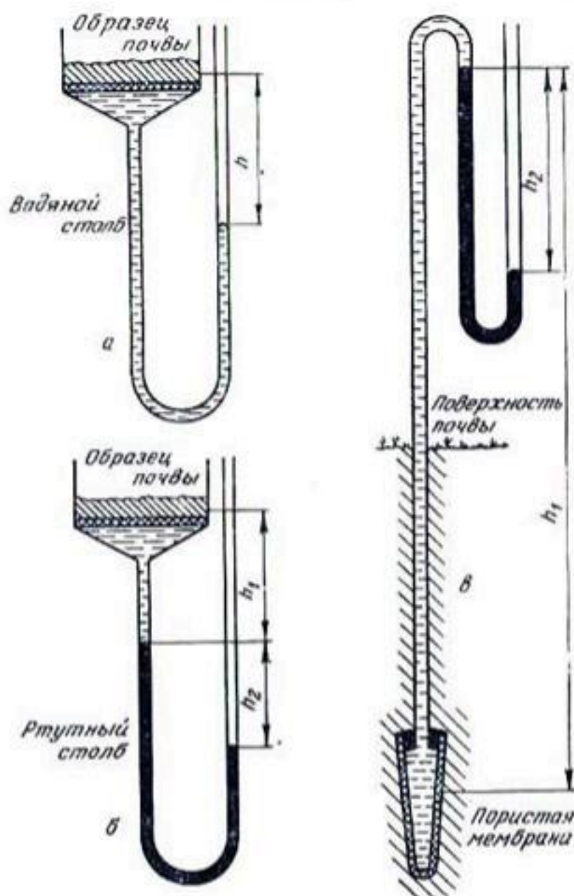
Рис. 3. Приборы для измерения всасывания:
