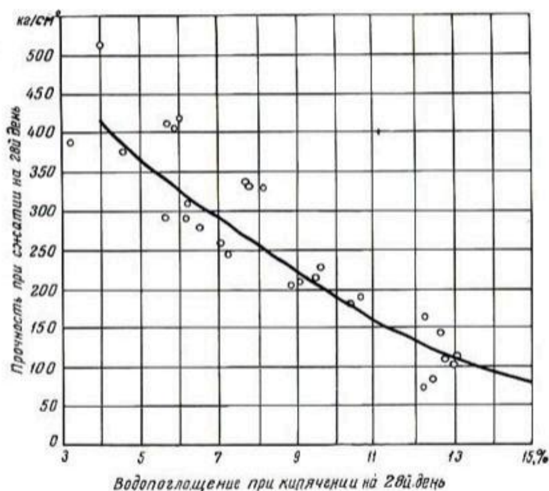
Рис. 151. Зависимость между прочностью и водопоглощением трамбованных цилиндров размером 5,1 \times 10,2 см с различной степенью уплотнения. Состав смеси 1 : 3 (такой состав применяется на предприятиях, изготавливающих трубы).
