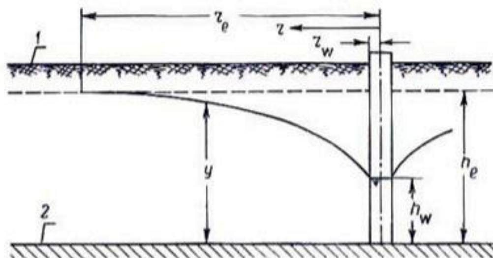
Рис. 95. Чертёж колодца Дююи:
