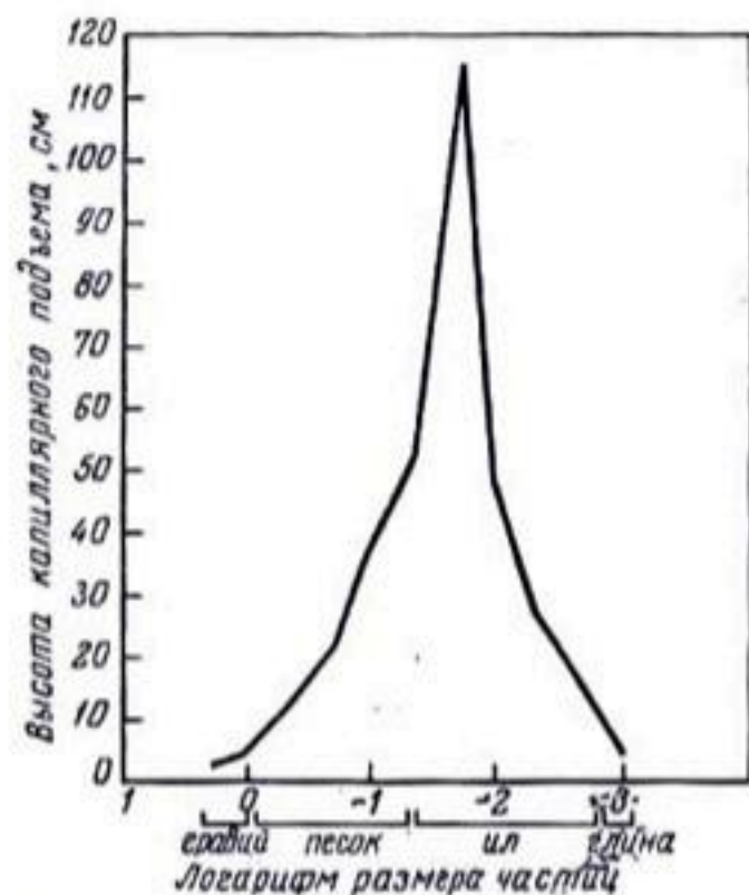
Рис. 229. Зависимость скорости капиллярного подъема воды от размера частиц при 17° С.
