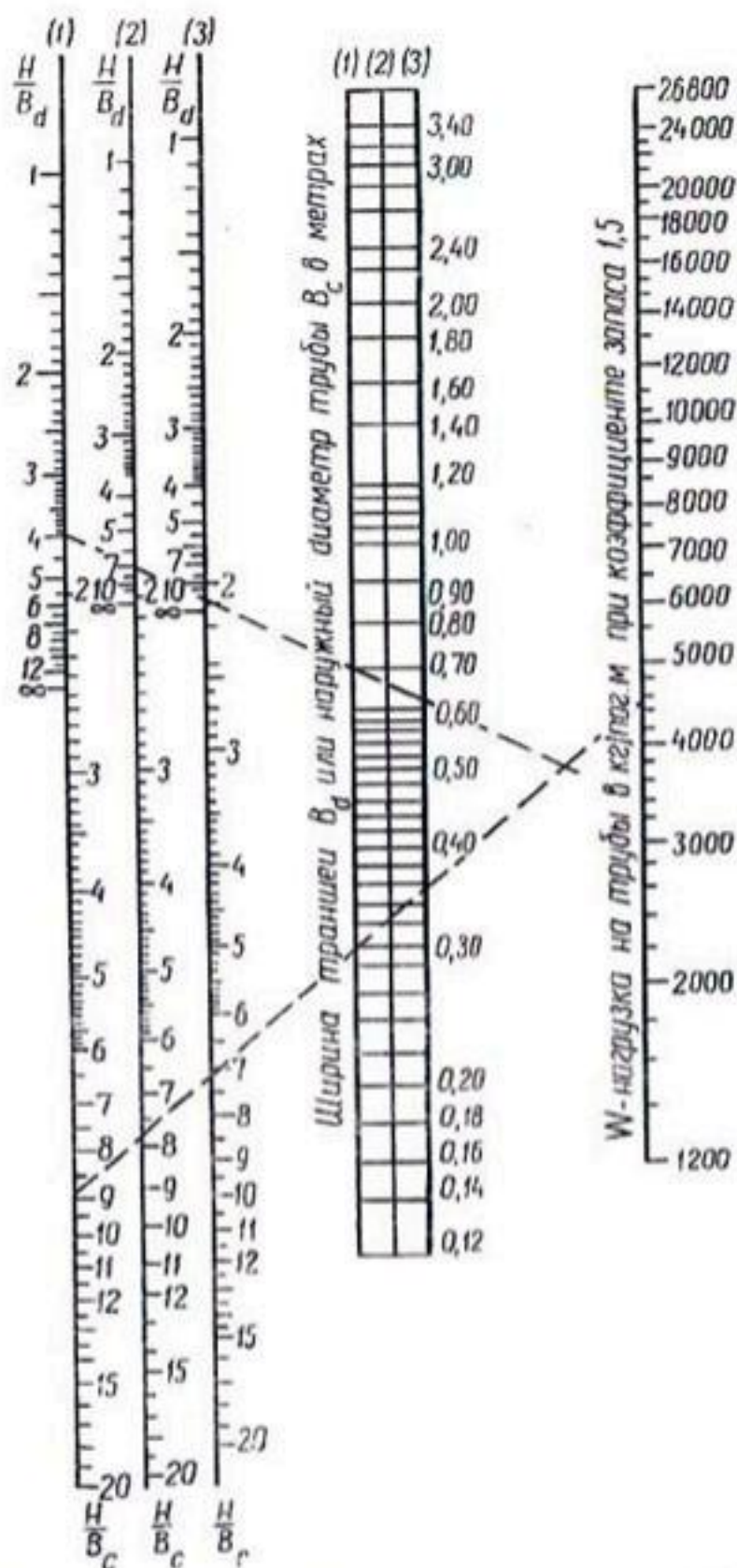
Рис. 145. Номограмма для определения нагрузок на трубы в траншеях по формулам Марстона.
