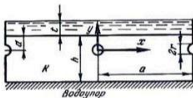
Рис. 78. Ряд труб, расположенных на одинаковом расстоянии друг от друга в грунте со скопившейся водой, который залегает на непроницаемом слое (водоупоре).
