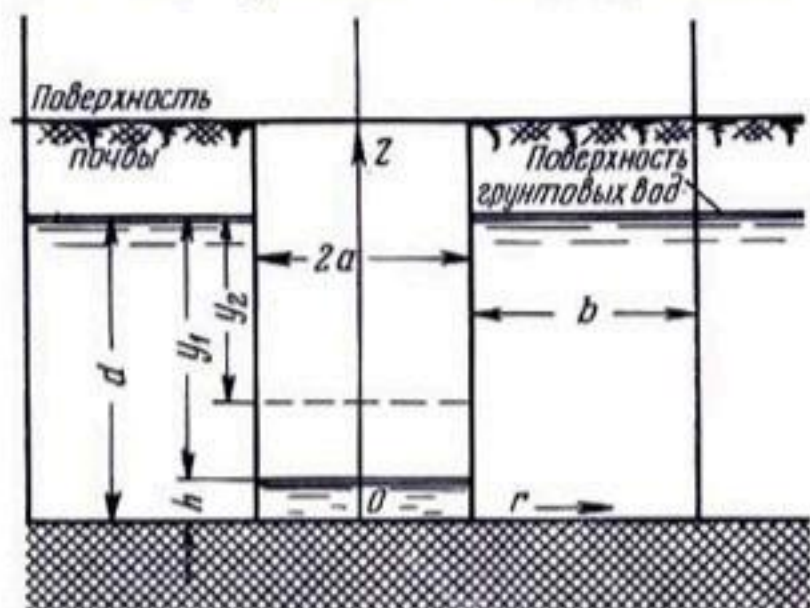
Рис. 189. Чертеж скважины, используемый при выводе формулы Киркхема (метод скважины в однородном грунте) 1 .
