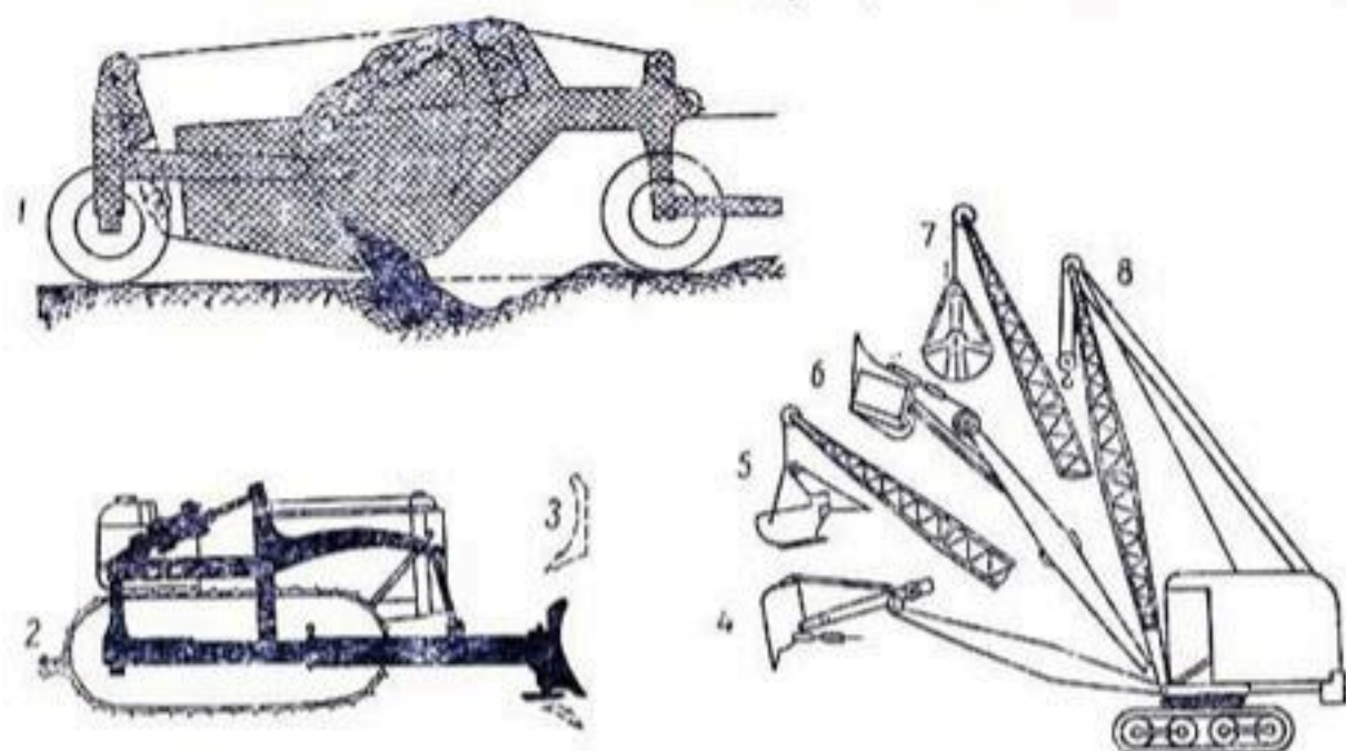
Рис. 136. Машины для выемки грунта при строительстве открытых каналов:
