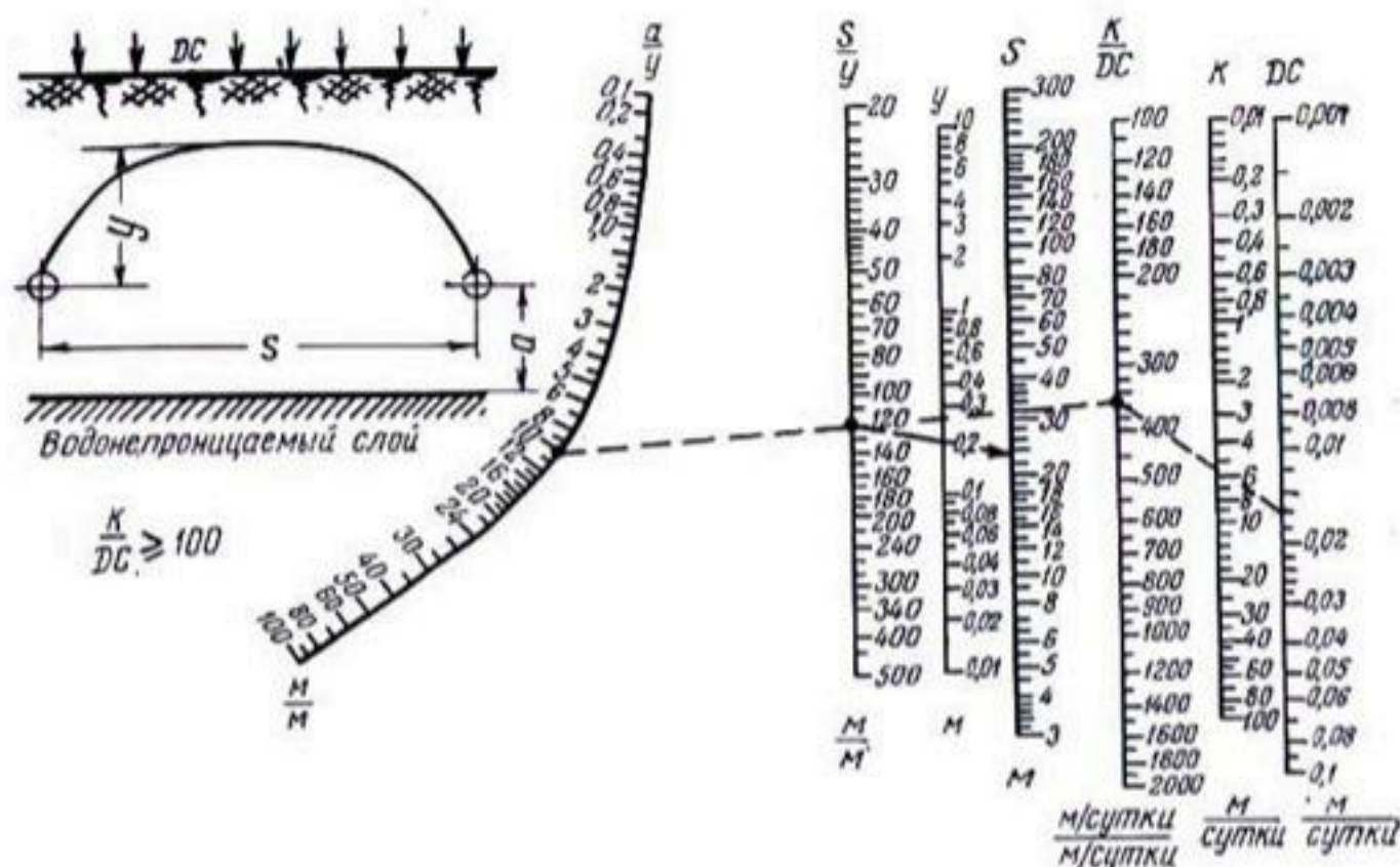
Рис. 174. Номограмма для определения расстояния между гончарными дренами при K/DC \geq 100 (по Виссеру). Все обозначения, как на рисунке 173.
