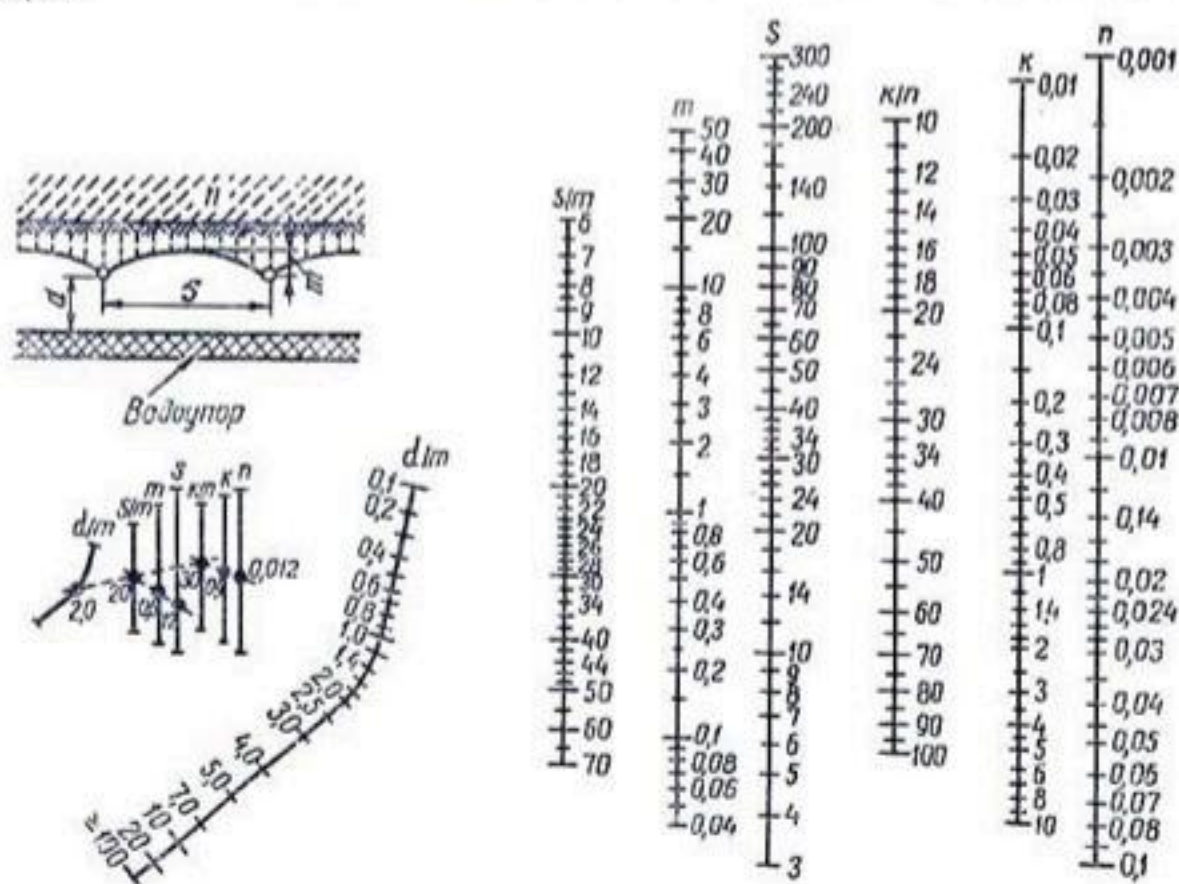
Рис. 37. Номограмма для определения расстояний между дренами при k/n \leq 100 (по Виссеру, 1954):
