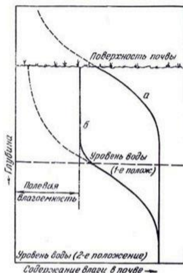
Рис. 11. Профили почвенной влажности при понижении уровня воды: а — 1-е положение (более ранняя стадия); б — 2-е положение (более поздняя стадия).
