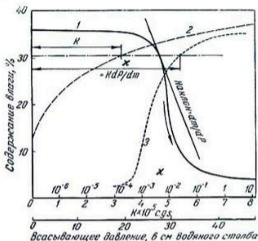
Рис. 25. Определение коэффициента диффузии почвенной влаги по гидравлической проводимости и характеристике влажности при данном содержании влаги:
