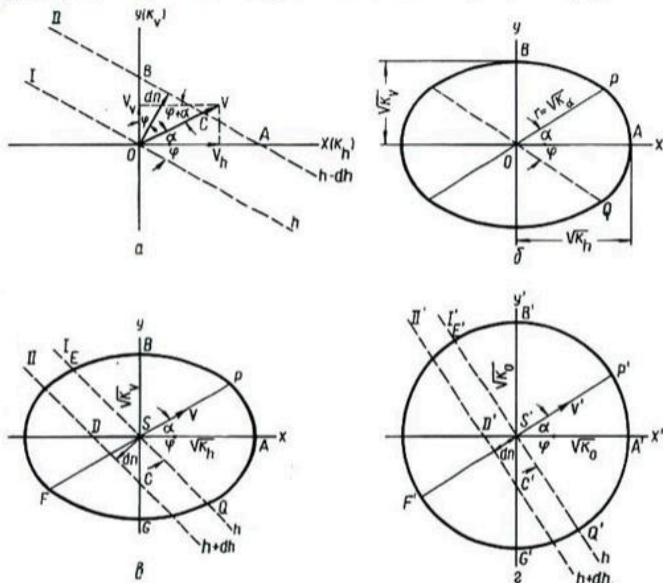
Рис. 114. Двухмерный поток в анизотропной среде:
