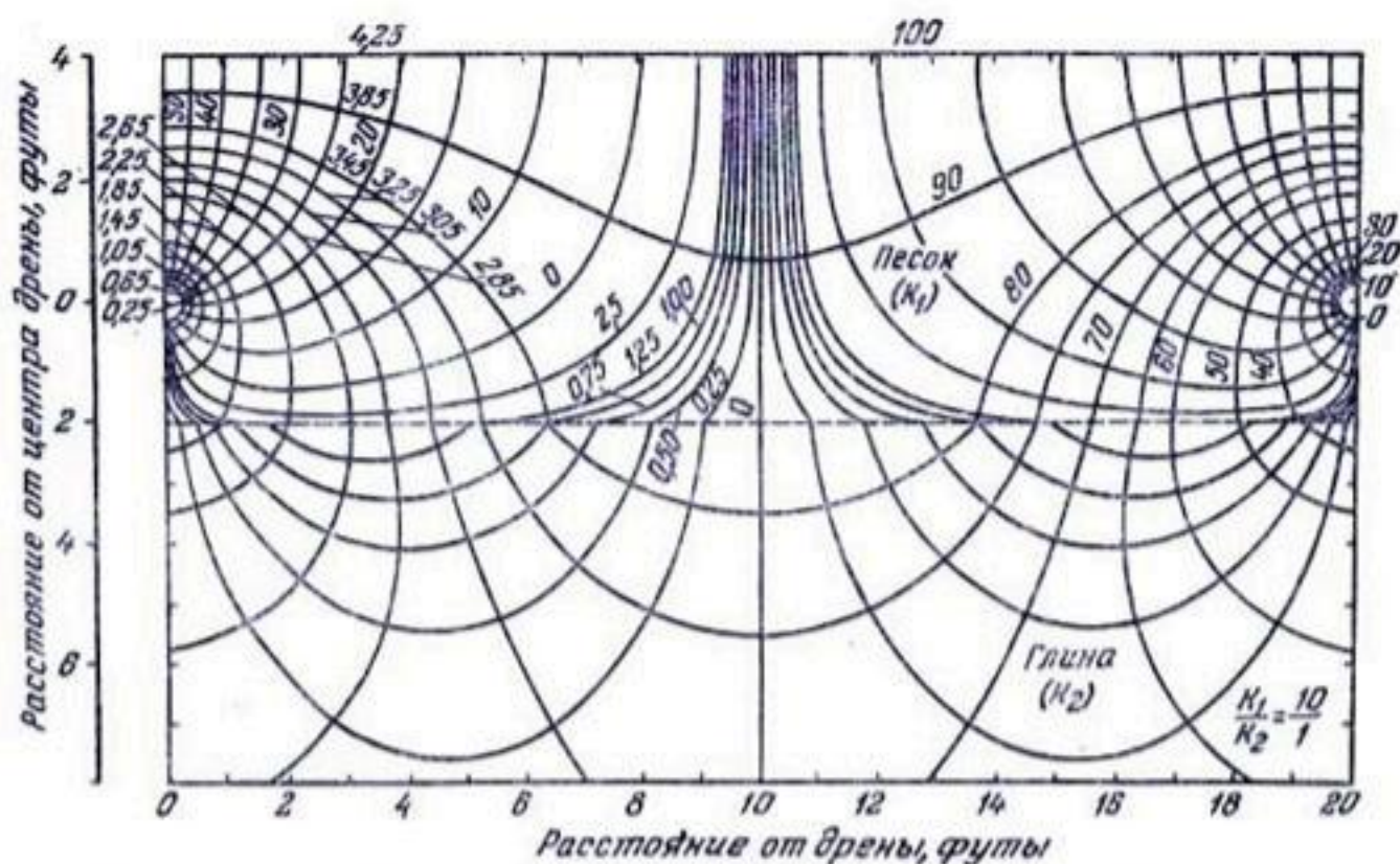
Рис. 83. Сетка токов для дренажных труб, показанных на рисунке 82. Величины гидравлического напора 4,25; 3,85 и т. д., показанные слева, относятся к поверхностному слою скопившейся воды глубиной 0,25 фута. По Киркхему (1951).
