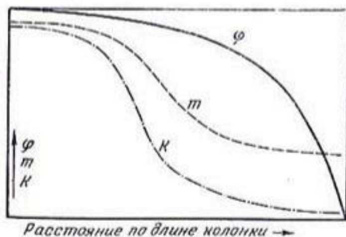
Рис. 23. Изменение содержания влаги ( m ), гидравлической проводимости ( k ) и потенциала ( \phi ) вдоль колонки гипотетической ненасыщенной почвы, пропускающей постоянный поток воды.
