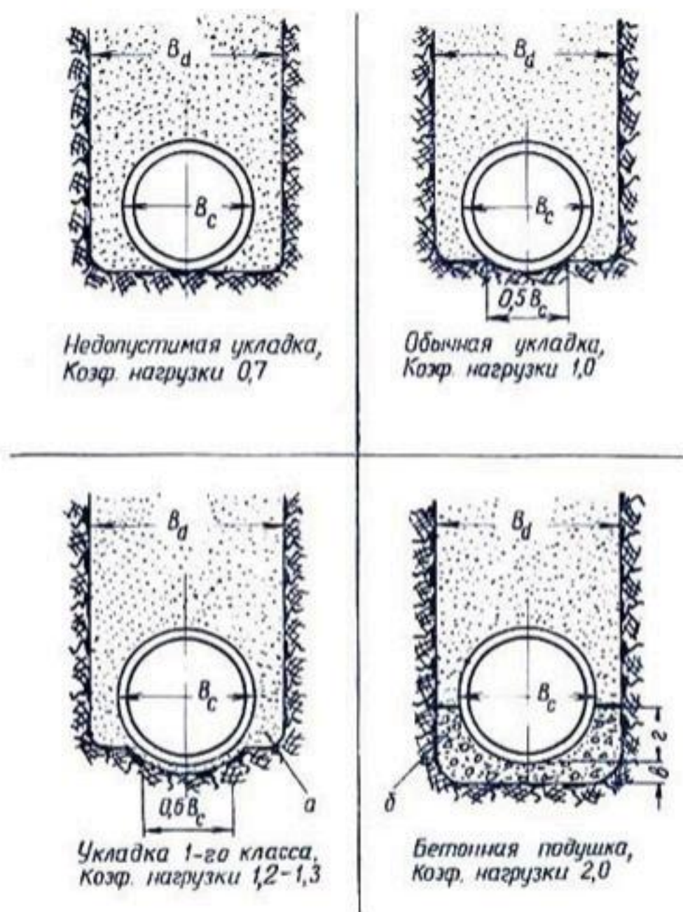
Рис. 144. Типы укладки труб в траншеях:
