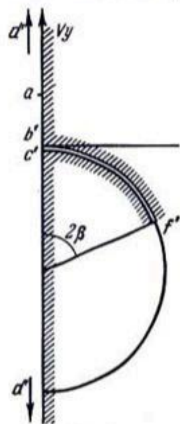
Рис. 58. Плоскость годографа.
