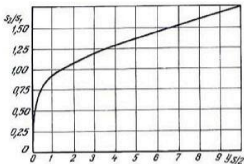
Рис. 39. График изменения соотношения расстояний, определенных по двум уравнениям Гловера, в случае расположения дрен на непроницаемом слое и при падении уровня грунтовых вод на один фут (0,3 м).
