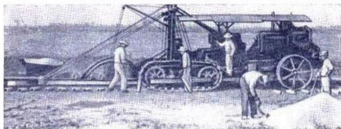
Рис. 162. Трубоукладочная машина в работе.
