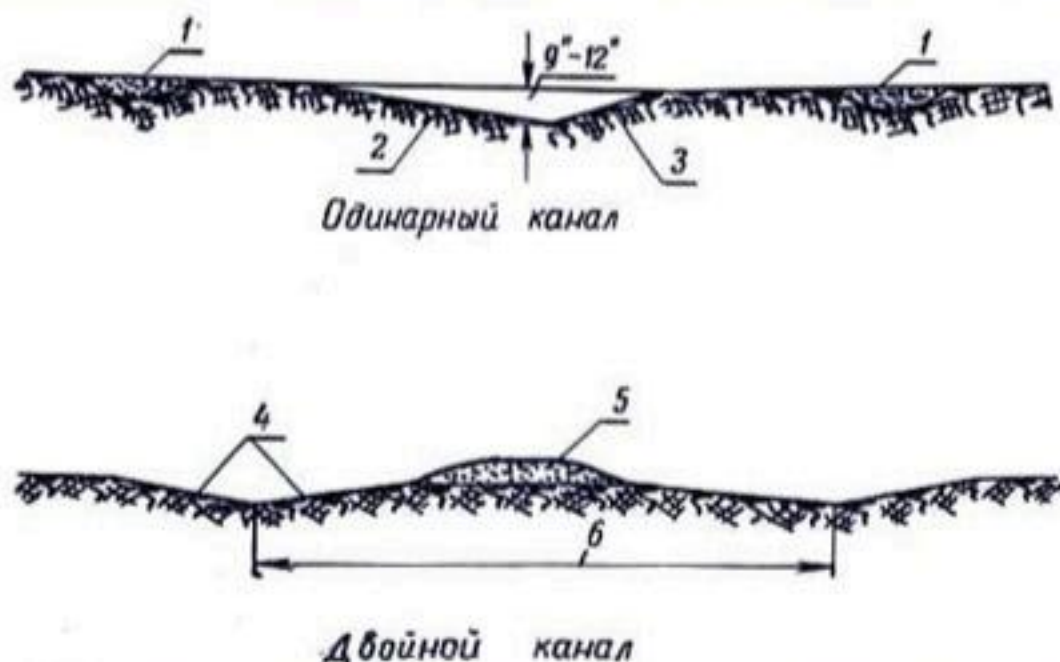
Рис. 168. Поперечные сечения полевых каналов для поверхностного дренирования (площадь сечения одинарного канала 0,5–0,7 м 2 ):
