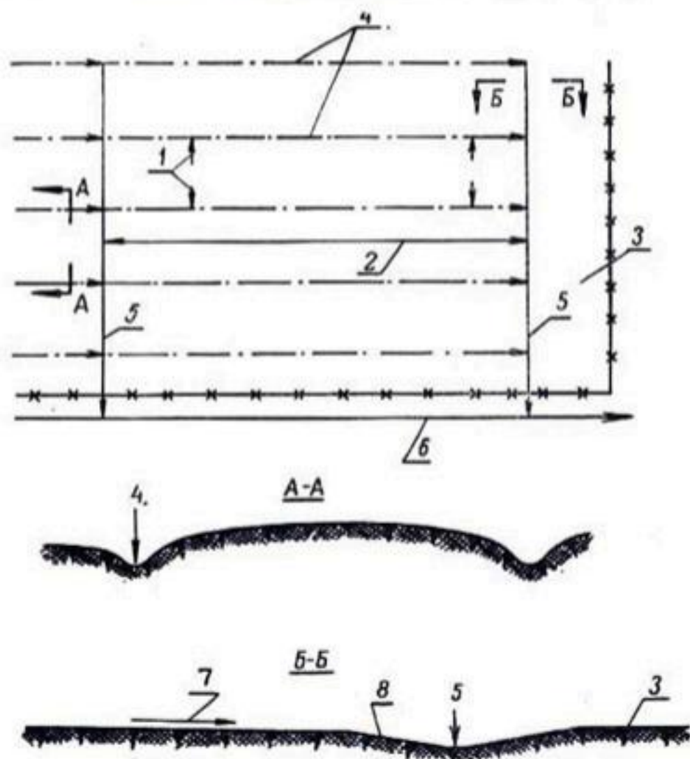
Рис. 166. Расположение дренажных канав и поперечные сечения гряд:
