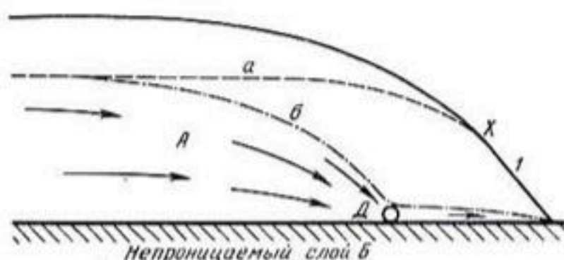
Рис. 28. Поверхность грунтовых вод в случае притока слева, обуславливающего необходимость дренажа у поверхности выклинивания I : a — поверхность грунтовых вод до установки дрены D ; b — поверхность грунтовых вод после установки дрены D .
