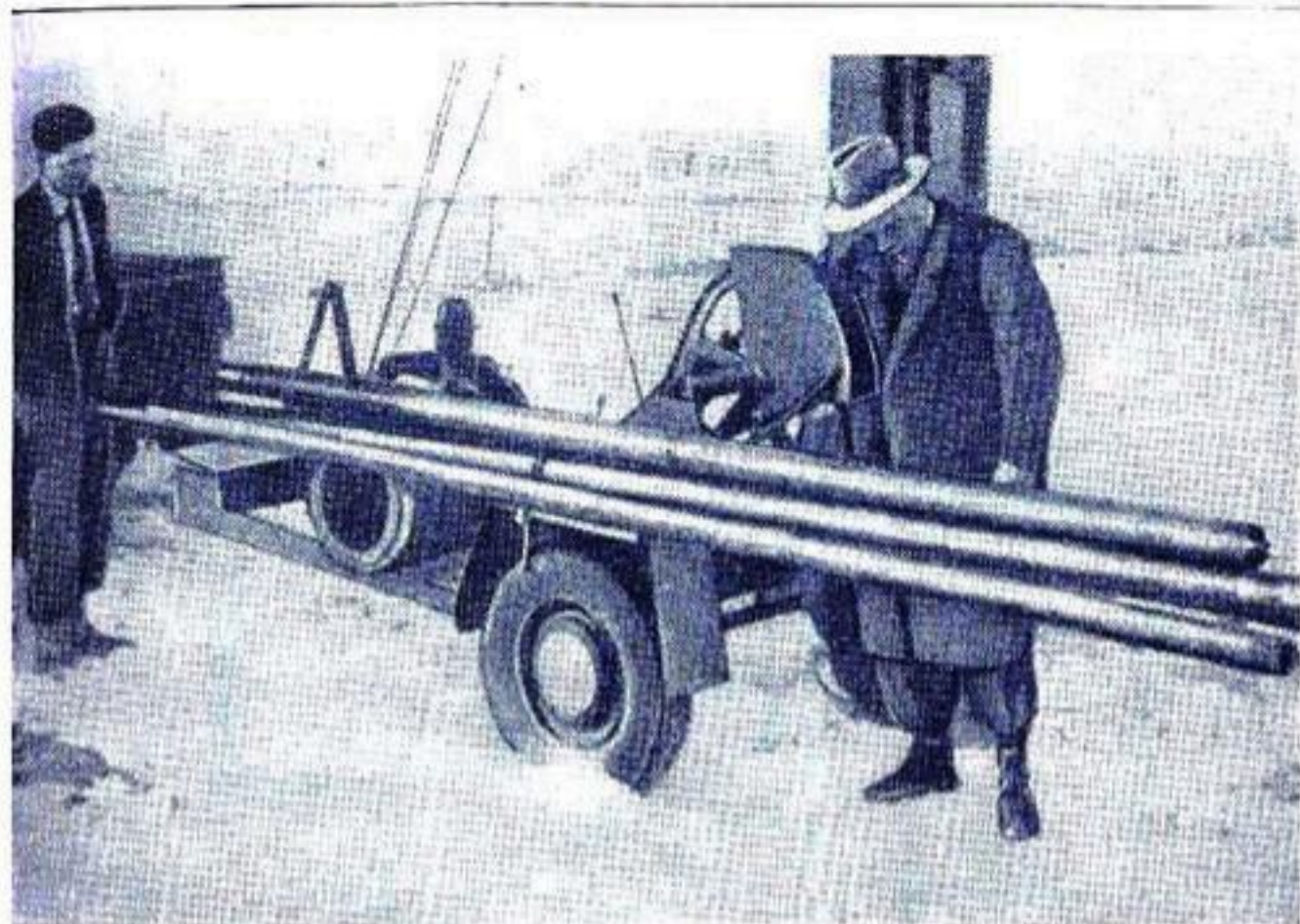
Рис. 183. Механизируемый бур для взятия почвенных монолитов. По Келли (1948).
