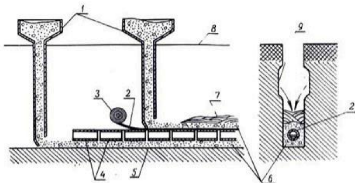
Рис. 152 и 153 (продольный и поперечный разрезы). Трубы, уложенные с гравийным фильтром и с защитным слоем просмоленной бумаги: 1 — воронка для засыпки гравия; 2 — защитный слой просмоленной бумаги; 3 — рулон просмоленной бумаги; 4 — дренажные трубы; 5 — дно траншеи; 6 — гравийная оболочка (фильтр); 7 — заполняющий грунт; 8 — поверхность почвы; 9 — заполнение из наиболее проницаемых слоев грунта.
