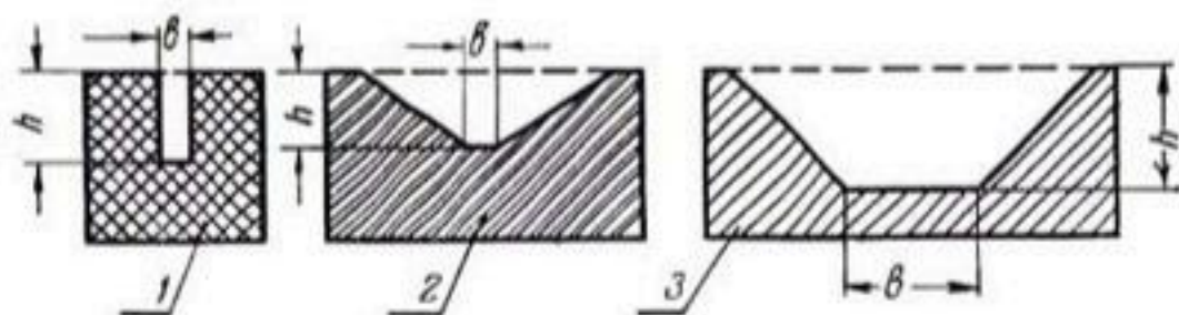
Рис. 171. Поперечные сечения каналов для регулирования уровня грунтовых вод (указаны минимальные размеры и уклоны). По Бошам:
