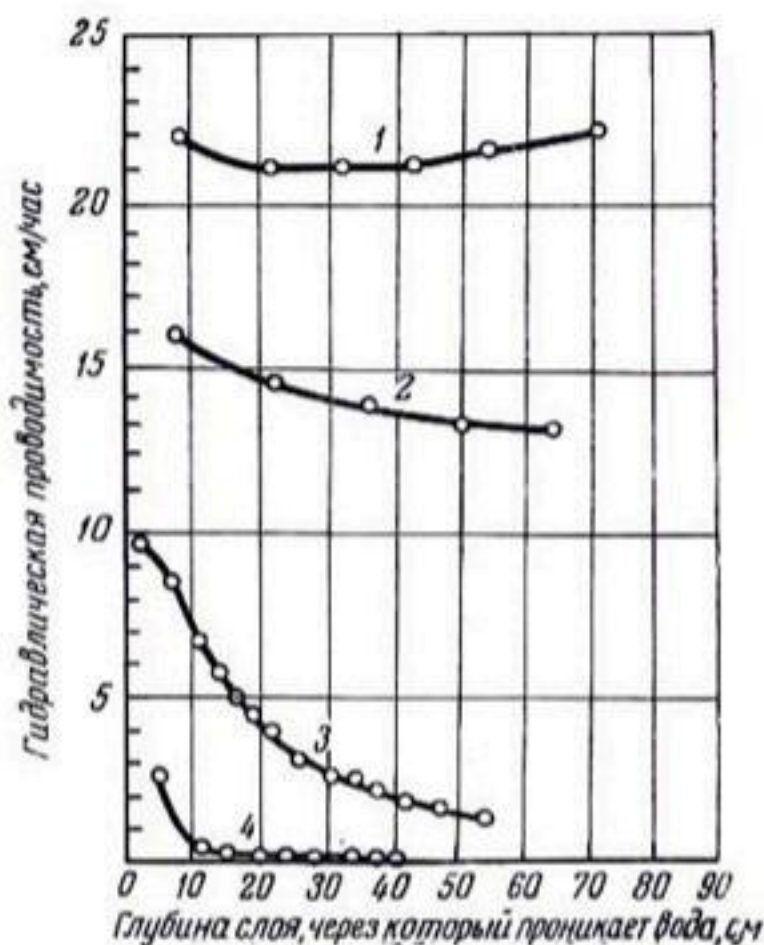
Рис. 176. Влияние состава воды на проницаемость супесчаных почв. По Файерману (1944): 1 — хлористый кальций (800 частей на миллион); 2 — смесь солей (280 частей на миллион) в водопроводной воде; 3 — хлористый натрий (4500 частей на миллион); 4 — дистиллированная вода.
