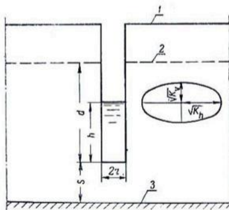
Рис. 132. Буровая скважина в анизотропном грунте ( k_h/k_v=4 ):
