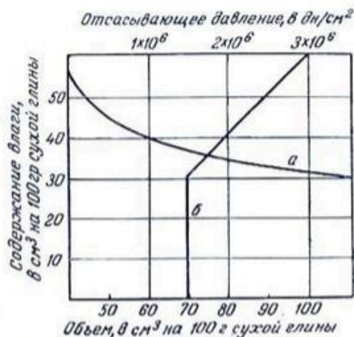
Рис. 10. Характеристика влажности (а) и кривая усадки образца каолина (б).
