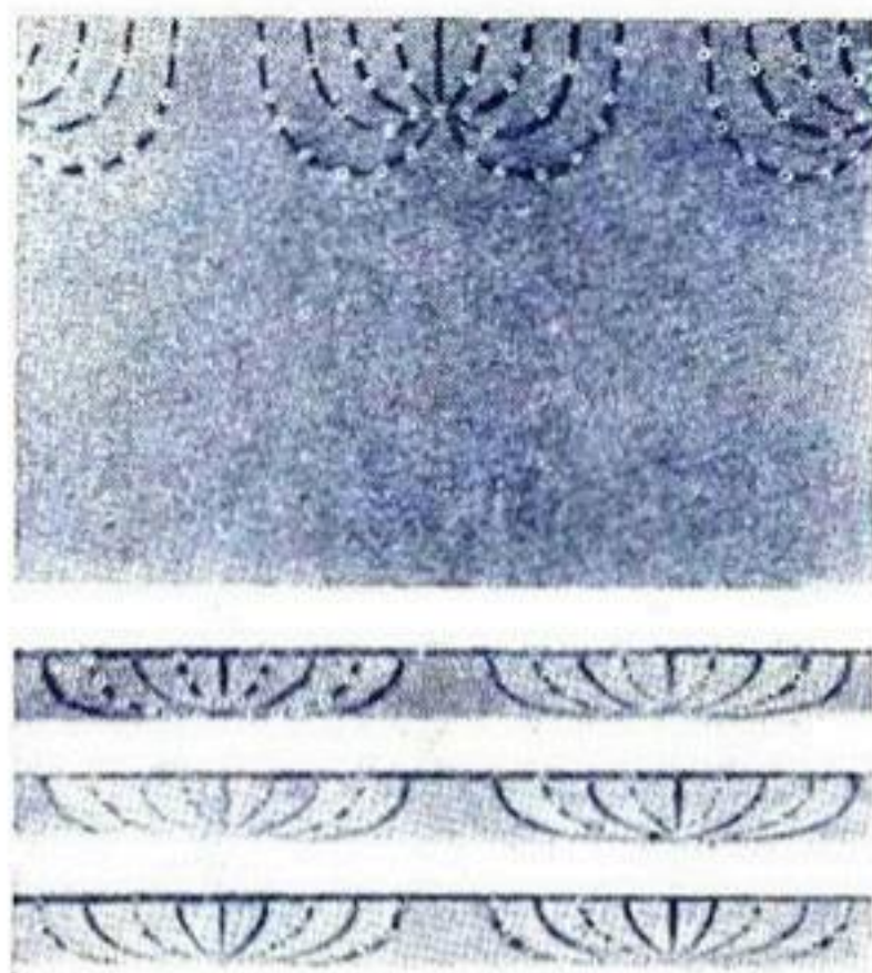
Рис. 81. Сравнение опытных и теоретических линий тока, соответствующих случаям, когда поверхность водоупора находится на большой и малой глубине. Белые кружочки соответствуют теоретическим решениям и нанесены на линии тока, полученные путем фотографирования их в резервуаре с песком (стенка резервуара стеклянная). По Киркхему (1941).
