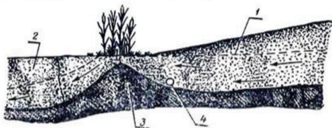
Рис. 157. Дренаж при наличии непроницаемого барьера: 1 — поверхность грунтовых вод; 2 — песчаный суглинок; 3 — глиняный барьер; 4 — местоположение дрены.
