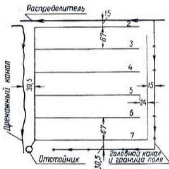
Рис. 158. Типовая дренажная система в долине Импириал, штат Калифорния (размеры на чертеже даны в метрах).
