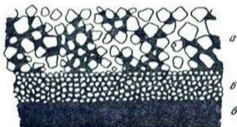
Рис. 2. Пористая мембрана б обеспечивает неразрывность между водой в почвенном образце а и внешней водной средой в, находящейся под действием всасывания.
