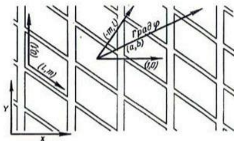
Рис. 19. Идеализированная система трещин структурной почвы. Выражения в скобках являются косинусами указанных направлений.
