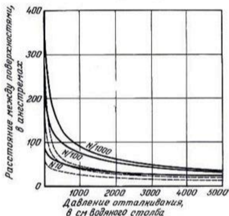
Рис. 8. Давление отталкивания между монтмориλλονитовыми пластинками, показанными на рисунке 7, как функция расстояния между этими пластинками. Сплошные кривые построены для кристаллов в растворах одновалентных ионов указанных концентраций. Штриховые кривые — для двухвалентных ионов таких же трех концентраций. Во избежание путаницы показатели концентраций опущены, но они расположены в том же порядке, как и на кривых для одновалентных ионов.
