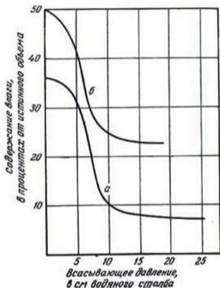
Рис. 9. Характеристики влажности:
