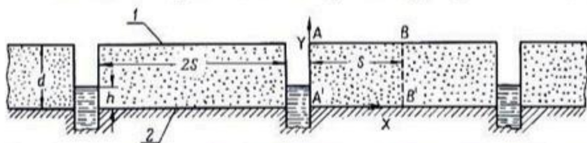
Рис. 92. Чертеж к задаче просачивания воды из водонасыщенной почвы в каналы, расположенные на одинаковом расстоянии друг от друга и врезающиеся в непроницаемый слой. По Киркхему (1950b): 1 — поверхность почвы; 2 — поверхность водоупора.
