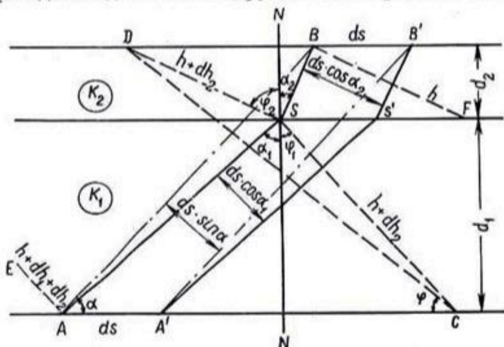
Рис. 116. Произвольно направленный линейный поток через два слоя с различными коэффициентами фильтрации.
