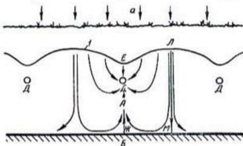
Рис. 26. Поверхность грунтовых вод I поддерживается на определенном уровне за счет устойчивых осадков a , выпадающих на водопроницаемый слой Л при наличии в нем дрен Д . Стрелки указывают приблизительное направление движения грунтовых вод к дренам.
