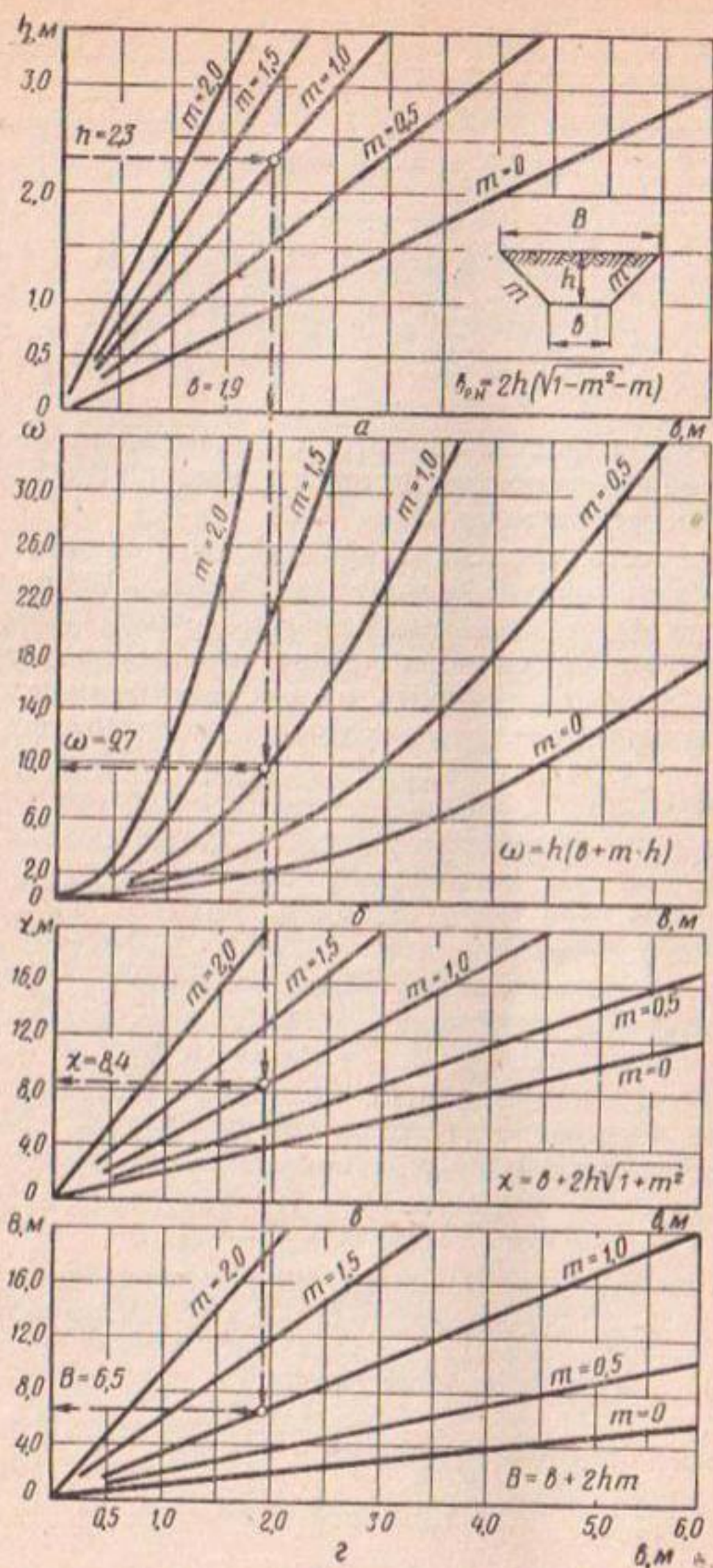
Рис. 18. Номограммы для определения параметров гидравлически наилучших сечений каналов: а — ширины канала по дну в м при глубине воды в канале h , м; б — живого сечения \omega , \text{м}^2 ; в — смоченного периметра \chi , м; г — ширины канала по поверхности воды B , м. При заложении откосов: m=0 , m=0.5 , m=1.0 , m=1.5 , m=2.0 .
