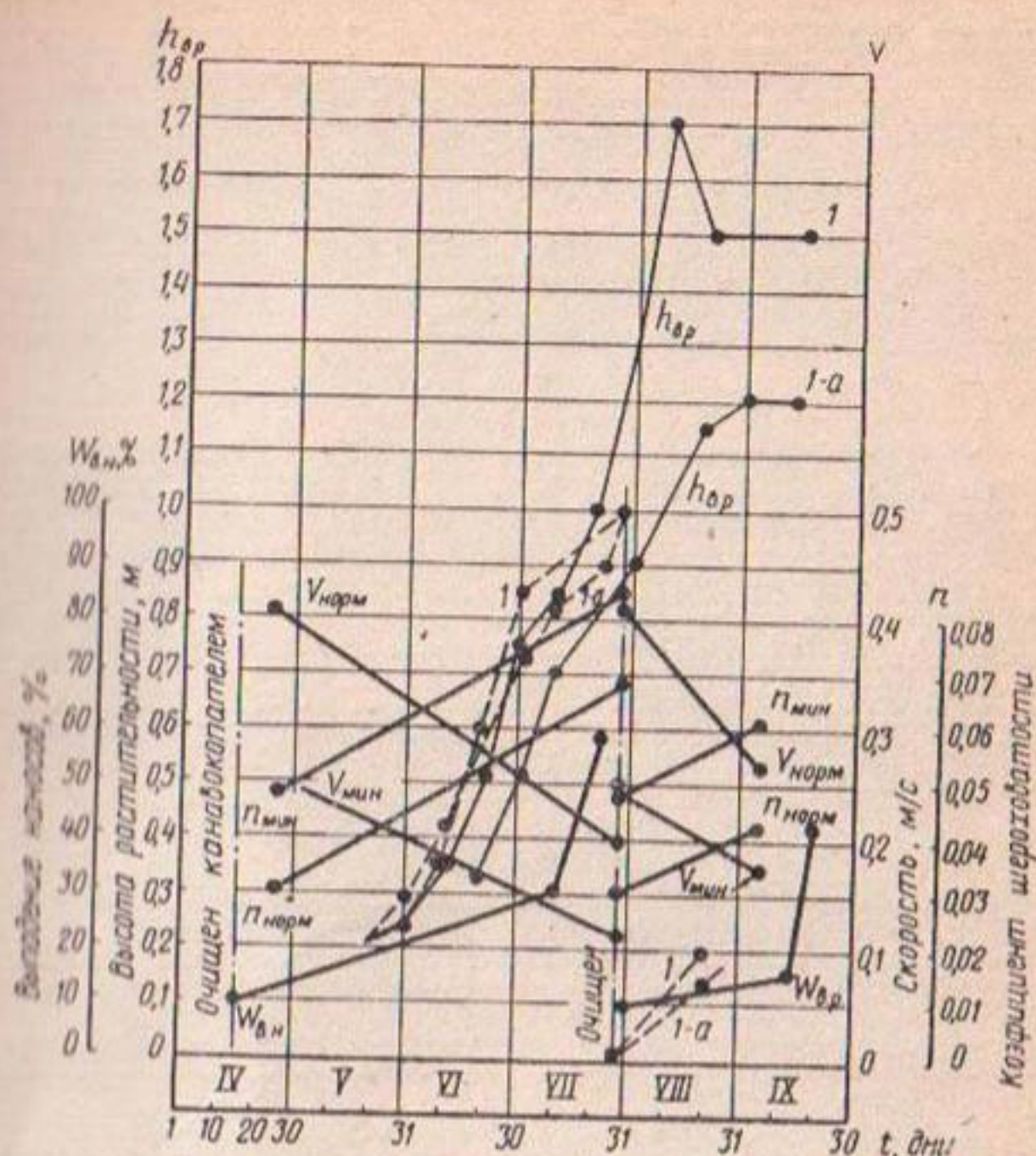
Рис. 11. Коэффициенты шероховатости n , скорости течения V и выпадение наносов W_{\text{нн}} . Канал Подкумок-Юца при зарастании растительностью (1967—1968 гг.):
